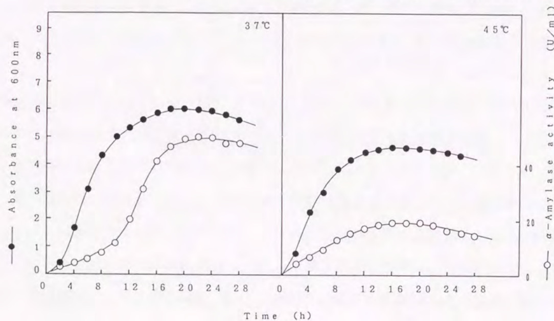
図6-5. B. subtilis NA-1/pTBA530の37 および45℃での菌体増殖と酵素生産。培養はカナマイシン5 \mu g/mlおよびテトラサイクリン20 \mu g/mlを含む培地で行った。培養上清は酵素活性測定に供した(○)。菌体増殖(●)は、600nmの吸収で測定した。
