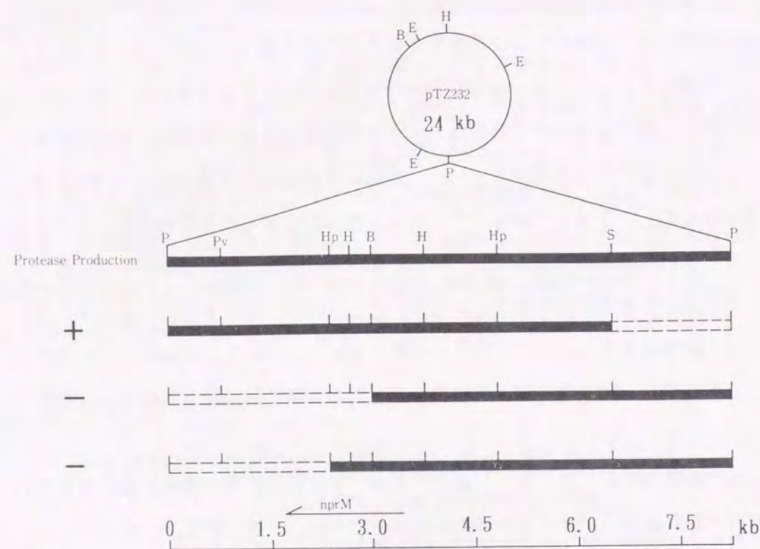
図2-1. プラスミドpTZ232およびその誘導体の制限酵素地図。黒太線は B. stearothermophilus MK232 由来 DNA。破線は欠失部分を示す。制限酵素部位の Bam H I、 Eco R I、 Hin d III、 Hpa I、 Pst I、 Pvu II、および Sa I はそれぞれ B、E、H、Hp、P、Pv、および S で示す。nprM 遺伝子の位置と転写方向は矢印で示す。
