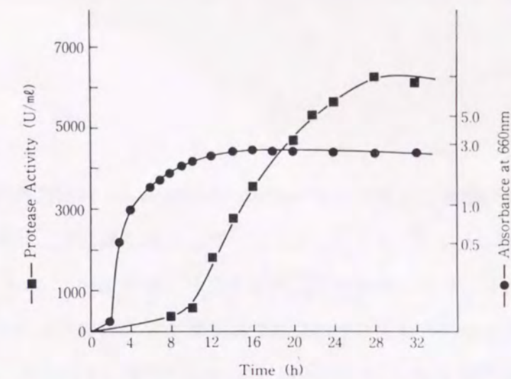
図2-7. pMK1を保持する B. subtilis MT-2の菌体増殖とプロテアーゼ生産における経時変化。培養は5 \mu g/mlのカナマイシンを含むL培地を用い37℃で行った。菌体増殖は●、培養液中の酵素活性は■、で示す。
