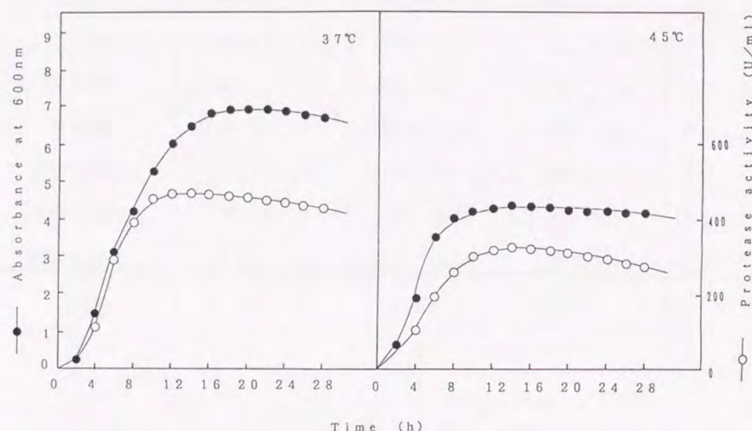
図6-4. B. subtilis MT-2/pNP22の37 および45℃での菌体増殖と酵素生産。培養はカナマイシン5 \mu g/mlを含む培地で行った。培養上清は酵素活性測定に供した(○)。菌体増殖(●)は、600nmの吸収で測定した。
