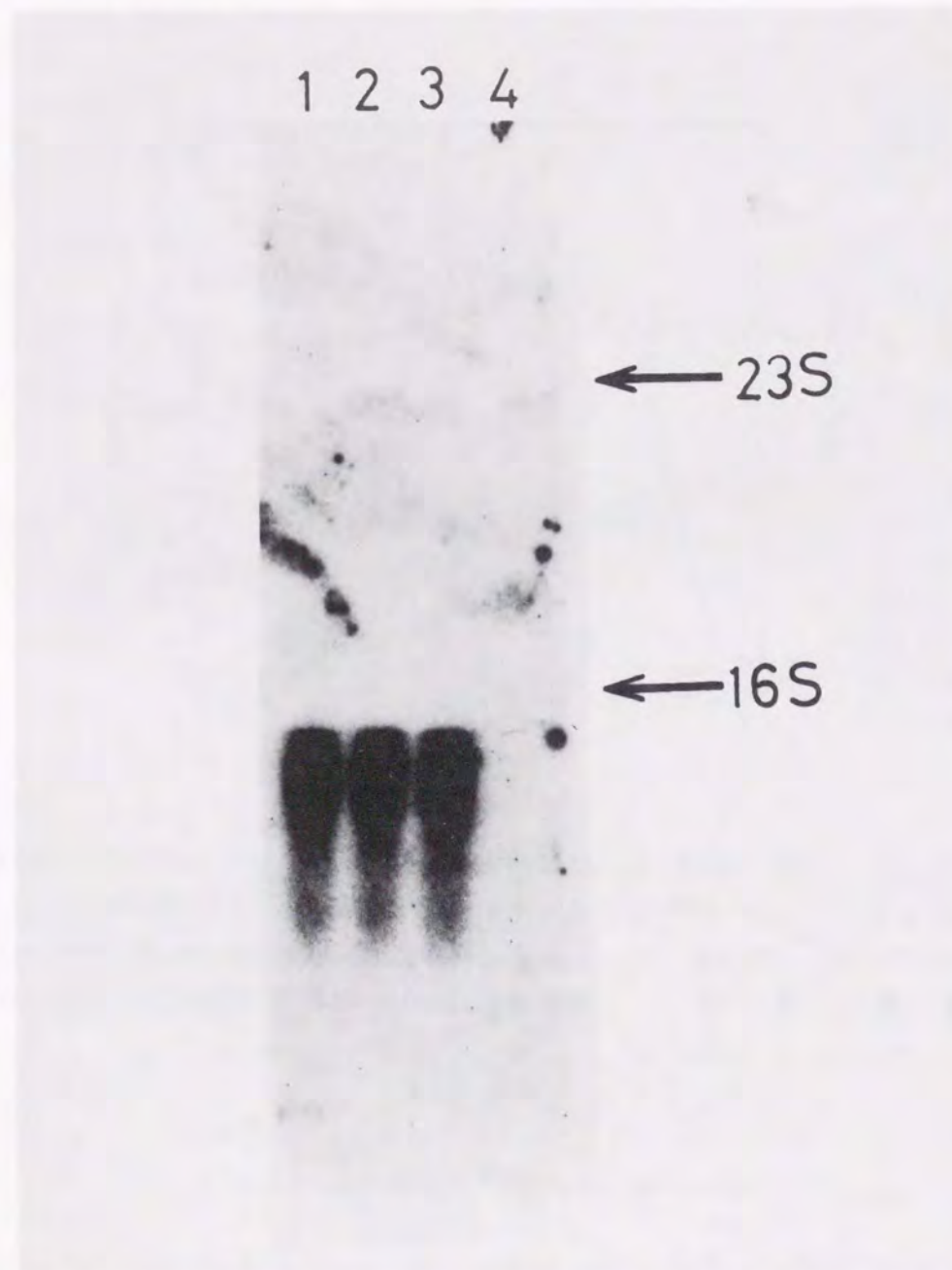
図3-3. nprM およびその変異遺伝子のノーザンブロット解析. nprM 遺伝子の Bam H I - Hpa I 断片(1,210bp)をハイブリダイゼーションプローブとして用いた. レーン1: B. subtilis MT-2/pMK1 から調製したRNA、2: B. subtilis MT-2/pMK2 から調製したRNA、3: B. subtilis MT-2/pMK3 から調整したRNA、4: B. subtilis MT-2/pTB51から調製したRNA. 16S 及び23S RNA の位置を矢印で示す.
