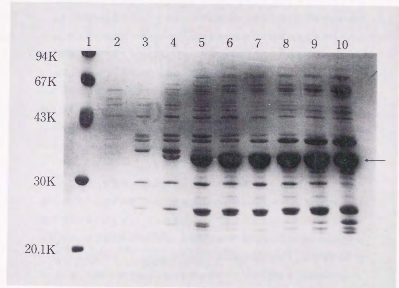
図2-8. B. subtilis MT-2/pMK1 の培養上清のSDS ポリアクリルアミドゲル電気泳動。レーン1:標準蛋白質マーカー (94.0K:phosphorylase b, 67.0K:albumin, 43.0K:ovalbumin, 30.0K:carbonic anhydrase, 20.1K:trypsin inhibitor)。レーン2、3、4、5、6、7、8、9、および10は各培養時間のサンプル (4、6、8、10、12、14、16、20、および24時間)。K:kilodaltons。
