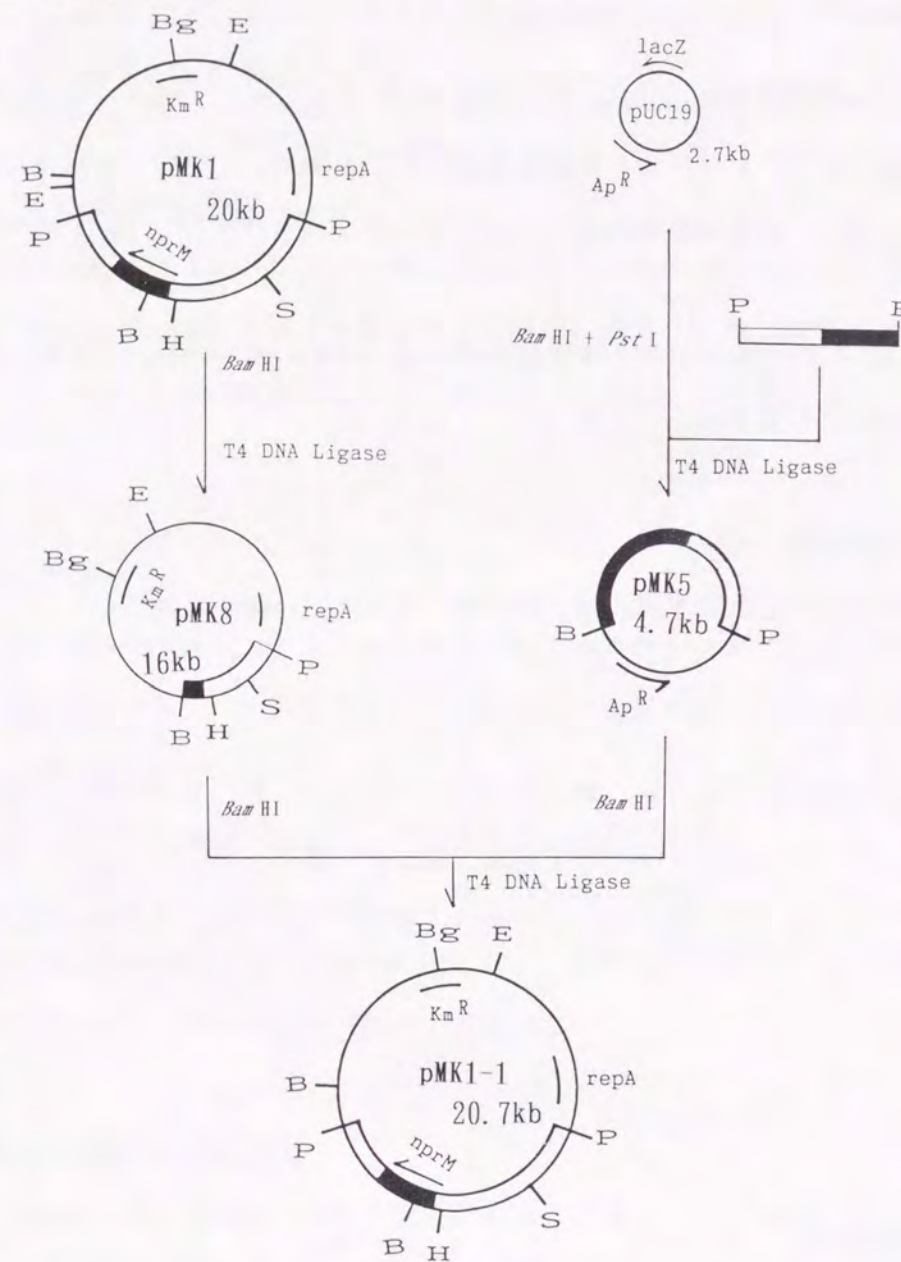
図5-2. プラスミドpMK8, pMK5, およびpMK1-1の構築。白と黒の太線は B. stearothermophilus MK232 由来DNAを示す。nprM 遺伝子の位置と転写方向を矢印で示す。制限酵素部位の Bam HI、Bgl II、Eco RI、Hind III、Pst I および Sal I はそれぞれB、Bg、E、H、PおよびSで示す。Kan, カナマイシン耐性遺伝子; Amp, アンピシリン耐性遺伝子; repA, プラスミドの複製開始点; lacZ, \beta -ガラクトシダーゼ遺伝子。
