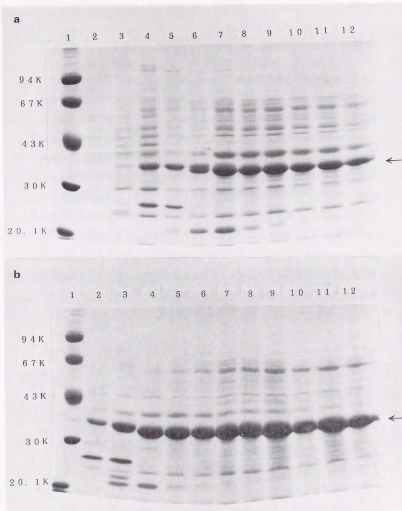
図6-2. B. subtilis MT-2/pMK1 の分泌する菌体外蛋白質のSDS-ポリアクリルアミドゲル電気泳動分析。 レーン1：標準蛋白質マーカー（94.0K: phosphorylase b, 67.0K:albumin, 43.0K:ovalbumin, 30.0K:carbonic anhydrase, 20.1K:trypsin inhibitor）。 K:kilodaltons。 レーン2～12は培養時間を示す（それぞれ4, 6, 8, 10, 12, 14, 16, 18, 20, 22, および24時間を示す）。 培養温度は、37℃（a）と45℃（b）である。 矢印はNprMを示す。
