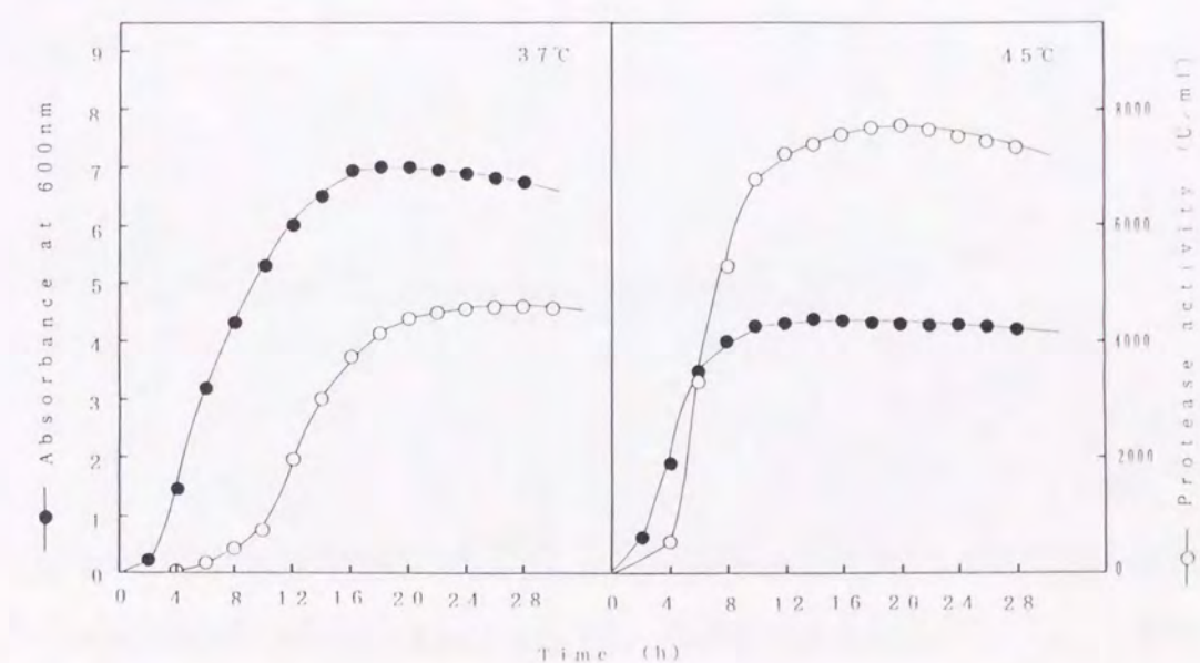
図6-1. B. subtilis MT-2/pMK1 の37 および45℃での菌体増殖と酵素生産。培養はカナマイシン 5 \mu\text{g}/\text{ml} を含む培地で行った。培養上清は酵素活性測定に供した（○）。菌体増殖（●）は、600nm の吸収で測定した。
