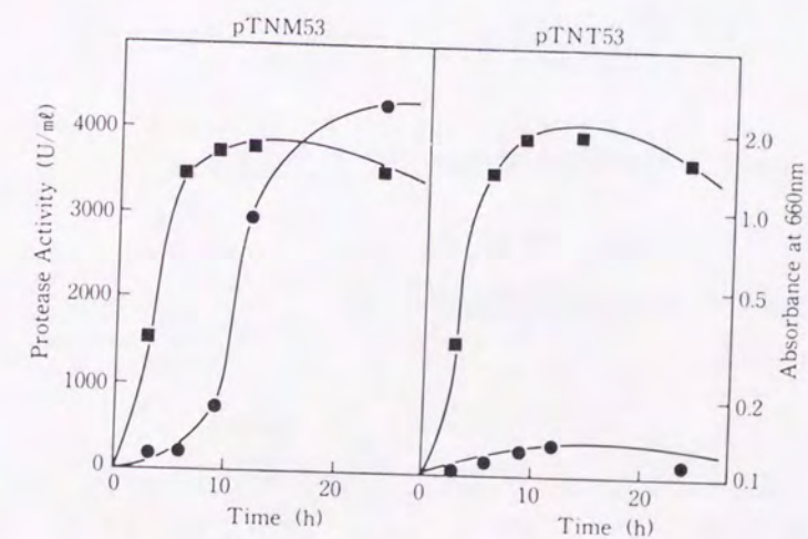
図2-5. pTNM53とpTNT53を保持する B. subtilis MT-2の菌体増殖とプロテアーゼ生産における経時変化。培養は20 μg/mlのテトラサイクリンを含むL培地を用い37℃で行った。培養液中の菌体増殖は■、酵素活性は●、で示す。
