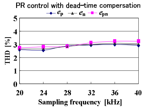
図 4.14 PR 制御のデッドタイム補償がある場合の負荷電圧の THD の測定結果
