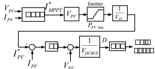
図 3.10 太陽電池用昇圧チョップの制御ブロック
