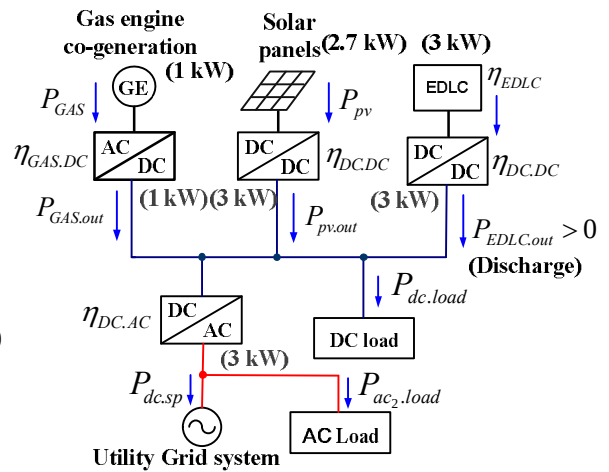
図 2.2 直流システム
