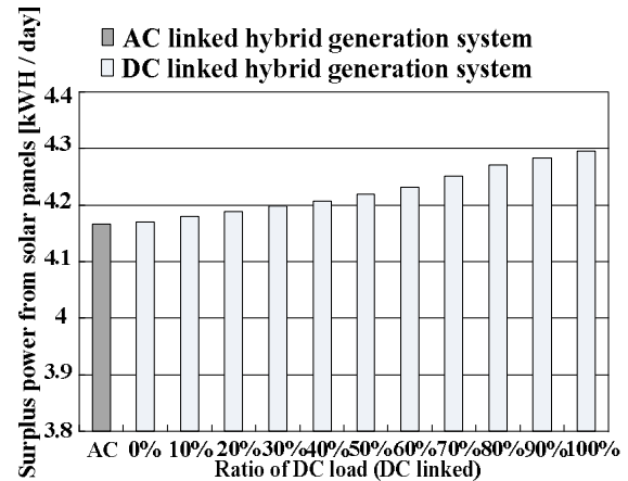
図 2.6 一日あたりの逆潮流電力量の計算結果
