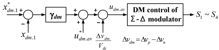
図 4.6 E- \phi 変調制御の DM 制御ブロック
