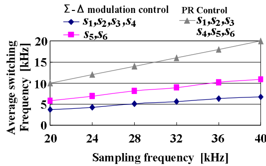
図 4.17 平衡負荷時の平均スイッチング周波数とサンプリング周波数の関係図
