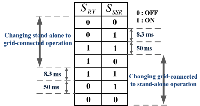
図 5.12 半導体リレー S_{SSR} と機械リレー S_{RY} の投入時間
