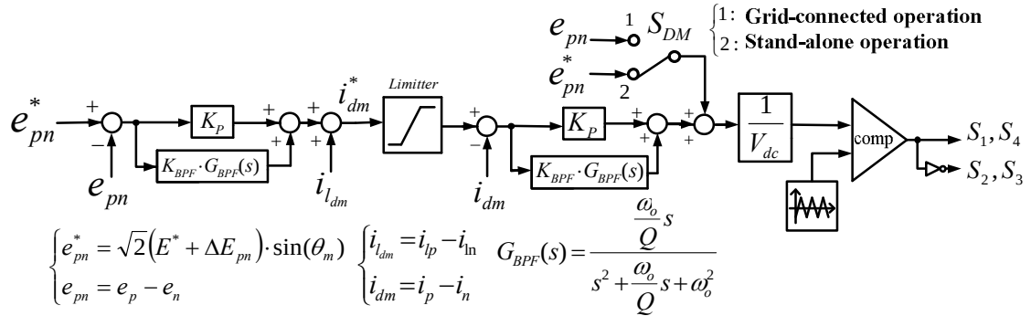
図 5.9 DM 制御ブロック
