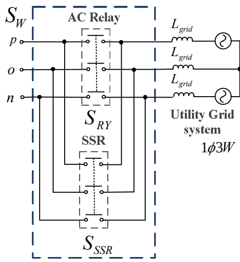
図 5.11 スイッチ S_w の回路構成
