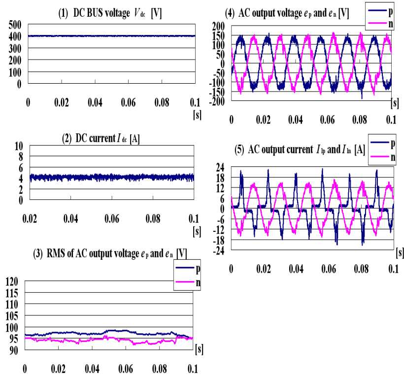
図 4.34 サンプル周波数を 40 kHz として、非線形負荷が 500 W の場合の実験結果 (E-q 変調制御)
