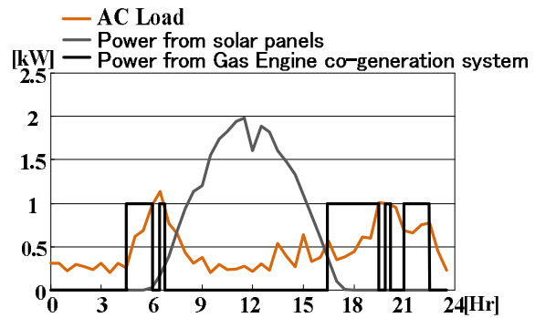
図 2.4 中間期の晴日の運転パターンの一例
