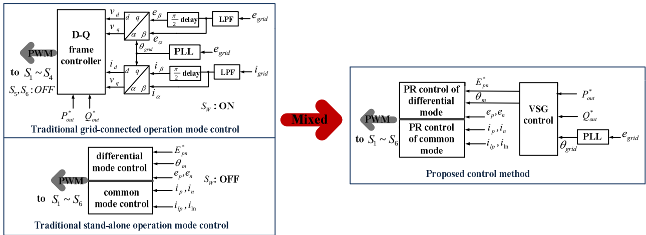
図 5.2 従来の制御方式と提案する制御方式
