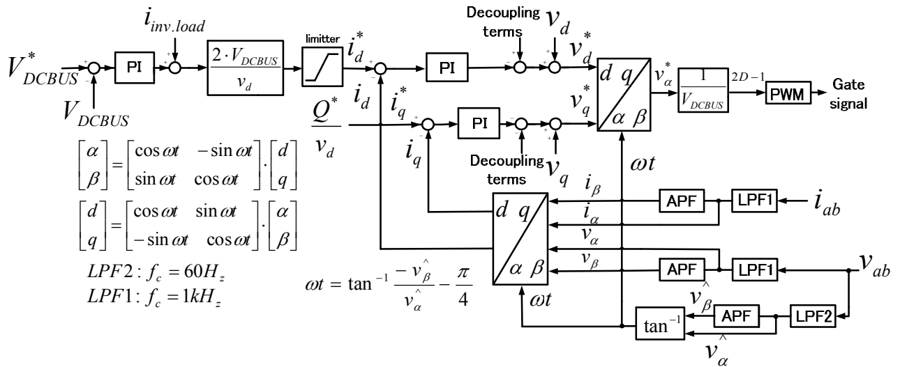
図 3.17 系統連系運転時の制御ブロック
