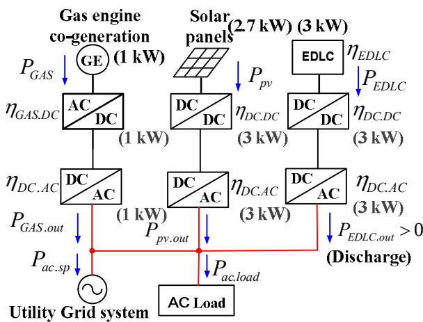
図 2.1 交流システム
