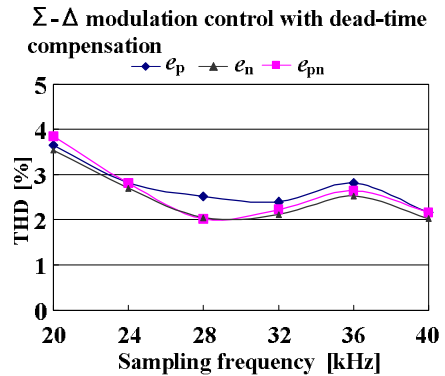
図 4.16 Σ-Δ 変調制御のデッドタイム補償がある場合の負荷電圧の THD の測定結果
