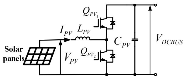
図 3.9 太陽電池用昇圧チョップの回路
