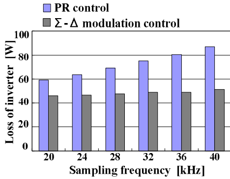
図 4.20 平衡負荷時のインバータ損失
