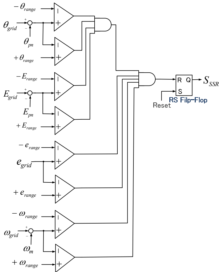
図 5.14 スイッチ S_{SSR} にオン指令を下す検出回路
