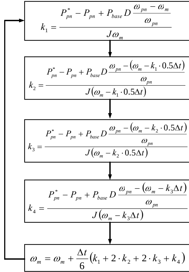
図 5.5 VSG 制御の計算フローチャート
