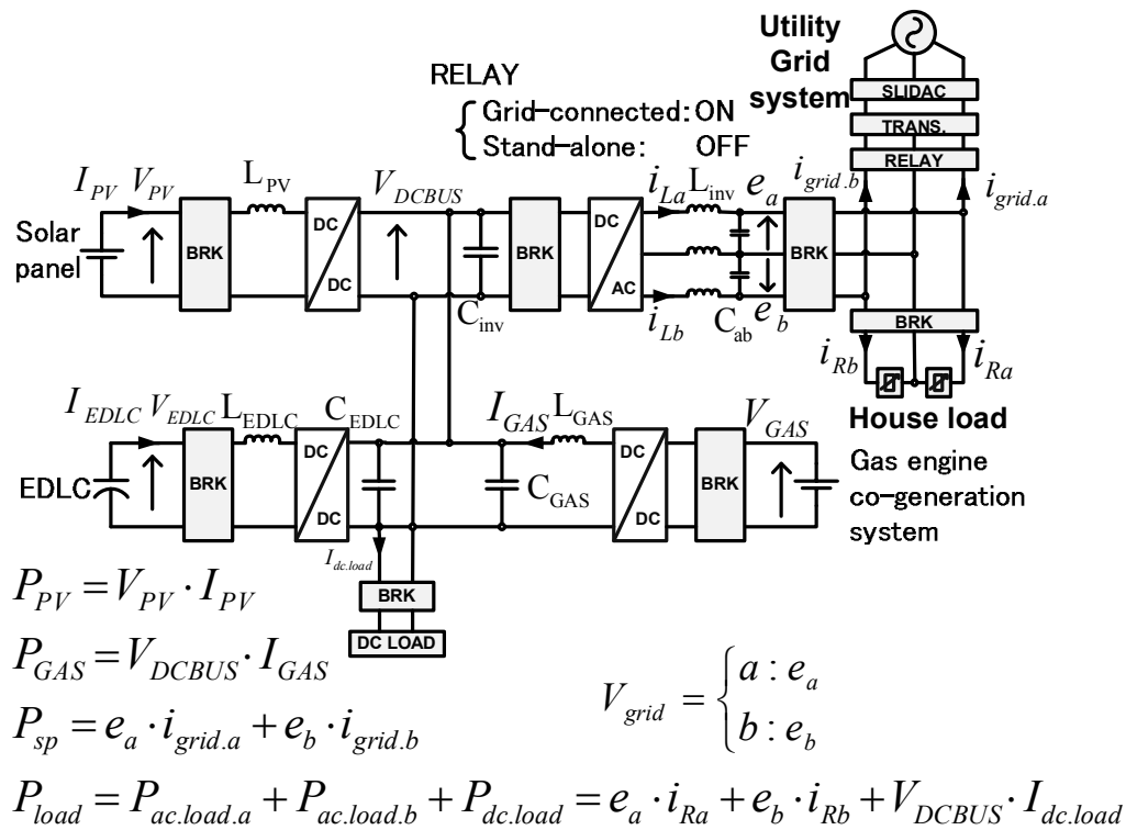
図 3.21 実験システムの回路図
