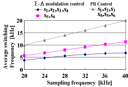
図 4.24 不平衡負荷時の平均スイッチング周波数とサンプリング周波数の関係図
