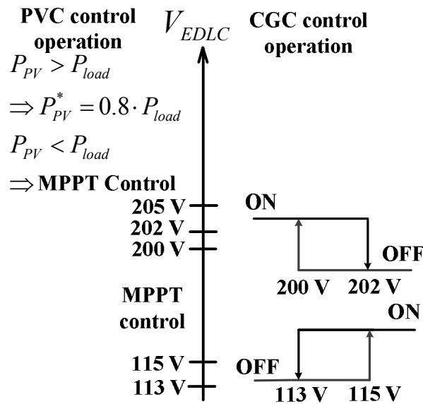
図 3.8 自立運転時の制御方法
