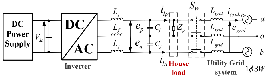
図 5.15 実験の構成と電圧および電流の測定の箇所
