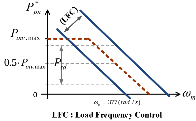
図 5.8 負荷周波数制御の概念図
