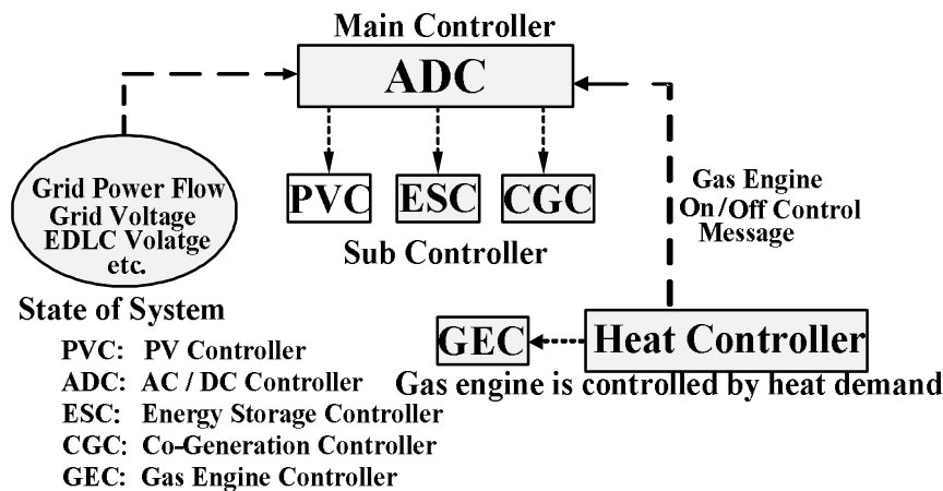
図 3.2 制御系の全体構成
