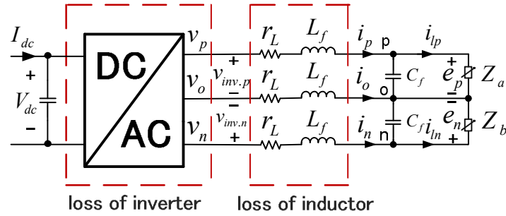
図 4.10 実験の主回路の構成図
