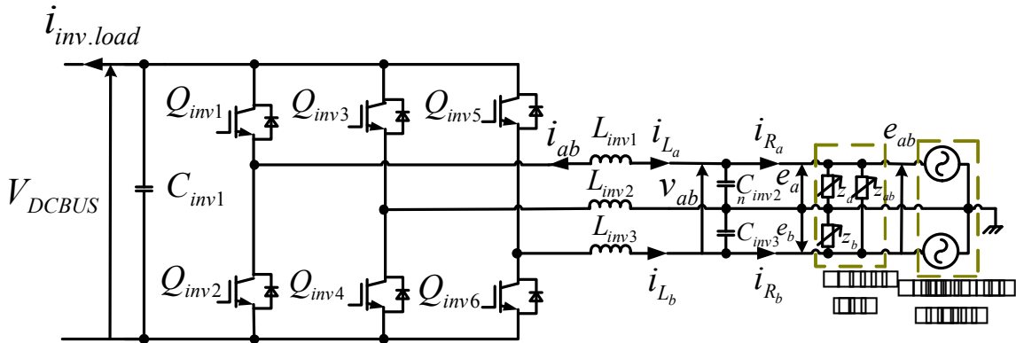
図 3.16 単相三線式インバータの回路
