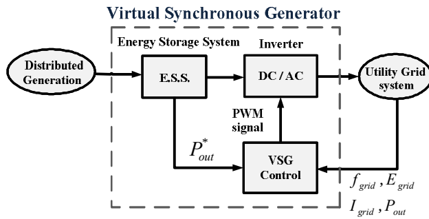
図 5.3 仮想同期発電機（VSG）の概念図
