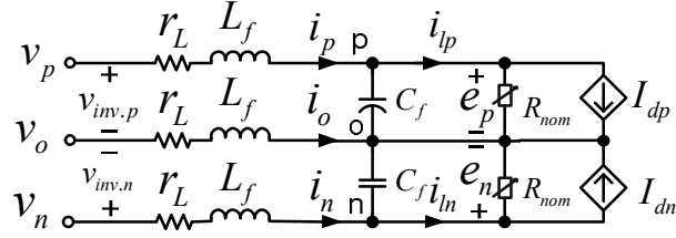
図 4.5 外乱電流源 I_{dp} , I_{dn} を接続した単相三線インバータの出力側回路
