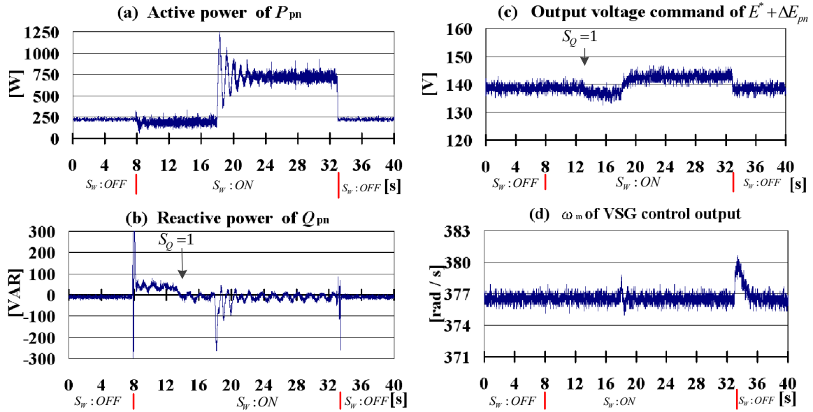
図 5.17 一連の 40 秒間の運転の実験結果
