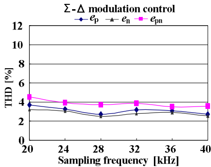
図 4.31 E-φ 変調制御の THD (不平衡負荷時)
