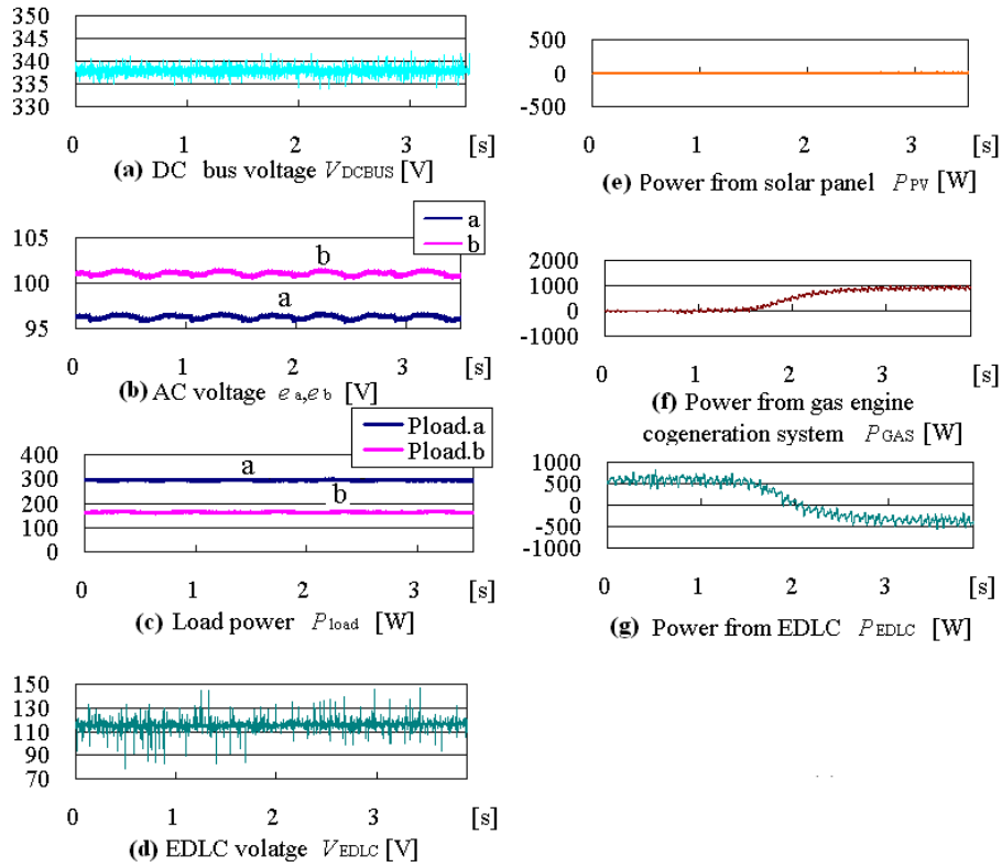
図 3.26 EDLC の電圧によるガスエンジンコージェネレーションがオフからオンとした実験結果
