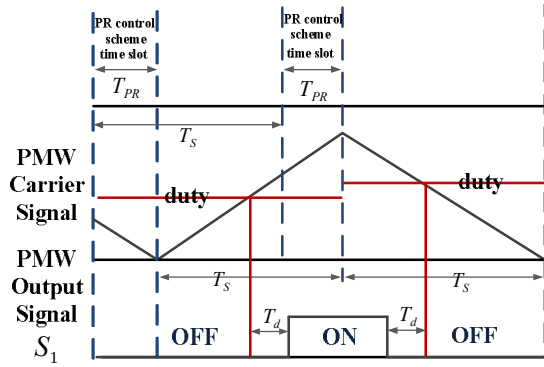
図 4.11 PR 制御の計算刻み
