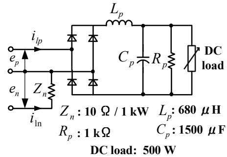
図 4.32 非線形負荷時の負荷条件
