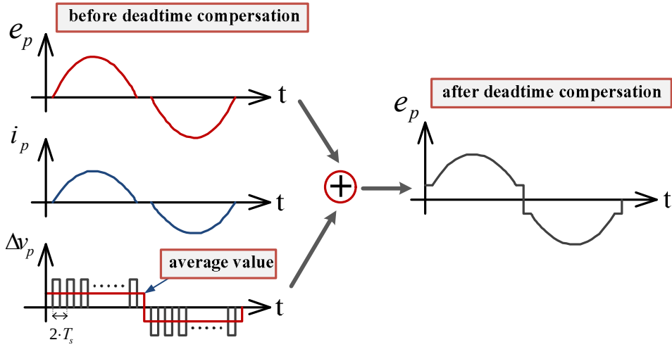
図 4.9 PR 制御の P 側回路のデッドタイム補償の原理図
