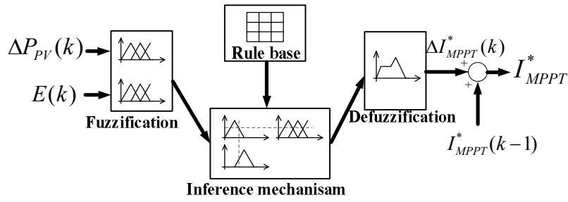
図 3.11 Fuzzy 制御ブロック
