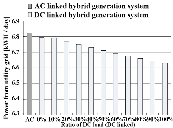
図 2.5 一日あたりの受電電力量
