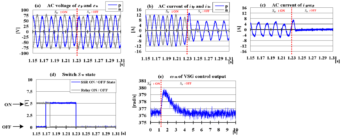
図 5.19 系統連系運転から自立運転への過渡状態の実験結果
