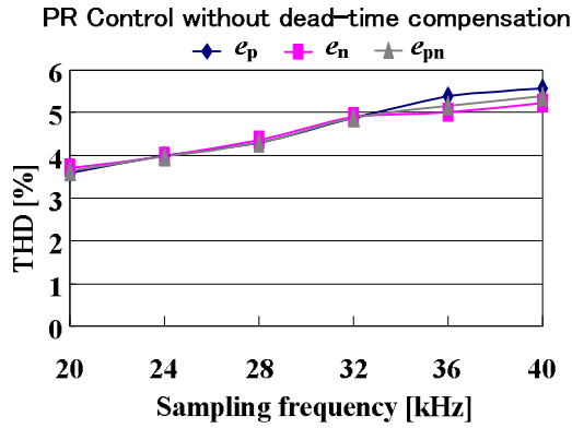
図 4.13 PR 制御のデッドタイム補償がない場合の負荷電圧の THD の測定結果
