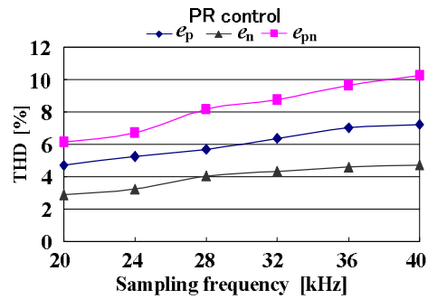
図 4.30 PR 制御の THD (不平衡負荷時)
