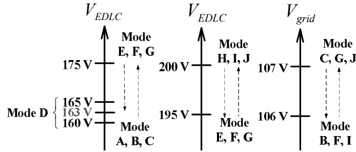
図 3.7 システム連系運転時の制御モードのヒステリシス
