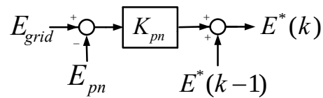
図 5.13 出力電圧の振幅と商用系統電圧の振幅を合わせる制御
