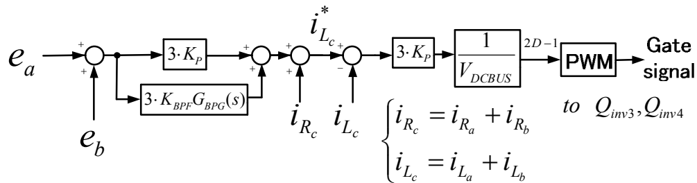
図 3.19 中性線電位の制御ブロック
