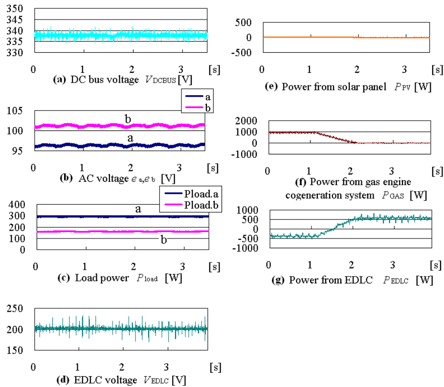
図 3.27 EDLC の電圧によるガスエンジンコージェネレーションがオンからオフとした実験結果
