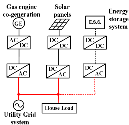
図 1.6 既存のハイブリッド発電システム 図 1.7 提案するハイブリッド発電システム
