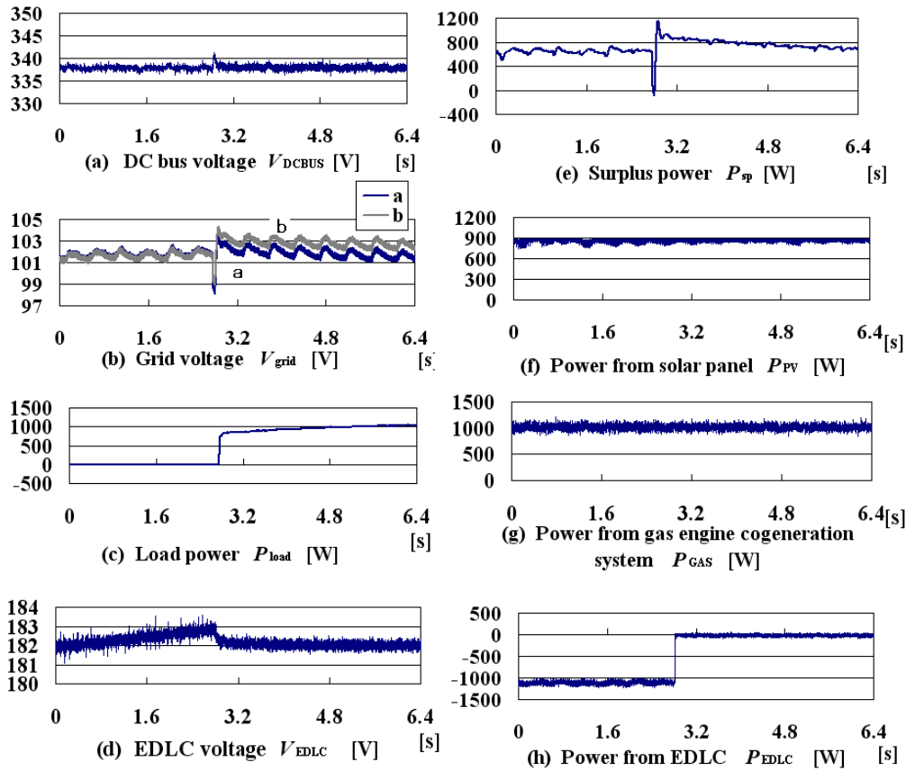
図 3.24 負荷変更におけるモード F の実験結果
