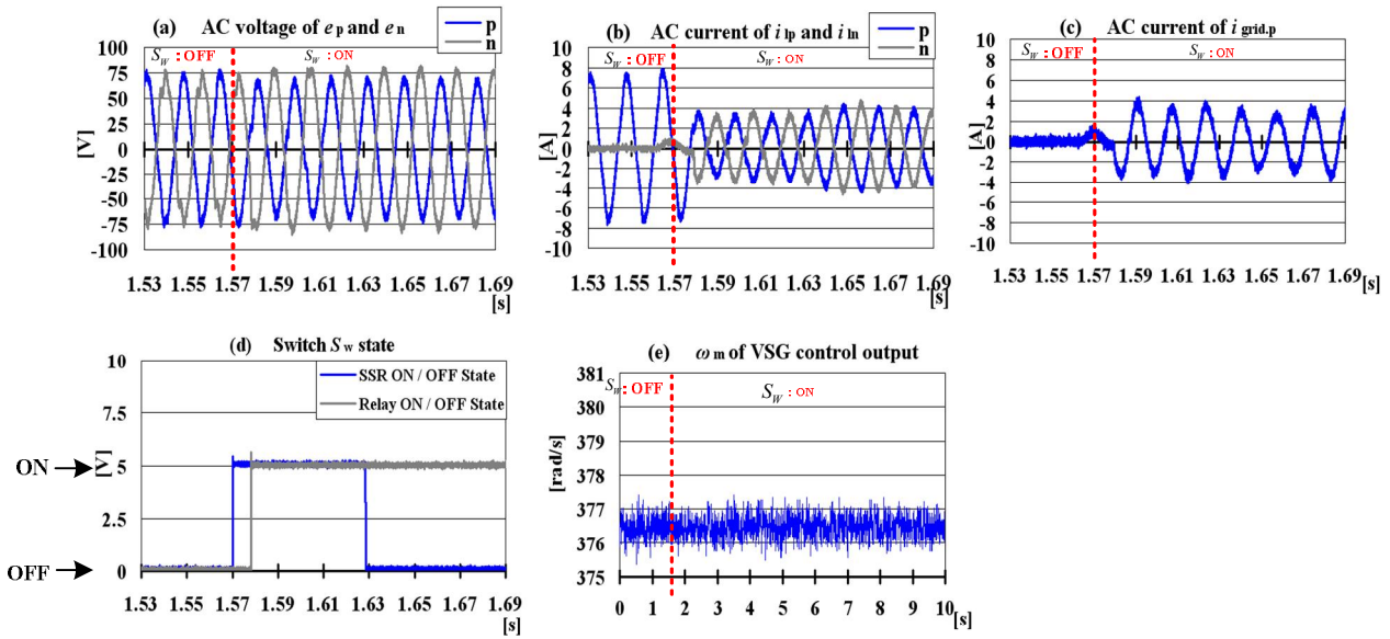
図 5.18 自立運転から系統連系運転への過渡状態の実験結果
