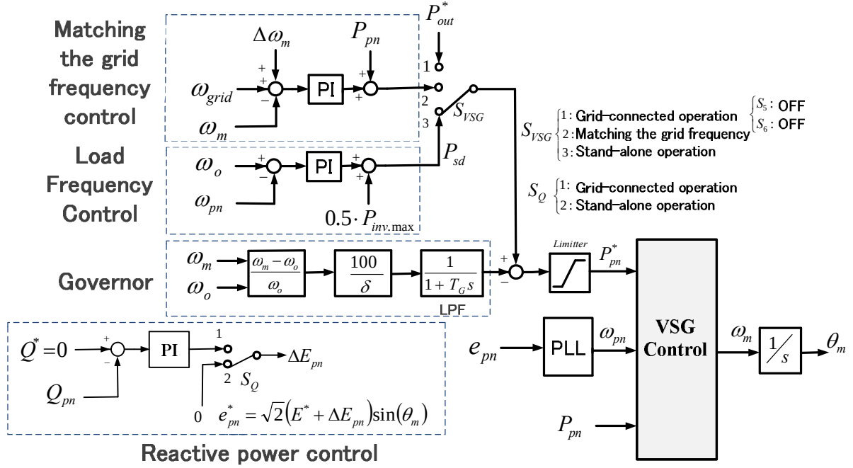
図 5.6 VSG 制御ブロック
