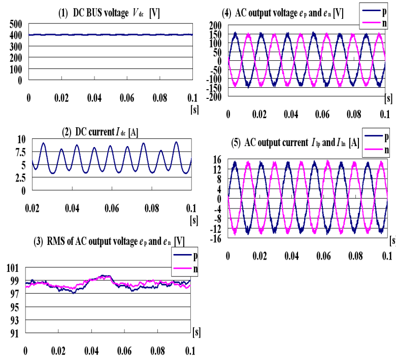
図 4.19 サンプル周波数が 40 kHz の場合で、平衡負荷時の E-q 変調制御の実験結果
