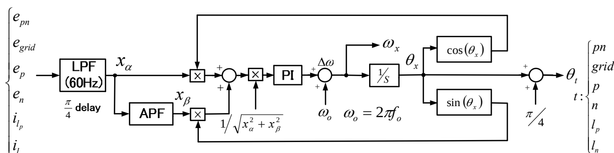
図 5.7 PLL の構成
