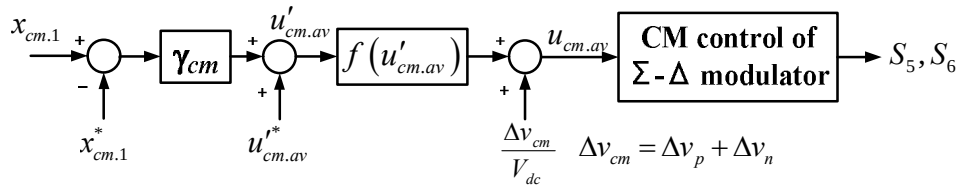
図 4.7 E-φ 変調制御の CM 制御ブロック
