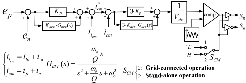
図 5.10 CM 制御ブロック
