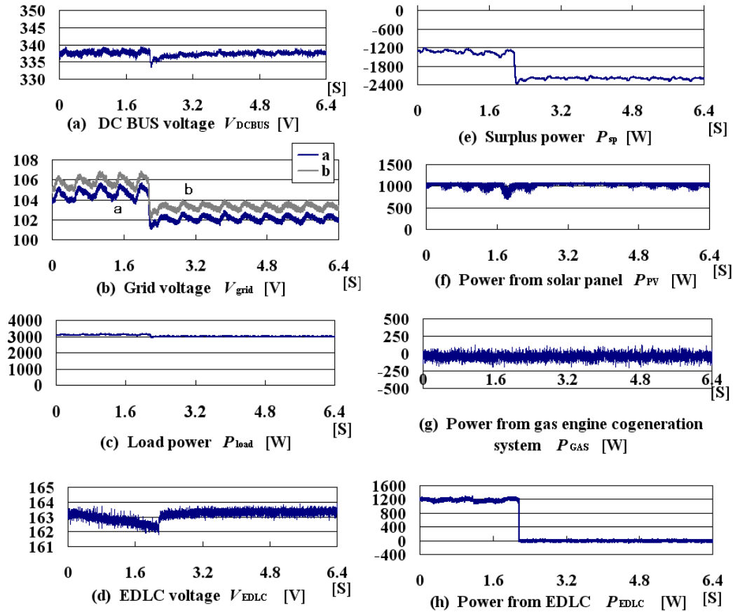
図 3.22 モード E からモード D への遷移の実験結果
