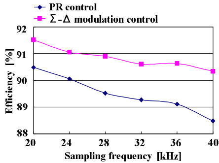
図 4.29 不平衡負荷時の効率曲線
