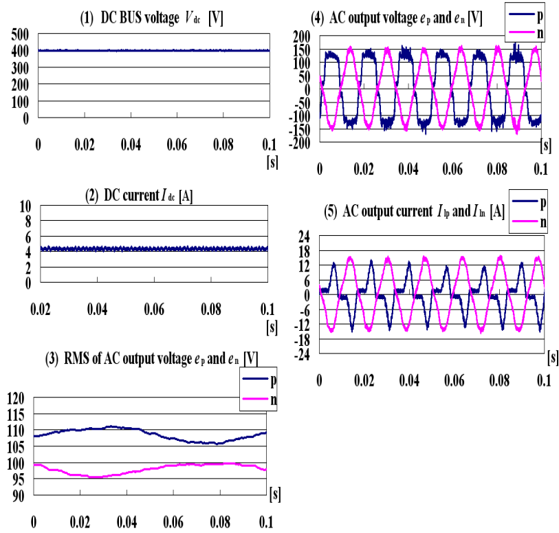
図 4.33 サンプル周波数を 40 kHz として、非線形負荷が 500 W の場合の実験結果 (PR 変調制御)
