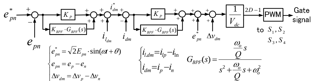
図 4.2 PR 制御の DM 制御ブロック
