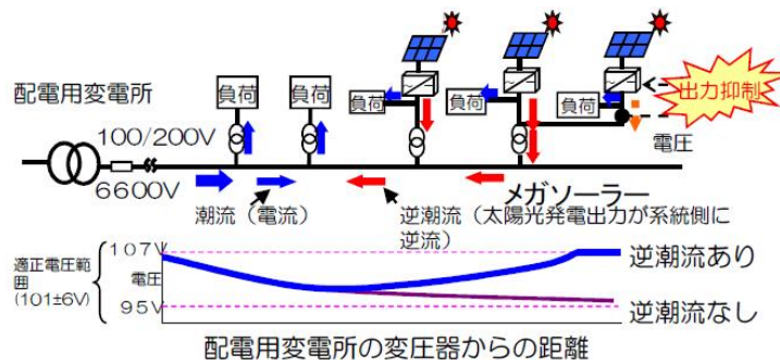
図 1.3 系統電圧上昇による太陽光発電の逆潮流の困難化（出典：参考文献[5]）
