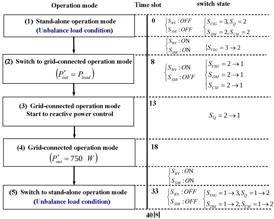
図 5.16 運転試験のフローチャート
