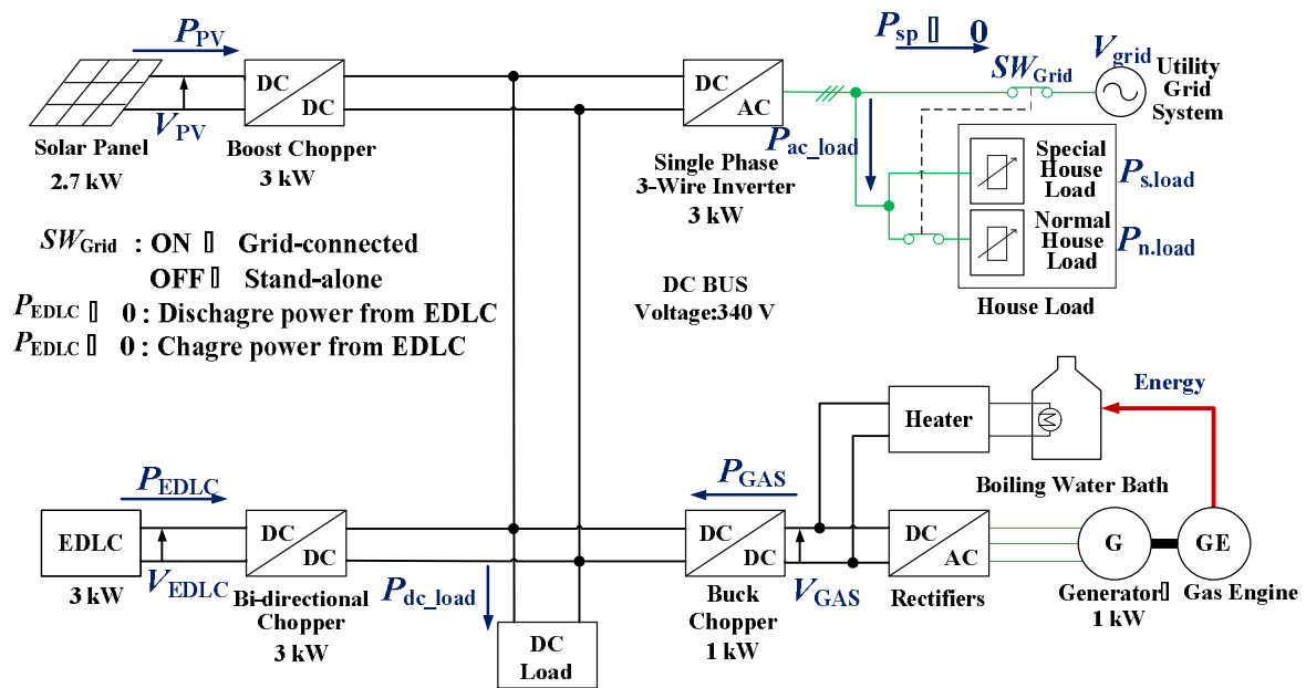
図 3.1 ハイブリッド発電システムの構成
