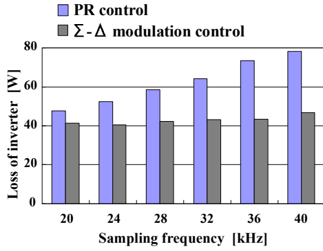
図 4.27 不平衡負荷時のインバータ損失
