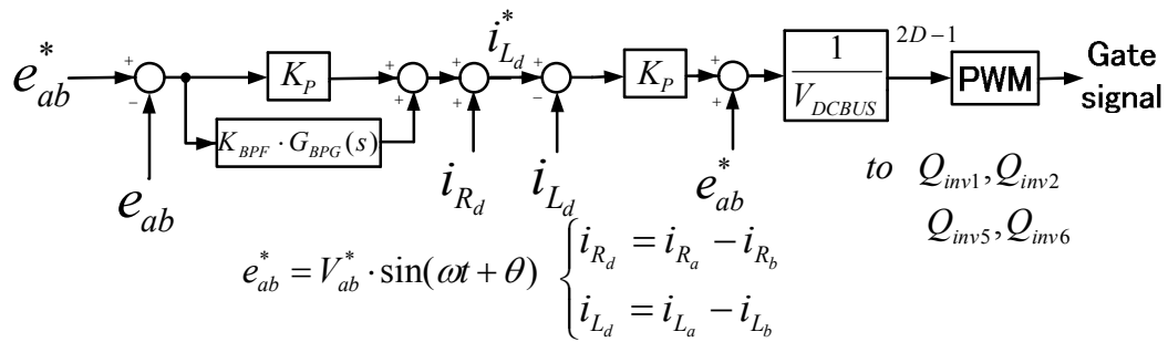
図 3.18 交流電圧の一定制御の制御ブロック
