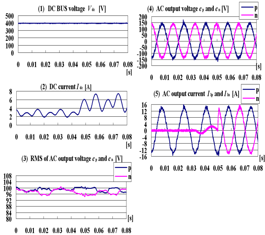
図 4.36 サンプル周波数が 40 kHz の場合において、 E-q 変調制御の過渡状態の実験結果が PR 制御より良いことを確認した。
