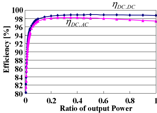
図 2.3 DC / DC コンバータと DC / AC インバータの効率曲線
