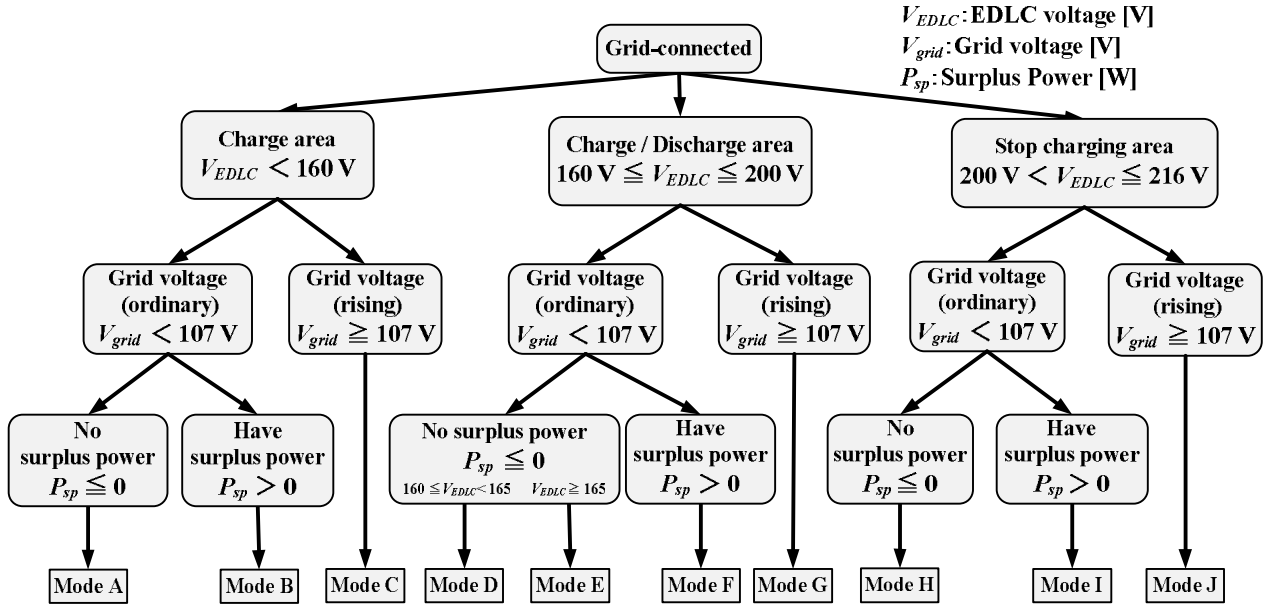
図 3.3 ハイブリッド発電システムの系統連系運転時のモード図
