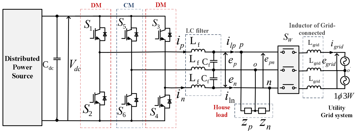
図 5.1 単相三線インバータの回路構成
