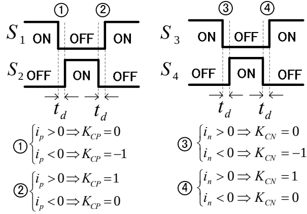
図 4.8 PR 制御のデッドタイム補償方法
