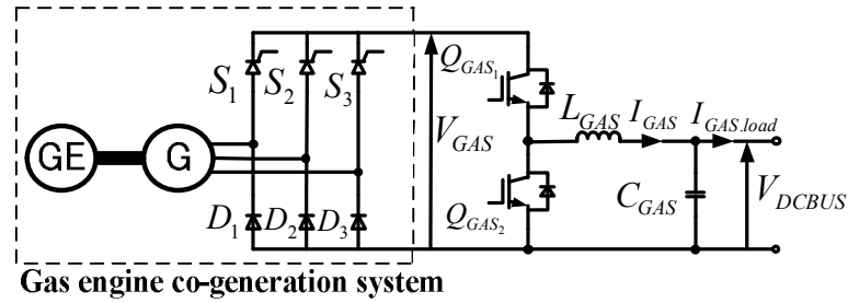
図 3.14 ガスエンジンコージェネレーション用降圧チョップパの回路
