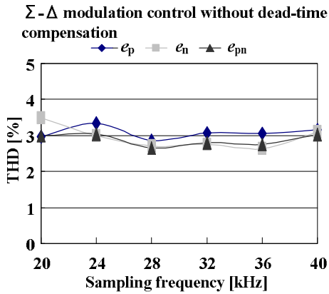
図 4.15 Σ-Δ 変調制御のデッドタイム補償がない場合の負荷電圧の THD の測定結果
