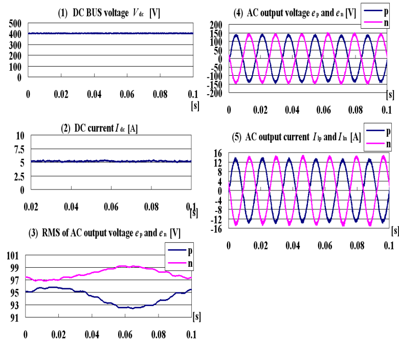
図 4.18 サンプル周波数が 40 kHz の場合で、平衡負荷時の PR 制御の実験結果
