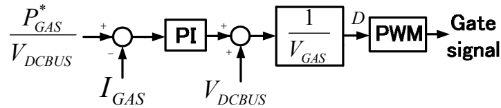
図 3.15 ガスエンジンコージェネレーション用降圧チョップパの制御ブロック
