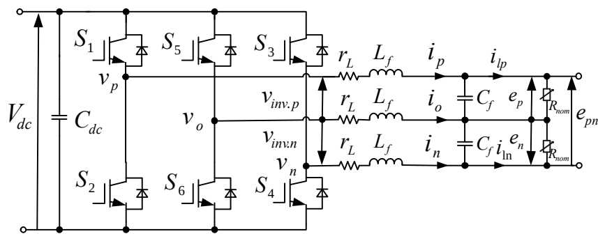
図 4.1 単相三線インバータの回路構成。
