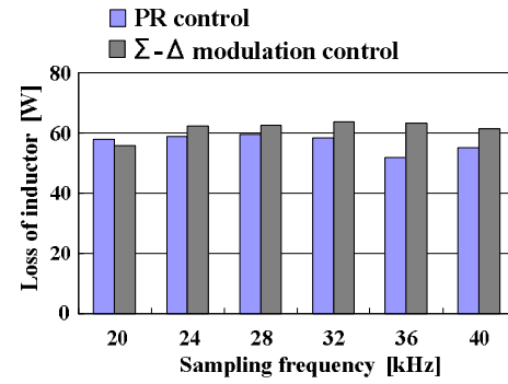
図 4.28 不平衡負荷時のインダクタ損失
