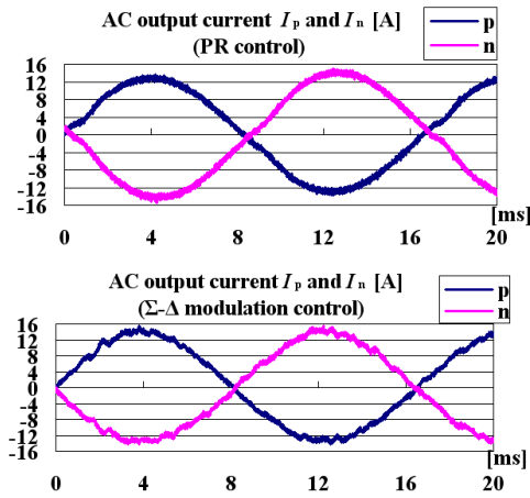
図 4.22 PR 制御と E-q 変調制御のインダクタ電流との比較
