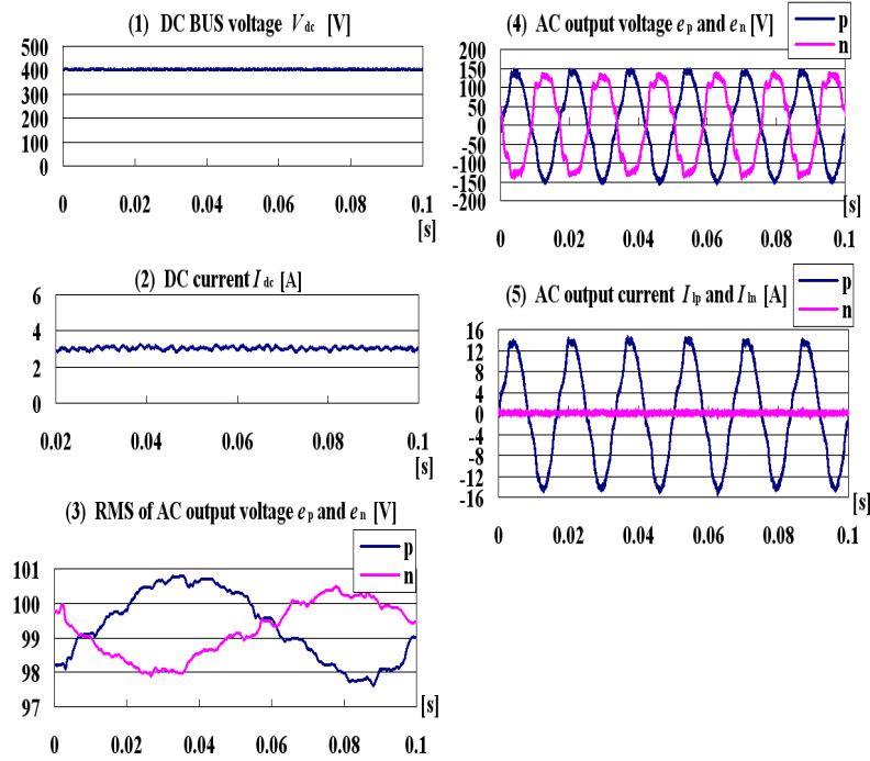
図 4.25 サンプル周波数が 40 kHz の場合で，不平衡負荷時の PR 制御の実験結果
