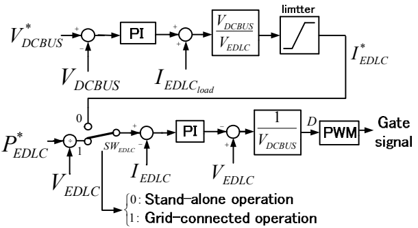
図 3.13 EDLC 用双方向チョップパの制御ブロック
