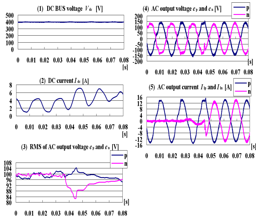
図 4.35 サンプリング周波数が 40 kHz の場合において、PR 制御の過渡状態の実験結果
