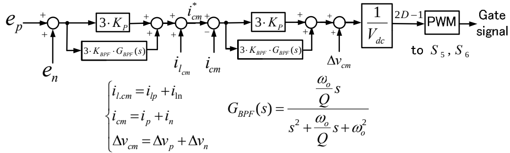
図 4.3 PR 制御の CM 制御ブロック
