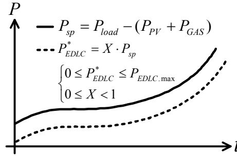
図 3.4 受電電力 P_{sp} と放電電力指令値 P_{EDLC}^* との関係図
