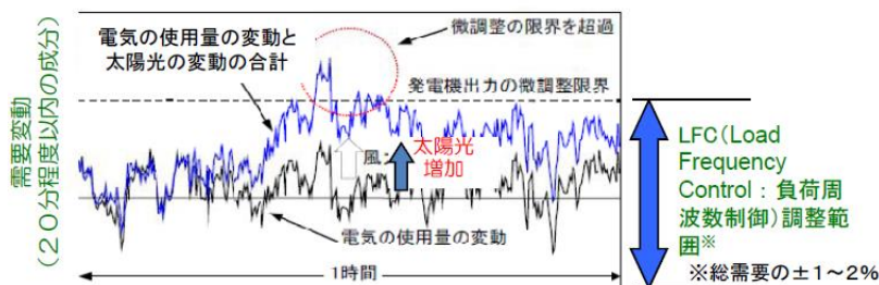
図 1.4 逆潮流電力の増加による周波数調整力の不足の概念図（出典：参考文献[5]）
