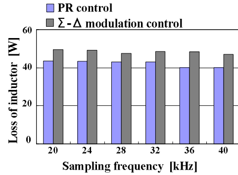
図 4.21 平衡負荷時のインダクタ損失
