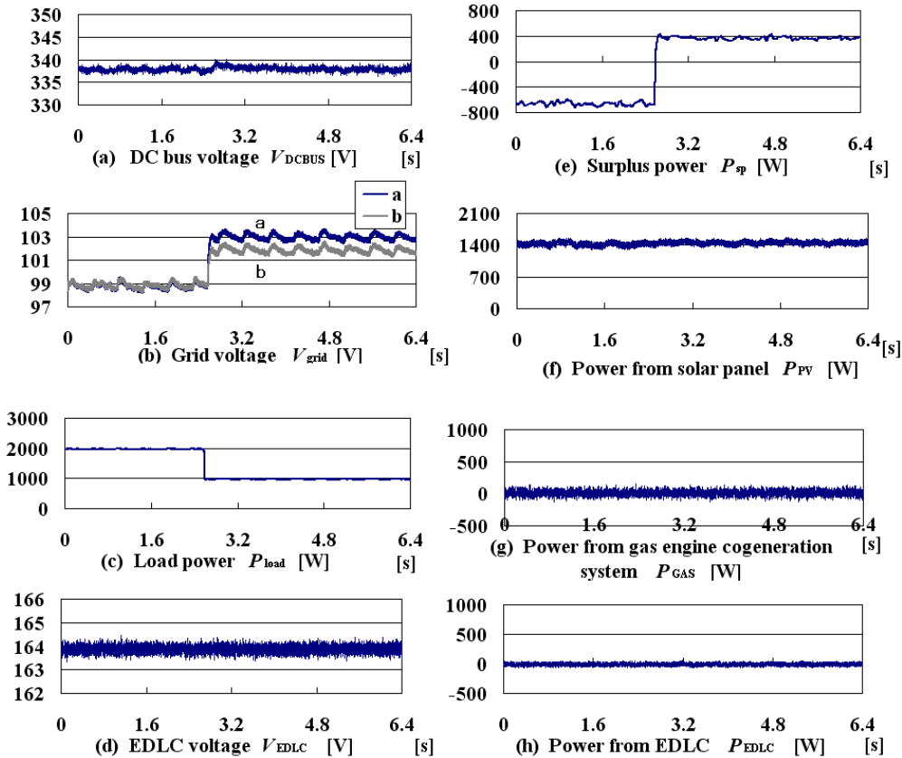
図 3.23 モード D からモード F への遷移の実験結果
