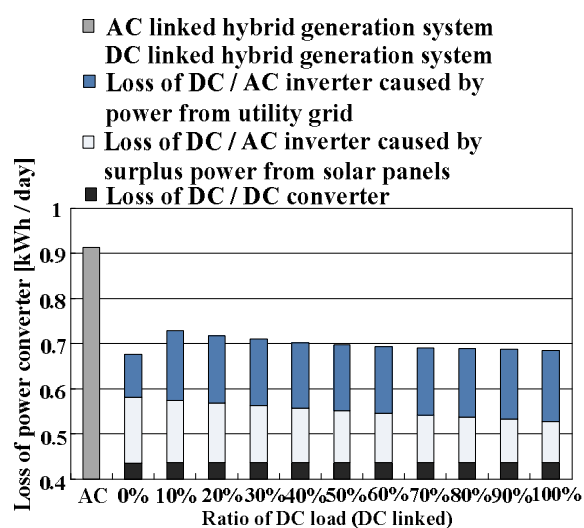
図 2.7 一日あたり電力変換器の損失の計算結果
