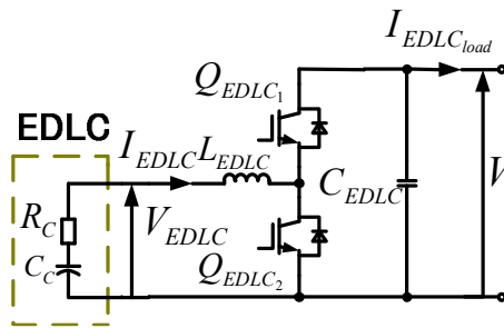
図 3.12 EDLC 用双方向チョップパの回路
