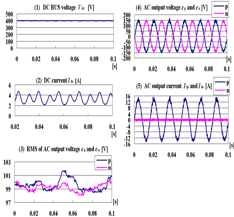
図 4.26 サンプル周波数が 40 kHz の場合で，不平衡負荷時の PR 制御の実験結果 が PR 制御より抑制されることを確認した。
