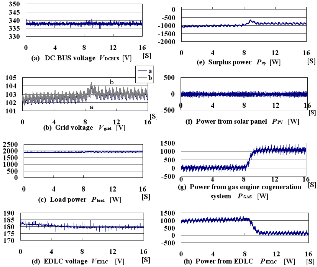
図 3.25 夜間を想定したモード E の実験結果
