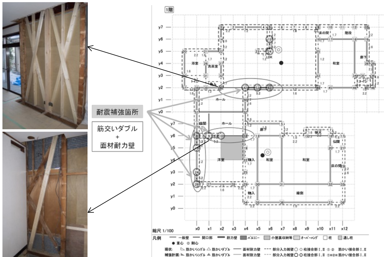
図6-7 耐震補強計画
