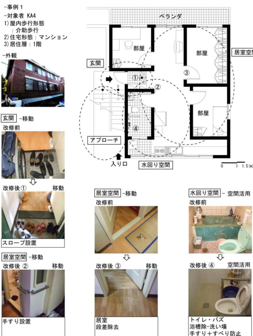
図3-6 事例 1 (マンション)の改修前後の状況
