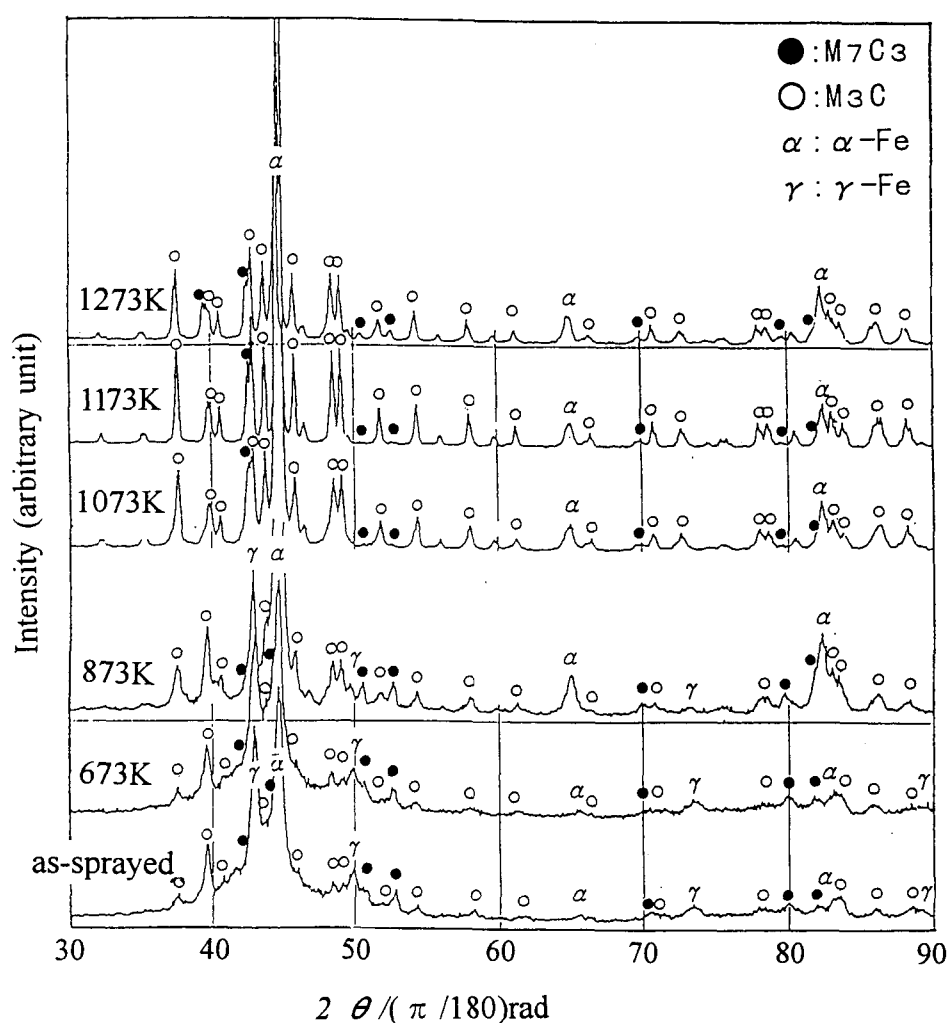
図 5-5 溶射したままおよびHIP処理を行った皮膜のX線回折図形
