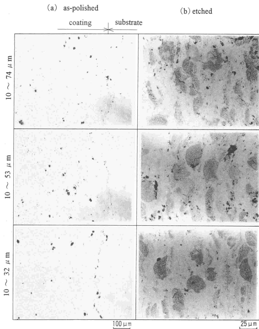
図 5-2 溶射したままの皮膜の垂直断面の光学顕微鏡組織
