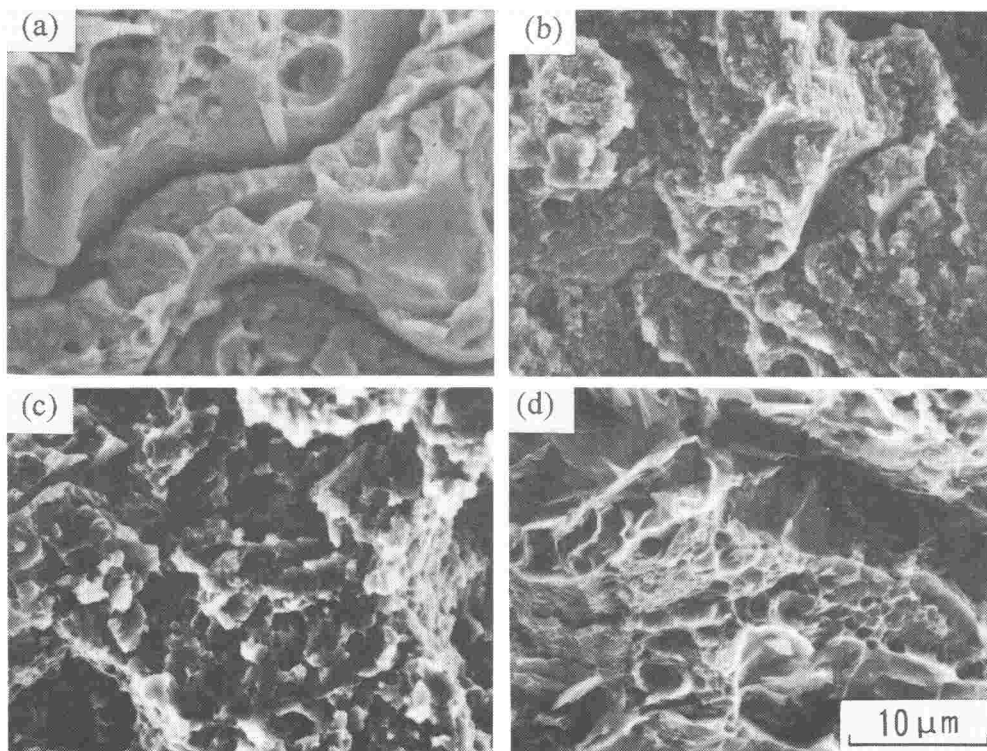
図 3 - 9 引張試験後の破断面の走査型電子顕微鏡像
