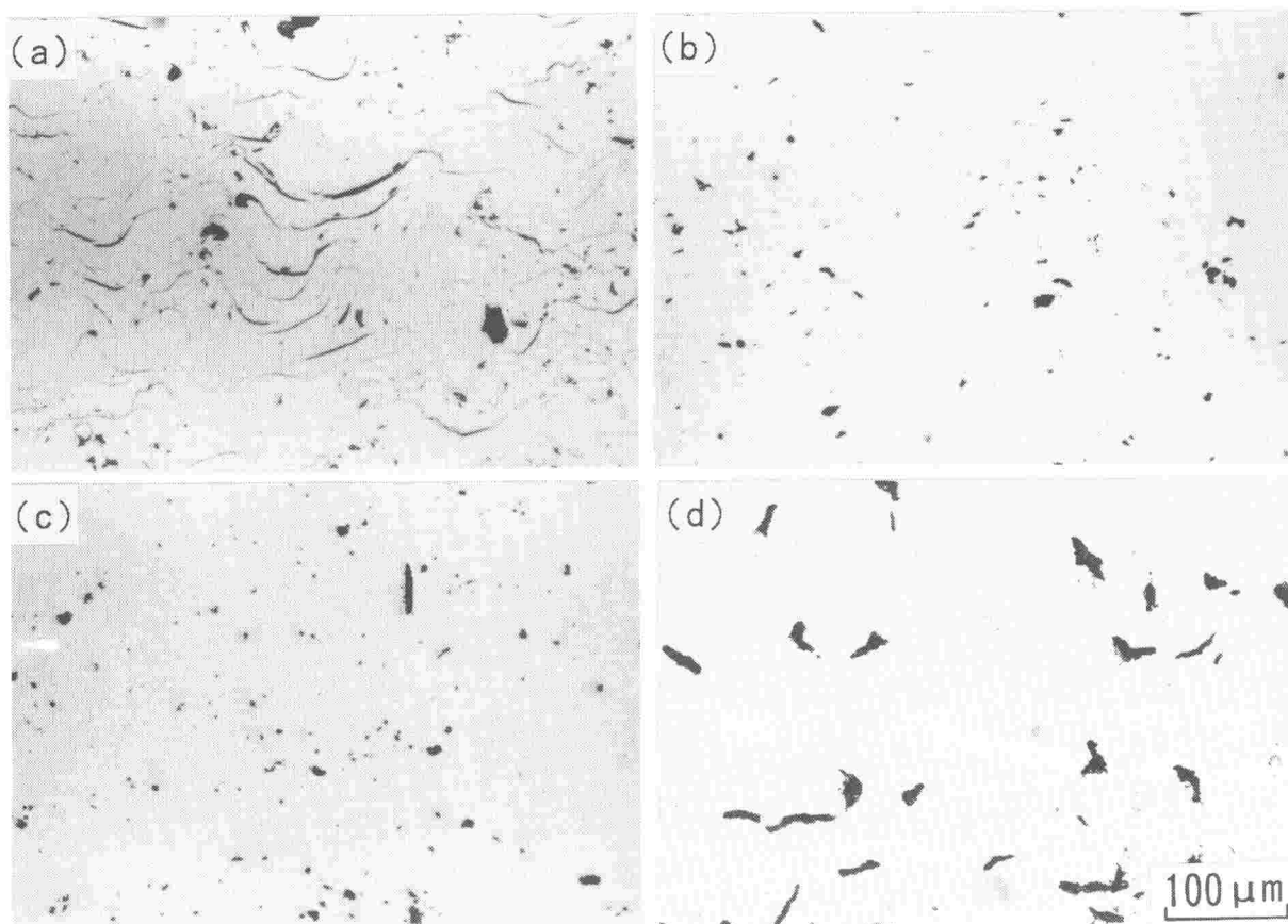
図 3-3 研磨したままの溶射皮膜の垂直断面の光学顕微鏡組織
