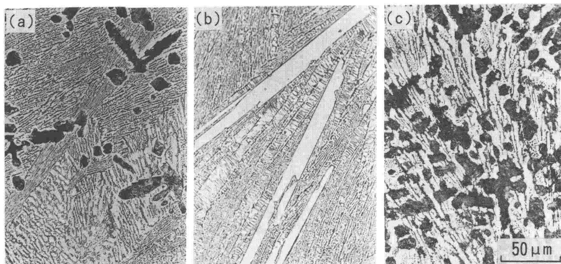
図 1 - 2 溶射用棒材の光学顕微鏡組織
