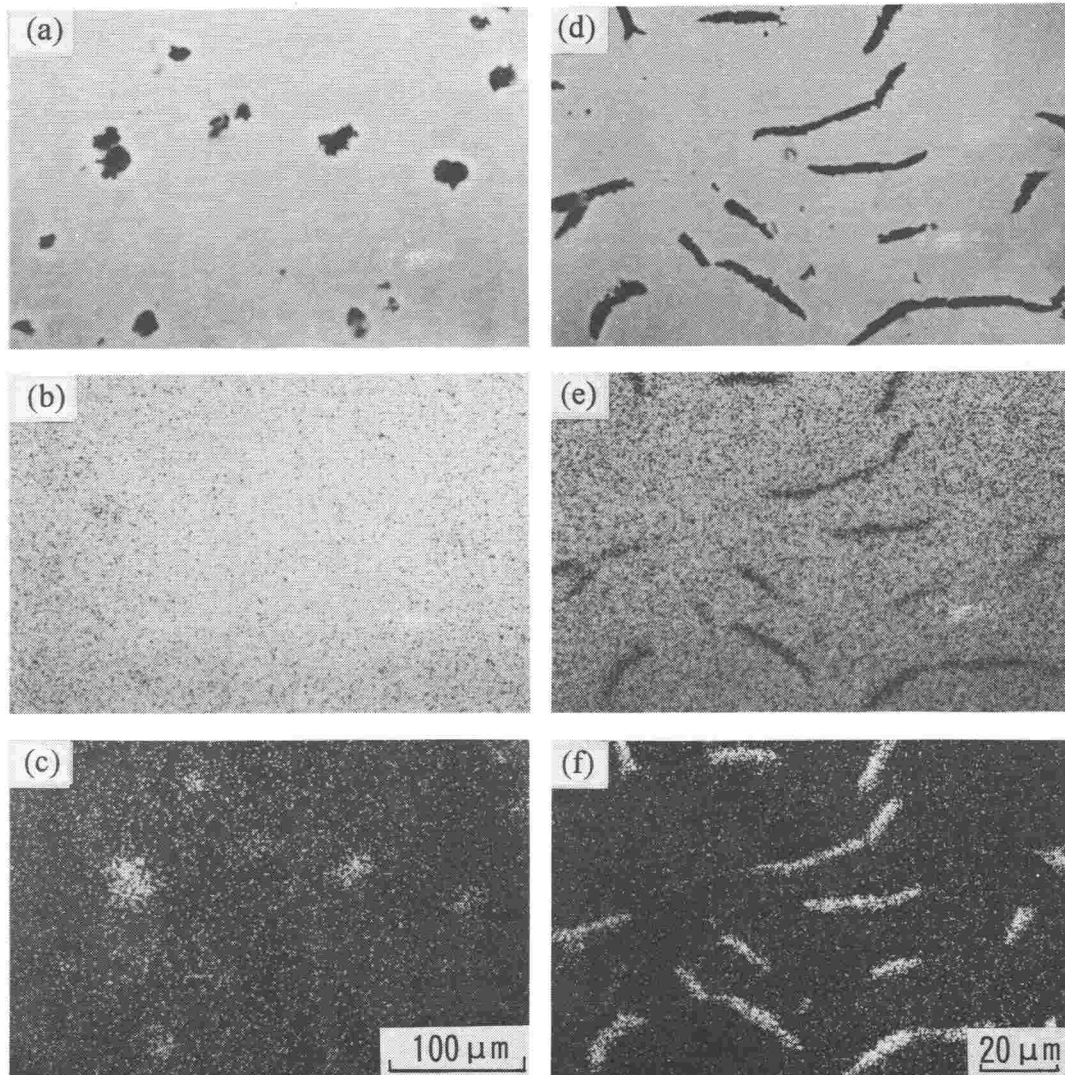
図3-4 溶射皮膜の垂直断面の走査型電子顕微鏡組織と特性X線像
