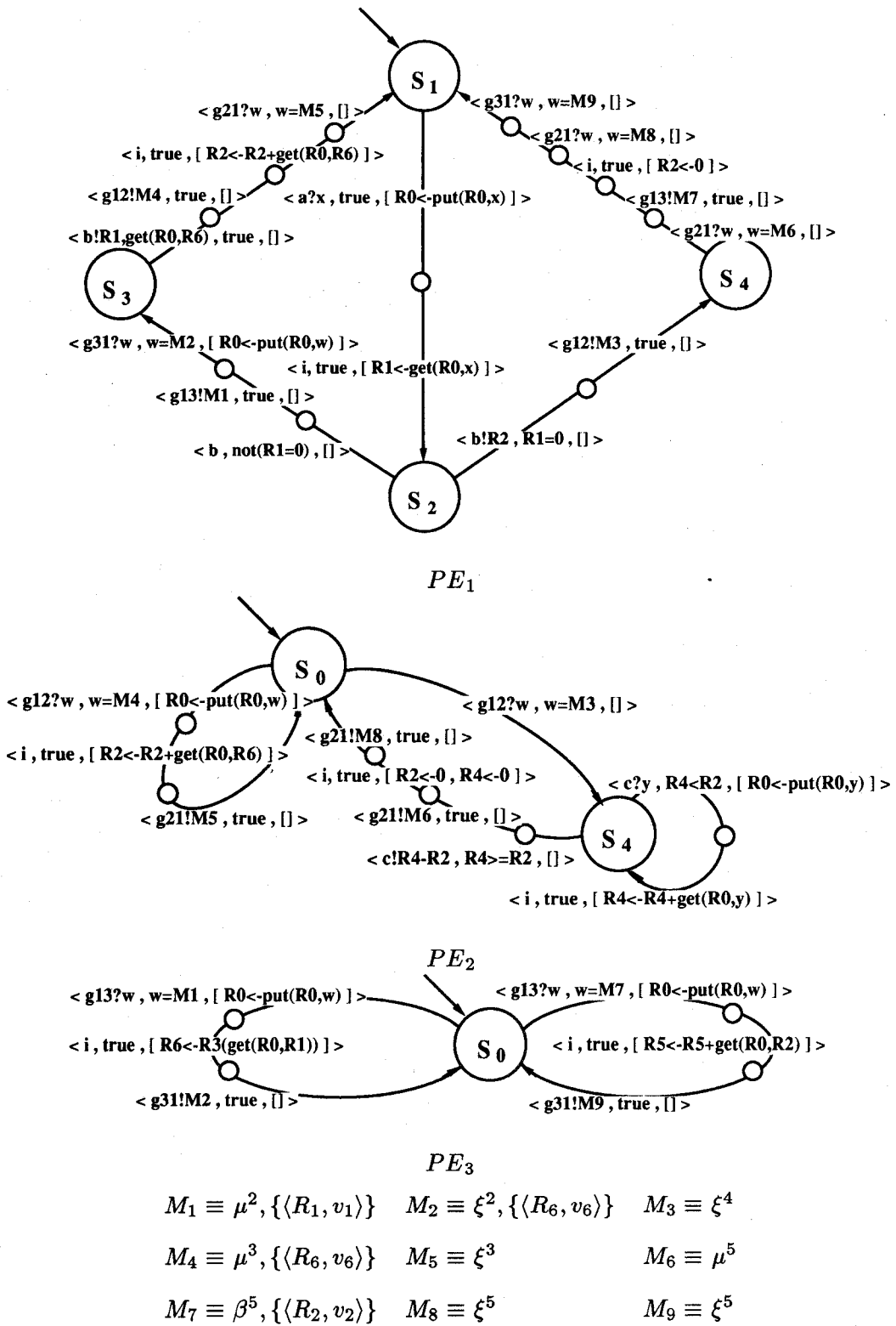
図 8: 各動作仕様 PE_k
