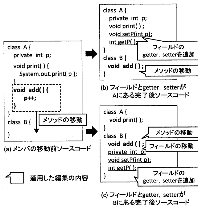
図 1 “メンバの移動”リファクタリングによる完了後のソースコード例 (完了後のソースコードに含まれるメソッド本体は省略)
