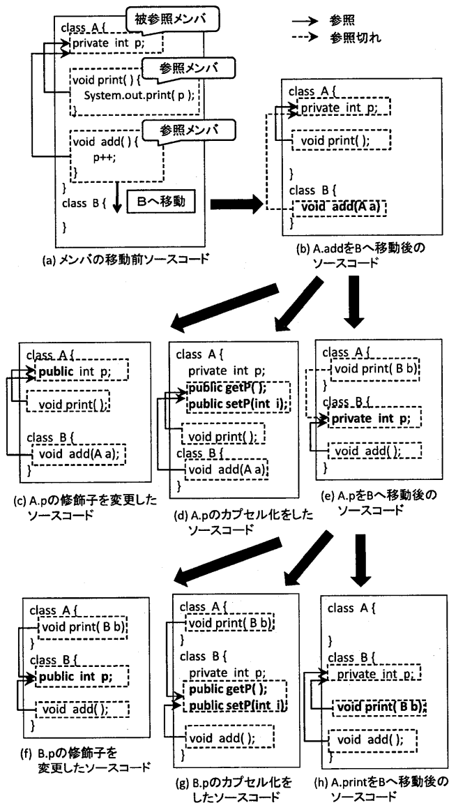
図4 メンバの移動に伴う参照切れを編集する例 ((b)~(h)のメソッド本体は省略)
