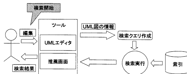
図4 検索の流れ
