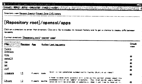
図 3 ディレクトリ構造表示画面
