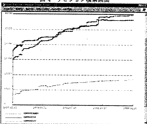
図 5 総行数の折れ線グラフ
