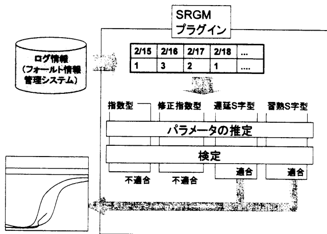
図4 SRGM プラグインの構成
