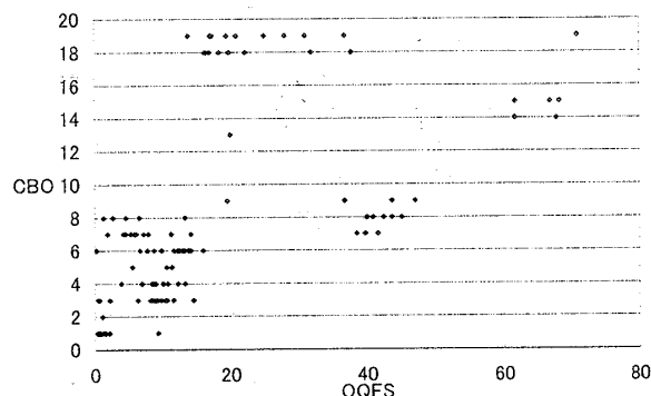
図 1: OQFS vs. CBO
