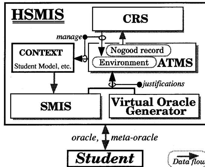
図 4.5: HSMIS の構成
