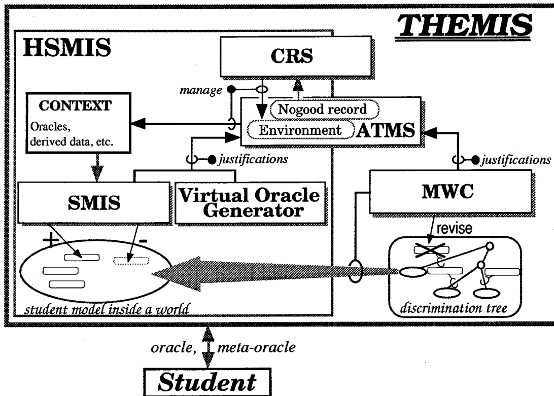
図 5.4: THEMIS の構成
