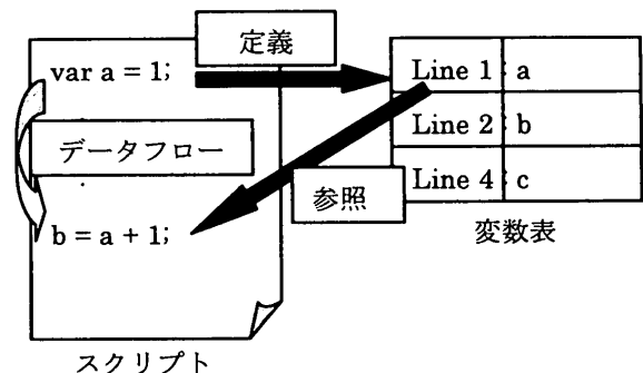
図2 データフロー解析
