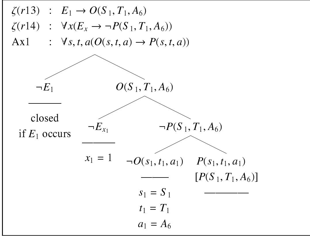
図 3.4 自由変数タブロー法による解析例
