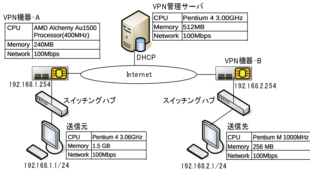
図 4.13 大容量画像データの転送実験環境
