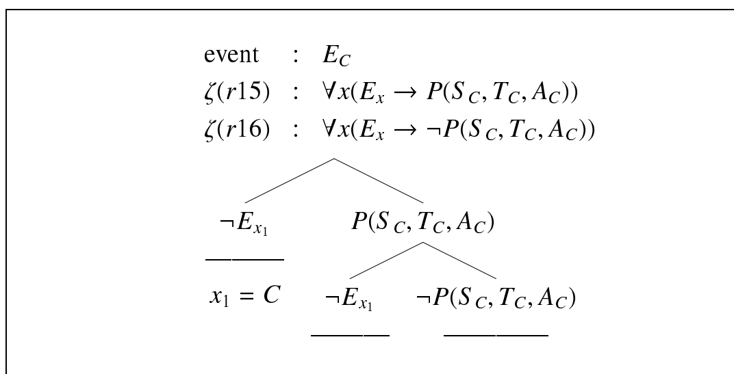
図 3.6 [Type I] 単純矛盾 (Auth+/Auth-) の検出
