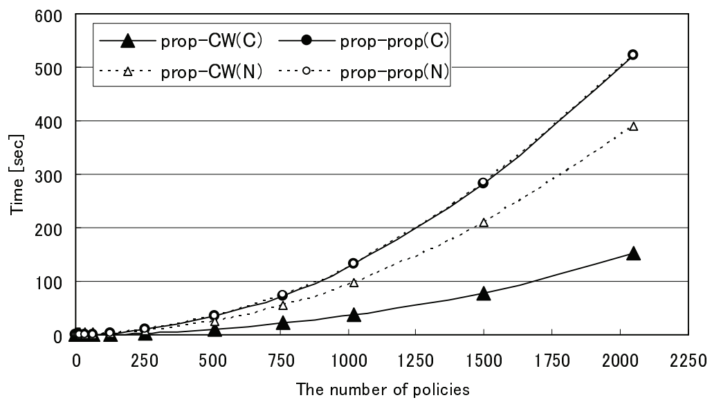
図 3.17 ケース IV：混合矛盾の検出時間
