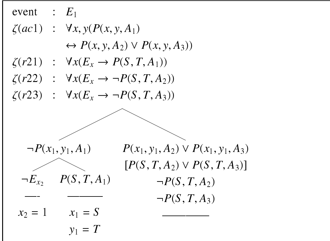
図 3.10 [Type IV] 制約矛盾 ( A_1 = A_2 \vee A_3 ) の検出
