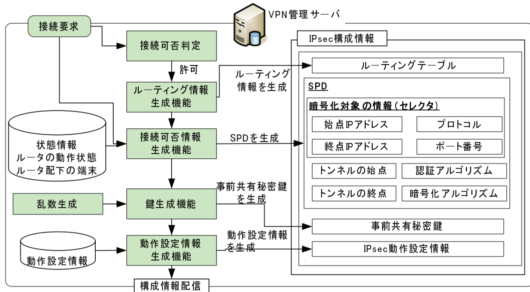
図 4.6 アクセス制御ポリシーの自動生成処理
