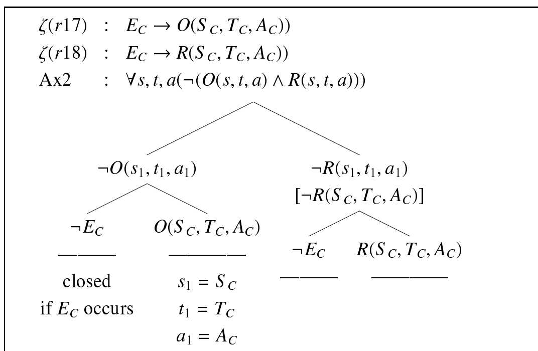
図 3.7 [Type II] 単純矛盾 (Obli+/Obli-) の検出
