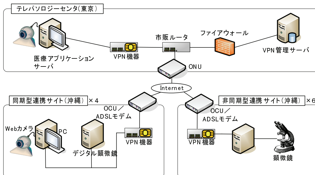
図 4.17 実証実験ネットワーク構成
