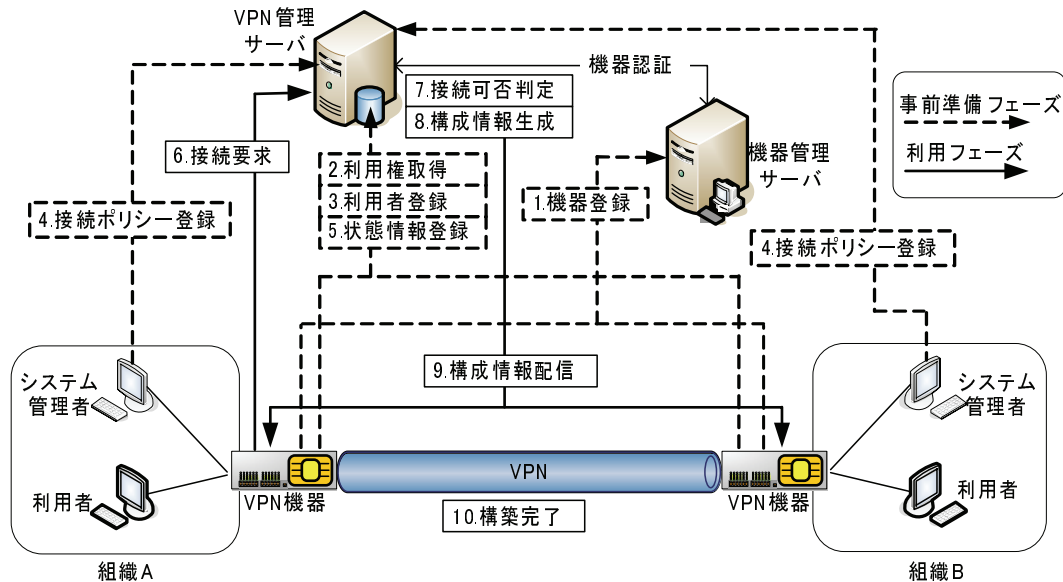
図 4.7 オンデマンド VPN システム構成図
