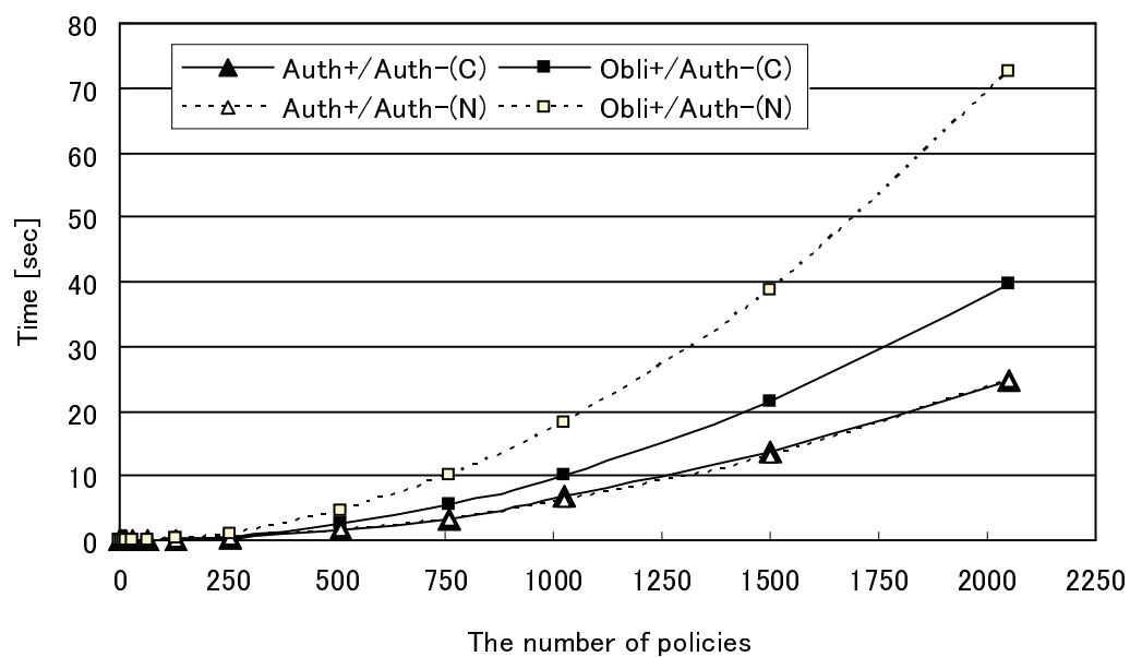
図 3.14 ケース I：単純矛盾の検出時間
