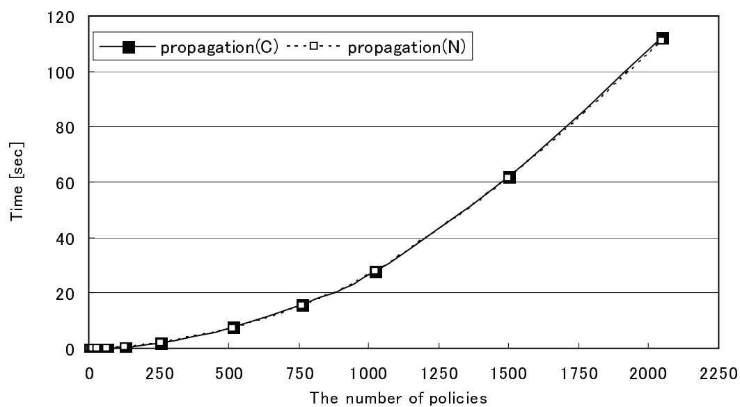
図 3.15 ケース II:暗黙的な単純矛盾の検出時間
