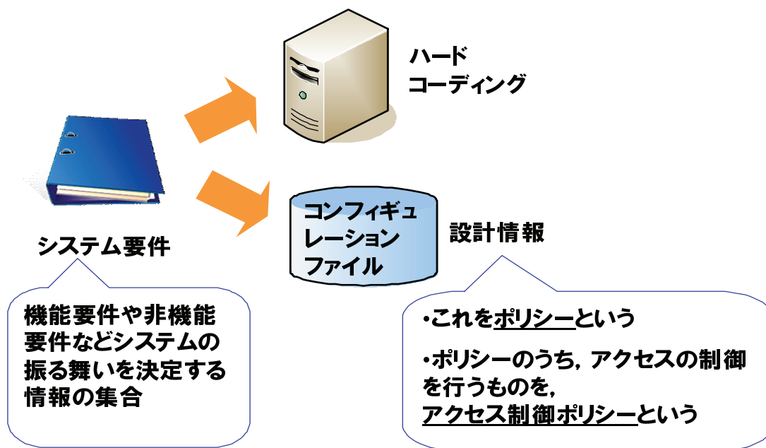
図 2.1 アクセス制御ポリシーの定義
