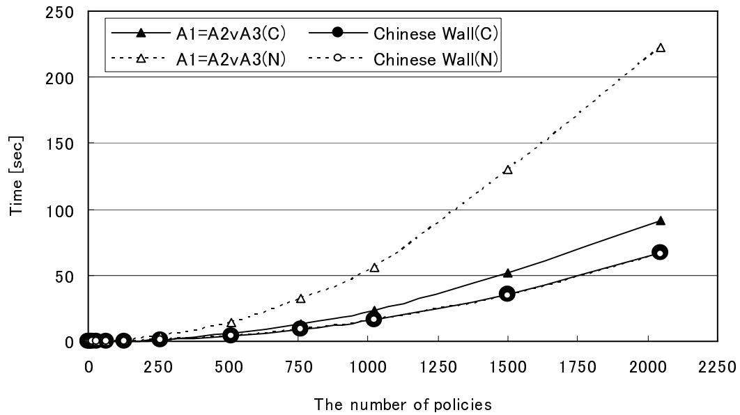
図 3.16 ケース III:制約矛盾の検出時間
