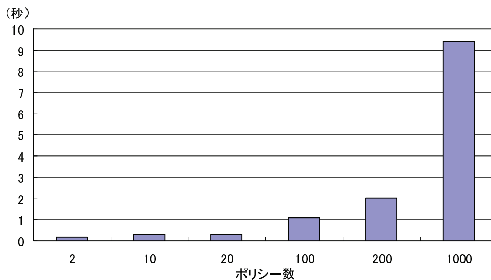
図 4.16 アクセス接続ポリシー可否判定時間
