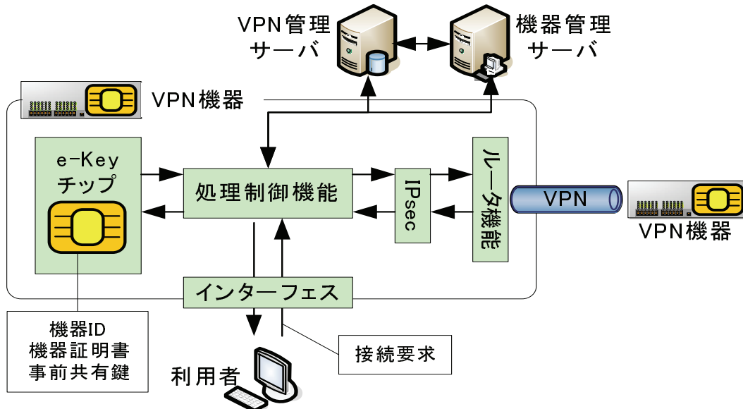
図 4.4 VPN 機器の機能構成
