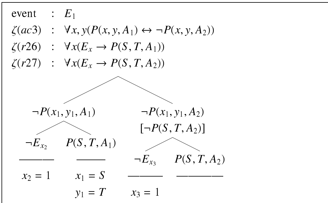
図 3.12 [Type VI] 制約矛盾 ( A_1 = \neg A_2 ) の検出
