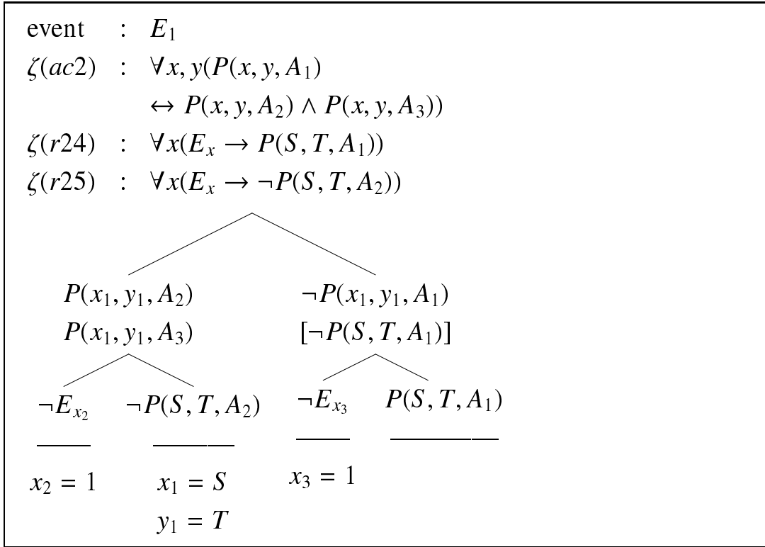
図 3.11 [Type V] 制約矛盾 ( A_1 = A_2 \wedge A_3 ) の検出
