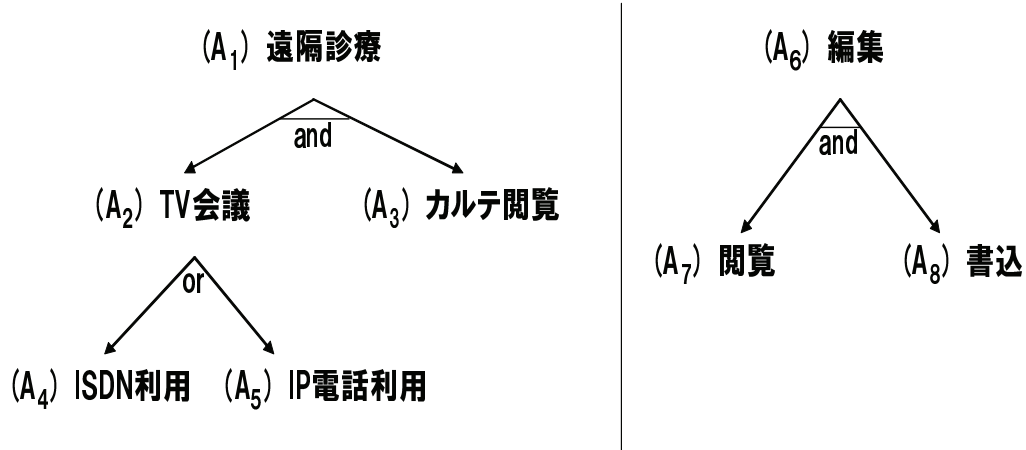
図 3.3 合成動作の例
