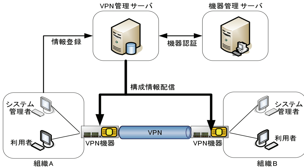
図 4.1 オンデマンド VPN システム全体構成
