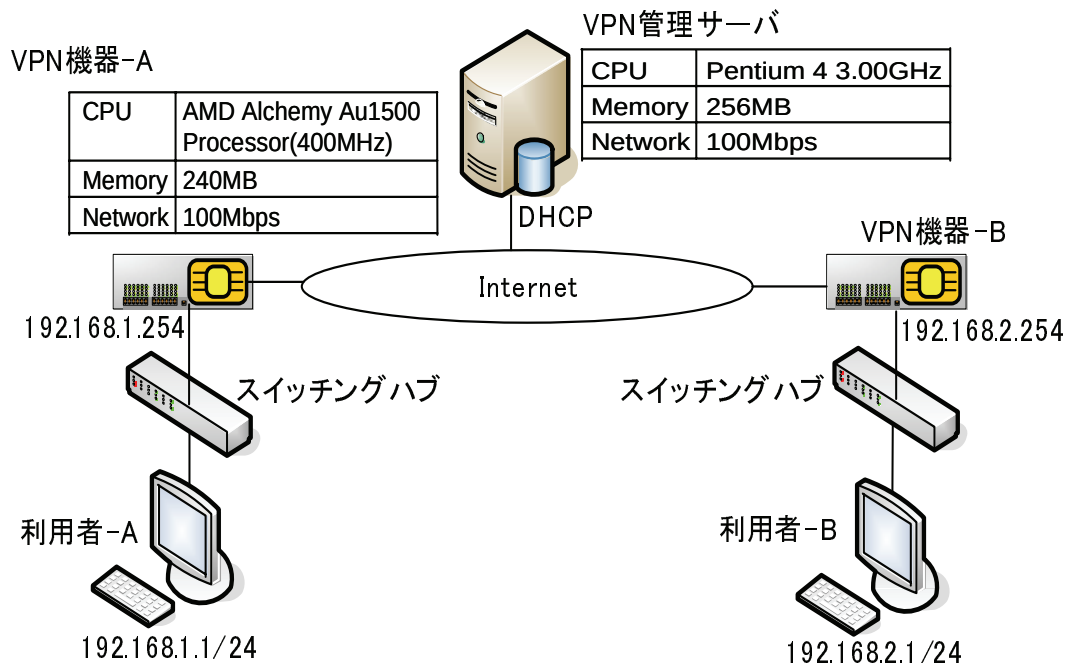
図 4.9 VPN 接続時間測定実験環境
