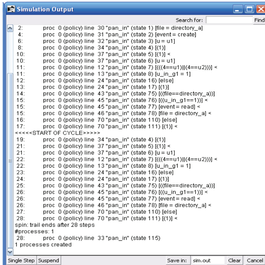
図 5.2 SPIN の反例トレース (可用性の不整合の検証結果)
