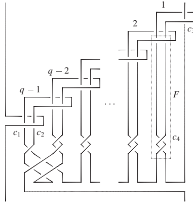
Fig. 8. Tangle $H_q$.
