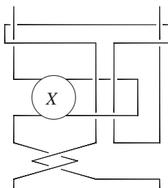
Fig. 9. Tangle R(X) .
