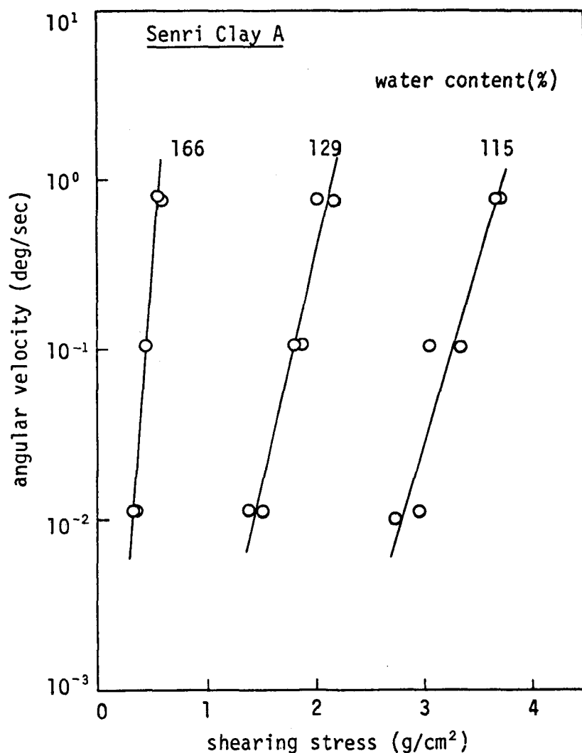
図一 1.2.11 b) 千里粘土 A
