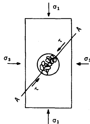
図-1.2.3 すべり面に沿う粒子接合点の模式図
