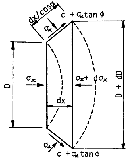
図-2.4.5 塑性変形地盤の微小要素(土塊 EBB'E' )
