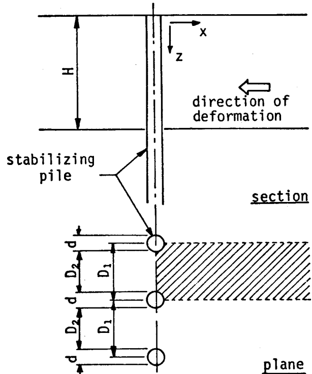
図-2.4.3 杭列と塑性変形地盤
