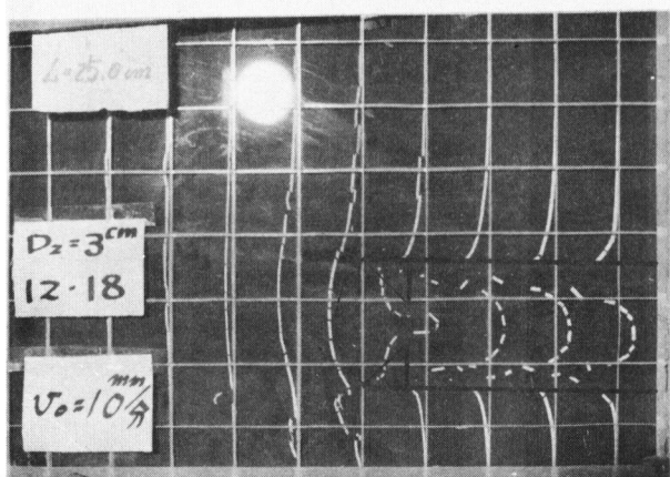
写真 2.3.3 周辺地盤の水平変位の挙動 ( D_2/D_1 = 0.3 )
