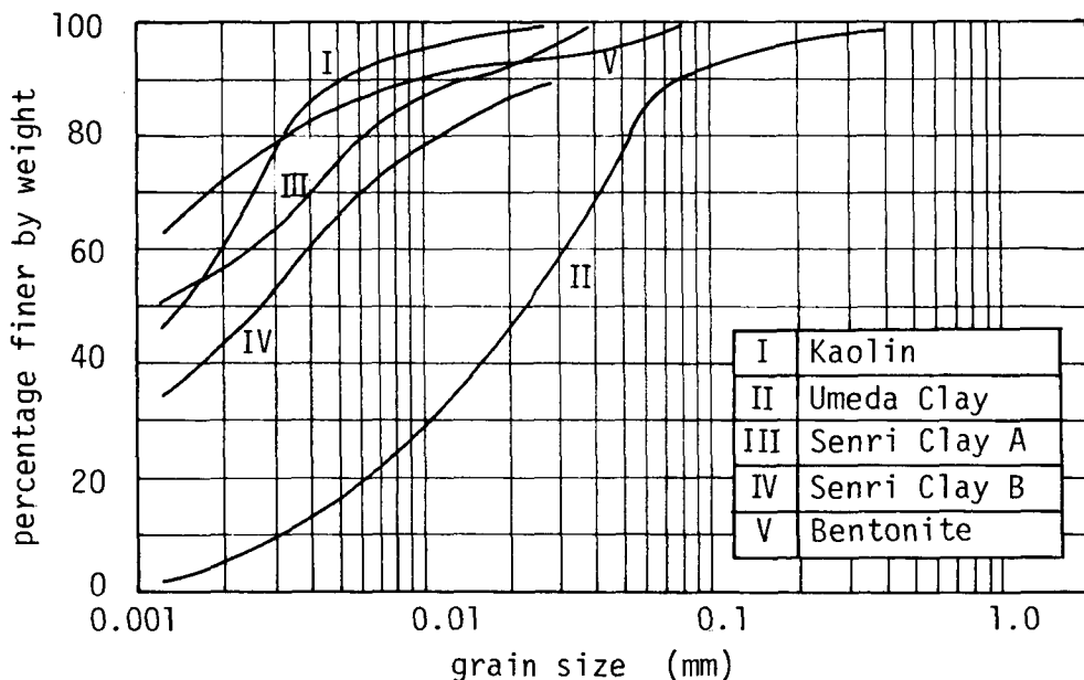
図一 1. 2. 6 粒径加積曲線
