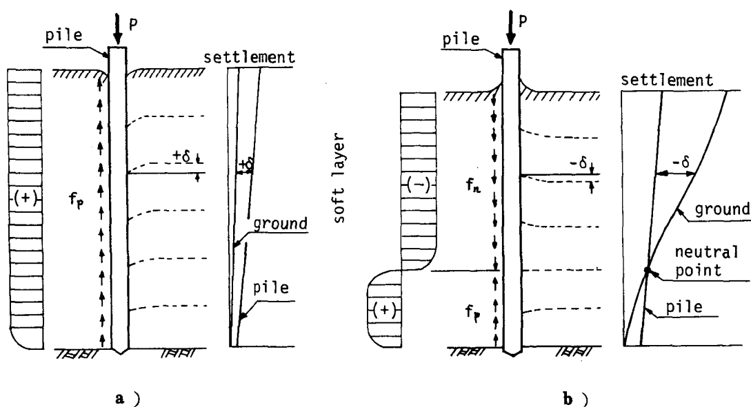
図- 2.5.1 杭に作用する摩擦力
