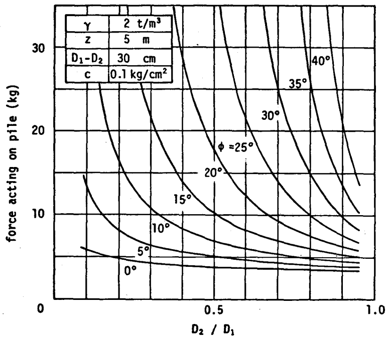
図-2.4.10 塑性変形理論式の特長 (内部摩擦角 \phi の影響)
