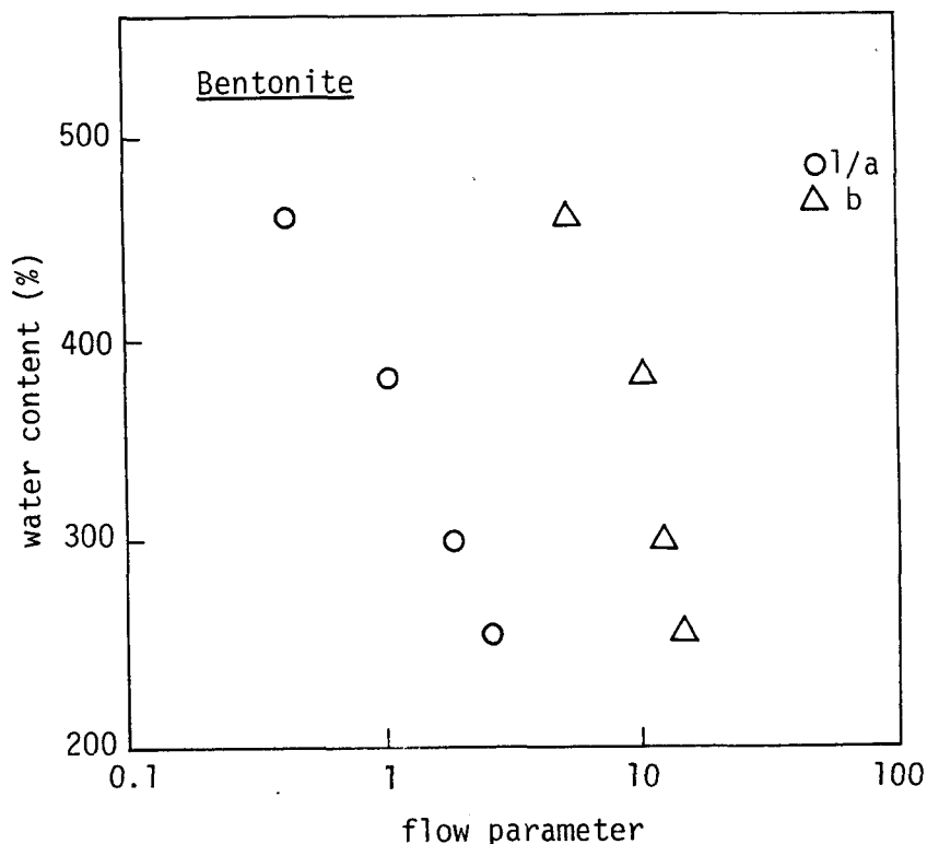
図- 1.2.12 d) ベントナイト
