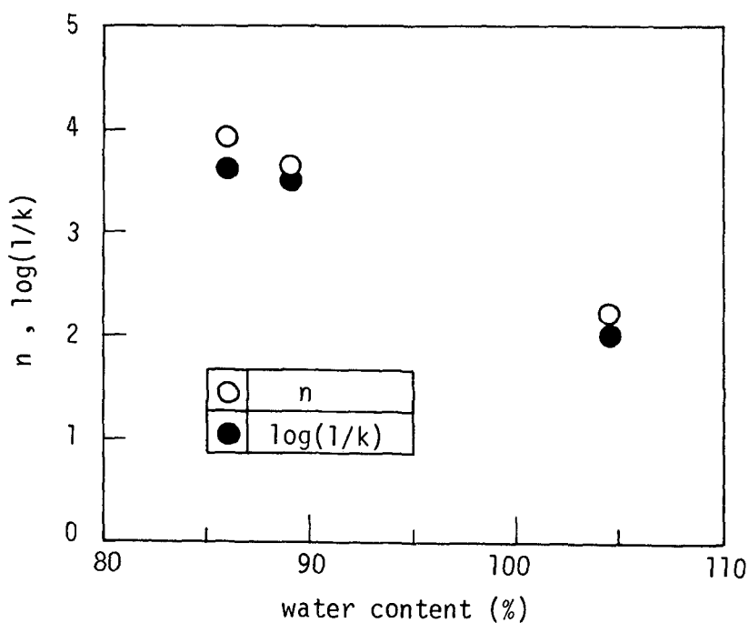
図- 2.1.7 n および \log(1/k) と含水比の関係
