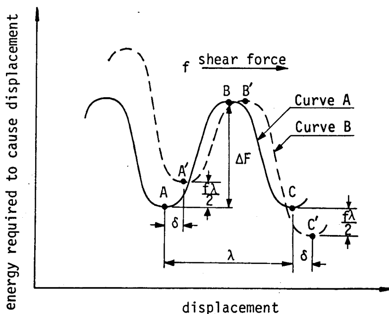
図—1. 2. 5 エネルギー障壁
