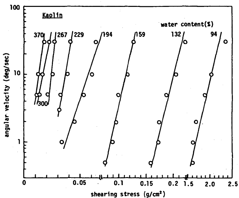
a) カオリン
