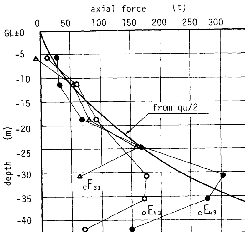
図-2.5.10 軸力分布 (鋼ぐい委 13) 14) )
