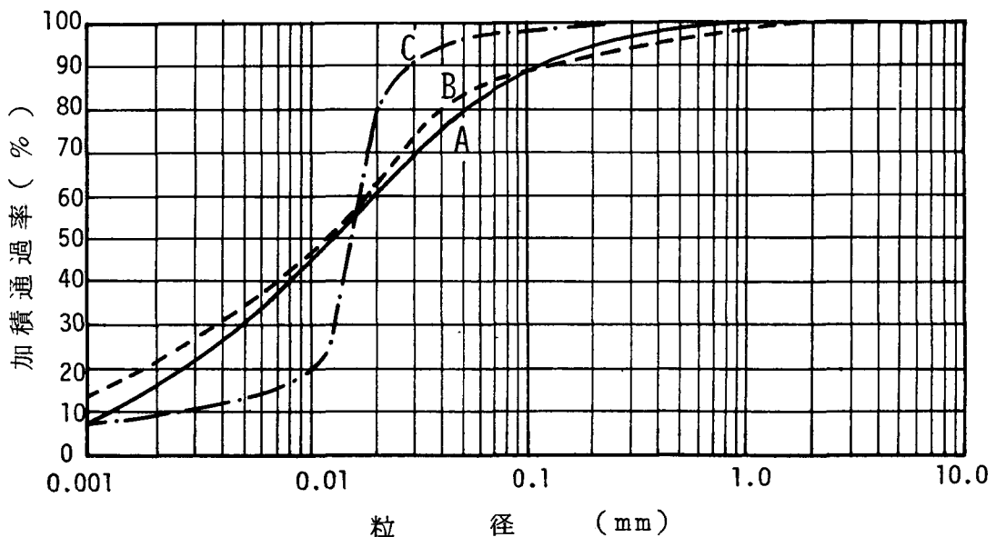
図—2.5.6 粘土試料の粒径加積曲線
