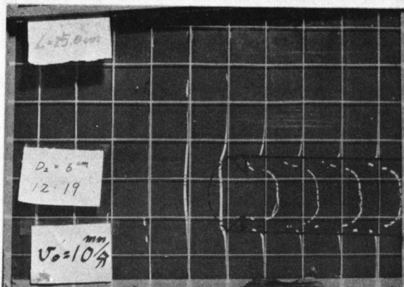
写真 2.3.4 周辺地盤の水平 変位の挙動 ( D_2/D_1 = 0.6 )
