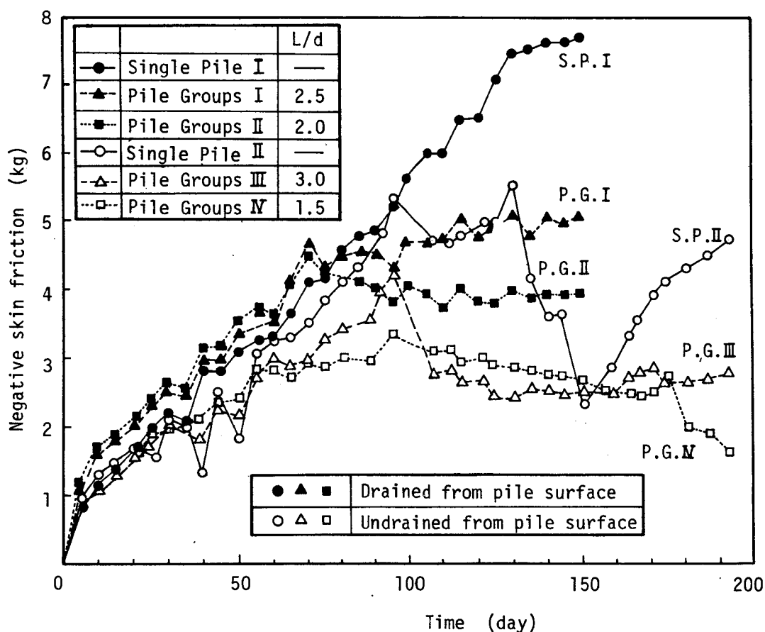
図－2.5.15 ネガティブフリクションの経時変化
