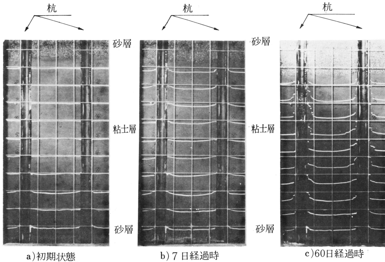
写真 2.5.1 杭周辺地盤の挙動
