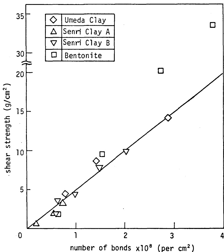
図- 1.2.23 粘土ペーストのせん断強さと結合数の関係
