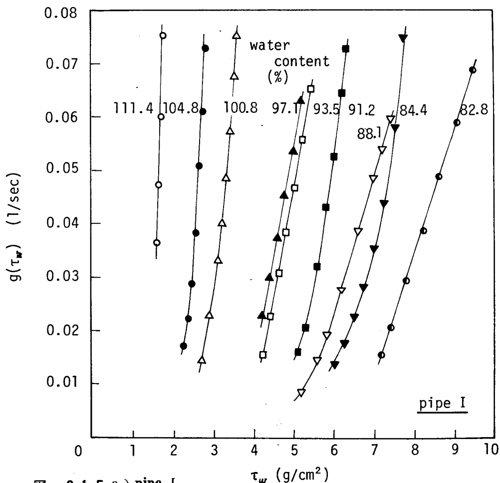
図 - 2.1.5 a) pipe I
