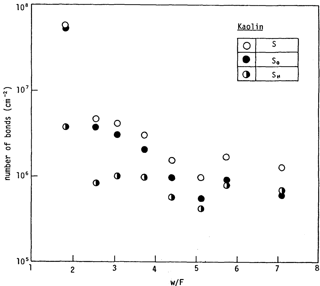
図- 1.4.6 結合数の分布状態 (カオリン)
