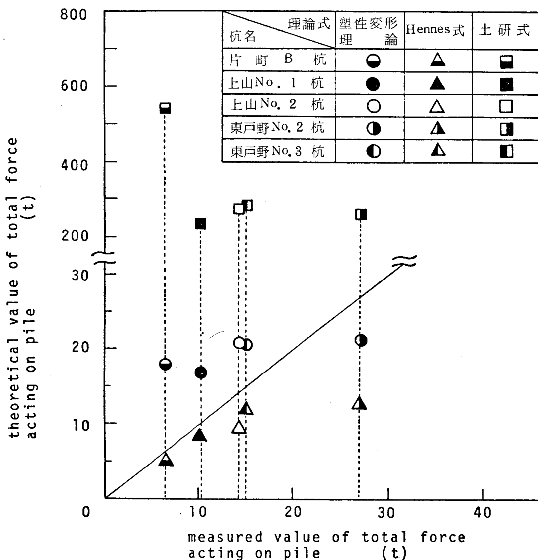
図－2.4.17 塑性地盤中の杭に作用する全合力の実測値と理論値の比較
