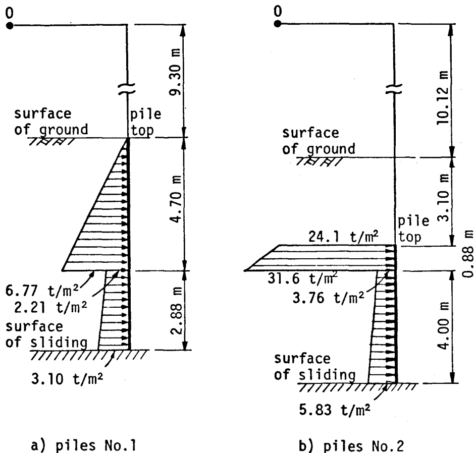
図－2.4.20 杭の反力分布の理論値
