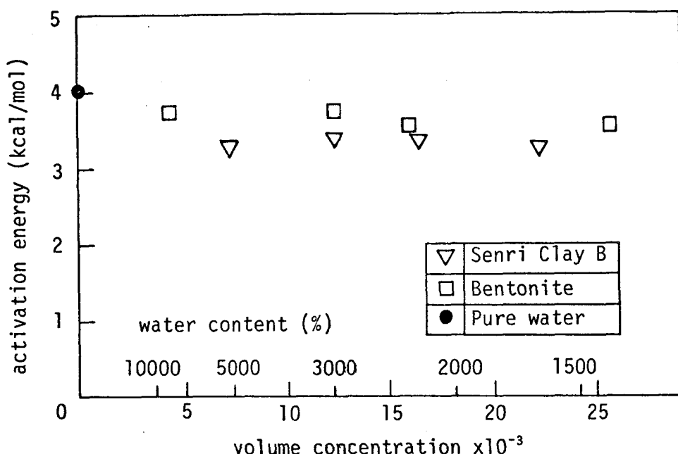
図－ 1.2.16 粘土サスペンションの活性化エネルギーと容積濃度の関係
