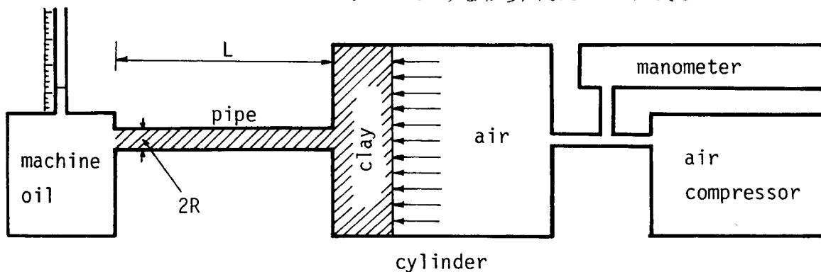
図-2.1.4 実験装置の概略図
