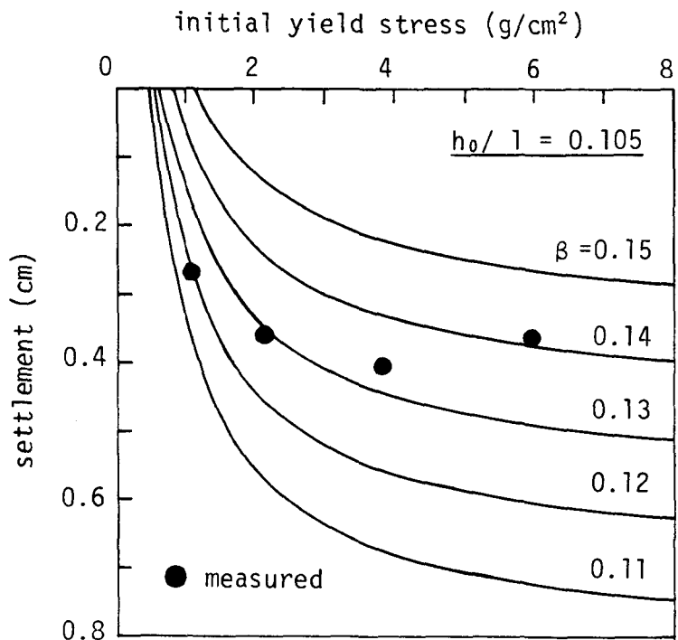
図-2.2.12 最終沈下量の計算値と実測値の比較 ( \tau_{yi} が既知とした場合)
