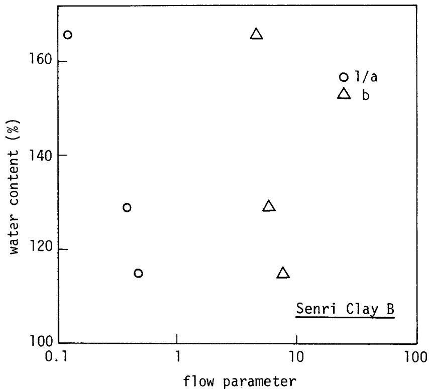
図一 1.2.12 c) 千里粘土B
