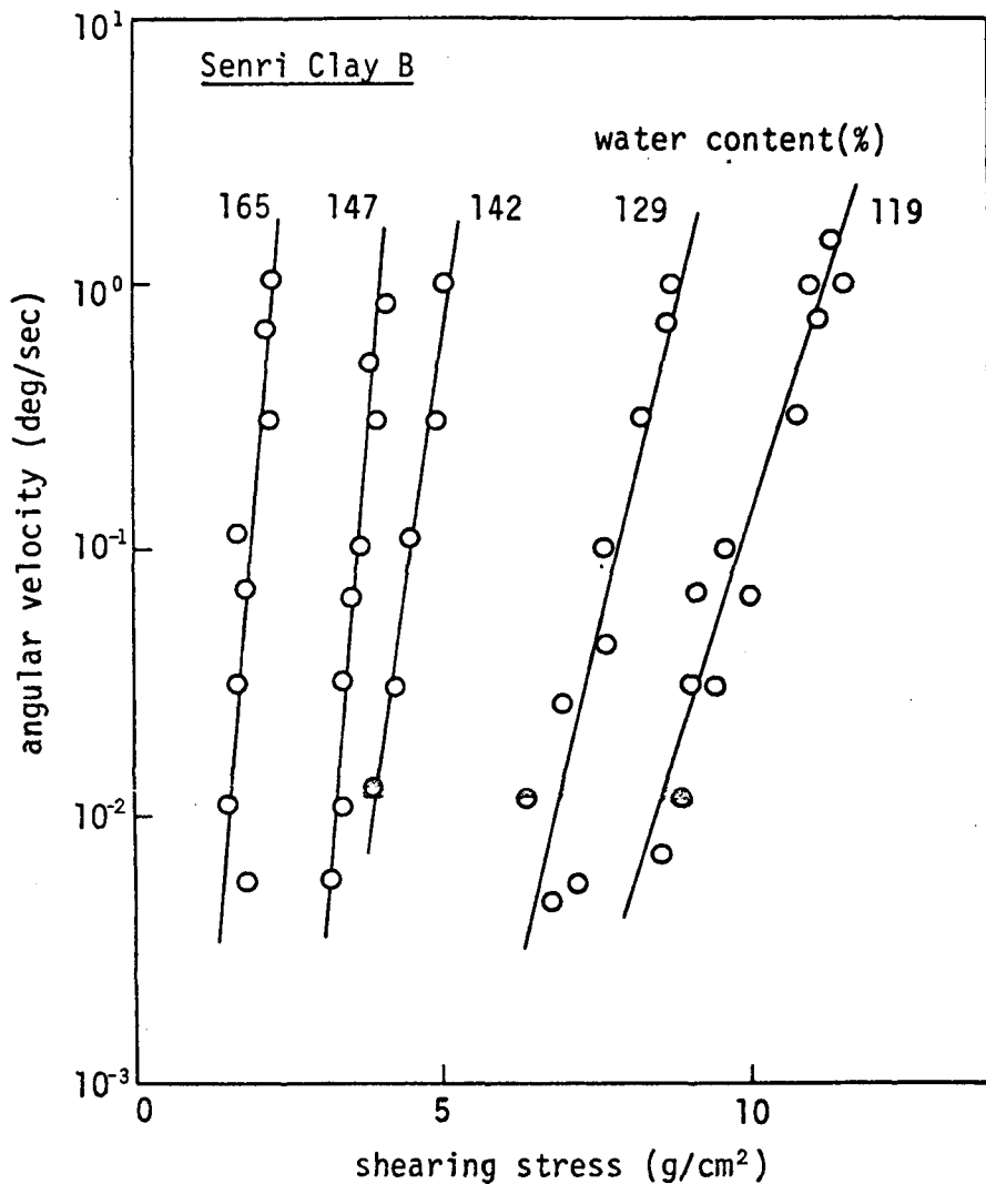
図一 1.2.11c) 千里粘土B
