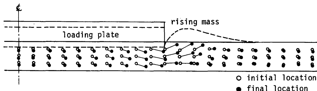
図一 2.2.9 軟弱粘土層の側方流動状態
