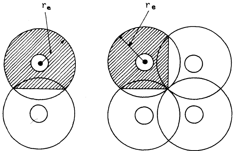
図一 2.5.2 群杭における杭の負担範囲
