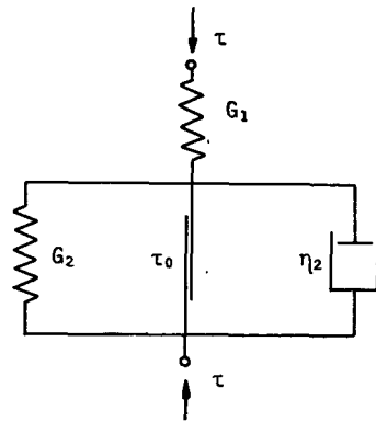
図-1.2.2 力学モデル(村山・柴田)
