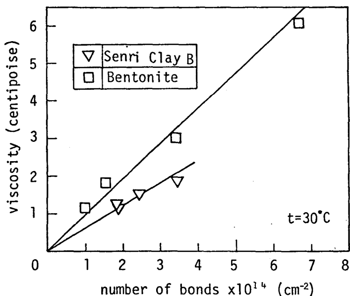
図-1.2.19 粘土サスペンションの粘度と結合数の関係
