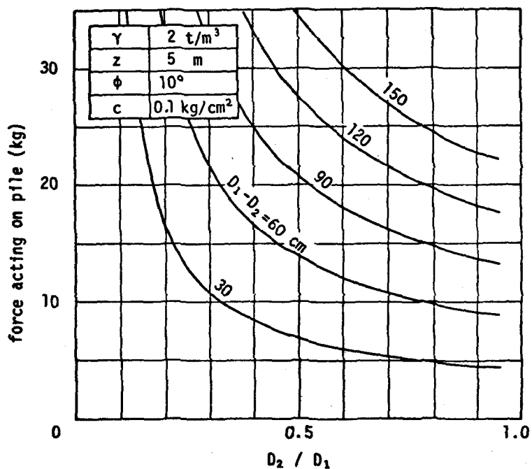
図 - 2.4.12 塑性変形理論式の特徴 (杭径 ( D_1 - D_2 ) の影響)
