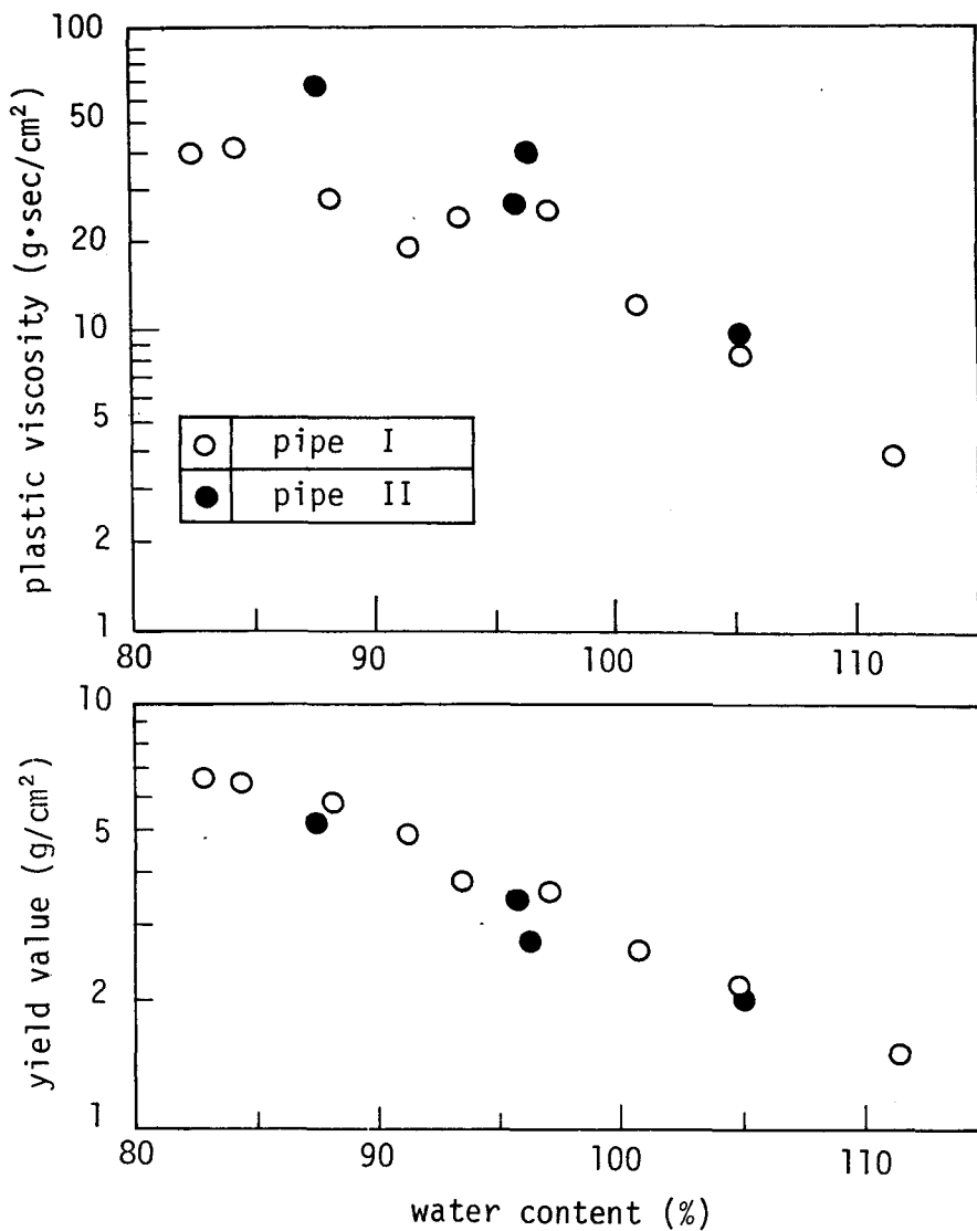
図-2.1.8 pipe I と pipe II による流動特性の比較
