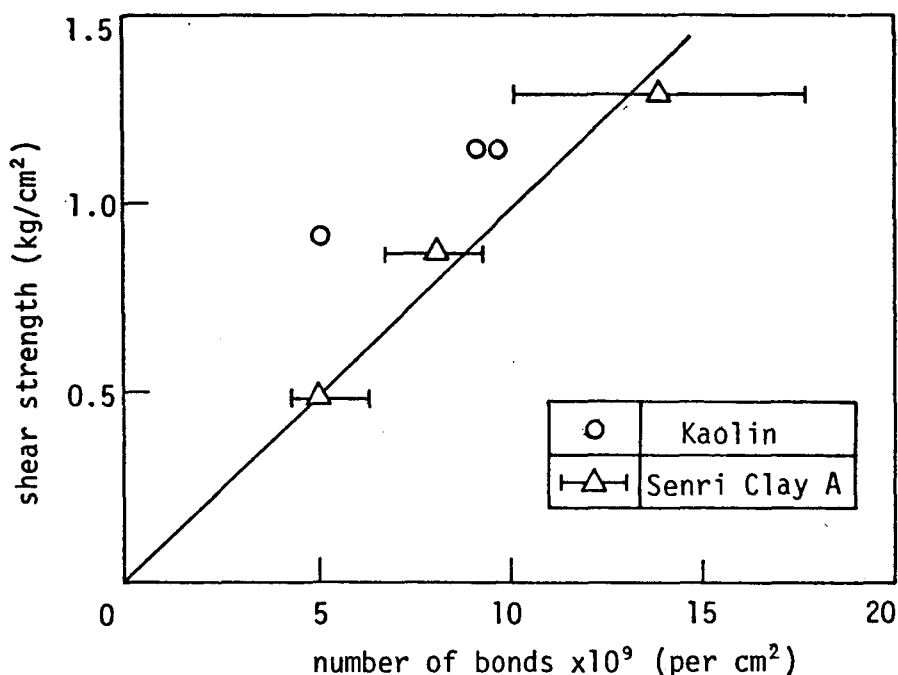
図－ 1. 2. 28 正規圧密粘土のせん断強さと結合数の関係
