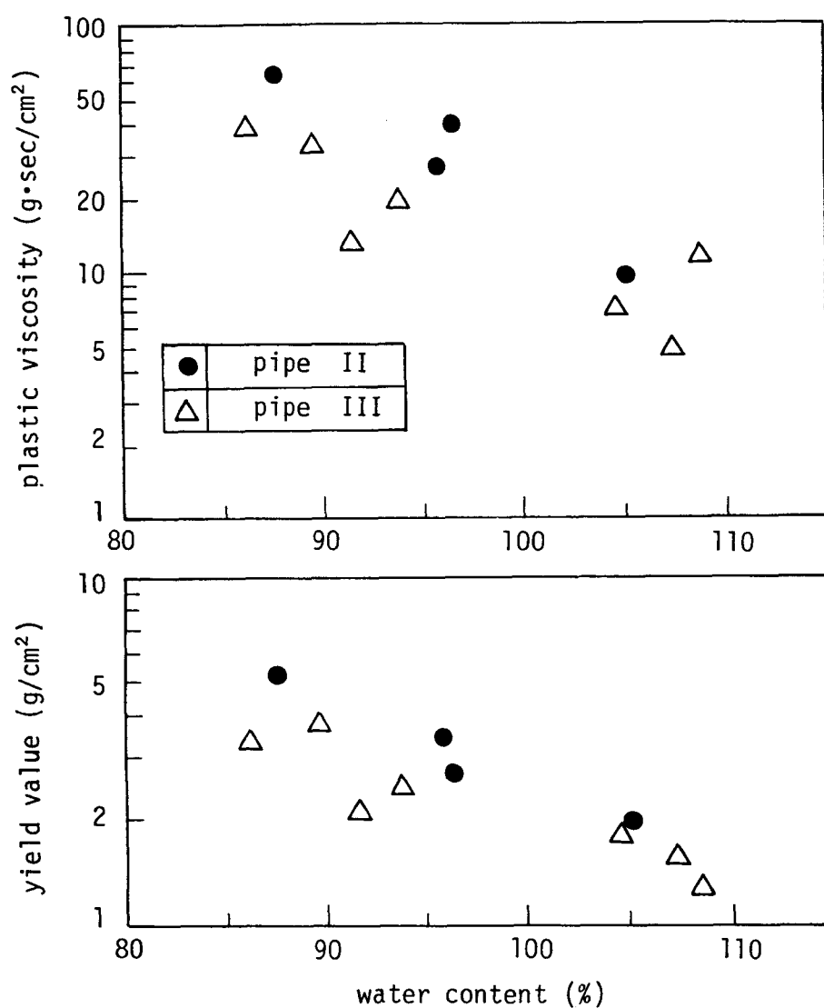
図- 2.1.9 pipe II と pipe III による流動特性の比較
