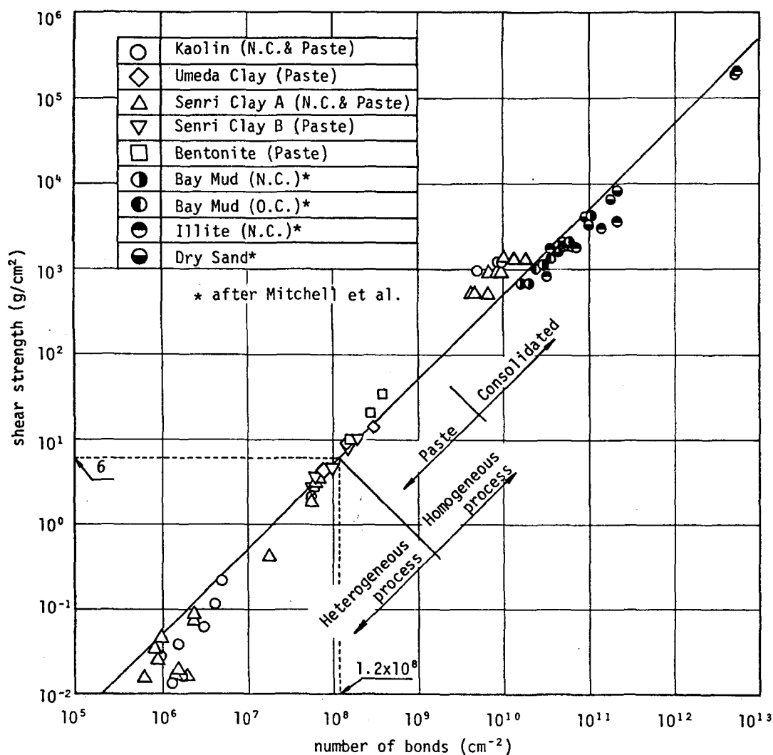
図— 1. 5. 3 広範なコンシステンシー状態の土のせん断強さと結合数の関係
