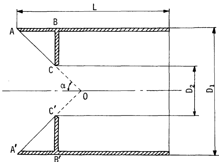
図－2.3.1 ブラインドシールドの断面
