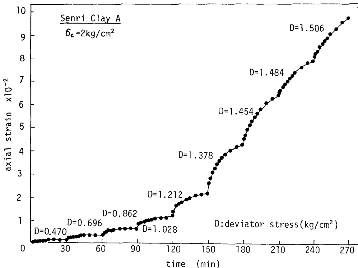
図-1.2.13 Multi-Increment試験における軸ひずみの経時変化
