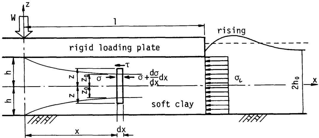
図－ 2.2.4 軟弱粘土層の応力状態
