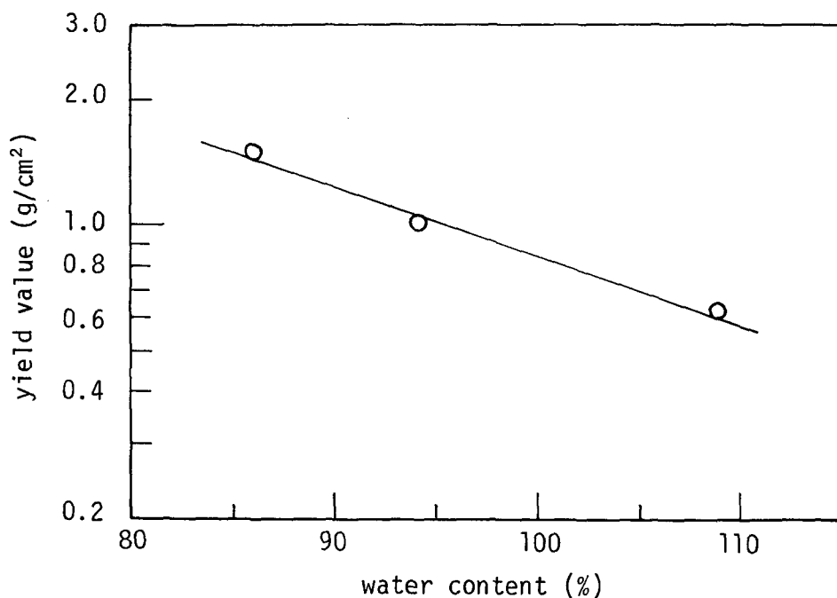
図- 2.1.6 \tau_y と含水比の関係
