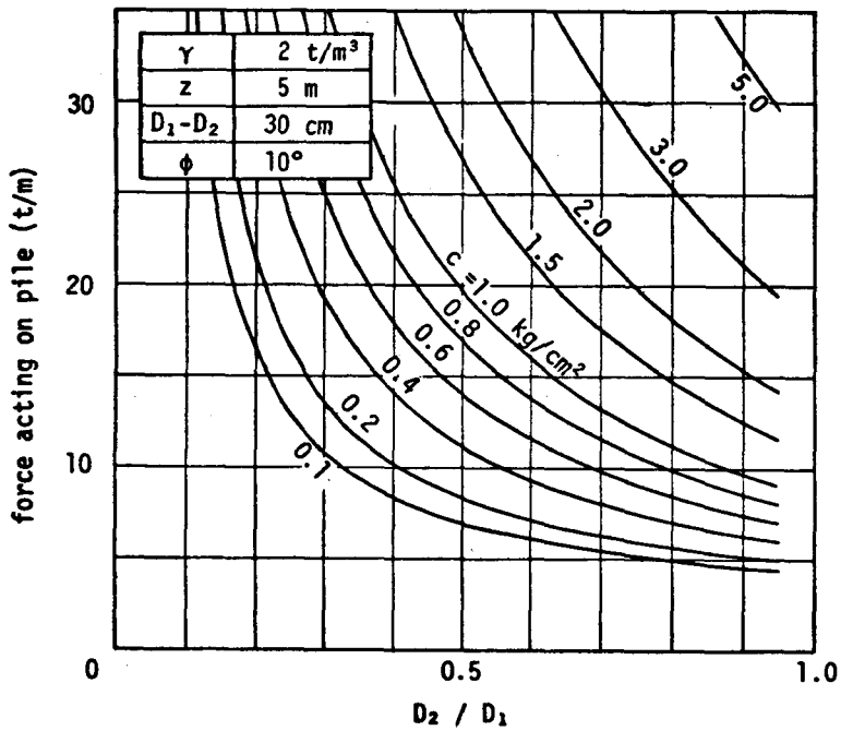
図 - 2.4.11 塑性変形理論式の特徴 (粘着力 c の影響)
