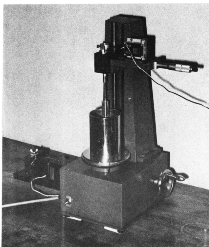
写真 1.4.1 ベーン型プラストメーター
