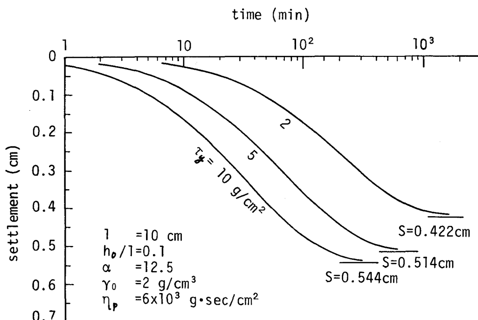
図－2.2.6 沈下量の経時変化の理論的特性
