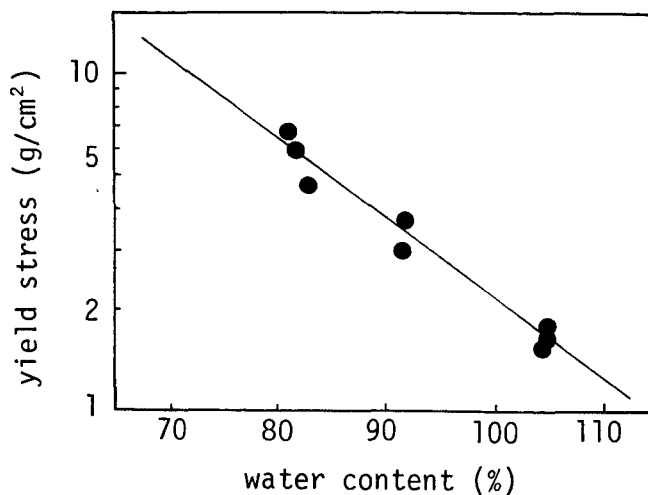
図一2.2.10 降伏応力 \tau_y と含水比 w の関係
