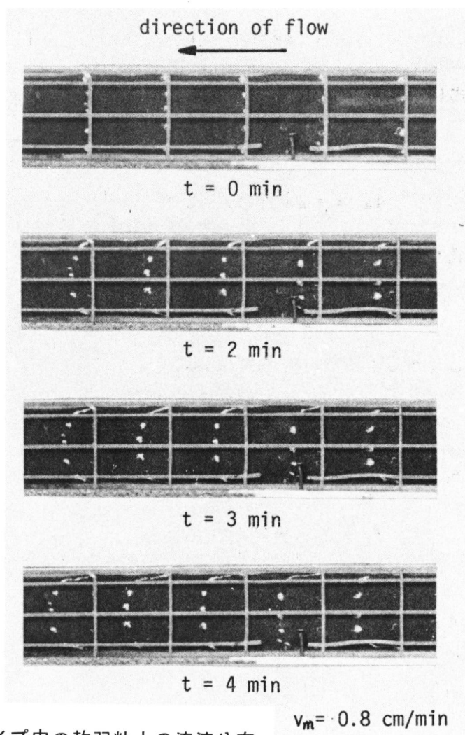
写真-2.1.1 矩形パイプ中の軟弱粘土の流速分布
