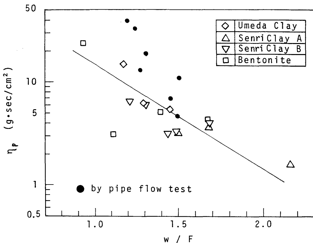
図 - 2.1.11 b) \eta_p と w/F の関係
