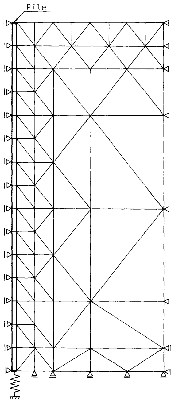
図－2.5.19 要素分割
