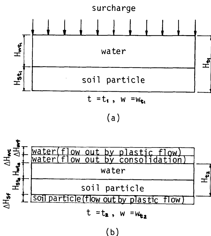
図一2.2.1 載荷重下の軟弱粘土層の模式図
