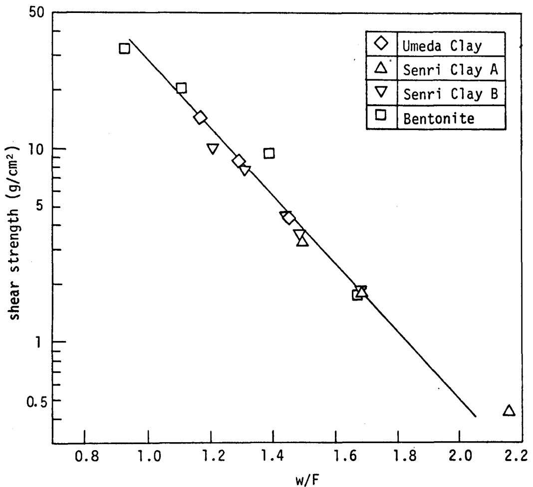
図— 1. 2. 22 粘土ペーストのせん断強さと含水比の関係
