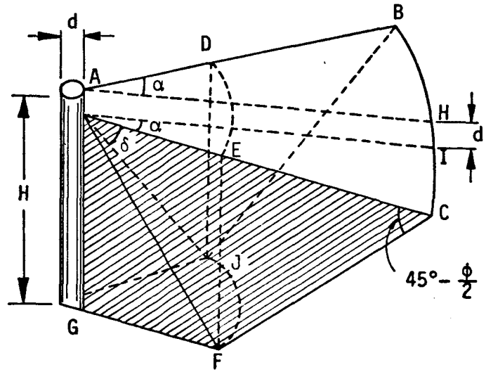
図-2.4.2 杭による地盤のせん断破壊
