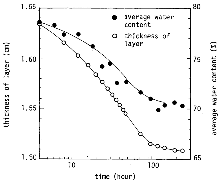
図－2.2.2 粘土層厚および平均含水比の経時変化
