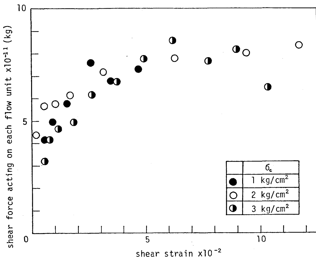
図-1.6.3 流動単位に作用するせん断力とせん断ひずみの関係
