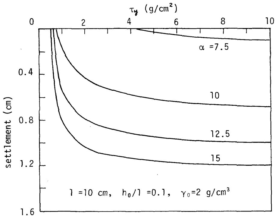
b) 沈下量と \tau_y の関係
