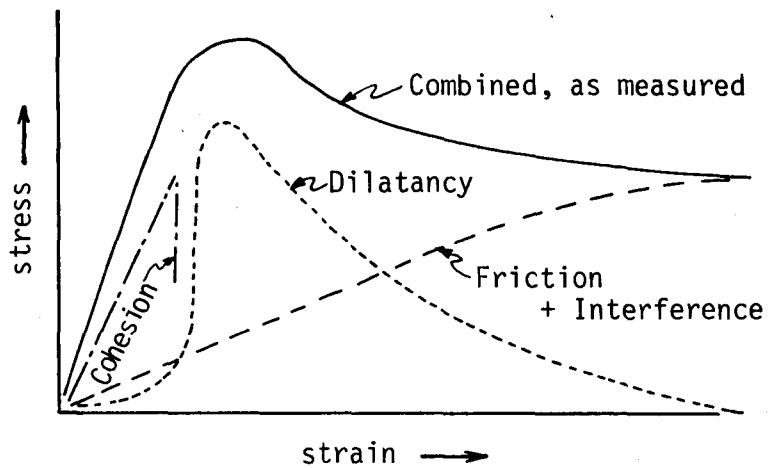
図—1. 2. 1 せん断抵抗力の成分
