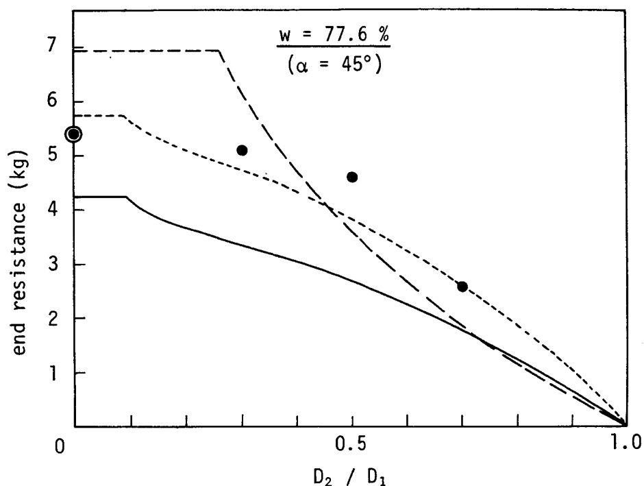
図-2.3.13 先端抵抗力の理論値と実験値の比較 (sample B)
