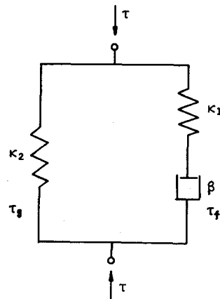
図-1.2.4 力学モデル (Christensen・Wu)
