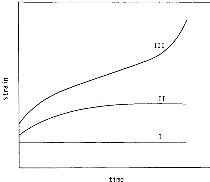
図-2.1.1 一定応力下におけるひずみと時間の関係
