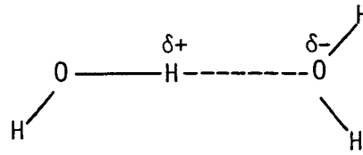
図- 1.2.17 水分子の水素結合
