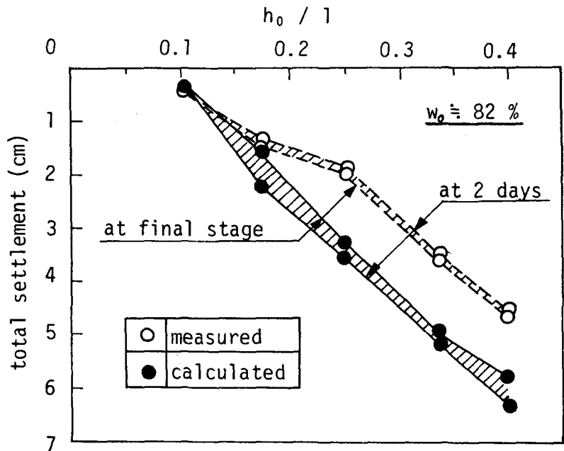
図-2.2.12 最終沈下量の計算値と実測値の比較 ( \tau_{yi} が既知とした場合)
