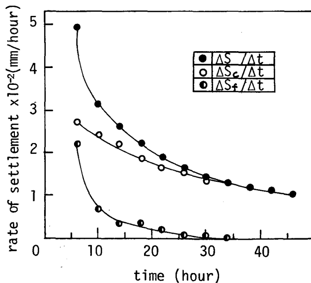
図－2.2.3 沈下速度の経時変化
