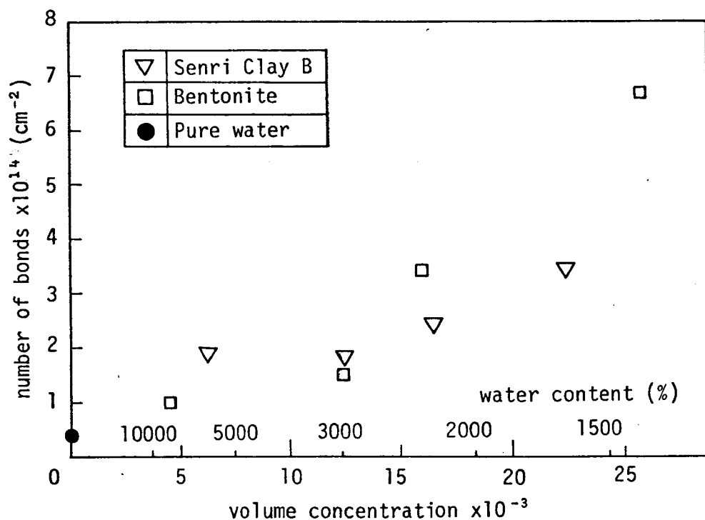
図－1.2.18 粘土サスペンションの結合数と容積濃度の関係
