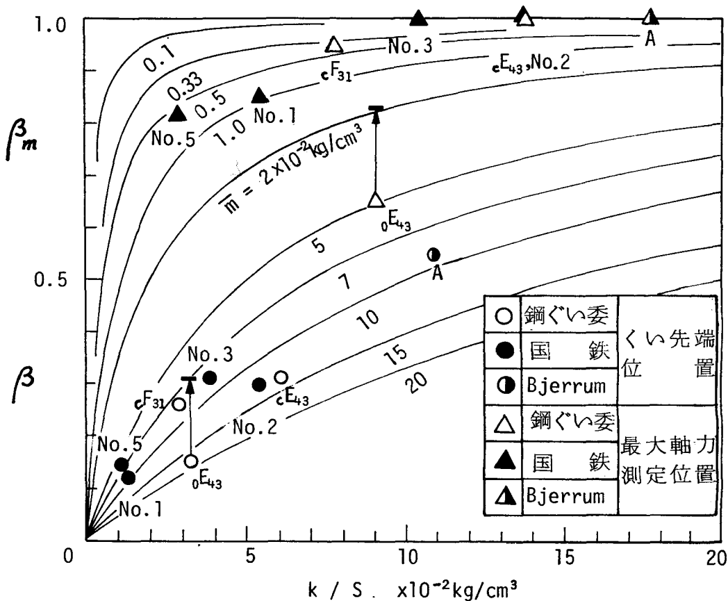
図-2.5.13 \beta , \beta_m と k/S の関係
