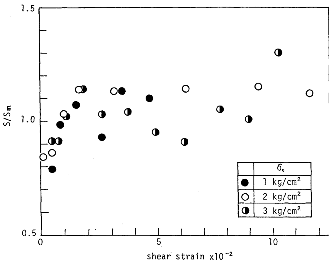
図－1.6.2 結合数とせん断ひずみの関係
