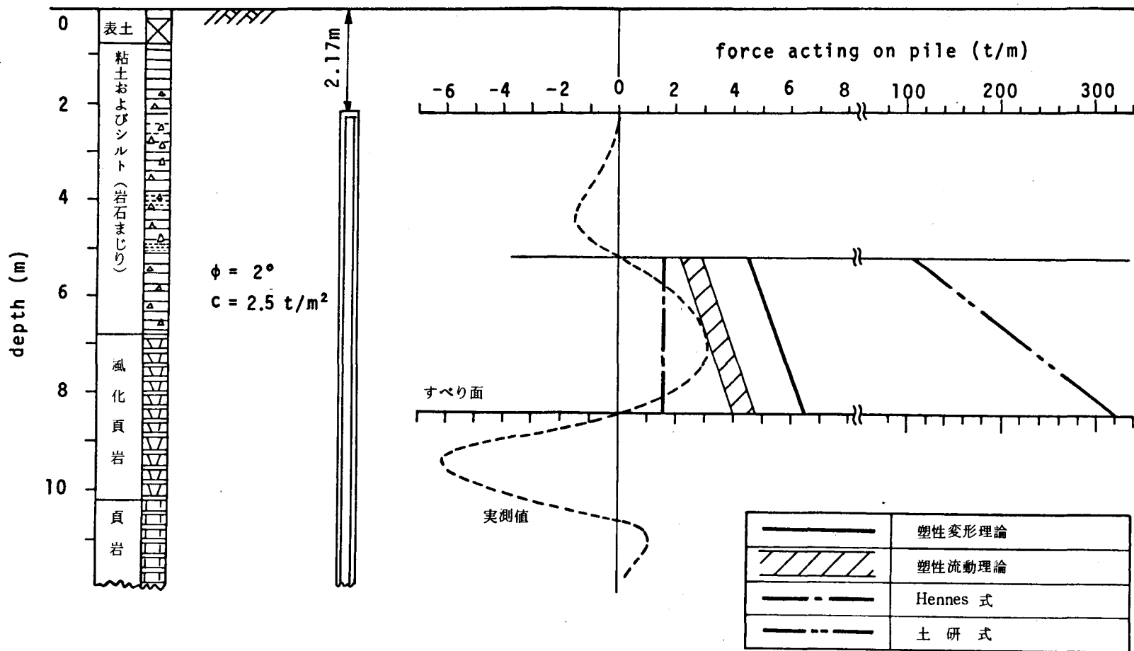
図-2.4.16a) 片町地すべり地B杭
