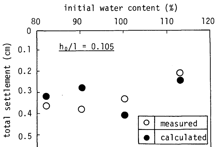
図一2.2.11 最終沈下量の計算値と実測値の比較 ( \tau_{yi} が既知とした場合)
