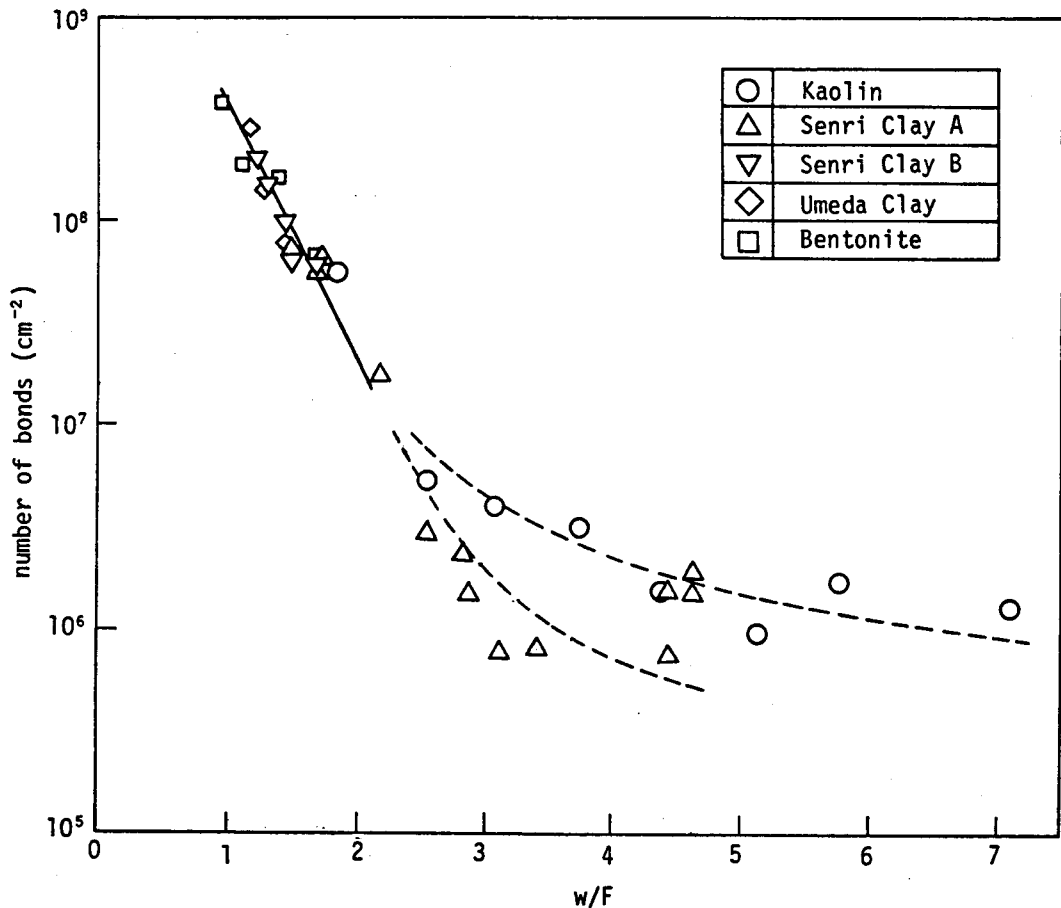
図一 1.4.4 結合数と含水比の関係
