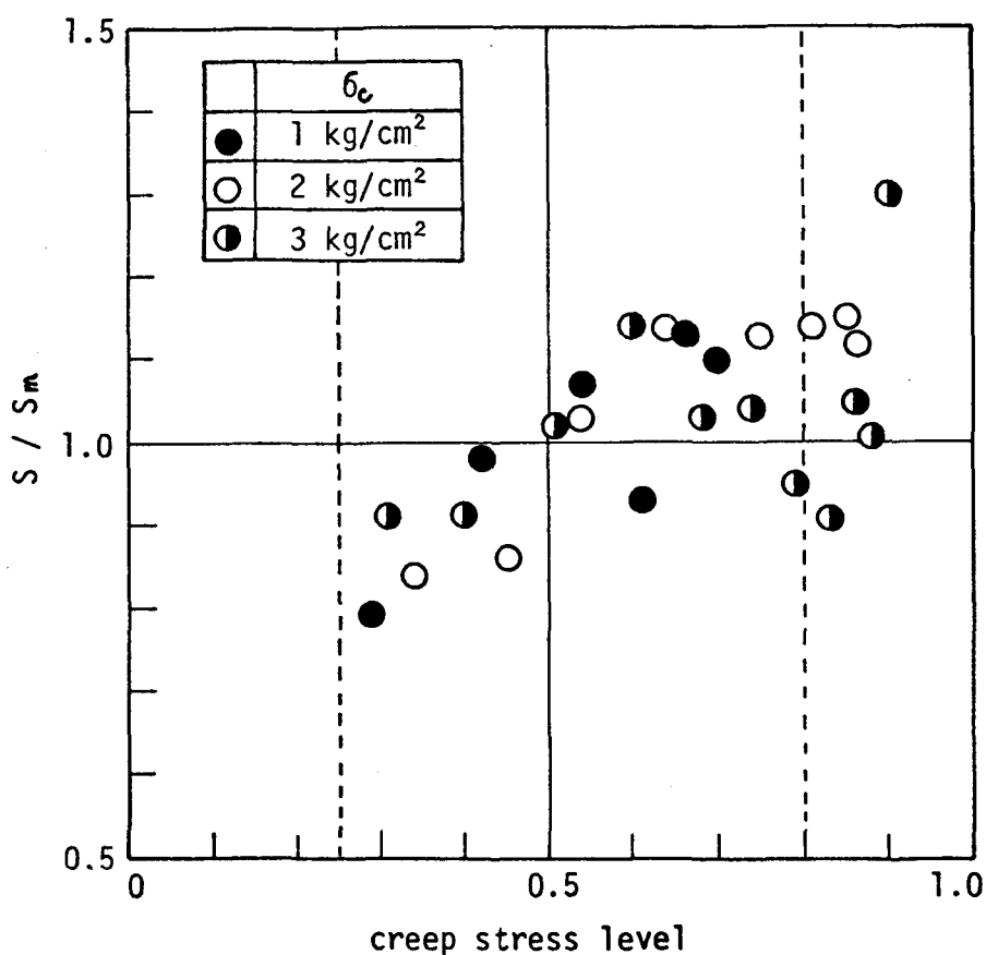
図－ 1. 2. 25 正規圧密粘土の結合数と応力レベルの関係
