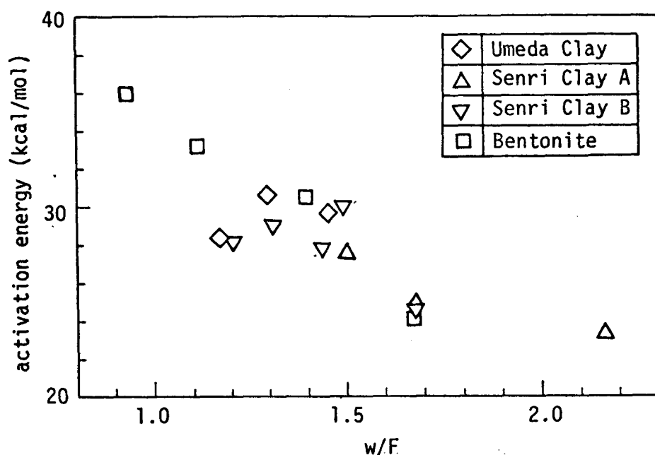
図- 1.2.20 粘土ペーストの活性化エネルギーと含水比の関係
