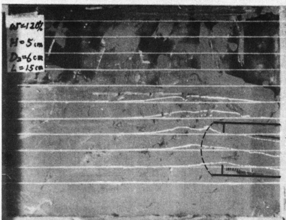
写真 2.3.5 周辺地盤の鉛直 変位の挙動 ( H = 5 \text{ cm} )
