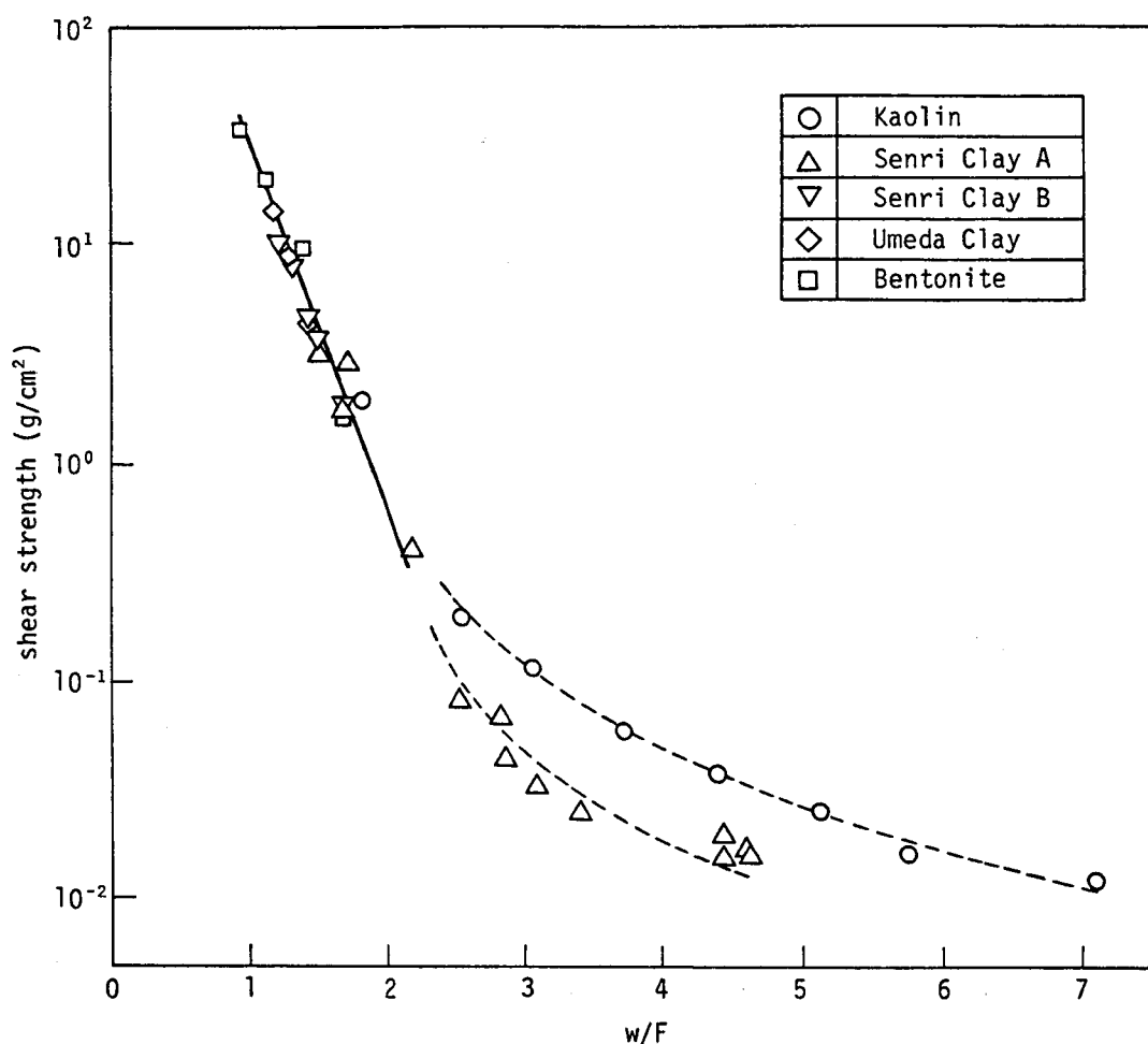
図－1.4.5 せん断強さと含水比の関係
