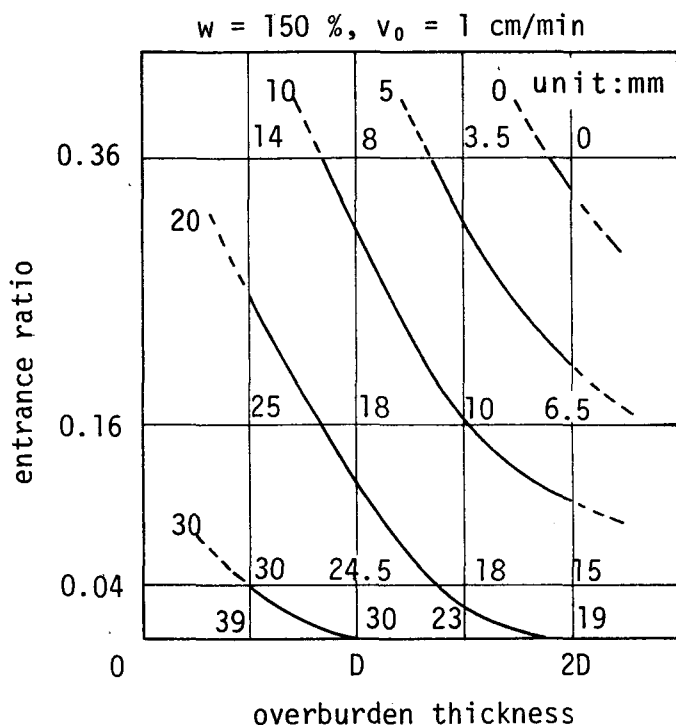
図－2.3.9 地表面の最大盛り高 ( w=150\% )
