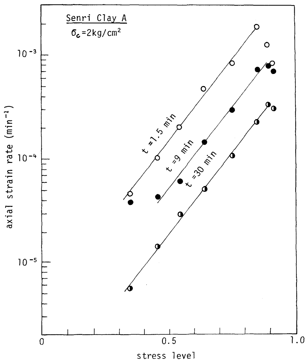
図-1.2.14 ひずみ速度と応力レベルの関係
