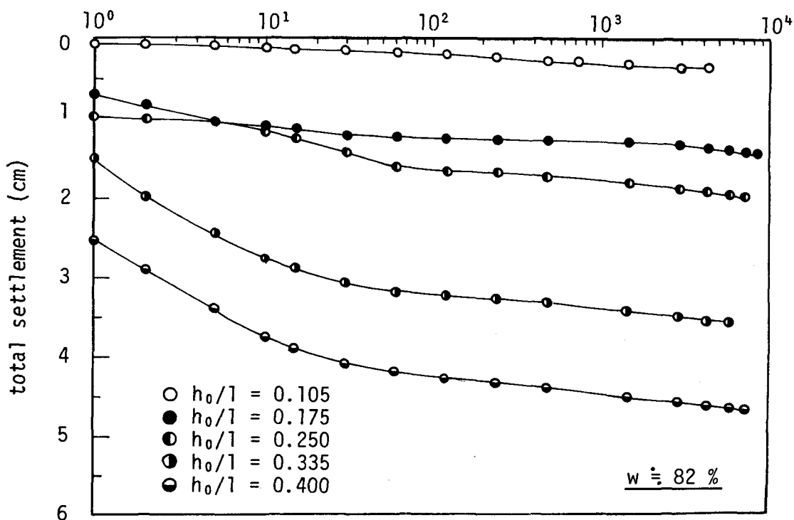
b) 初期層厚を変化させた場合
