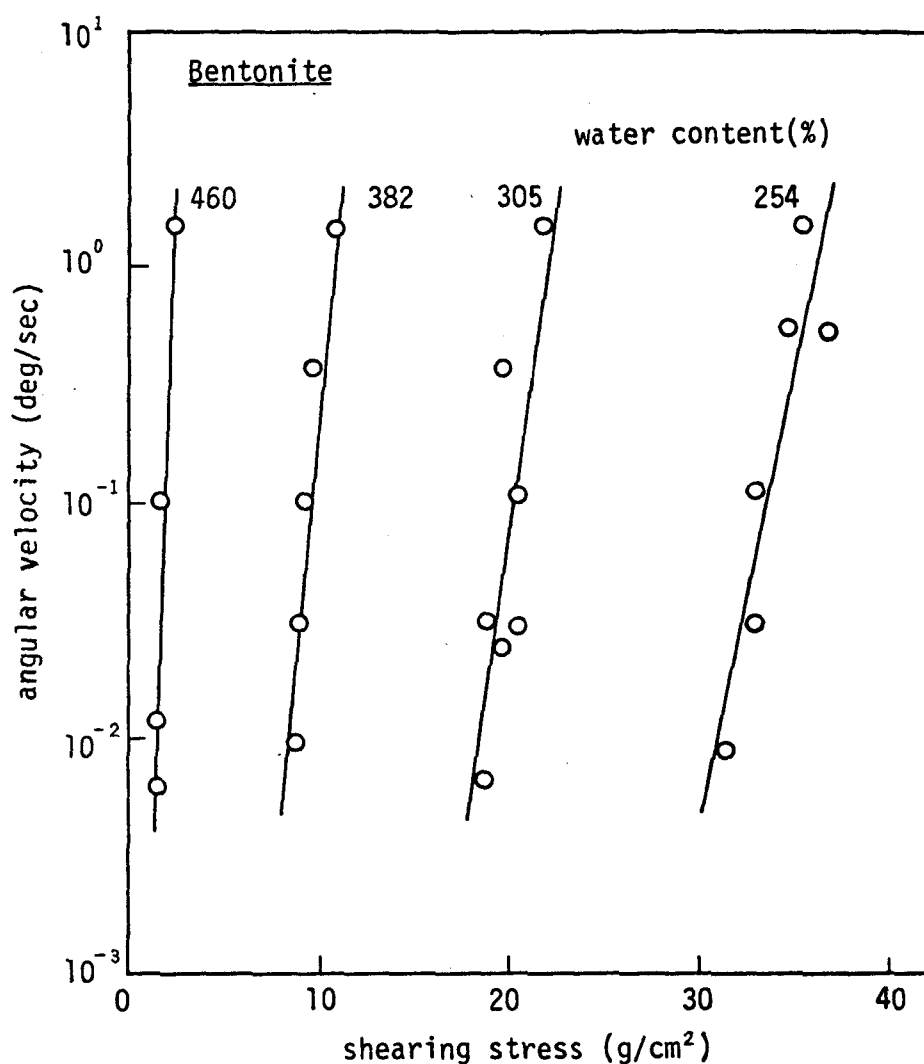
図- 1.2.11 d) ベントナイト
