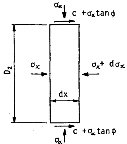
図-2.4.6 塑性変形地盤の微小要素(土塊A E E' A')
