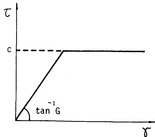
図一2.5.18 応力-ひずみ関係
