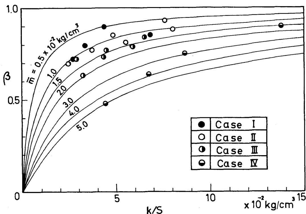
図-2.5.8 \beta と k/S の関係
