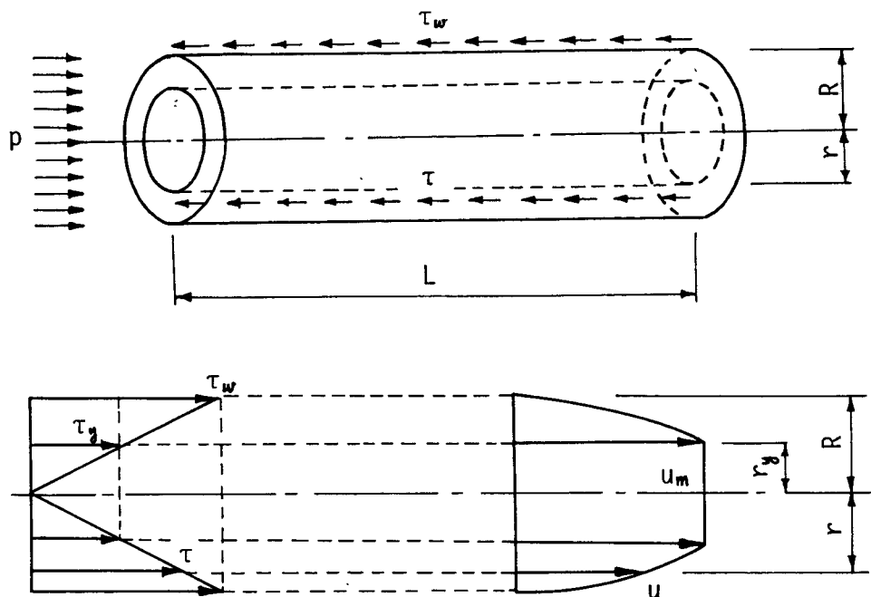
図－ 2.1.2 管内流動における流速およびせん断応力の分布
