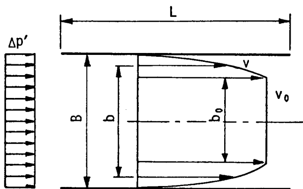
図-2.4.8 底面滑らかなチャンネル内の塑性流動
