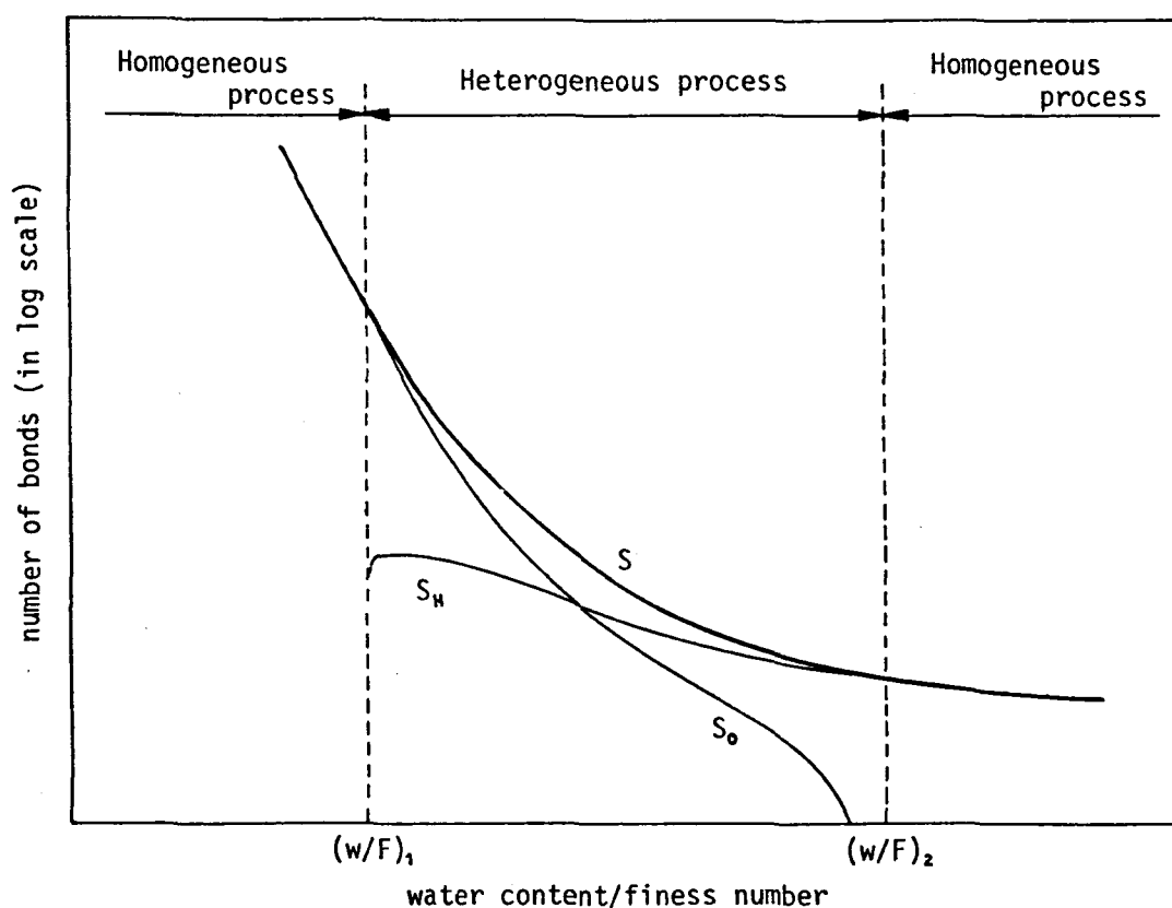
図— 1.5.2 結合数と含水比の関係の統一的表示
