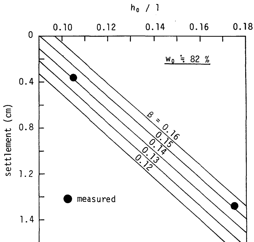
図－2.2.14 最終沈下量の計算値と実測値の比較 ( \tau_{yi} が未知の場合)
