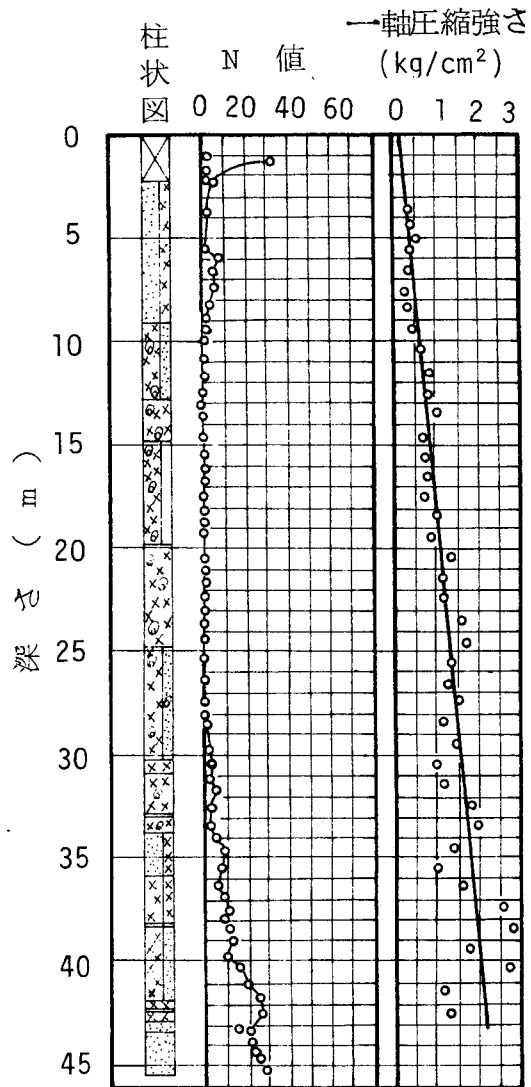
図— 2.5.20 土層断面
