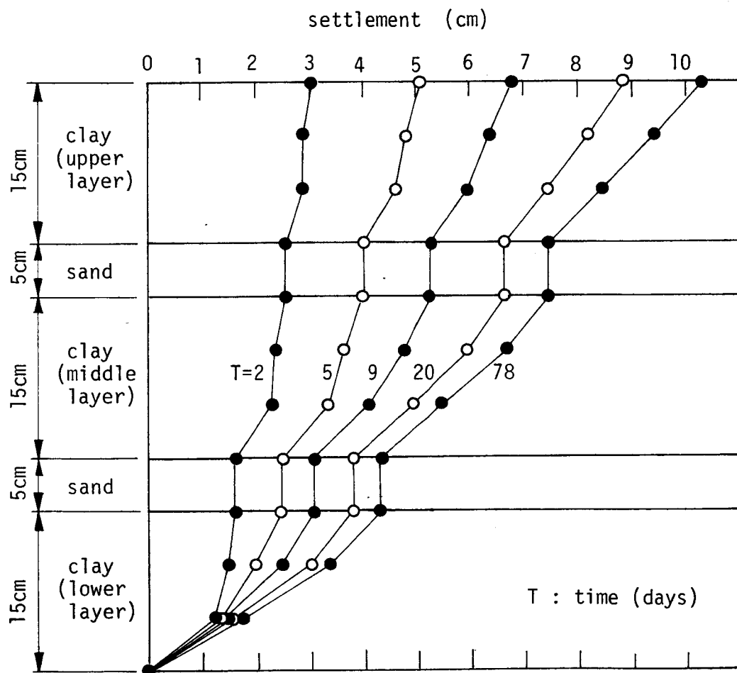
図－ 2.5.9 粘土層内部の沈下量
