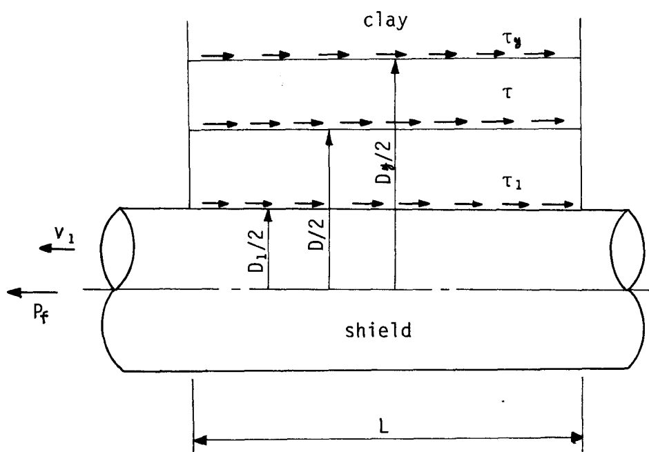
図－2.3.2 シールド周面付近のせん断応力
