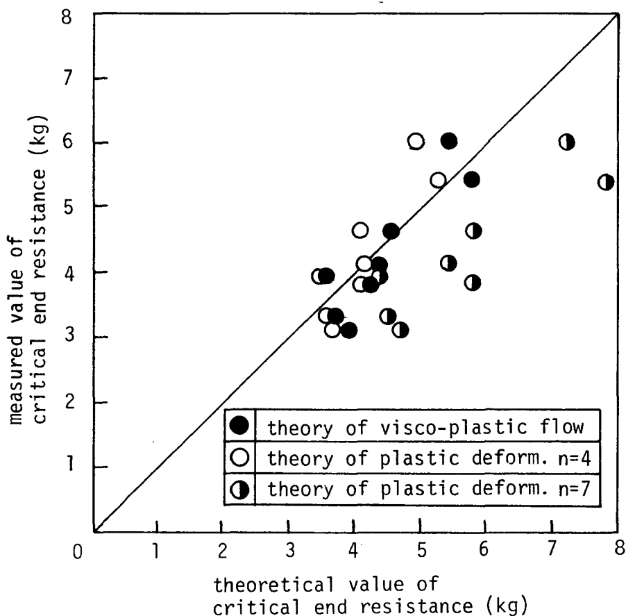
図-2.3.14 限界先端抵抗力の理論値と実験値の比較
