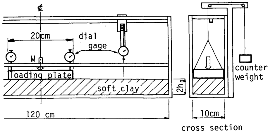
図－ 2.2.7 実験装置の概略図
