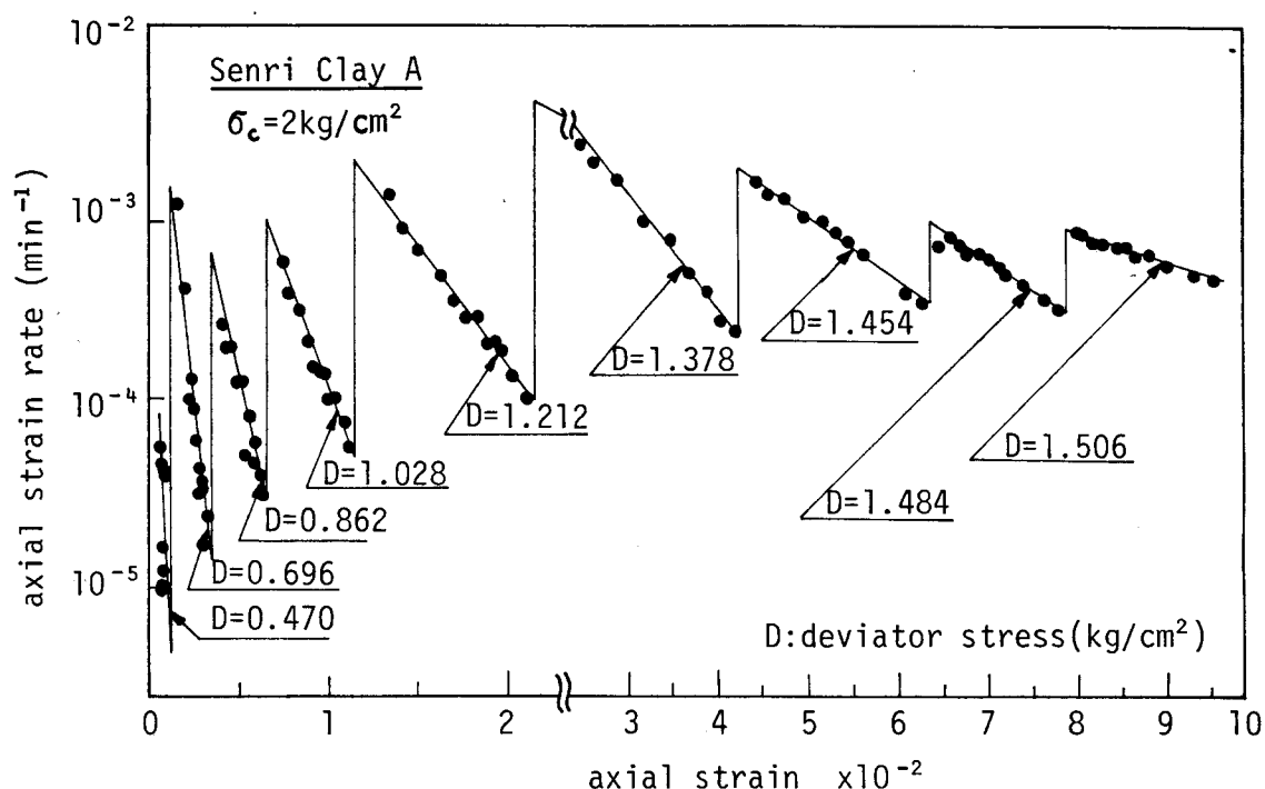
図- 1.2.15 ひずみ速度とひずみの関係
