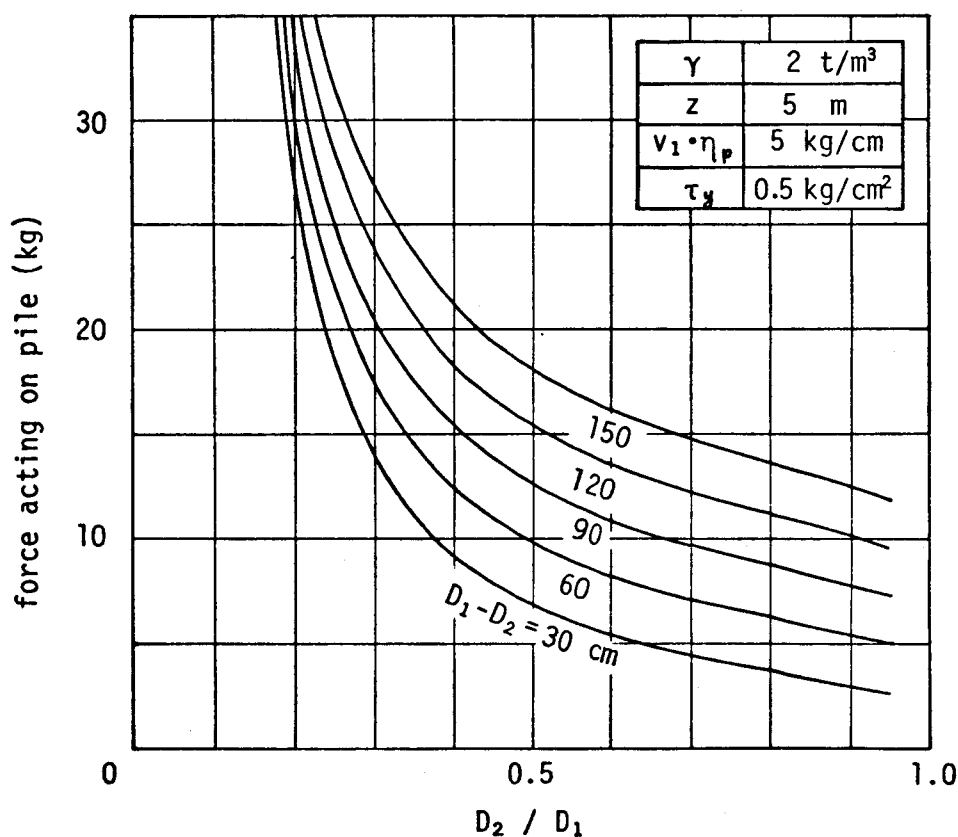
図－2.4.15 塑性流動理論式の特性（杭径（ D_1 - D_2 ）の影響）
