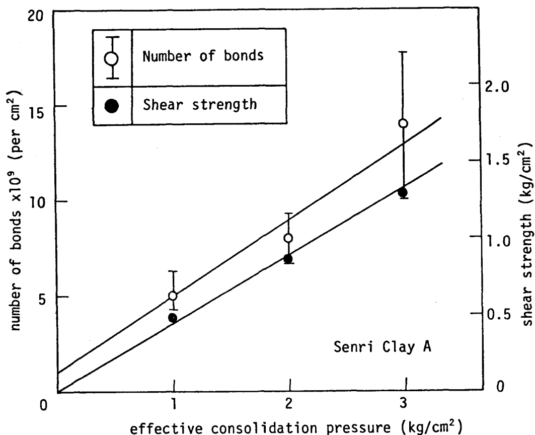
図－1.2.27 正規圧密粘土の結合数およびせん断強さと圧密圧力の関係
