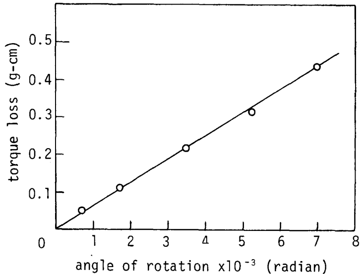
図-1.4.1 ペーン軸の摩擦によるトルクの損失量
