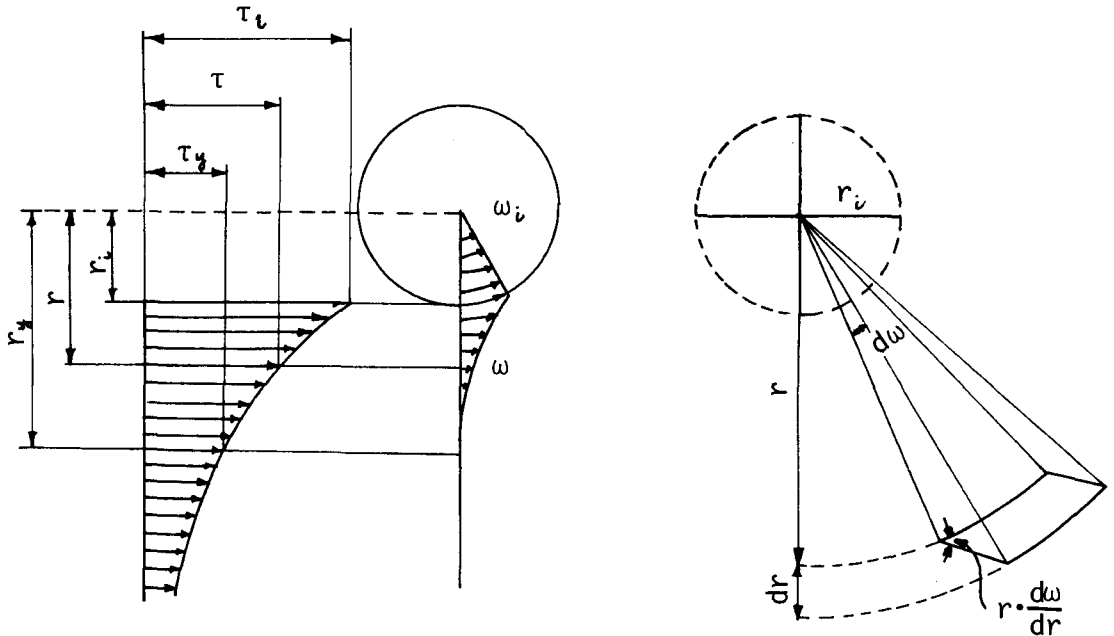
a) 流速およびせん断応力の分布
