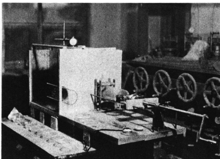
写真 2.3.1 実験装置
