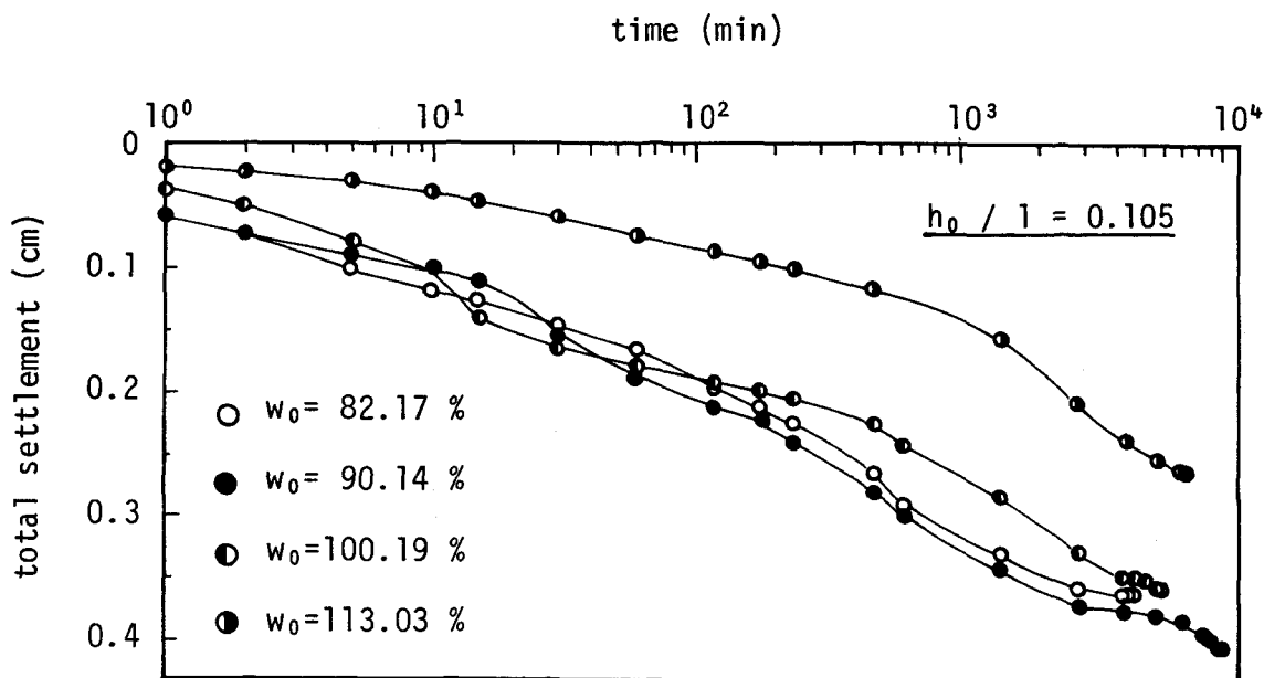
a) 初期含水比を変化させた場合 time (min)
