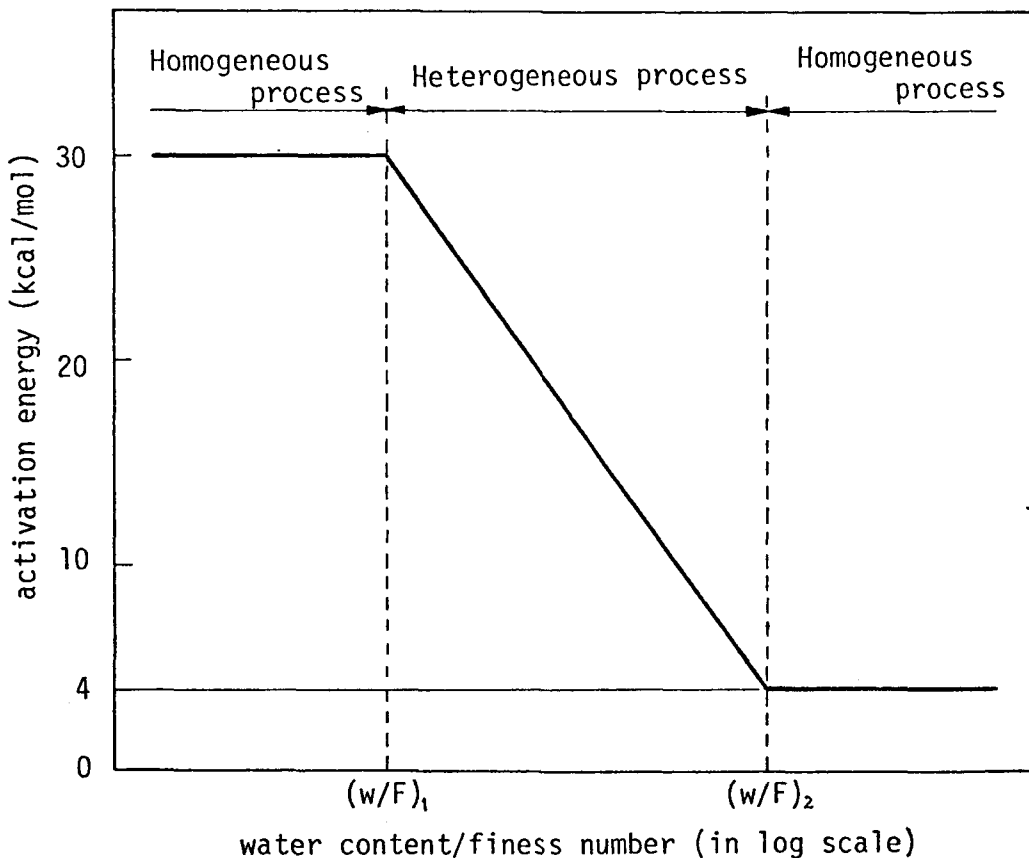
図－1.5.1 活性化エネルギーと含水比の関係の統一的表示
