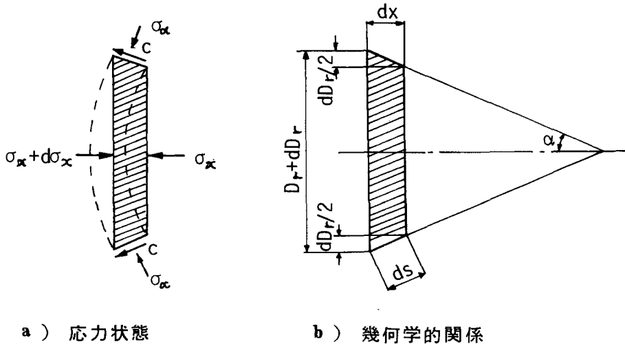
図-2.3.5 ブラインドシールド先端部の粘土の微小要素
