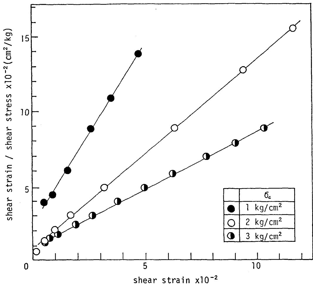
図-1.6.5 \gamma/\tau と \gamma の関係
