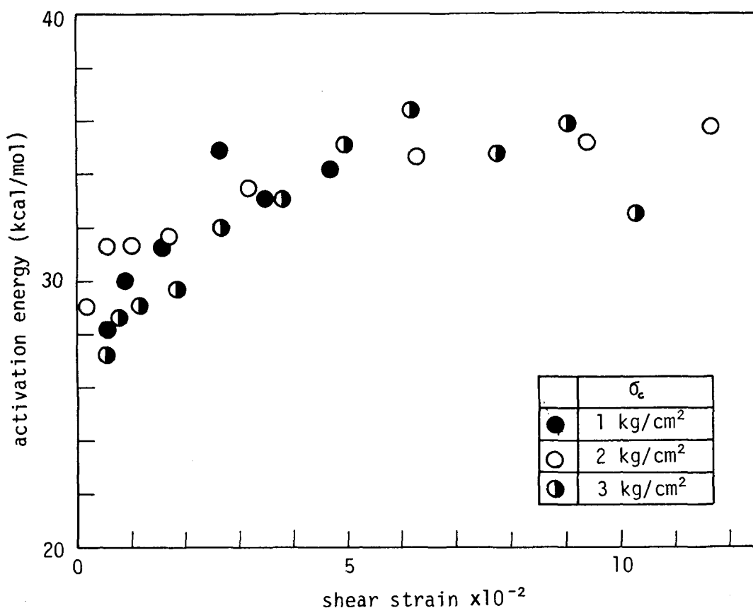
図-1.6.1 活性化エネルギーとせん断ひずみの関係
