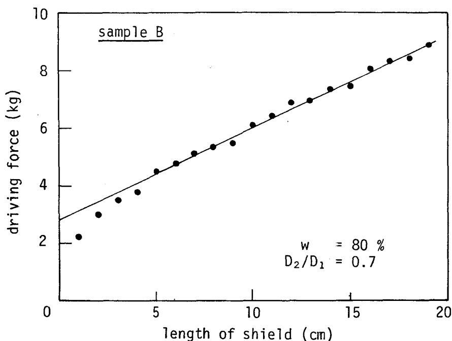
図－ 2.3.10 ブラインドシールドの推進力と貫入長の関係
