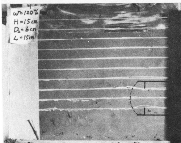
写真 2.3.6 周辺地盤の鉛直 変位の挙動 ( H = 15\text{ cm} )
