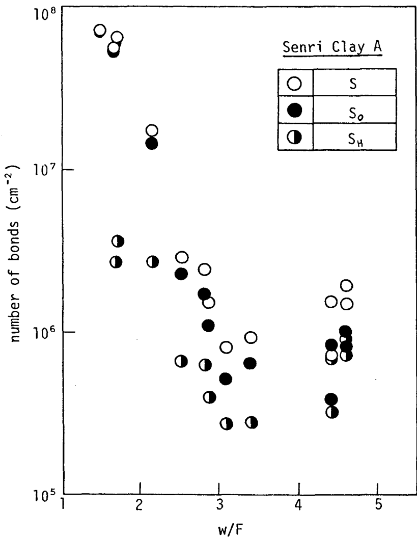
図－1.4.7 結合数の分布状態（千里粘土 A）
