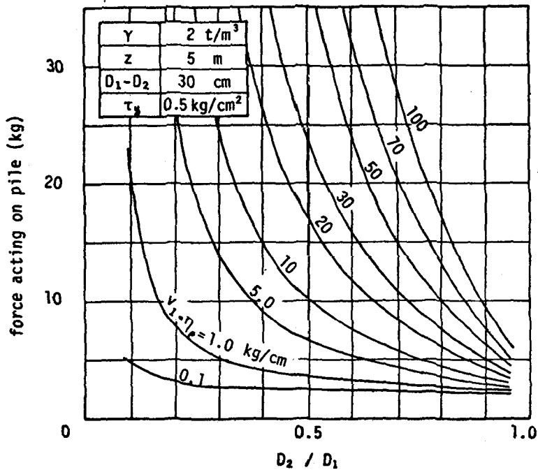
図 - 2.4.13 塑性流動理論式の特徴 (流動速度と塑性粘度の積 ( v_1 \cdot \eta_p ) の影響)
