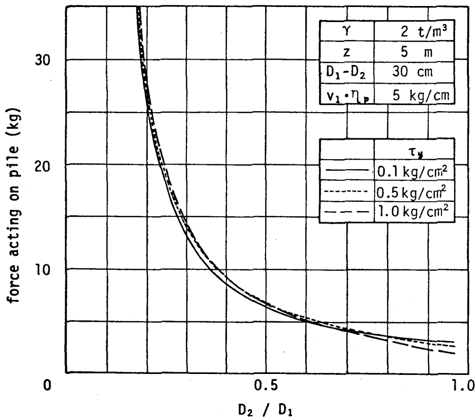
図－ 2.4.14 塑性流動理論式の特性（降伏応力 \tau_y の影響）
