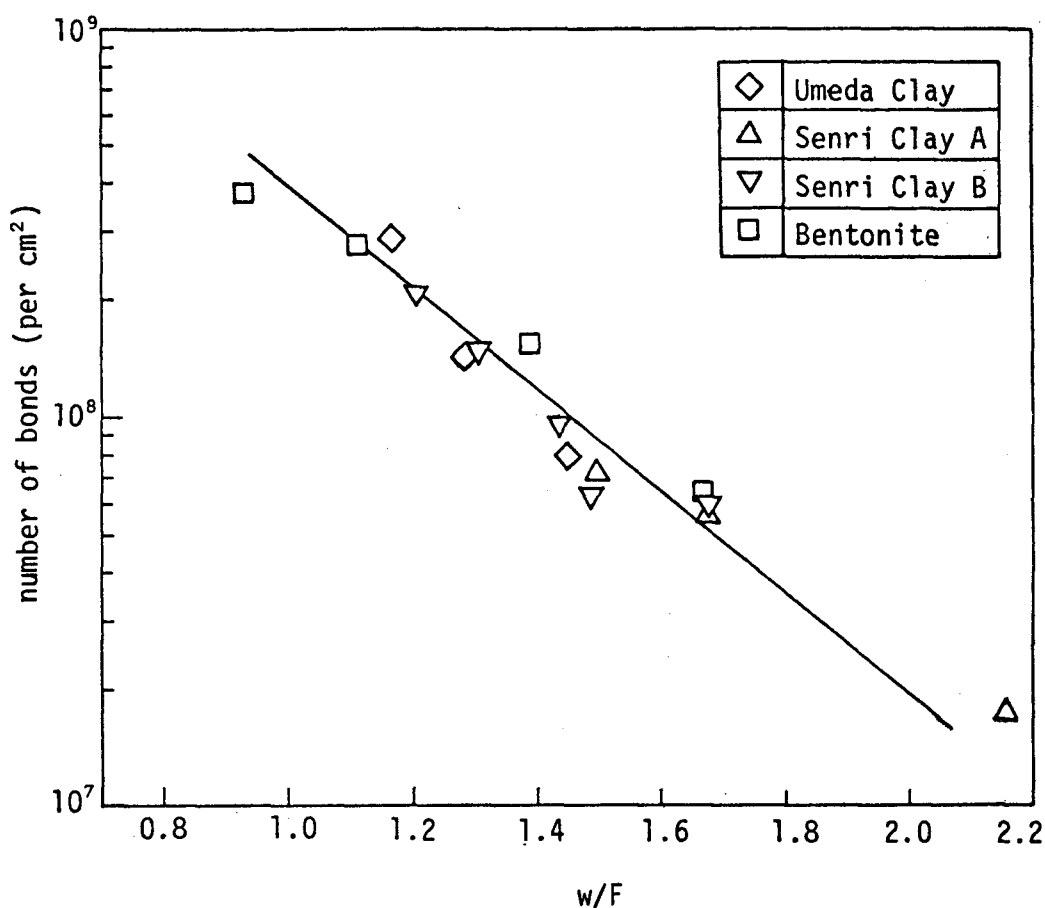
図－ 1.2.21 粘土ペーストの結合数と含水比の関係
