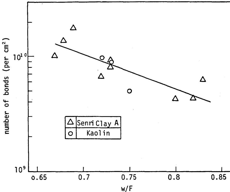
図－ 1. 2. 26 正規圧密粘土の結合数と含水比の関係
