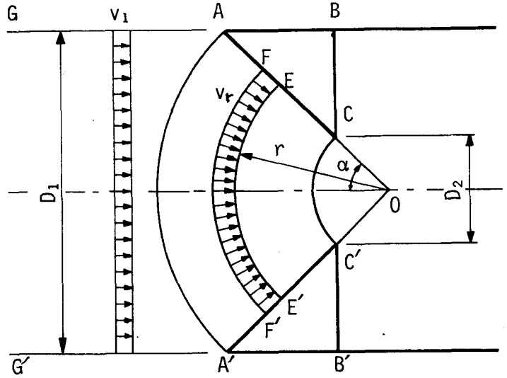
図-2.3.4 ブラインドシールド先端部の粘土の塑性流動速度
