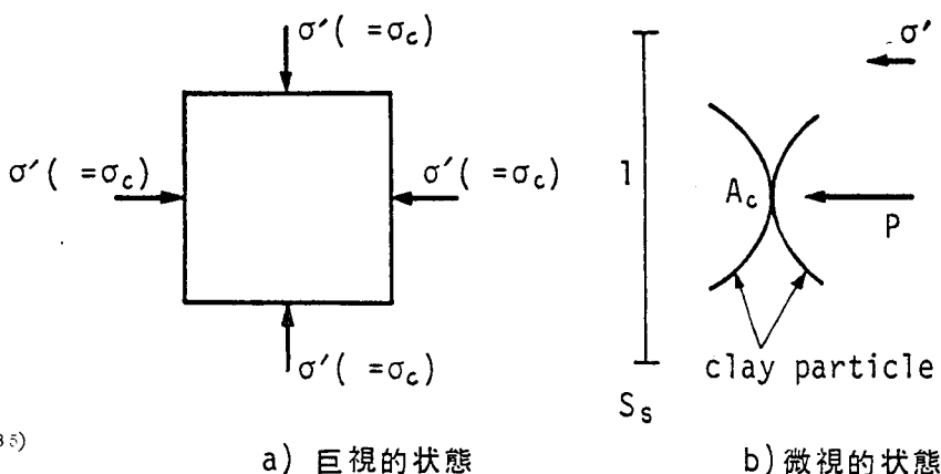
図一 1.6.6 粘土要素
