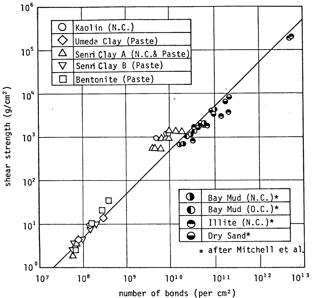
図－ 1. 2. 29 種々の土のせん断強さと結合数の関係
