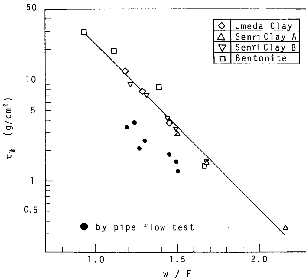
図 - 2.1.11 a) \tau_y と w/F の関係
