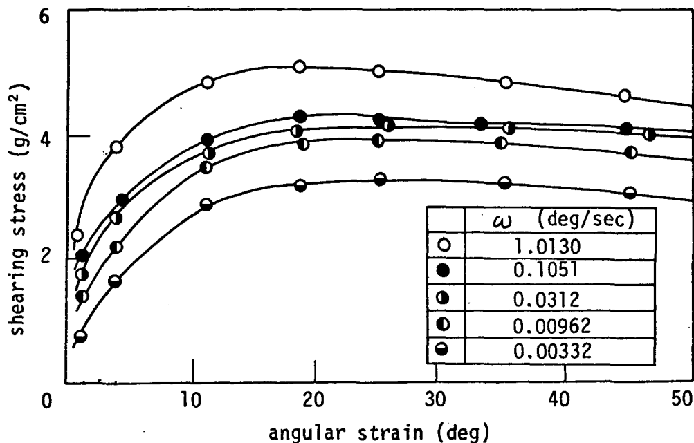
図- 1.2.10 ペーン回転角とせん断応力の関係
