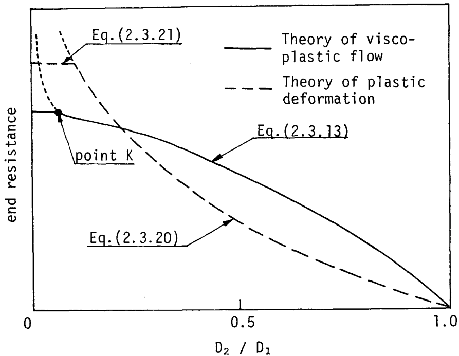
図－ 2.3.6 先端抵抗力の理論曲線
