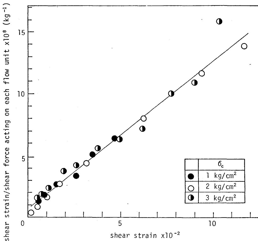
図-1.6.4 \gamma/f と \gamma の関係
