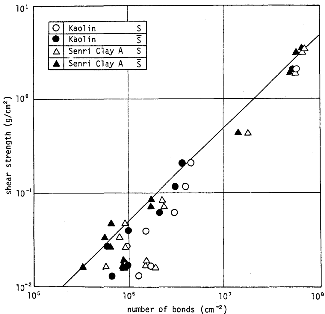
図－ 1. 5. 4 高含水比粘土ペーストのせん断強さと換算結合数の関係
