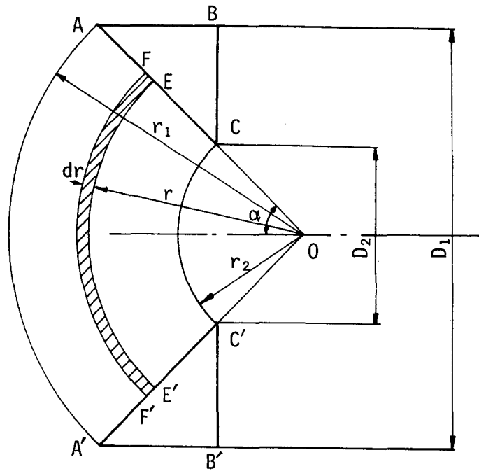
図- 2.3.3 ブラインドシールド先端部の粘土の塑性流動状態
