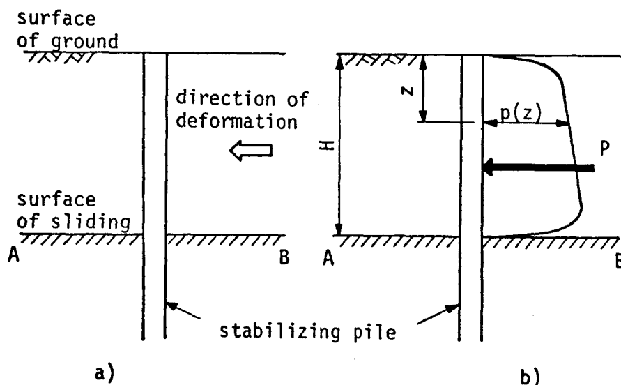
図－ 2.4.1 塑性変形地盤中の杭に作用する外力
