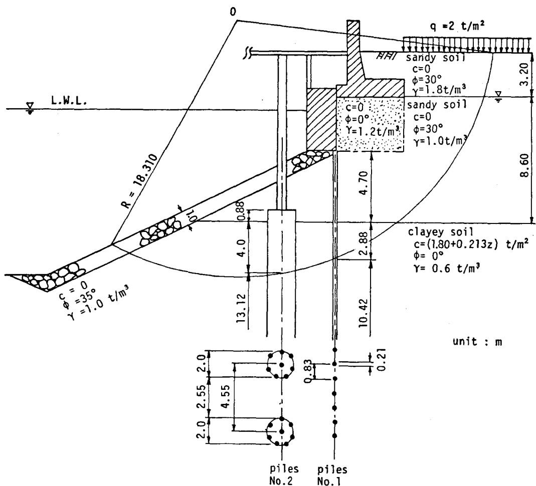
図－2.4.19 大阪港第1号岸壁横棧橋および地盤の断面図
