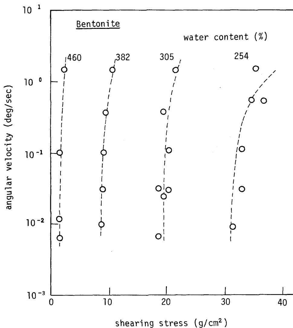
図 - 2.1.10 d) ベントナイト
