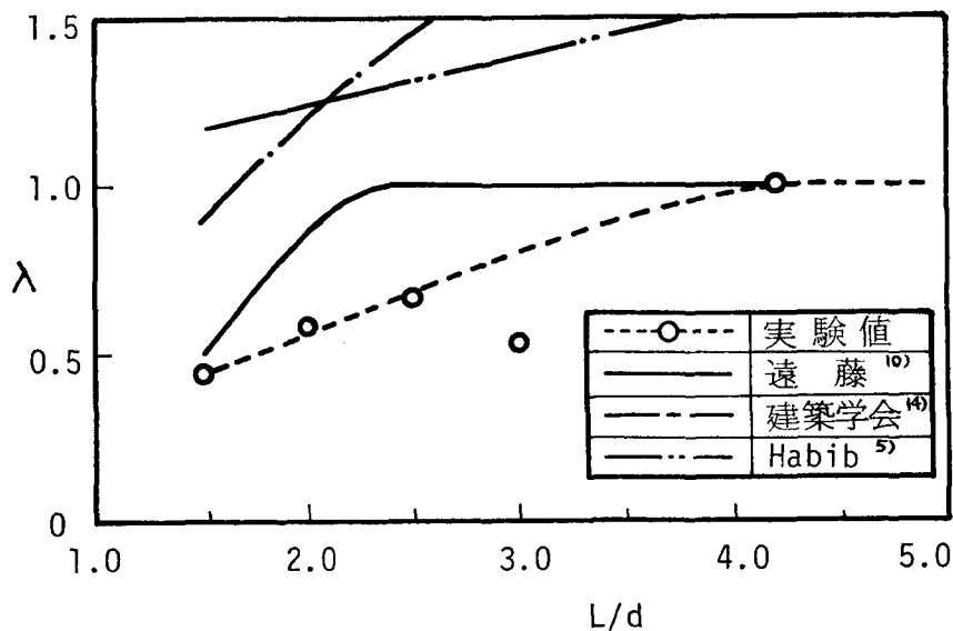
図一 2.5.17 \lambda と L/d の関係
