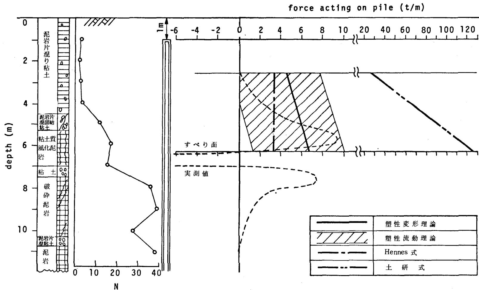
e) 東戸野地すべり地No. 3 杭
