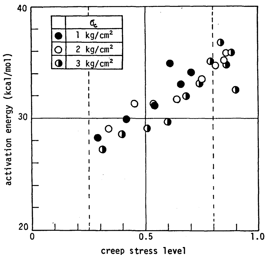
図－ 1.2.24 正規圧密粘土の活性化エネルギーと応力レベルの関係
