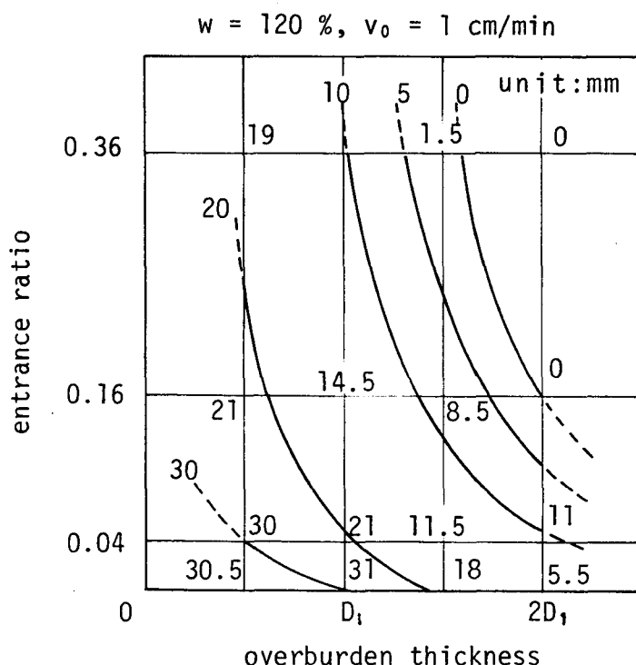
図— 2.3.8 地表面の最大盛り高 ( w=120\% )
