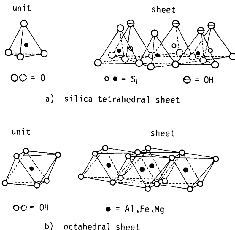
図-1.2.30 粘土鉱物の構造
