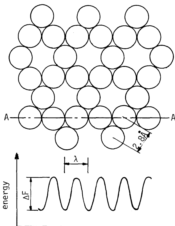
図－ 1. 2. 31 シリカ鉱物表面の酸素原子の分布
