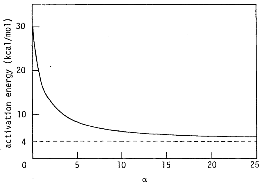
図- 1.3.1 heterogeneous process の活性化エネルギーと \alpha の関係
