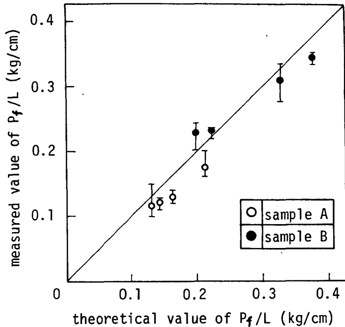
図一 2.3.11 P_f/L の理論値と実験値の比較 (塑性流動理論)
