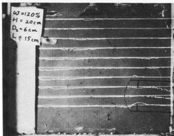
写真 2.3.7 周辺地盤の鉛直 変位の挙動 ( H = 20 \text{ cm} )
