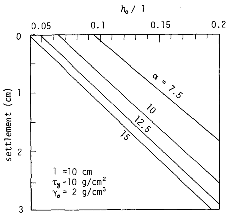
a) 沈下量と h_0/l の関係
