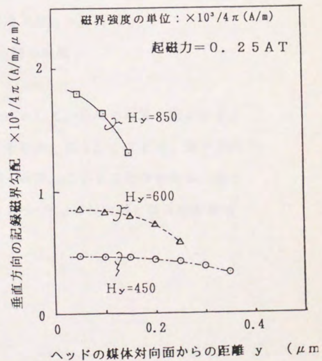
(b) 垂直成分
