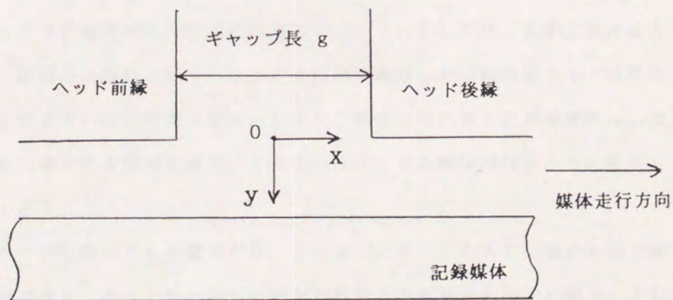
図2. 9 記録磁界解析における座標系
