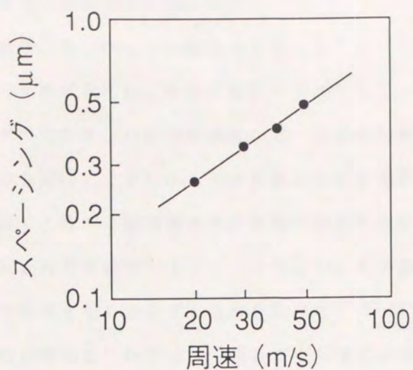
図4. 18 スレーシングの周速依存性
