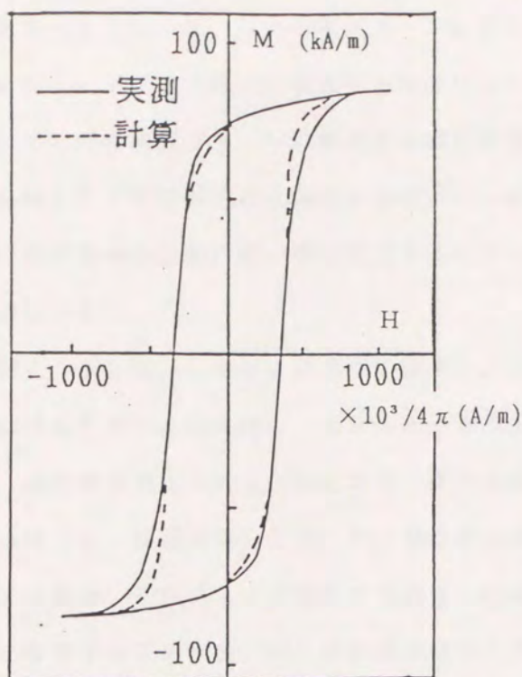
(a) 円周方向
