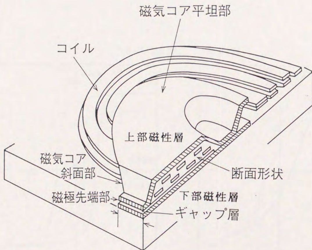
図 4. 21 薄膜磁気ヘッドの外観
