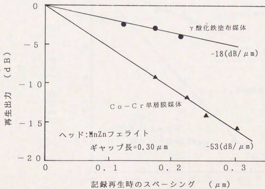
(b) 記録再生スペーシング損失
