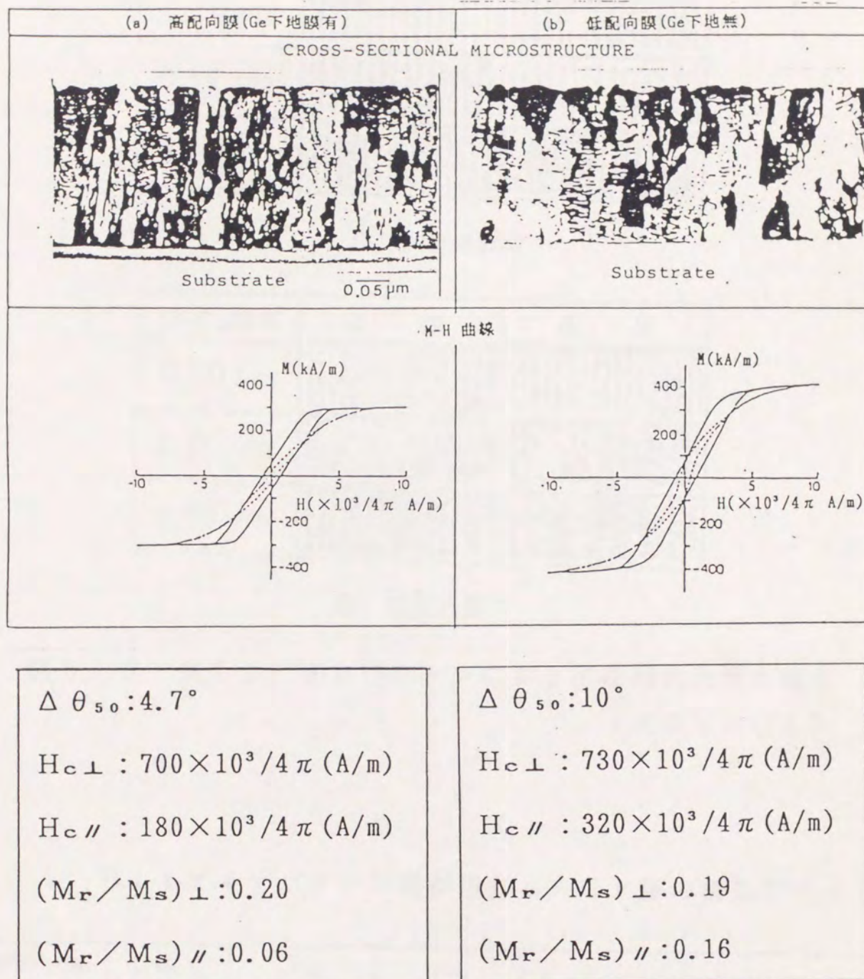
図 5. 2 Co-Cr 膜の断面組織と磁化曲線
