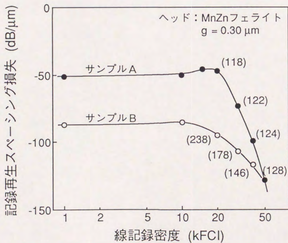
図 3. 6 記録再生スペーシング損失の線記録密度依存性 (1)
