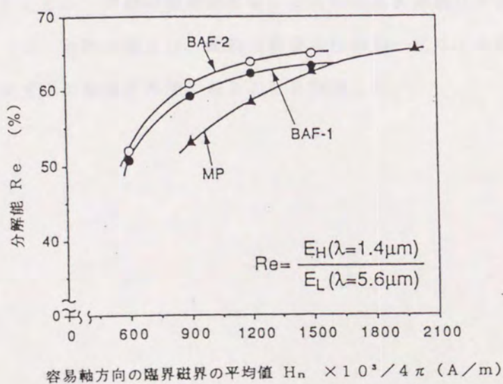
図4. 41 分解能と容易軸方向の臨界磁界との関係
