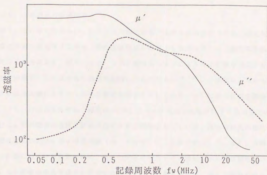
図2. 4 MnZnフェライトの複素透磁率の周波数依存性
