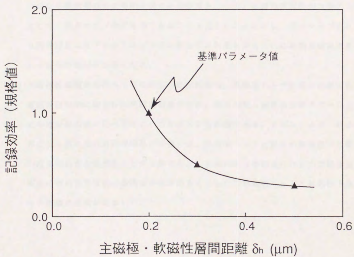
図 2. 3 5 記録効率およびすそ広がり率と 主磁極・下層膜間の距離との関係
