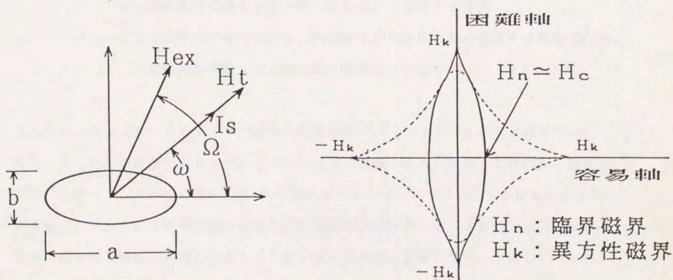
(a) 針状粒子の近似形状 (b) 針状粒子の臨界磁界
