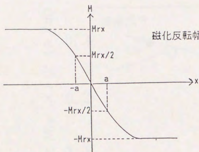
(a) 長手成分
