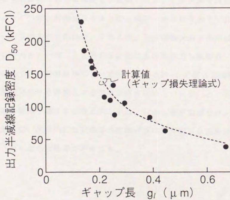
図 5. 18 D_{50} のギャップ長依存性
