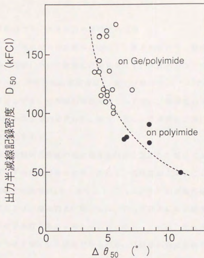
図 5. 17 Co-Cr 垂直配向度向上の効果
