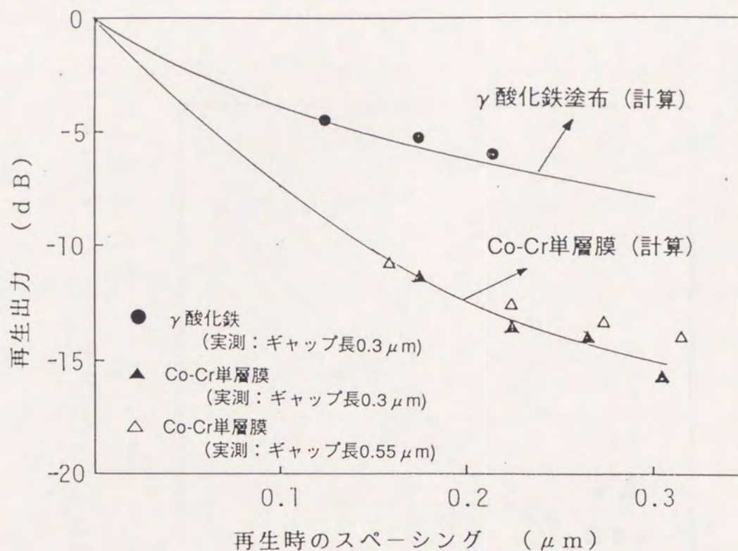
図3. 16 16 kHzにおける再生スペーシング損失の実測と計算の比較
