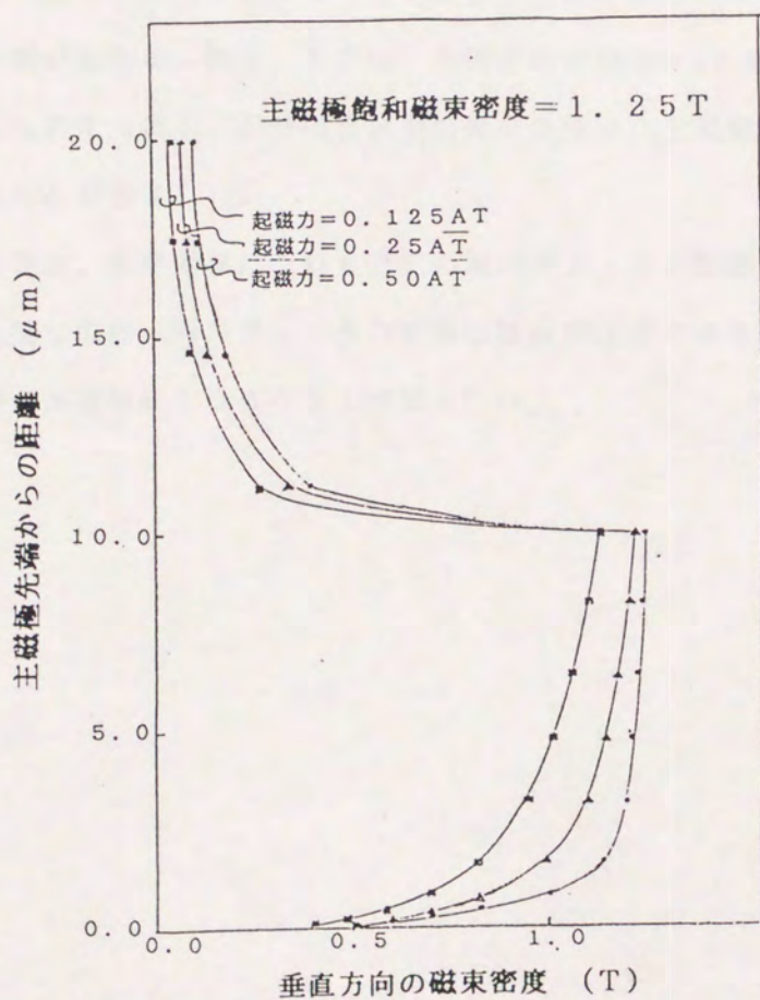
図 2. 29 主磁極内部における垂直方向磁束密度分布
