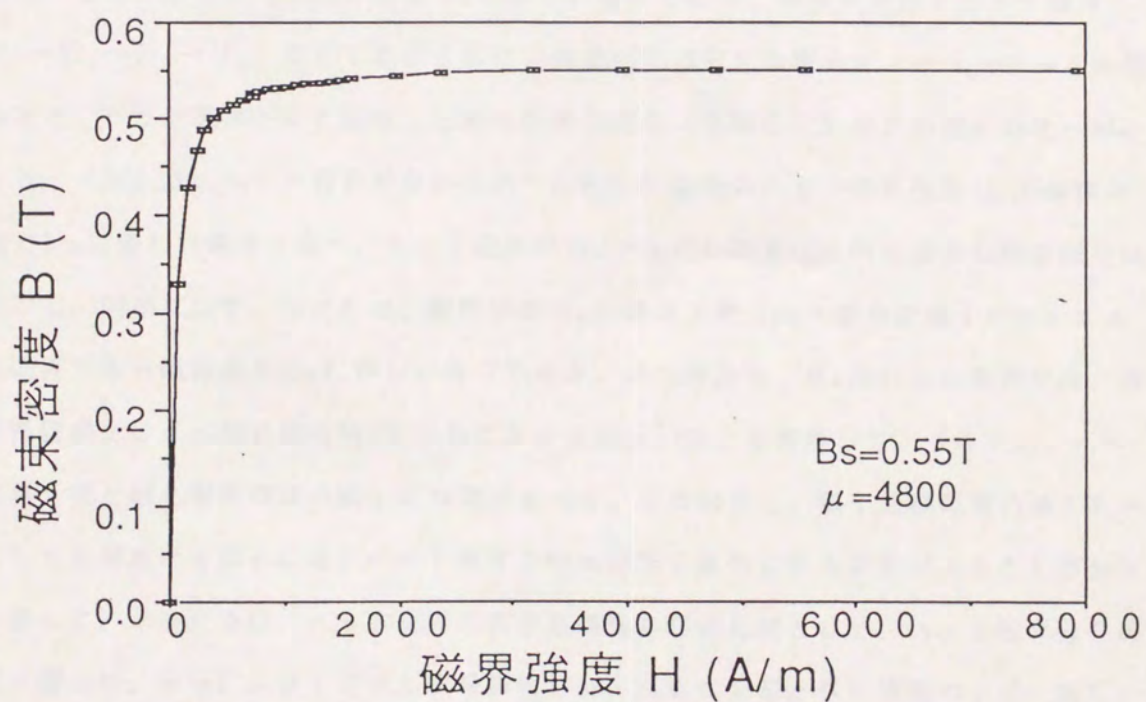
図2. 5 磁気ヘッド材料のB-H特性の計算例 (MnZnフェライト)
