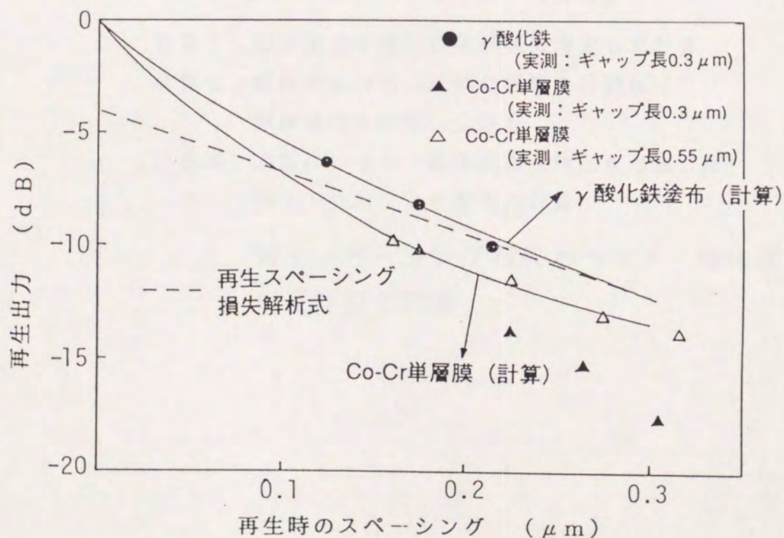
図3. 17 25 kHzにおける再生スペーシング損失の実測と計算の比較
