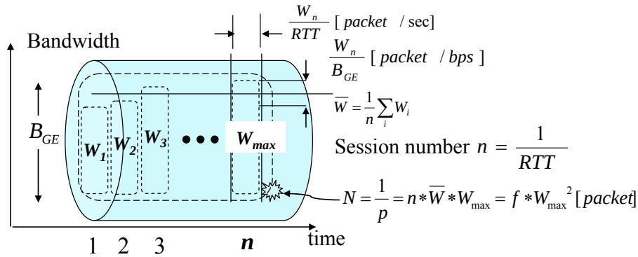
図 3.1 パケットロス率 p とウィンドウサイズの関係
