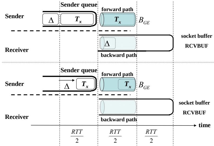
図 2.5 IP 層最適バッファサイズ
