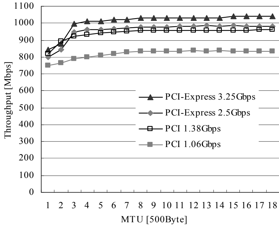
図 3.17 スループット上限値の PCI 帯域依存性
