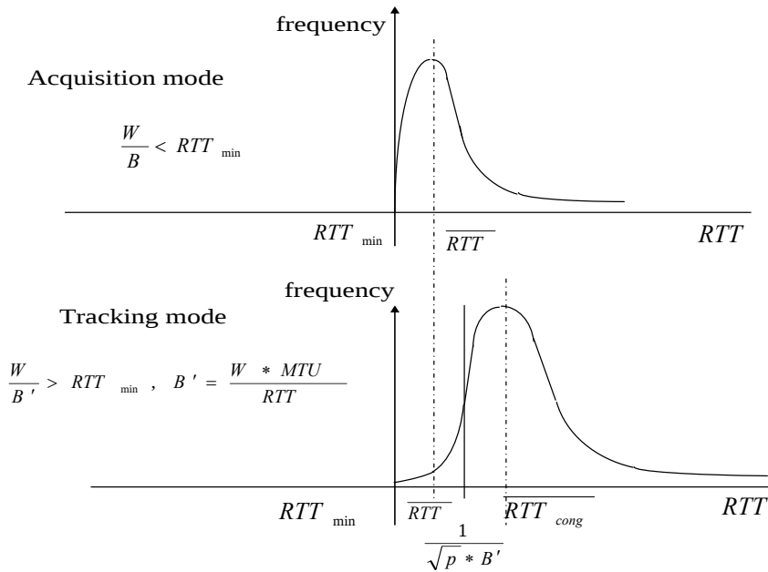
図 4.16 RTT 諸量の関係
