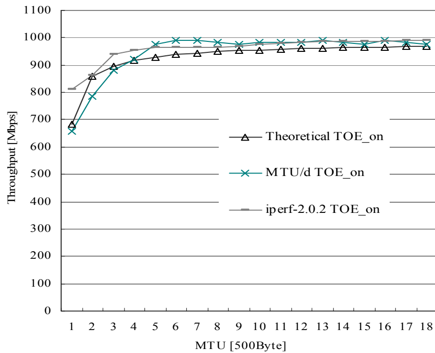
図 3.15 TOE-TCP スループット上限値
