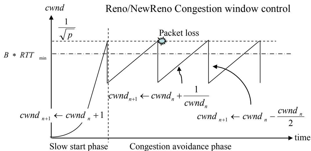
図 2.8 TCP . 輻輳制御ウィンドウ( cwnd )の動き
