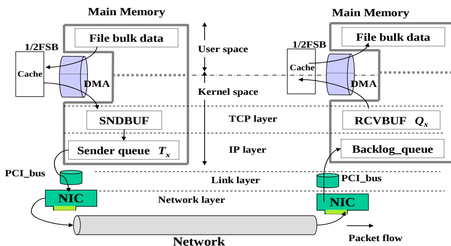
図 2.2 端末内部バッファ構成
