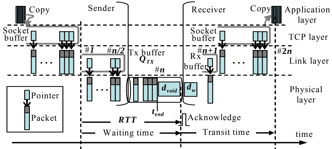
図 3.8 E2E システム内パケット数
