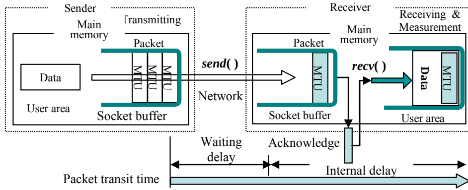
図 3.11 受信端末遅延 d
