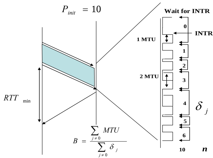
図 4.9 受信端末による帯域測定
