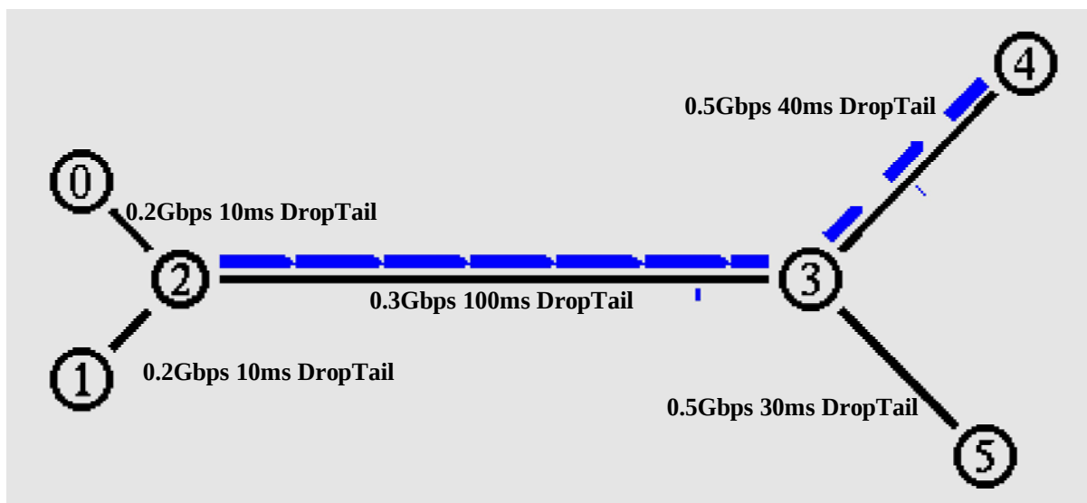
図 4.22 シミュレーションモデル
