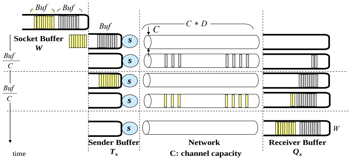
図 4.2 端末各層内バッファとパケットタイミング
