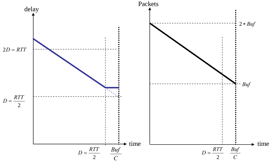
図 4.6 オーババッファのパケット遅延とパケット数
