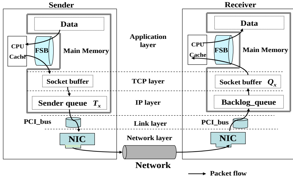
図 4.1 端末バッファ構成
