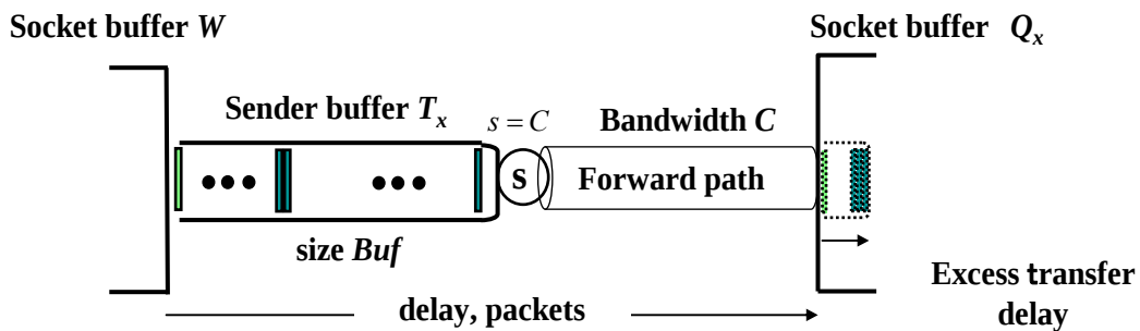
図 4.5 送出バッファサイズがネットワーク帯域遅延積より大きい場合
