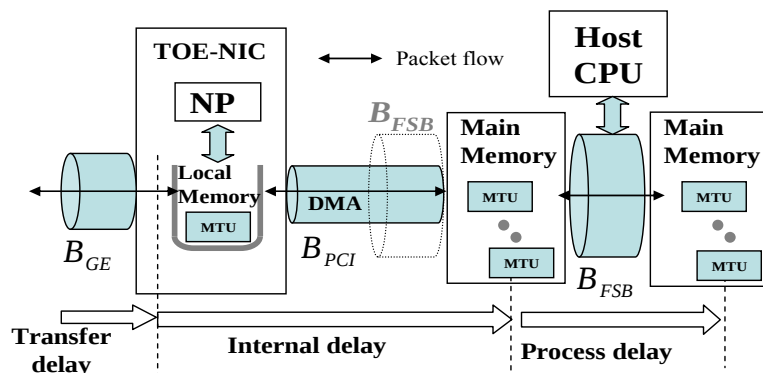
図 3.4 パケットフロー
