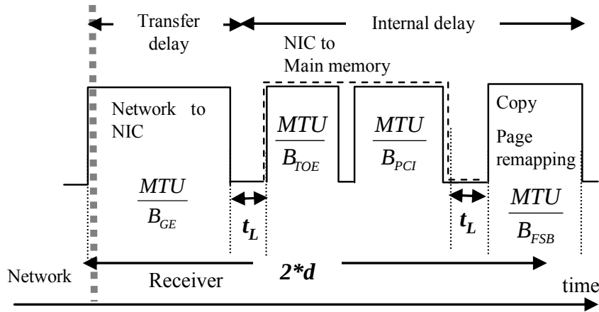
図 3.6 1 パケット通過遅延時間
