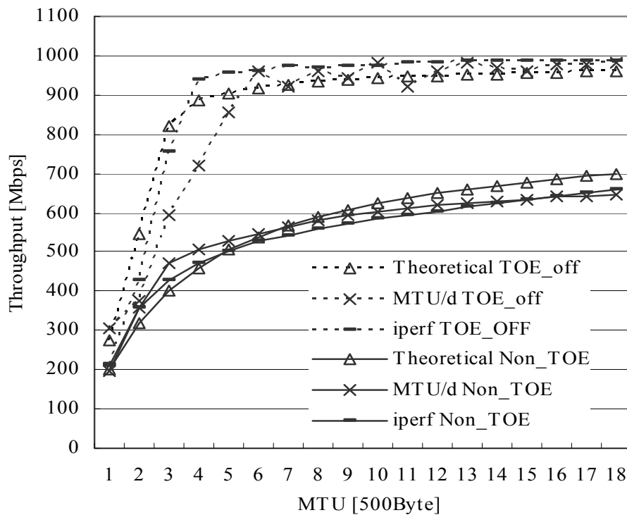
図 3.16 TOE オフ対 Non_TOE スループット上限値
