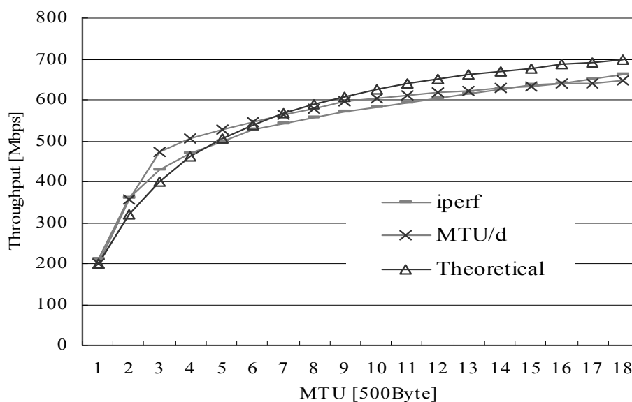
図 3.14 Non_TOE-TCP スループット上限値
