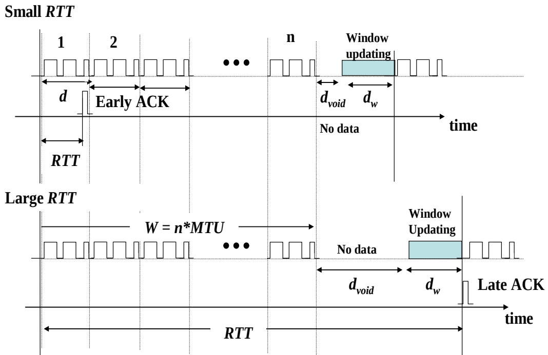
図 3.7 d_{void} , d_w , d_{ntwk} タイミング関係
