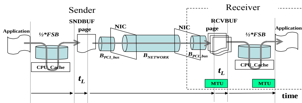
図 3.5 端末バッファとネットワークと端末内部バスの構成
