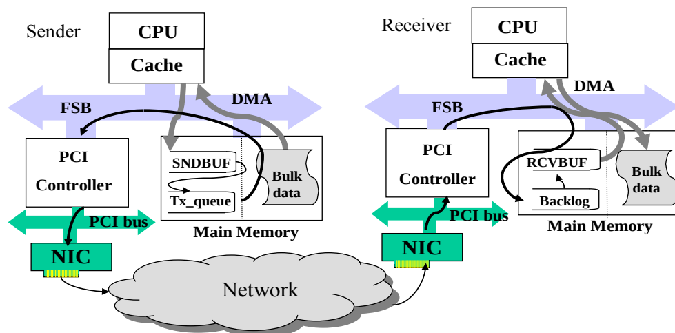
図 2.1 端末内部バッファとパケットフロー
