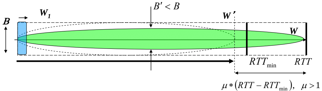
図 4.15 輻輳時ウィンドウ更新
