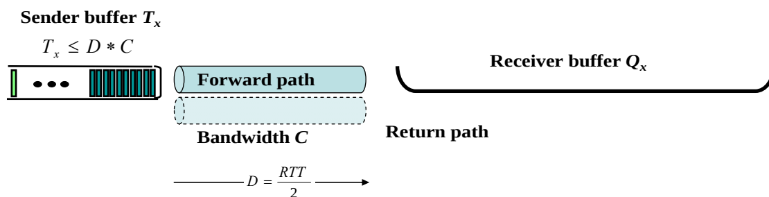
図 4.7 受信バッファサイズとパケット数
