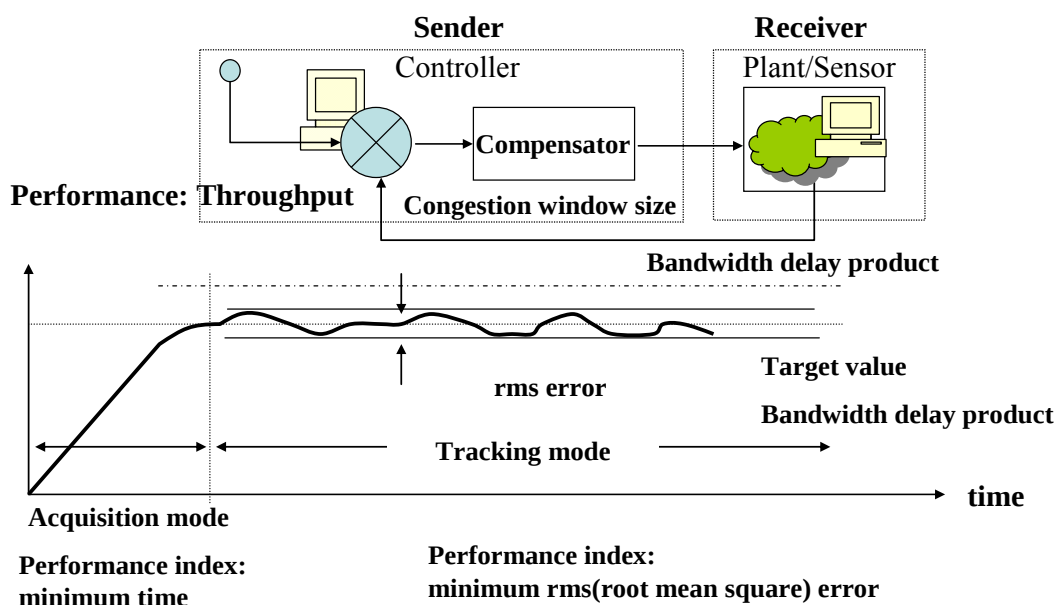
図 2.6 送受信端末ネットワーク総合系とフィードバック制御系との対応
