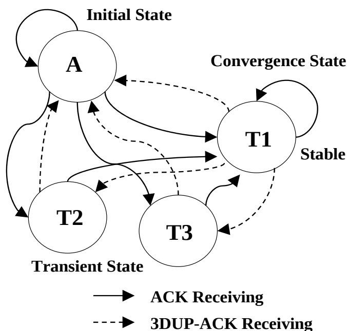
図 4.19 輻輳ウィンドウ状態遷移
