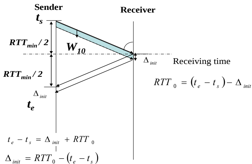
図 4.10 初期セッションのタイミングチャート
