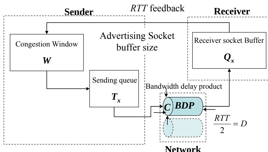
図 2.7 フィードバック制御系におけるバッファと制御の流れ
