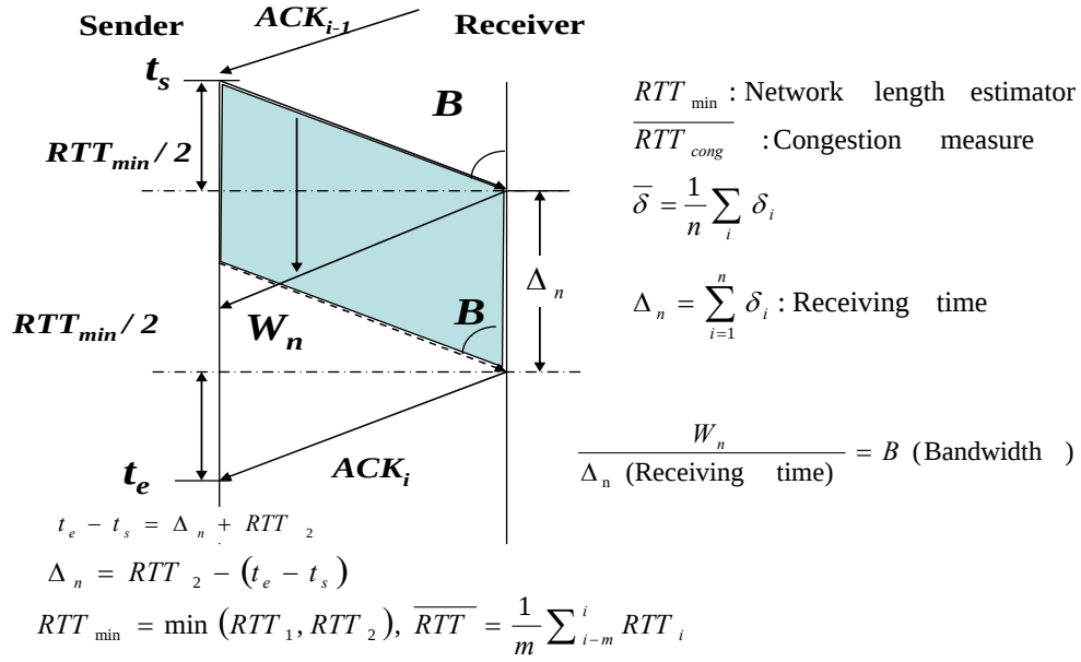
図 4.12 一般的なアキュジション時の RTT の計算
