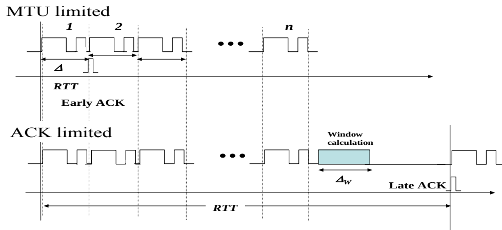
図 3.3 ACK と RTT のタイミング関係
