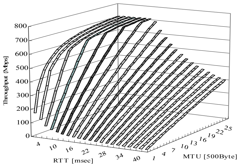
図 3.9 Non_TOE-TCP スループット上限値
