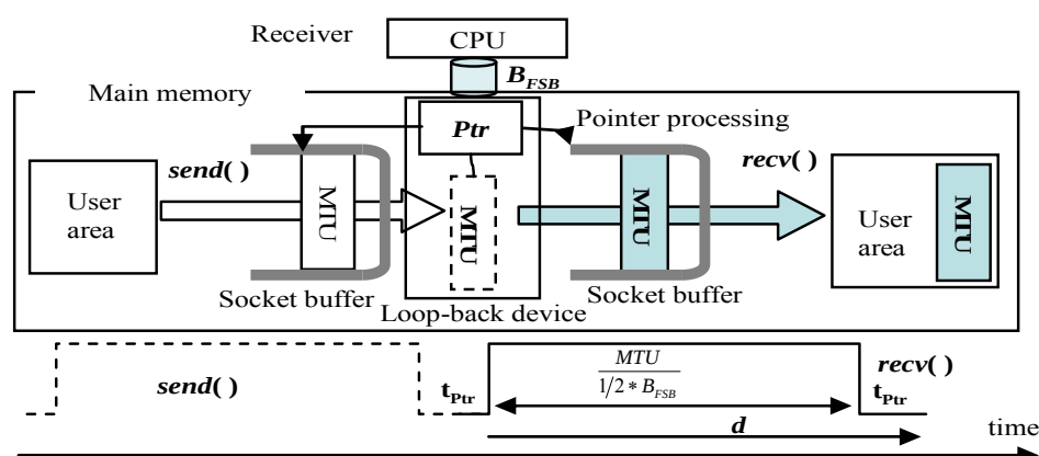
図 3.13 ループバック測定
