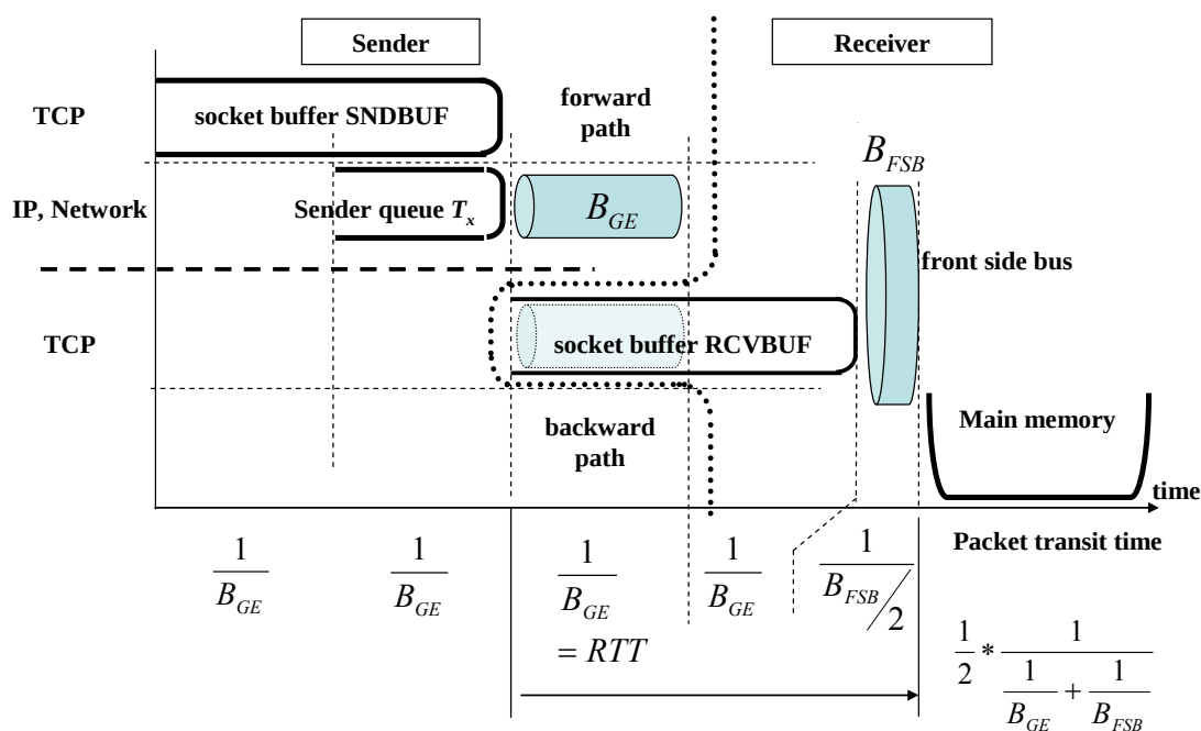
図 2.4 TCP/IP 層バッファ構成
