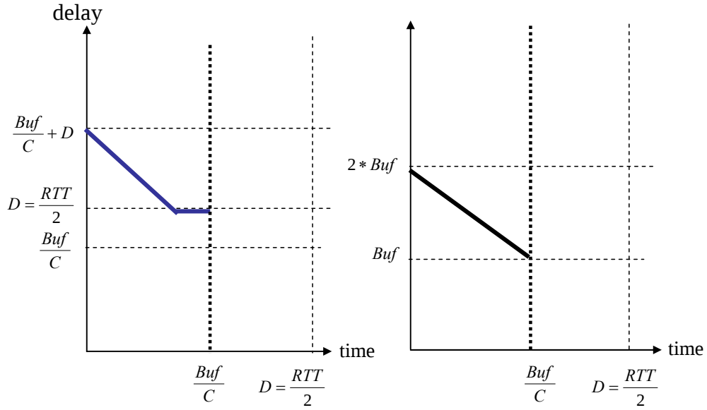
図 4.4 アンダーバッファの packets 遅延と packets 数
