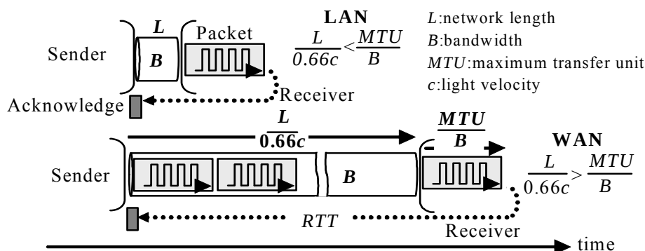
図 3.2 ネットワーク距離対 RTT
