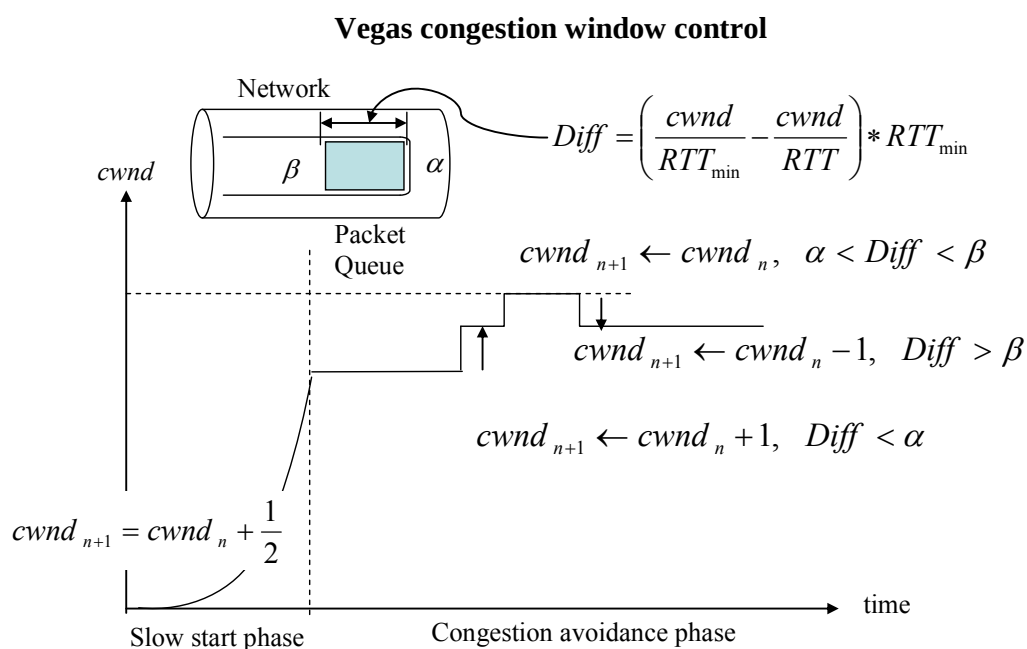
図 2.9 TCPVegas 輻輳制御ウィンドウ( cwnd )の動き
