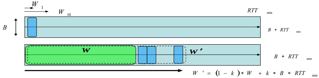
図 4.14 非輻輳時ウィンドウ更新
