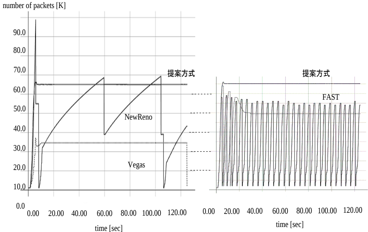
図 4.23 NewReno, Vegas, FAST, 提案方式ウィンドウサイズ
