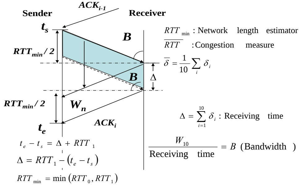
図 4.11 第2セッション以降のタイミングチャート
