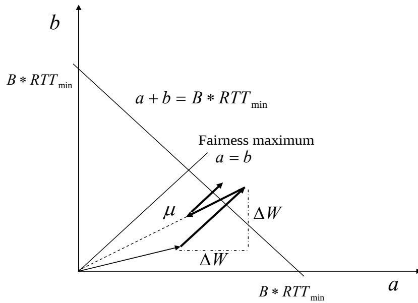
図 4.20 公平性（フェアネス）収束点
