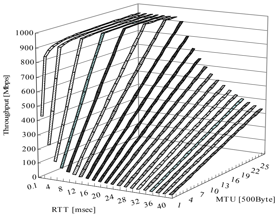
図 3.10 TOE-TCP スループット上限値
