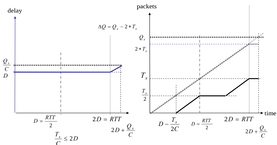
図 4.8 受信バッファ遅延とパケット数の関係
