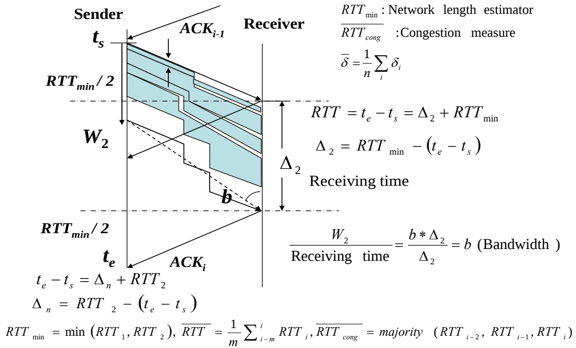
図 4.13 輻輳時の RTT 計算
