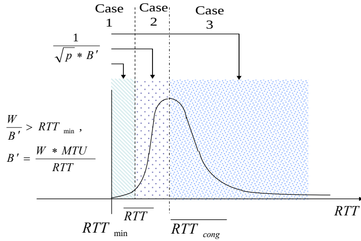
図 4.17 パケットロス率と RTT 量の関係
