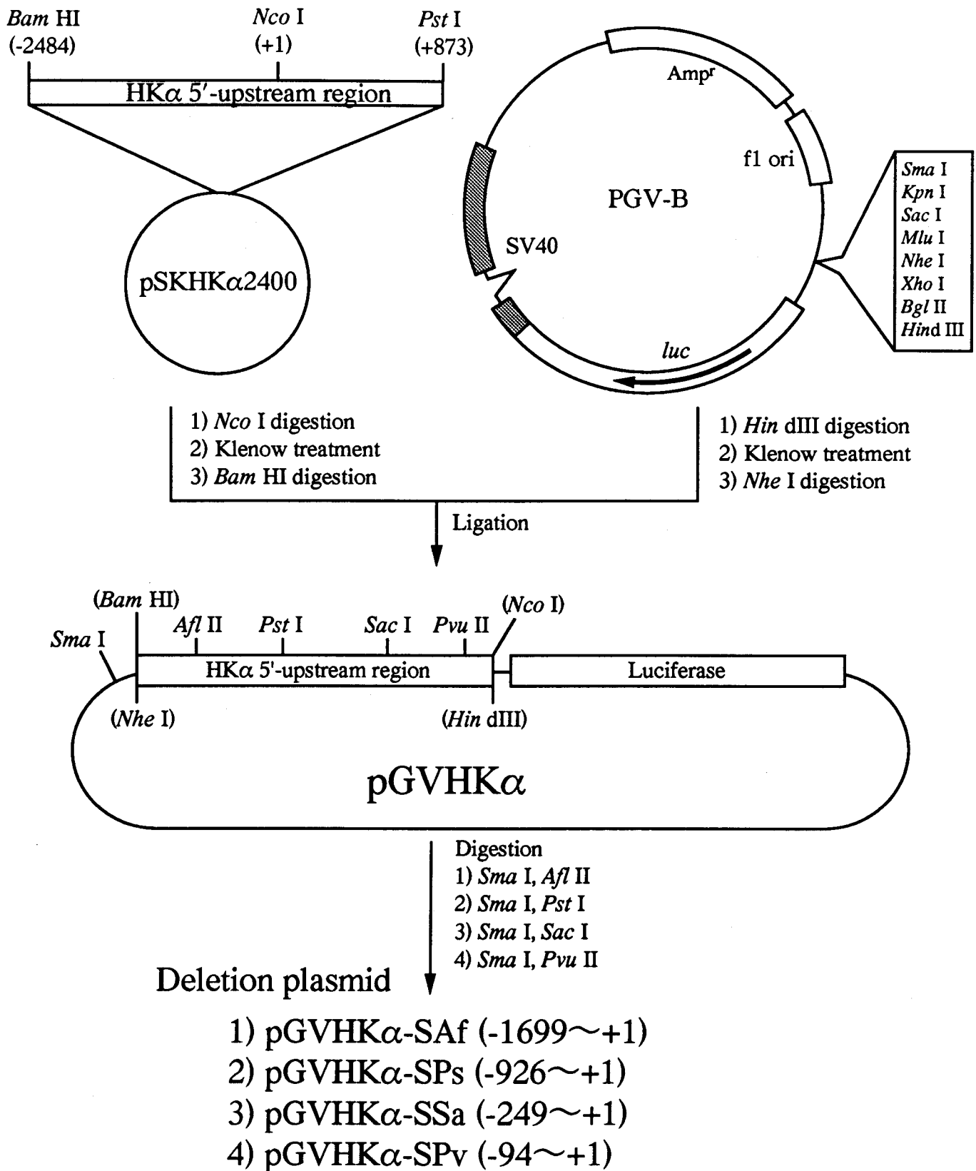
図3-3) ルシフェラーゼ遺伝子上流にラット H^+/K^+ -ATPase \alpha サブユニット遺伝子5'上流を結合させたレポーター遺伝子の構築
