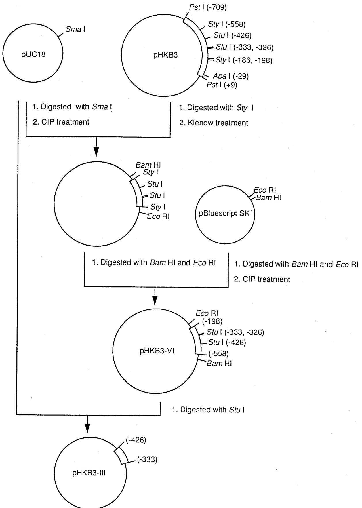
図2-3) プローブ調製用に用いたプラスミドの構造および作成方法。
