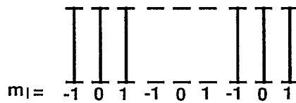
( b ) 核スピン I = 1 をもつが、 J と I がカップリングしていない場合
