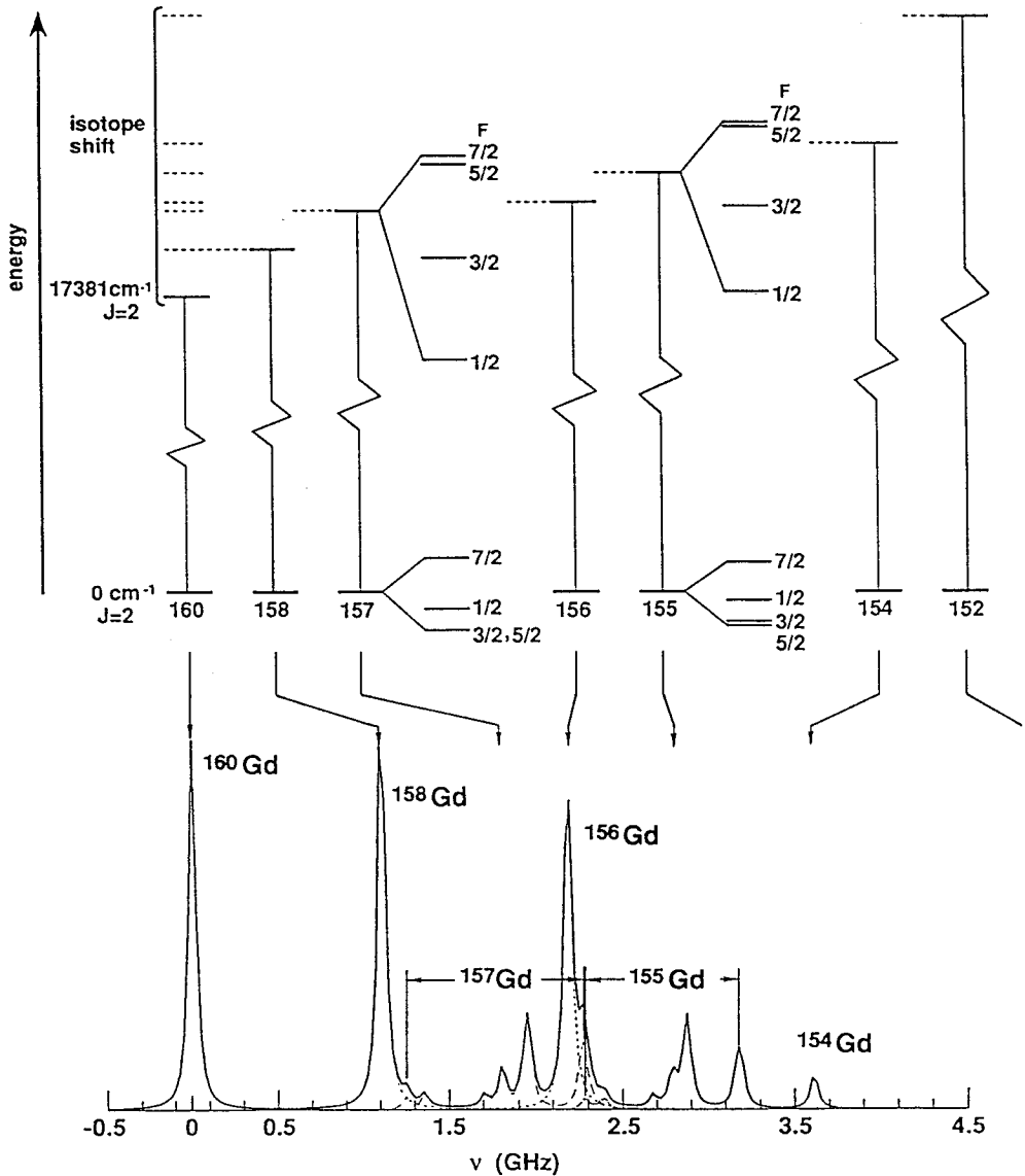
図 2-2 Gd のエネルギー準位の分裂と超微細構造 ( 0 \text{ cm}^{-1} - 17381 \text{ cm}^{-1} ) 核スピン I \neq 0 をもつ同位体では、電子軌道角運動量 J をもつ 1 つの準位が原子核のスピン I との相互作用により、 2J + 1 個 ( J < I の場合) または 2I + 1 個 ( J > I の場合) の準位に分 裂する。図では超微細構造分裂部分は 10 倍のエネルギースケール で描いている。
