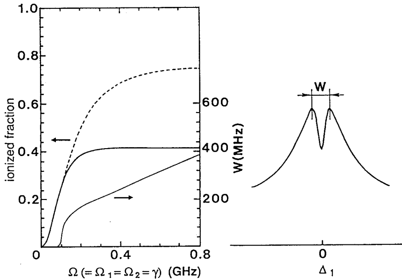
図4-7 最も効率のよい組合せ ( \Omega_1 = \Omega_2 = \gamma ) での トラップされる谷の深さと幅 W ( \Delta_2 = 0 GHz) の 点線：最大イオン量 実線： \Delta_1 = 0 (2光子共鳴条件) でのイオン量
