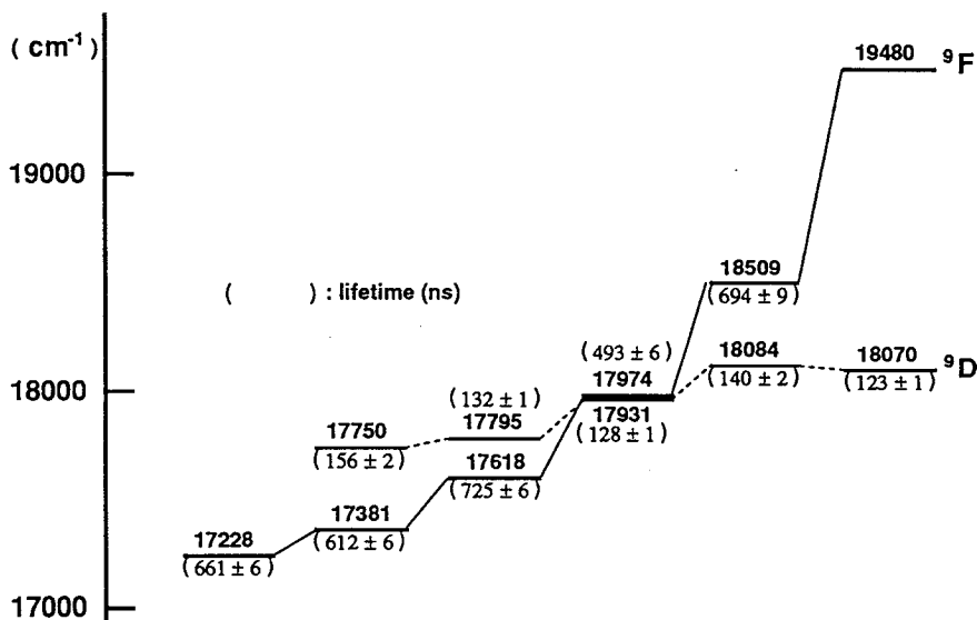
図 3-7 測定した励起準位とその寿命 ^9\text{F} 項の寿命はすべて数100 nsと非常に長い。
