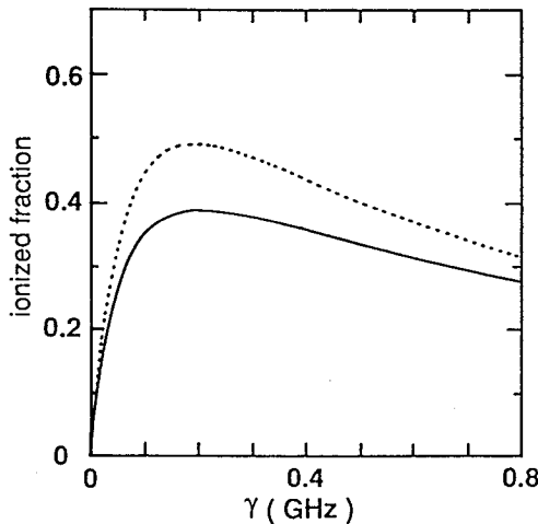
図 4-6 イオン化率 \gamma 依存性 \Omega_1 = \Omega_2 = 0.2 \text{ GHz} \Delta_2 = 0 \text{ GHz} 実線: \Delta_1 = 0 (2光子共鳴条件) 点線: 最大イオン量
