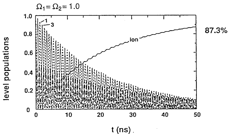
図 2-17 ドップラー広がりのない場合の各準位密度の時間発展
