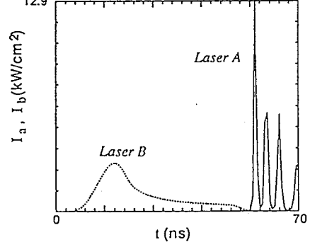
図5-12 イオン化のある3準位原子系における閉じた2準位系的 ふるまいに基づくパルス変形
