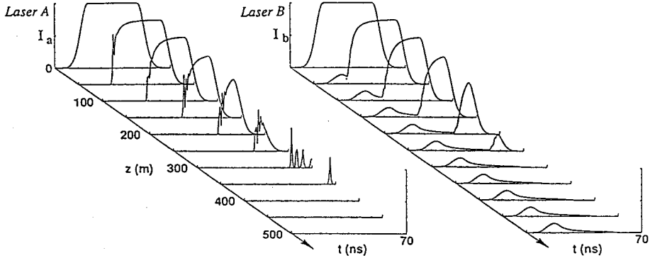
図5-11 共鳴同位体原子のみを考えた場合の伝播パルス波形変化 レーザーA, Bのパルスは計算された全伝播距離での最大強度 の値でそれぞれ規格化している。
