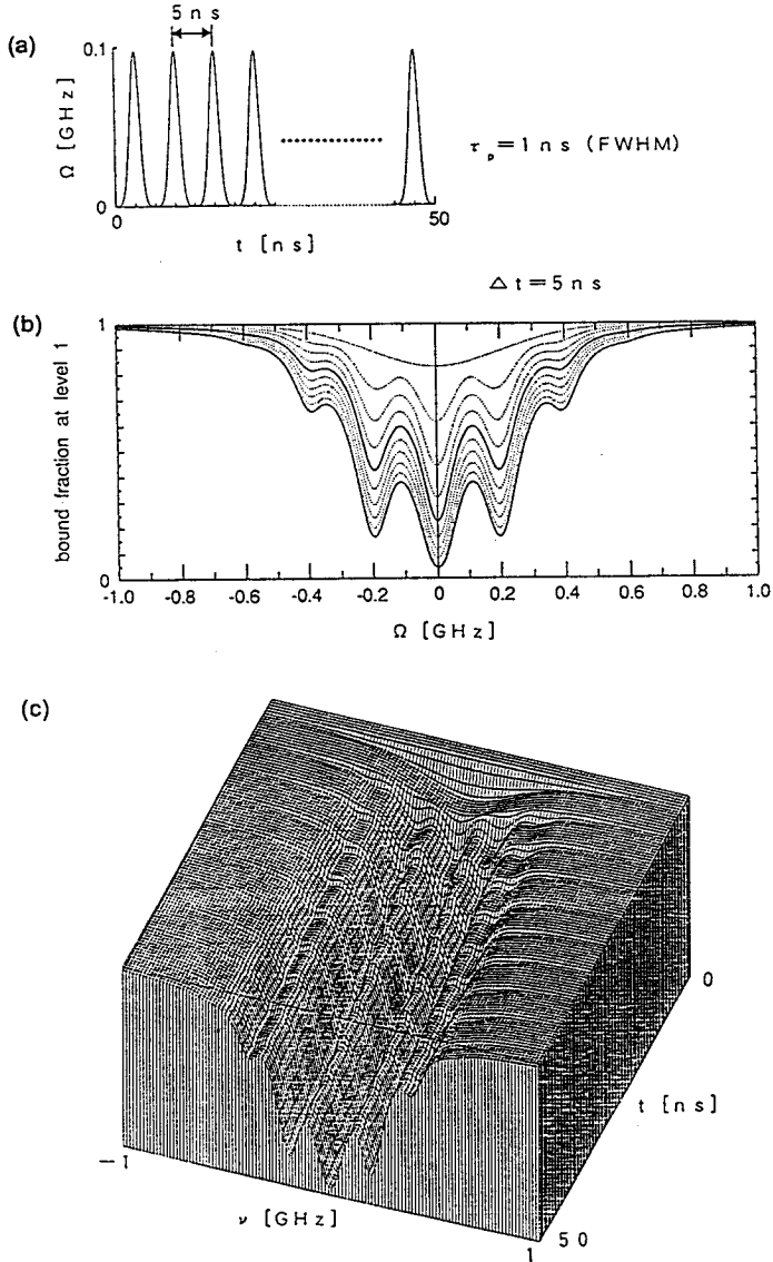
図 2 - 1 6 位相の合ったパルス列による励起 (a)モードロックレーザーのパルス列
