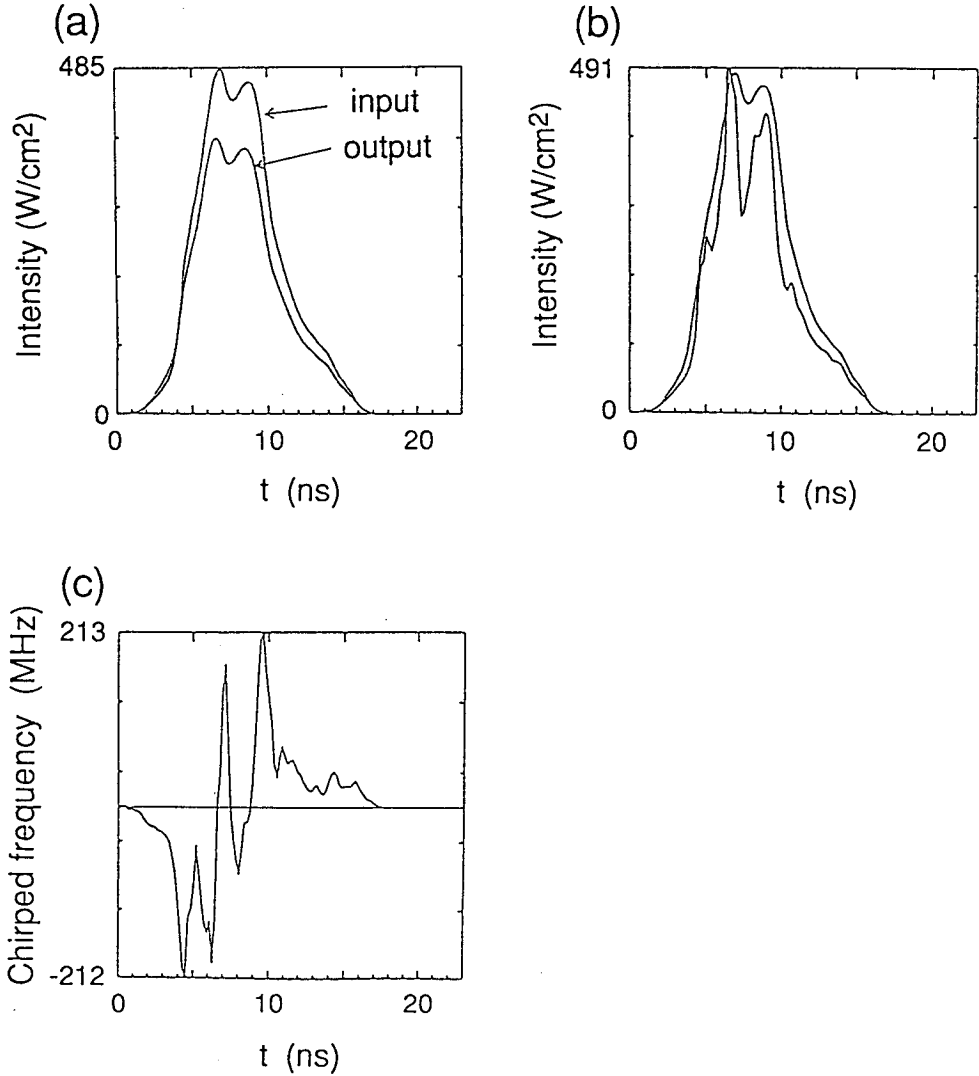
図5-6 図5-4 (b)の実験結果に対する断熱追従モデルによる計算結果 (a) 強度に依存するパルス伝播速度のみを考慮した場合 (b) 自己位相変調効果も考慮した場合 (c) 出射パルス内の周波数変調
