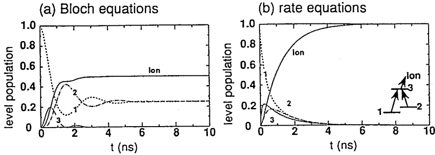
図2-5 コヒーレント励起とインコヒーレント励起の比較(3準位λ型) (a)では1/2の原子しかイオンにできない現象が、2光子共鳴条件で起こる。(b)ではいかなるパラメーター領域でもそのような現象は現われない。
