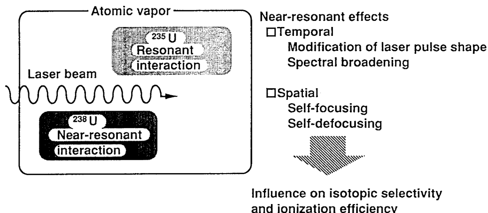
図5-1 レーザー同位体分離におけるレーザーパルス伝播 共鳴・近共鳴状態にある両方の同位体原子からレーザー パルスは時間的・空間的な変化を受ける。
