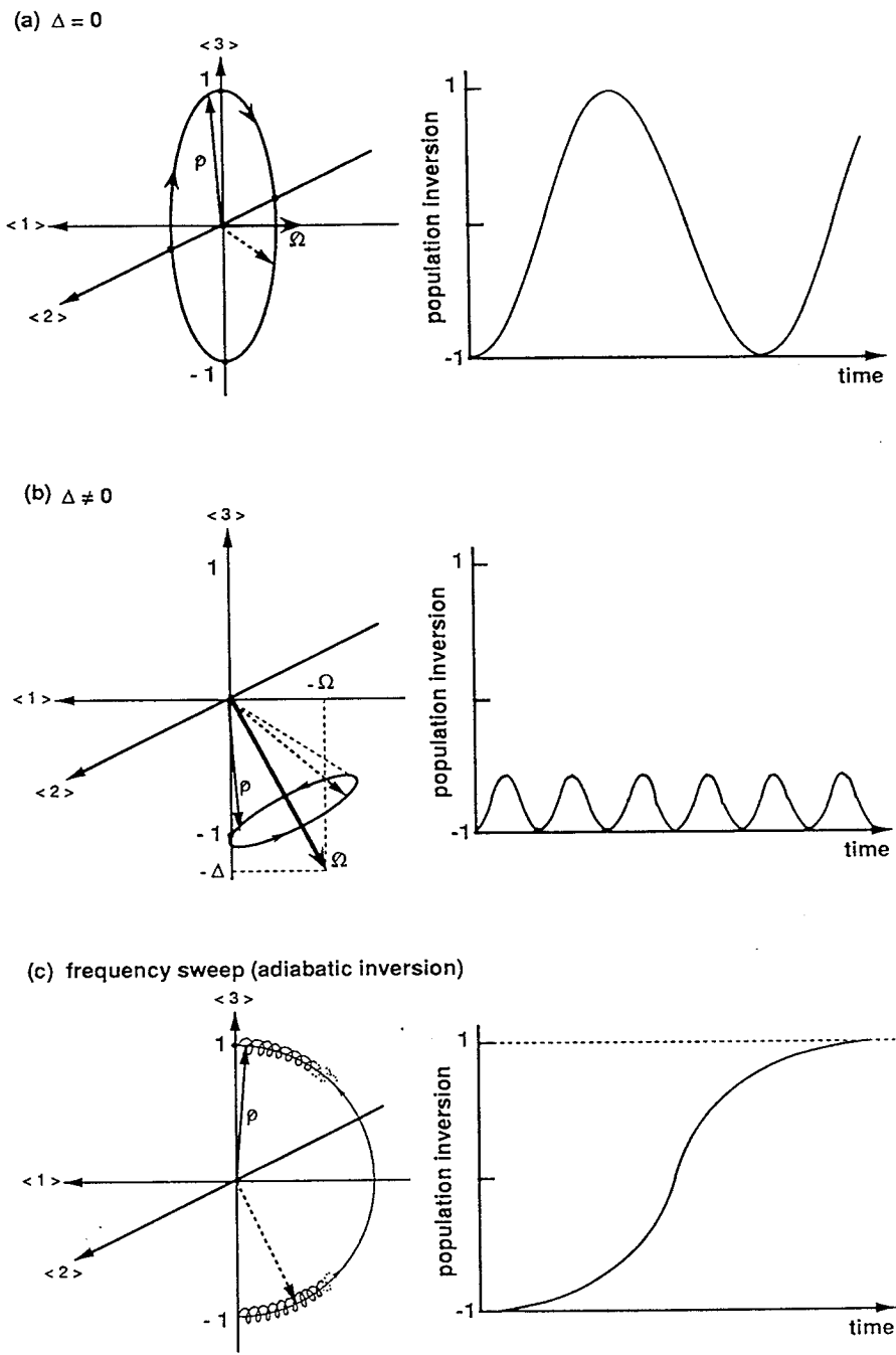
図 4-9 detuningの違いによるブロッホベクトル \rho の挙動 遷移の共鳴周波数とレーザーの周波数との差 \Delta が、(a) \Delta = 0 の場合、(b) \Delta \neq 0 の場合、(c) \Delta = 0 を通るよう に周波数を適当な速度で掃引した場合。左側はベクトルモデル、右側は反転分布の時間発展。ベクトルモデルの \langle 3 \rangle 軸 が反転分布に対応する。
