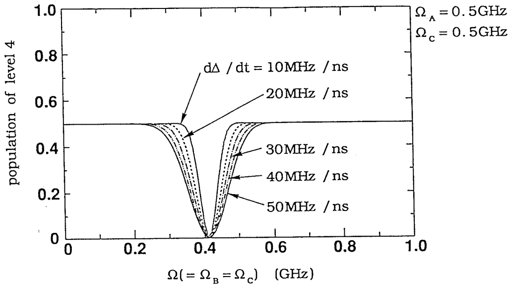
図4-19 準位4の分布数密度のRabi周波数依存性 \Omega_A = \Omega_C = 0.5 GHz
