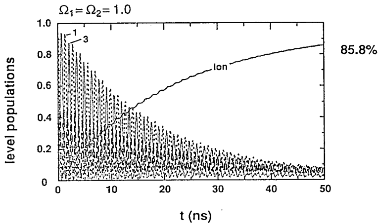
図 2 - 1 8 ドップラー広がりのある場合の各準位密度の時間発展
