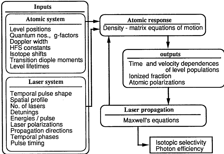
図 2 - 6 レーザー同位体分離の光反応過程のモデリング
