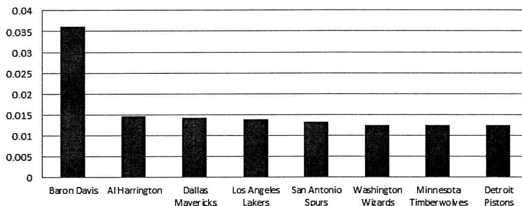
図 3.6: 入力テキスト「Microsoft denies Xbox Live security breach」に対して推測された関連語句とそれらの確率
