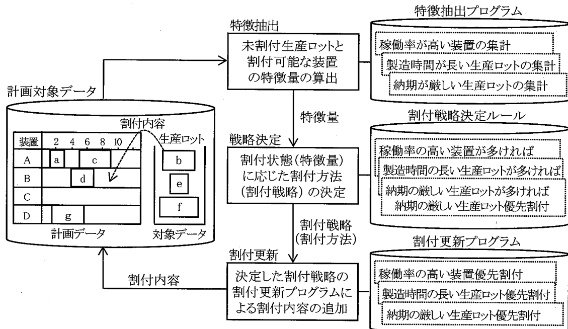
図 3.3 知識型スケジューリング方式
