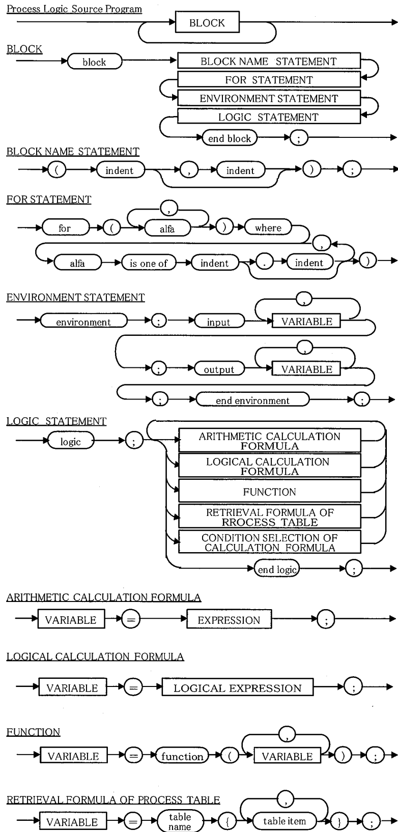
図 2.4 構文グラフ (その1)
