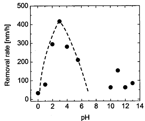
図 4.19 石英ガラス加工速度の pH 依存
