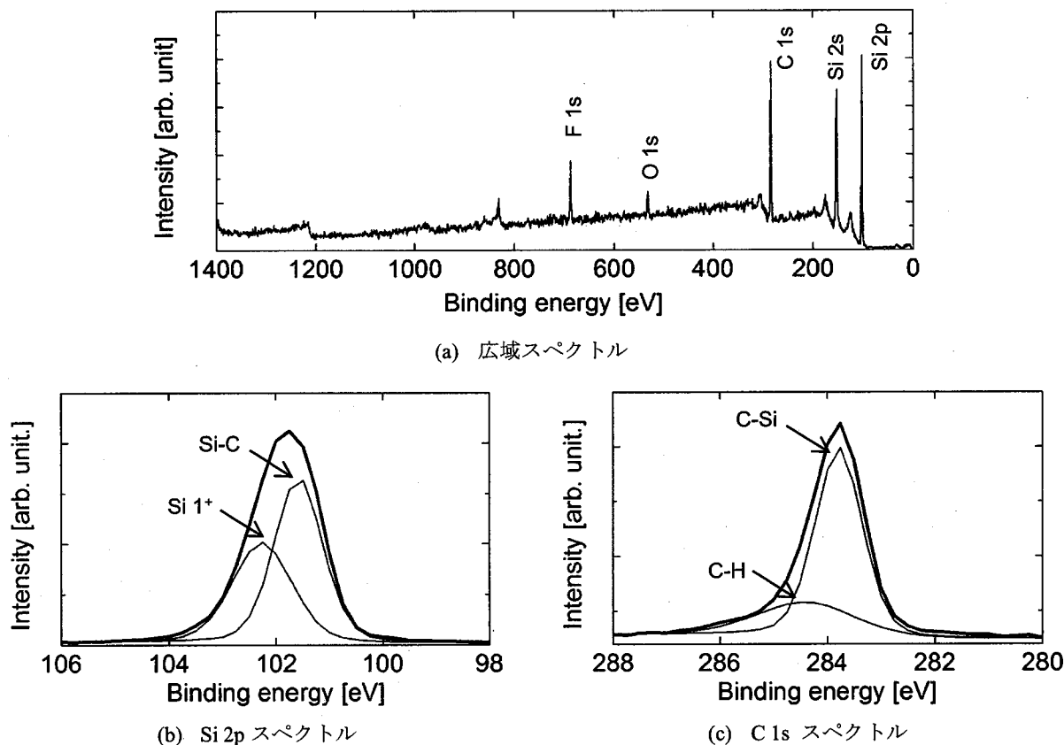
図 2.20 CARE 加工後 4H-SiC(0001) 4° off-axis 基板の XPS スペクトル
