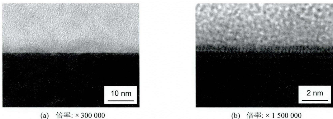
図 5.5 加工後 GaN(0001) 表面の断面 TEM 像. \langle 11\text{-}20 \rangle 方向に沿って観察.
