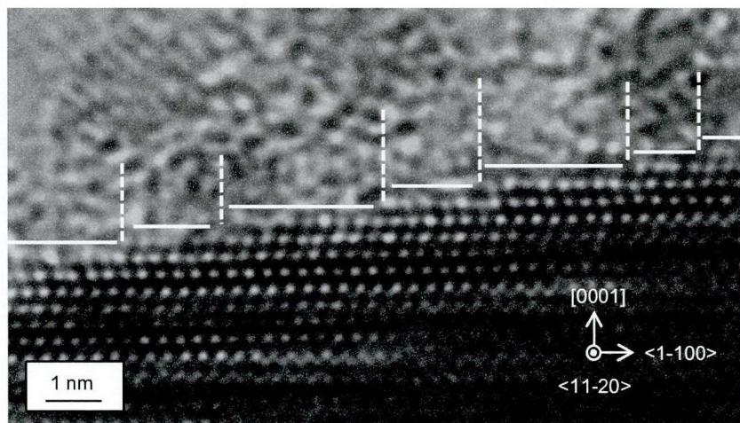
図 2.16 加工後の4H-SiC(0001) 8° off-axis 基板表面近傍の断面 TEM 構造像 (×1 000 000)
