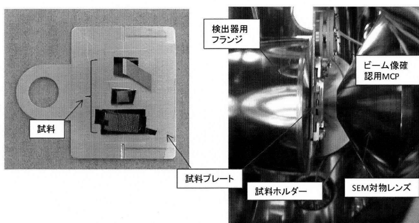
図 2.4-5 (左)試料プレートと(右)試料ホルダー近辺。
