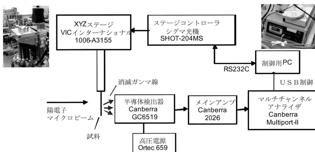
図 2.4-9 陽電子マイクロビーム二次元走査測定系のブロックダイアグラム。
