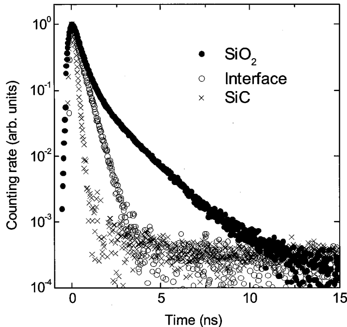
図 3.1-5 SiC 層、SiO 2 層及び界面層における陽電子消滅寿命測定の結果。
