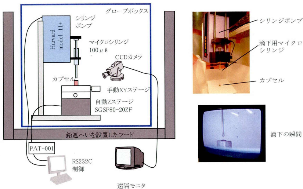
図 2.4-13 ^{22}\text{NaCl} 水溶液自動滴下装置と、滴下の様子。
