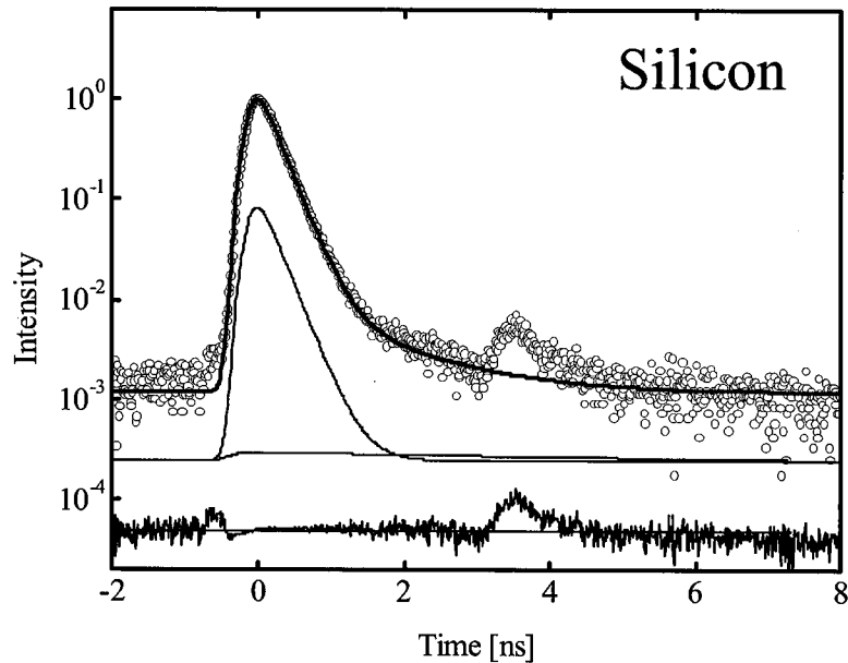
図 2.3-13 測定された陽電子消滅寿命スペクトルの例(シリコン)。
