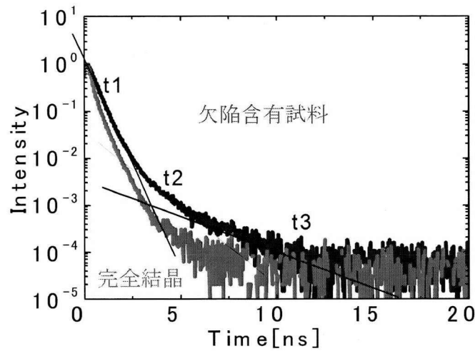
図 2.1-5 陽電子寿命曲線および成分分解の例
