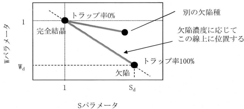
図 2.1-3 S-W プロットの概略。
