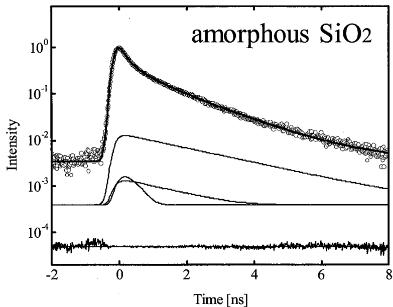
図 2.3-14 測定された陽電子消滅寿命スペクトルの例( \text{SiO}_2 )。
