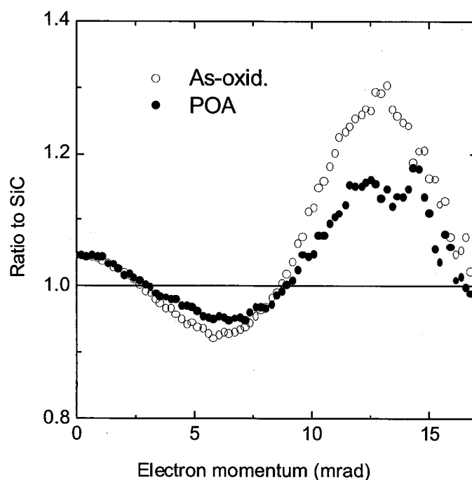
図 3.1-8 POA 処理前後での界面中間層における電子運動量分布の比率曲線の比較。
