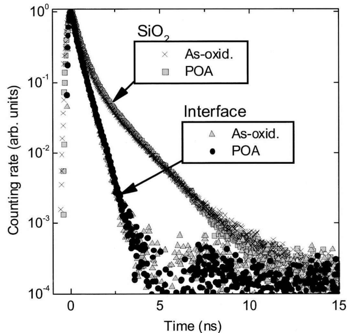
図 3.1-7 界面中間層及び \text{SiO}_2 層における POA 処理前後での陽電子寿命の比較。
