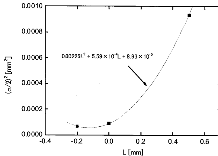
図 2.4-8 ビーム半径の 2 乗 \sigma^2 と像面位置 L の関係。曲線は 2 次関数によるフィッティング結果。実線は得られたパラメータを用いて描いた楕円関数 (粒子の中心軸からの距離 R と角度 \theta の関係、エミッタンス図)。
