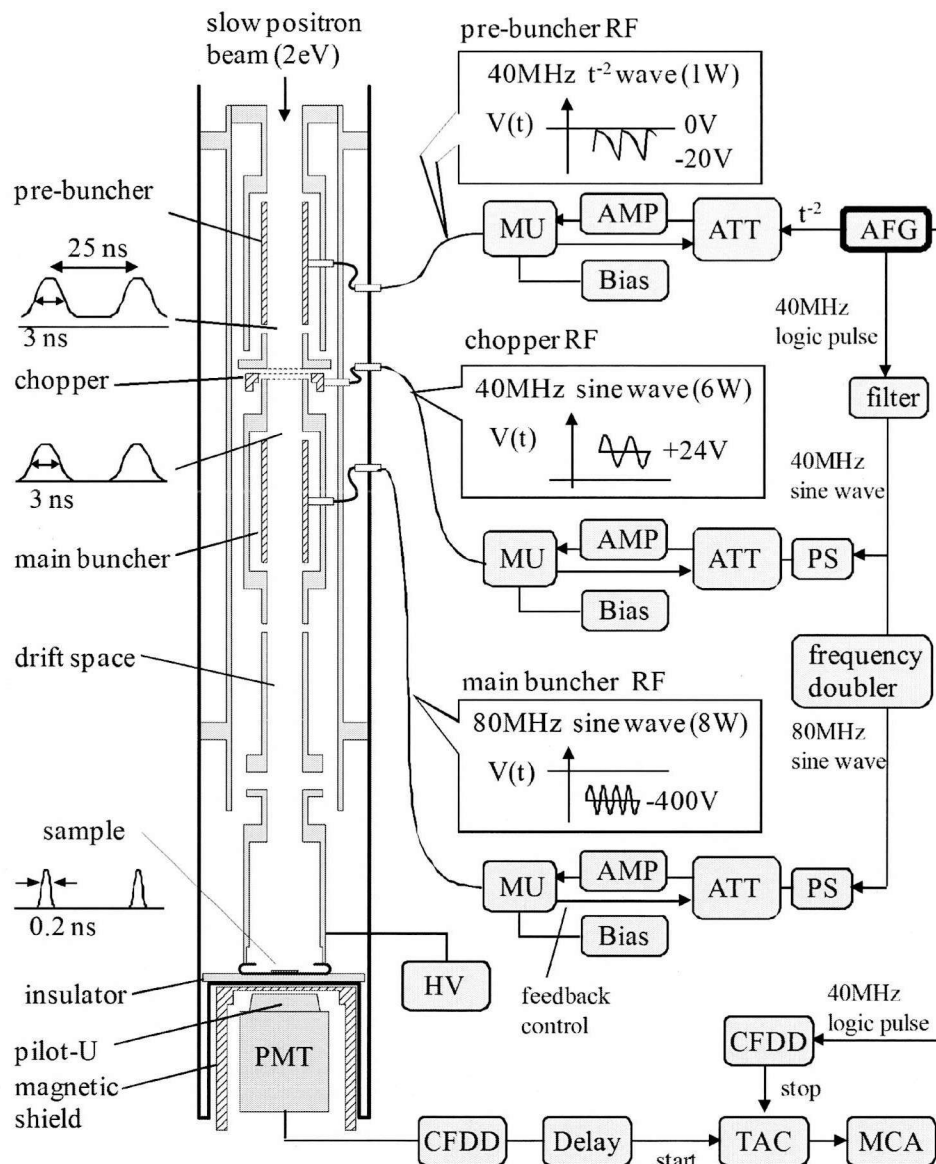
図 2.3-8 高周波回路システム系統図、及び各電極に印加される波形の概形。
