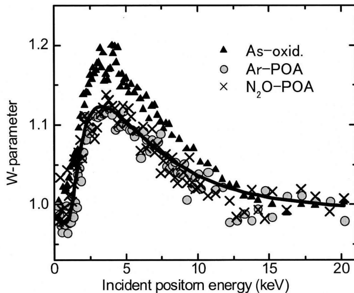
図 3.1-10 Ar および N 2 O ガスを用いた POA 処理の、界面中間層における電子運動量分布への影響。
