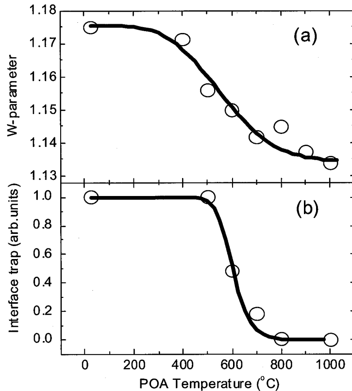
図 3.1-9 (a)電子運動量分布測定における p=10\sim15\text{mrad} 領域の強度変化、および(b)C-V 測定における界面準位量の熱処理温度依存性の比較。
