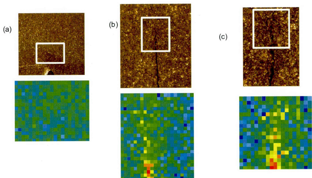
図 3.2-7 試料に熱鋭敏化した SUS316L を用いた場合の試験結果。(a)が亀裂進展前、(b)が 100 時間、(c)が 190 時間のものである。上は光学顕微鏡像、下は枠内を陽電子マイクロビームで走査した S パラメータ分布。走査エリア(横)は 800 ミクロン。
