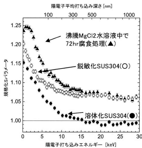
図 3.2-13 鋭敏化 SUS304 試料片の、MgCl 腐食前後における S パラメータの陽電子入射エネルギー依存性(深さ依存性)。比較のため、溶体化 SUS304 の測定結果も示す。
