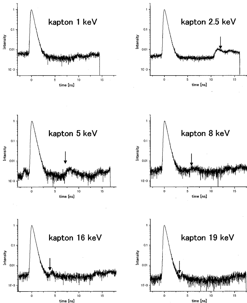
図 2.3-12 測定された陽電子消滅寿命スペクトルの例(カプトン)。打ち込みエネルギーを変化させた場合のスペクトルの変化。矢印はサブピーク位置を示す。
