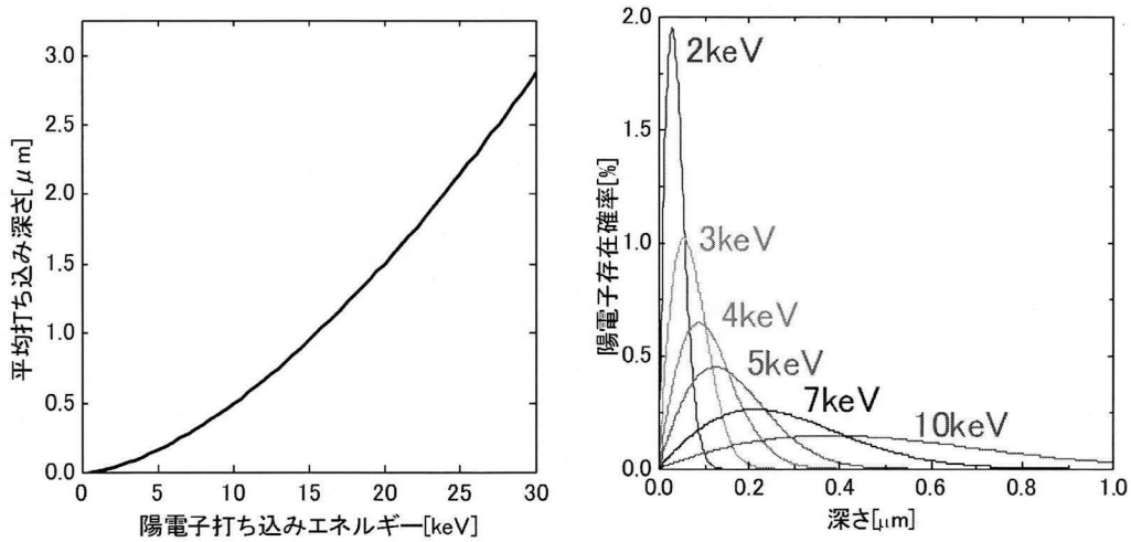
図 2.1-6 SiC に対する陽電子の(左)平均打ち込み深さ、(右)打ち込みプロファイルの計算結果。
