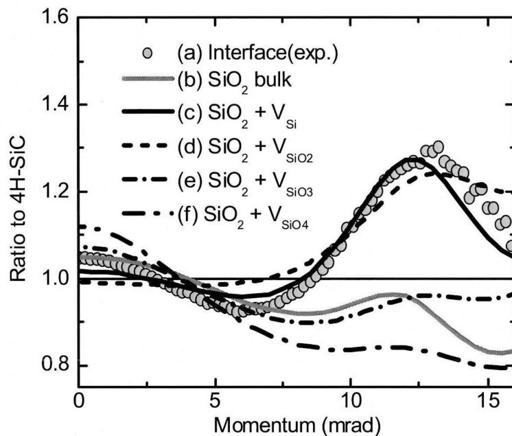
図 3.1-3 測定された E=3.7\text{keV} での運動量分布の比率曲線、および第一原理計算によって得られたいくつかの欠陥構造の運動量分布。
