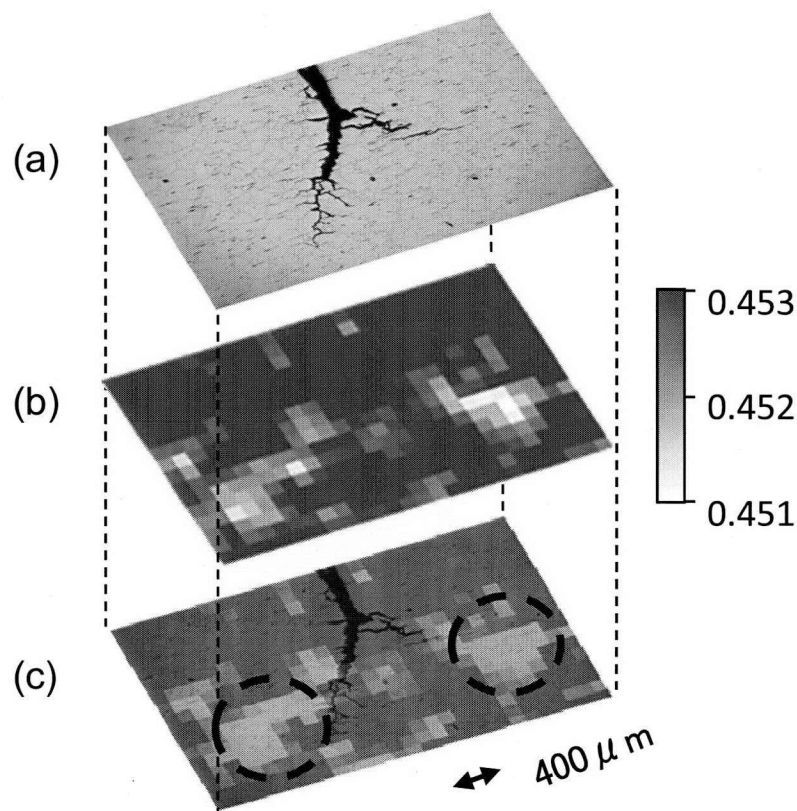
図 3.2-2 S パラメータの二次元分布測定を行った結果。(a)応力腐食割れを生じたステンレス材の亀裂先端部分の光学顕微鏡像。(b)対応する領域での S パラメータ分布。(c)両者を重ね合わせたもの。
