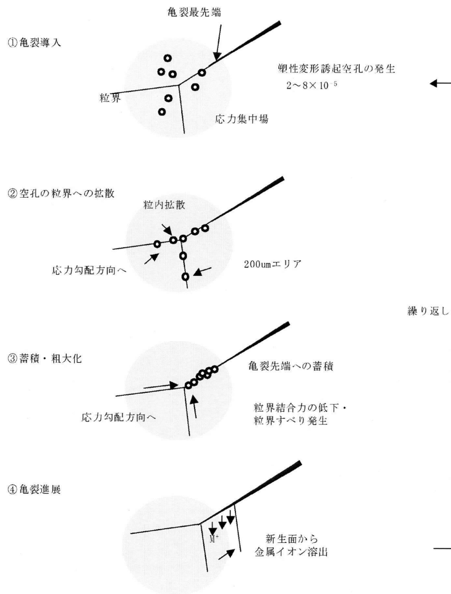
図 3.2-15 陽電子マイクロビームを用いて測定した結果から考えられる、空孔の発生と亀裂進展への影響モデル。
