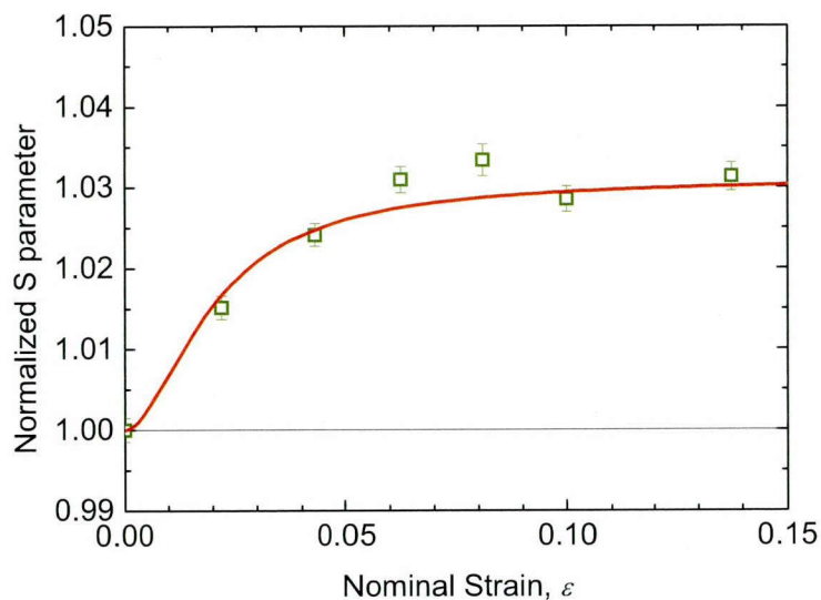
図3.2-12 引っ張り試験片のSパラメータの変形量依存性。
