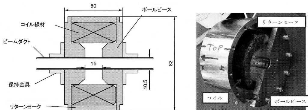
図 2.4-4 (左)磁界レンズ概略図と(右)分解写真。ポールピース間のギャップ間隔は15mm、リターンヨーク外形は \phi 82 \times 50 mm。ビームダクト直径は10mm。軟鉄製。
