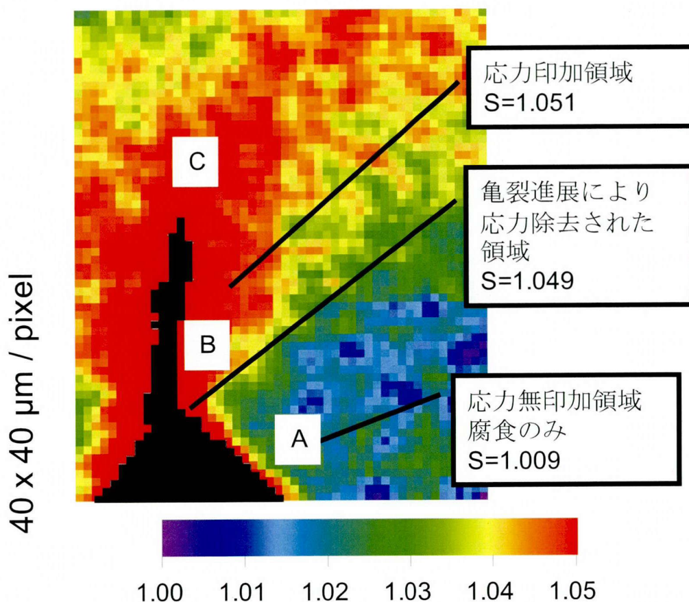
図 3.2-9 鋭敏化 SUS304 試料に応力を印加し腐食させたのち、亀裂を含む広範囲な領域で S パラメータ分布を測定した結果。
