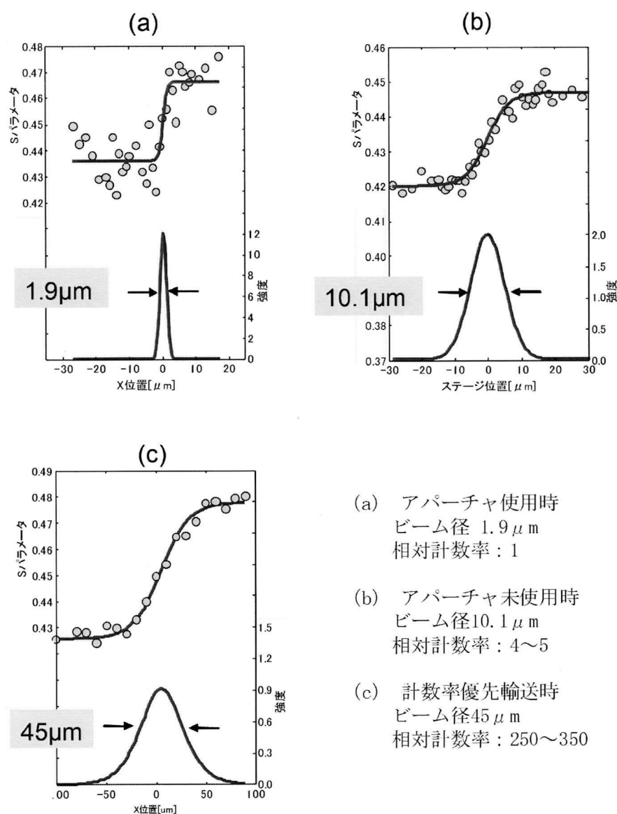
図 2.4-7 ビーム収束条件によるビーム径と強度変化。
