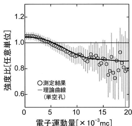
図 3.2-3 欠陥蓄積領域における電子運動量分布測定結果と、第一原理計算による単空孔欠陥モデル計算結果との比較。
