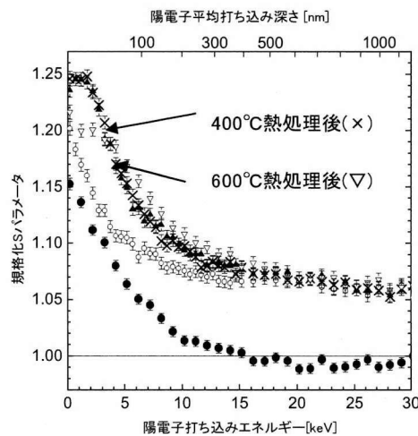
図 3.2-14 ステンレス腐食処理試料に 400 度および 600 度の等時昇温処理を加えた場合の S パラメータ深さ分布測定結果。比較のため、図 3.2-13 の結果も併記する。
