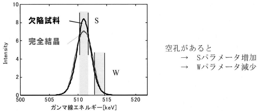
図 2.1-2 S パラメータ及び W パラメータの定義
