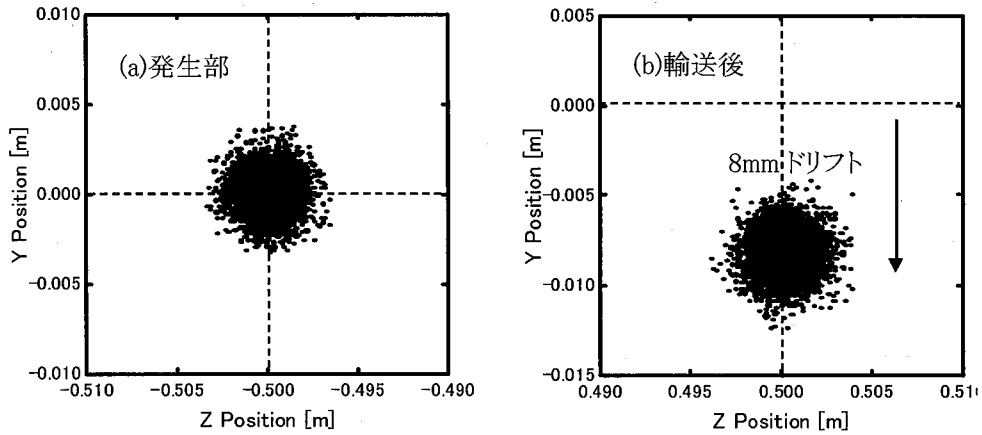
図 2.3-4 曲率ドリフトの計算結果。
