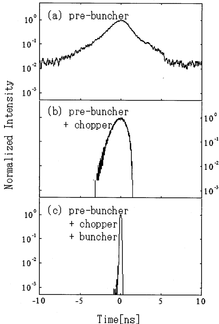
図 2.3-7 (a)プリバンチャー出口、(b)チョッパー出口、(c)試料位置におけるビームパルス時間構造の計算結果。
