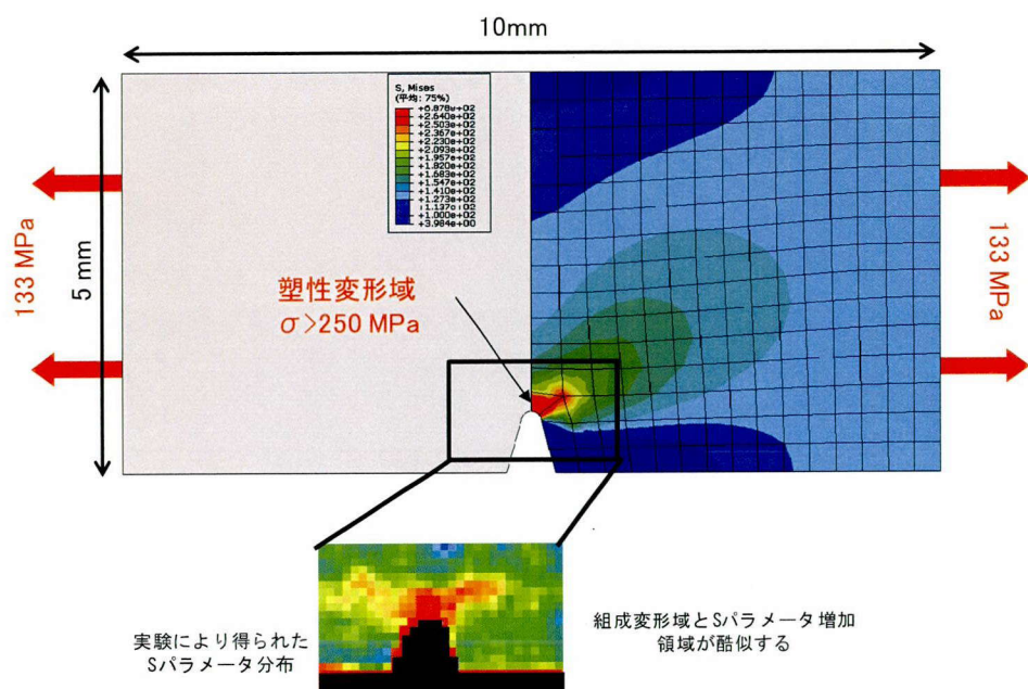
図 3.2-11 有限要素法により切り欠き部周辺における応力分布の計算を行った結果と、塑性変形を起こした引っ張り試験片の S パラメータ分布を比較したもの。
