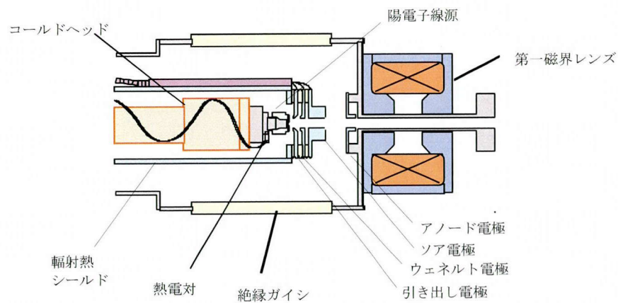
図 2.4-14 陽電子銃部概略図。線源はコールドヘッド先端にマウントされ、ビーム形成電極を取り付けた輻射熱シールドで覆われる。
