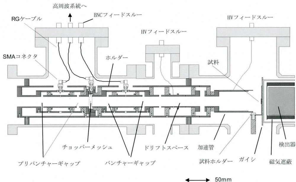
図 2.3-5 開発したパルス化装置の概略構造。
