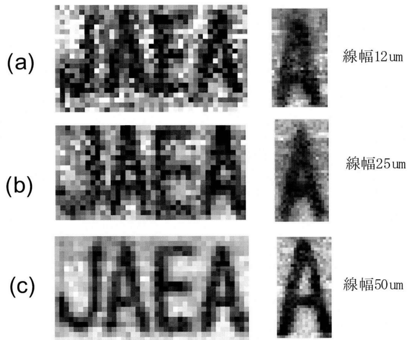
図 2.4-11 陽電子マイクロビームにより測定されたテストパターン。走査領域は図 2.4-10 の矩形領域に対応する。右は「A」文字の高精細像。
