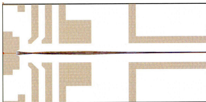
図 2.4-16 SIMION7 コードを用いて計算した陽電子銃部でのビーム挙動計算結果。最終的にビーム径 0.2mm のビームが得られた。ビーム加速電圧 20kV。
