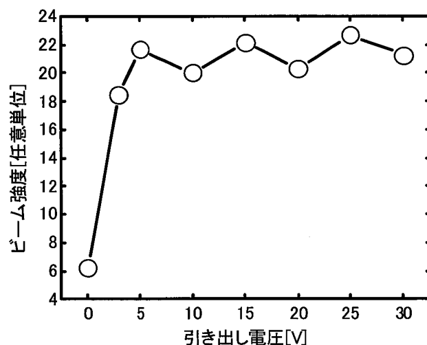
図 2.3-3 減速材からの引き出し電圧と発生陽電子ビーム強度。
