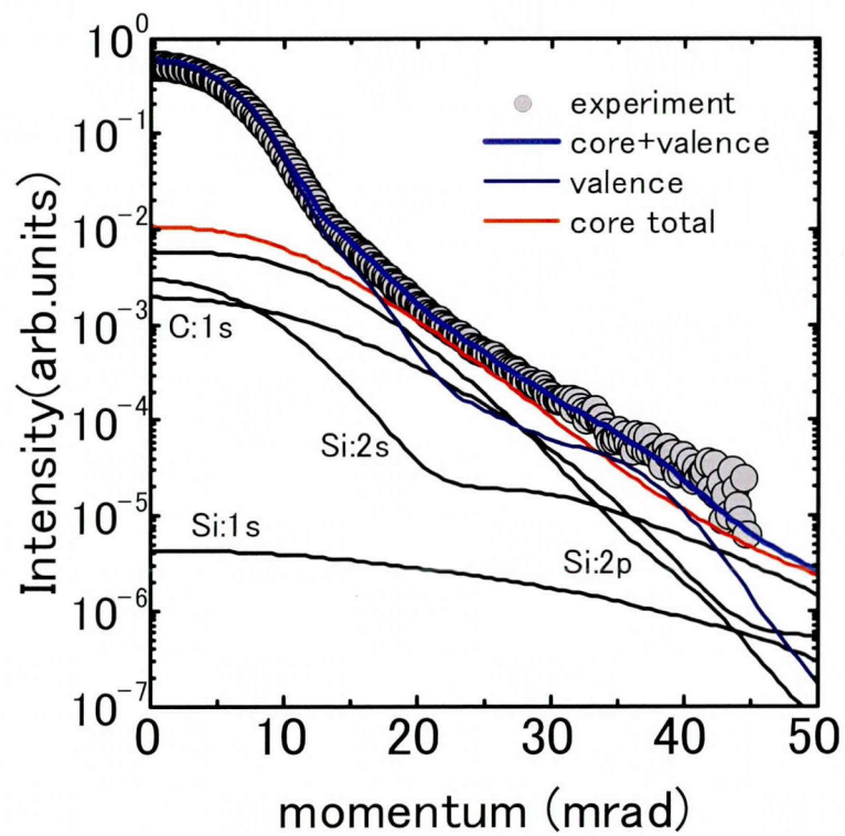
図 2.5-1 陽電子状態計算コードにより計算されたSiCの運動量分布およびCDB測定によって得られた実験値との比較。
