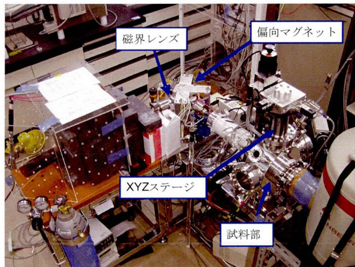
図 2.4-2 マイクロビーム装置全体写真。
