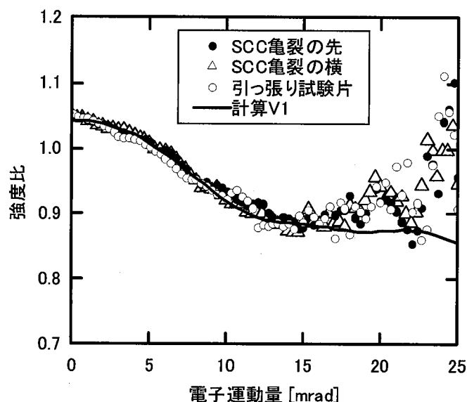
図 3.2-10 引張試験片のガンマ線エネルギー分布ならびに応力腐食割れ亀裂先端部のガンマ線エネルギー分布の運動量分布を詳細に測定し、比率曲線を導出したもの。理論計算による V1 欠陥の計算結果もあわせて示した。
