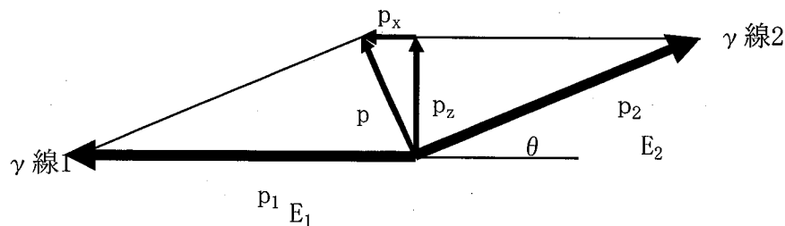
図 2.1-1 角相関法及びドップラー法の原理
