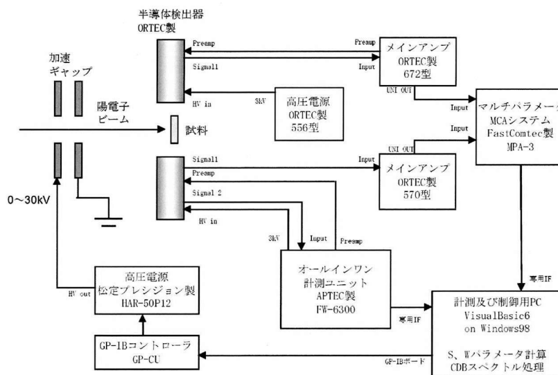
図 2. 2-2 エネルギー可変低速陽電子ビーム装置の計測制御系ダイアグラム
