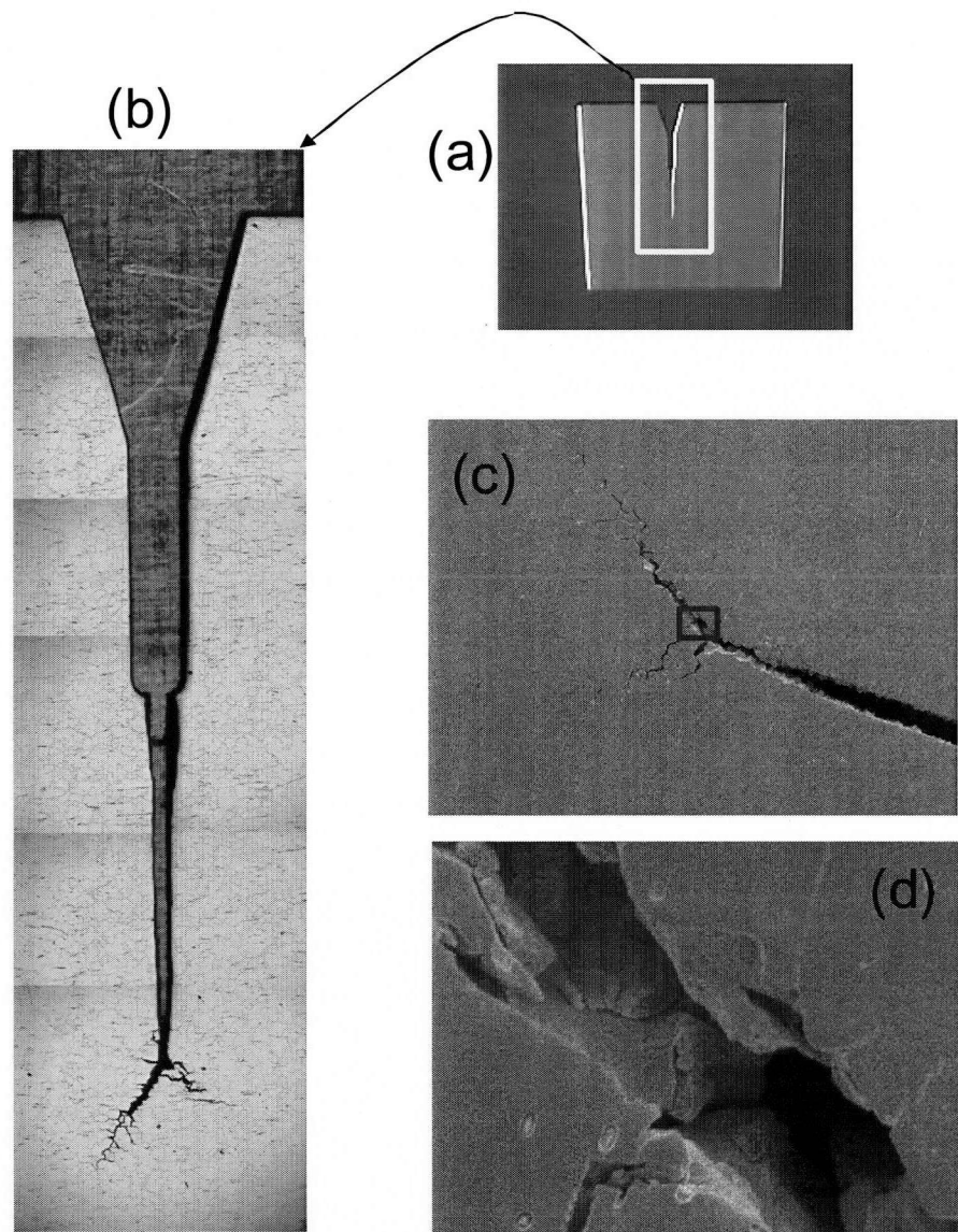
図 3.2-1 SCC 亀裂を誘発させた SUS304 試料の光学顕微鏡像および電子顕微鏡像
