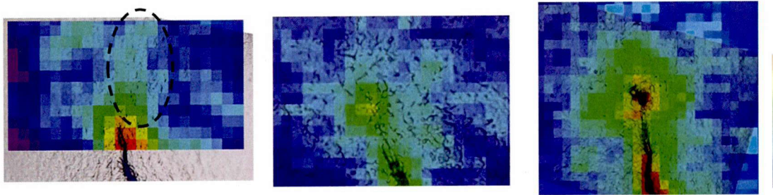
図 3.2-6 試料に熱鋭敏化 SUS304 を用いた場合の、腐食環境にさらしながら亀裂の進展状態を繰り返し観察した結果。左から腐食前、腐食時間 24 時間、腐食時間 100 時間のものである。光学顕微鏡写真と S パラメータ分布を重ね合わせてある。S パラメータ分布の 1 ピクセルは 50 ミクロン。
