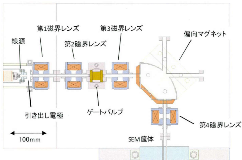
図 2.4-3 陽電子ビーム輸送・収束部の概略図。4つの磁界レンズと偏向マグネットによりビームを線源部からSEM筐体まで輸送する。
