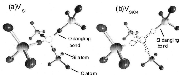
図 3.1-4 計算に用いた欠陥構造の模式図。(a) \text{Si} 空孔、(b) \text{SiO}_4 空孔。
