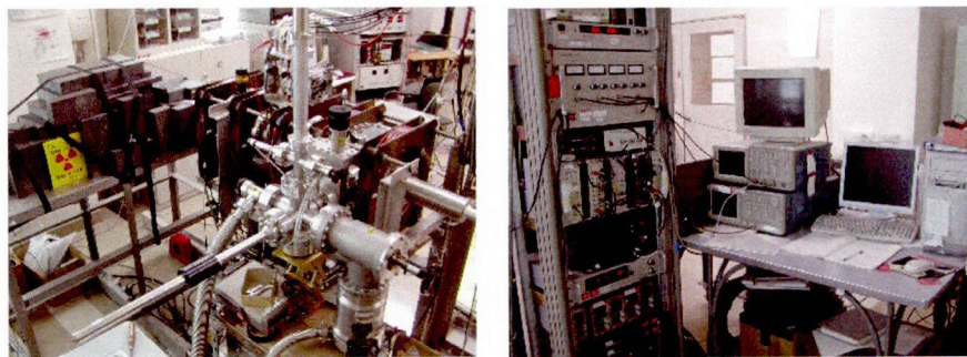
図 2.3-1 開発したパルス化装置の全体外略図(上)、および外観写真(下)。
