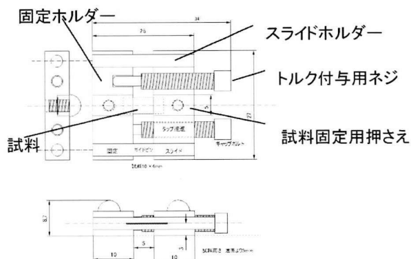
図 3.2-4 新たに開発した応力印加ホルダー概略図及び外観図。
