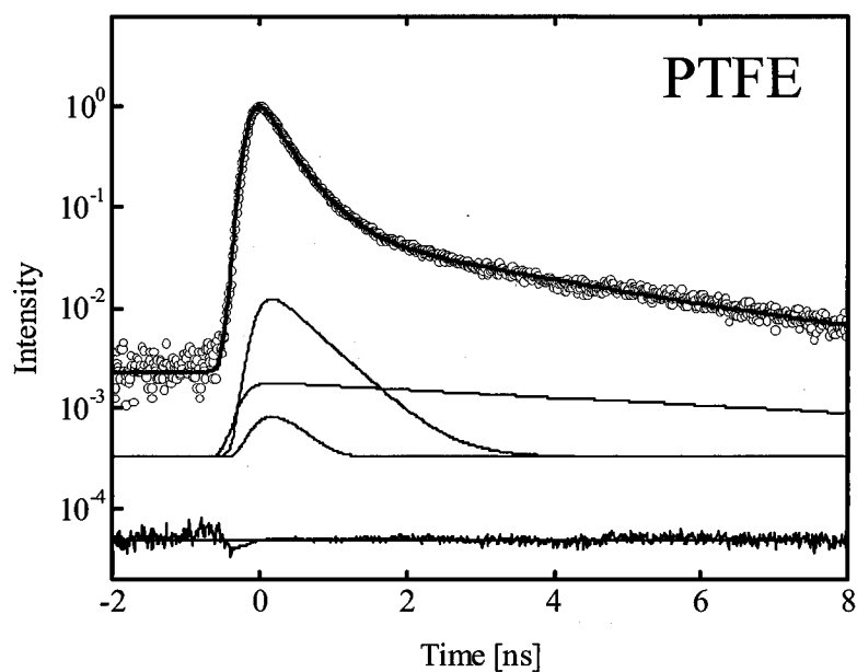
図 2.3-15 測定された陽電子消滅寿命スペクトルの例(PTFE)。
