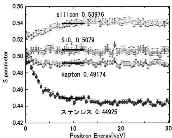
図 2. 2-3 いくつかの物質に対する S パラメータの陽電子打ち込みエネルギー依存性 (S-E 曲線) 測定結果。E=8keV~13keV における平均 S パラメータの値もあわせて示す。
