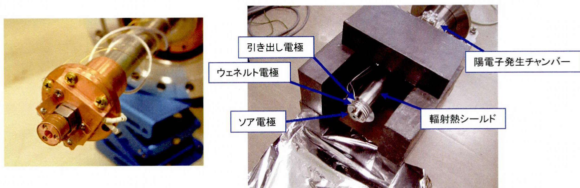
図 2.4-15 左：コールドヘッドにマウントされた線源。右：陽電子銃部外観図。
