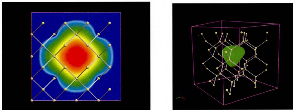
図 2.5-2 原子空孔を導入した結晶構造において計算した陽電子の波動関数分布。欠陥に局在している。
