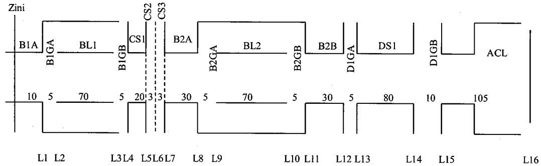
図 2.3-6 ビールパルス化挙動計算にもちいた計算モデル。
