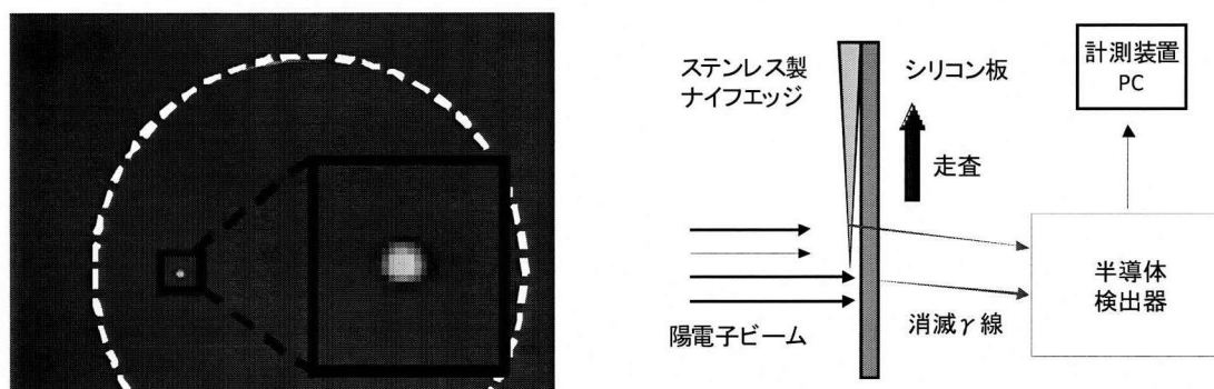
図 2.4-6 (左)MCP で観測された陽電子ビーム像。破線は直径 10mm の有効径を示す。(右) ナイフエッジ法によるビームサイズ決定法の概略図。
