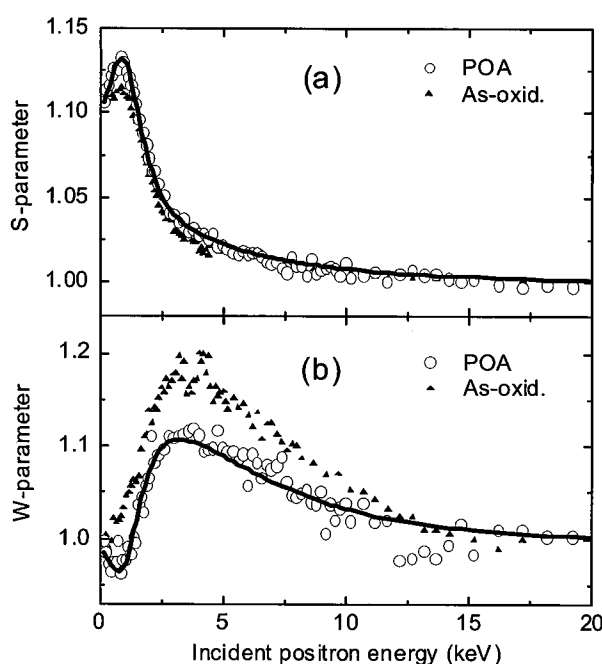
図 3.1-6 POA 処理後に得られた S-E 及び W-E カーブ。
