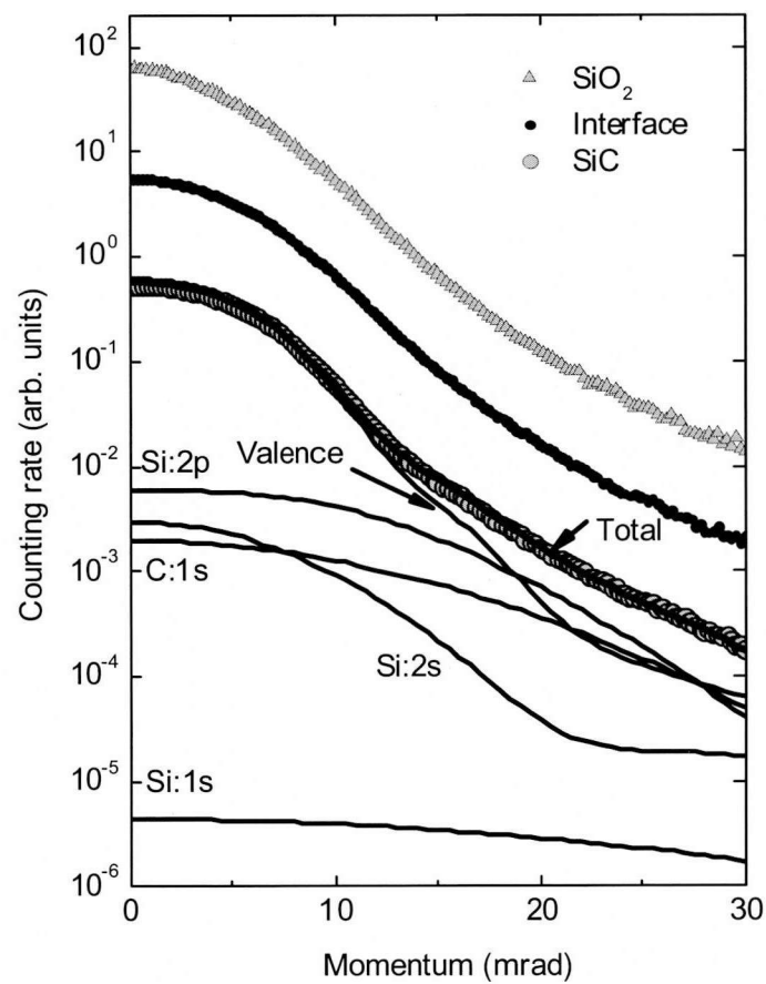
図 3.1-2 CDB 測定によって得られた運動量分布および計算によって得られた SiC バルクに対する運動量分布。
