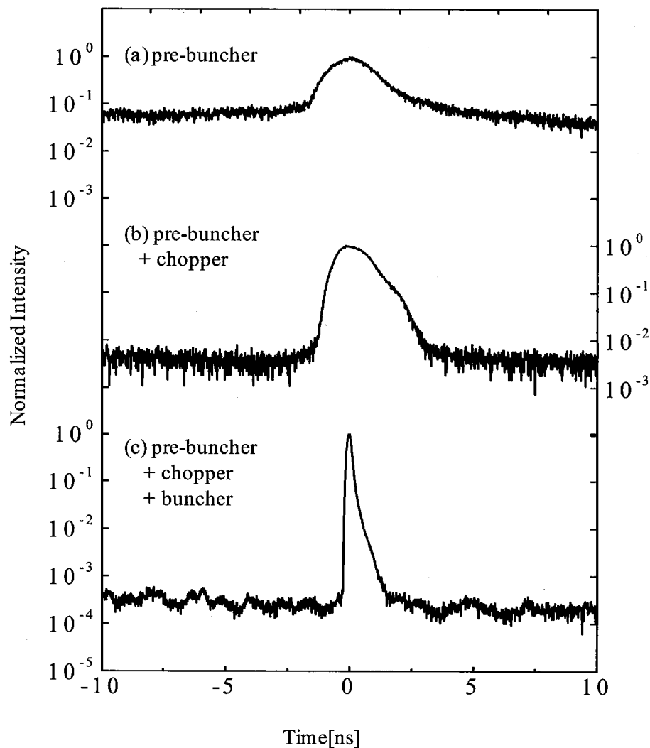
図 2.3-11 高速 MCP により計測されたパルスビーム時間構造。
