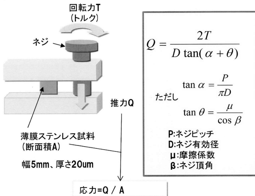
図 3.2-5 ネジの回転力による試料への応力印加およびその換算式。ステンレスの破壊応力(500～1000MPa)に対し、M4 ネジで 50～100kgf-cm に相当。また応力腐食割れに必要な応力(～100MPa) は、十分印加可能。
