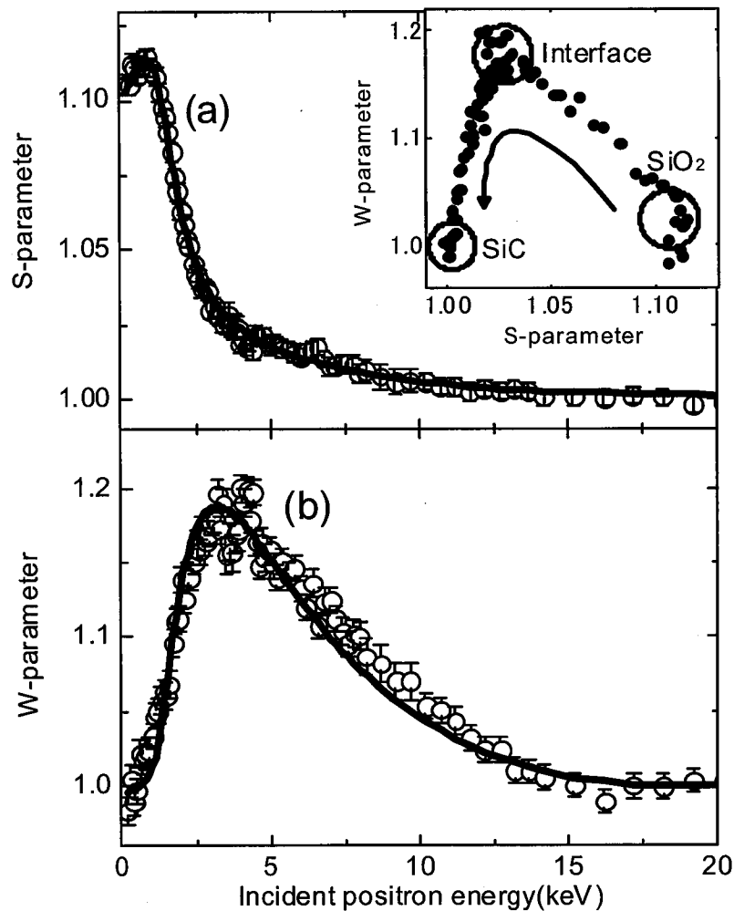
図 3.1-1 ドライ酸化試料に対する(a)Sパラメータ、(b)Wパラメータの陽電子打ち込みエネルギー依存性。(a)にはS-Wプロットをあわせて示す。
