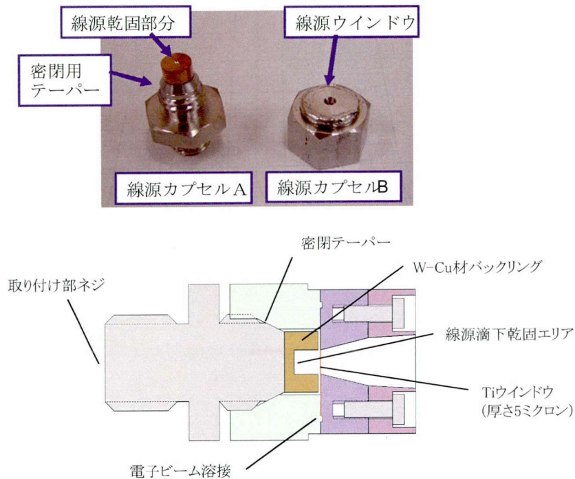
図 2.4-12 製作した小型密閉線源の概略図と外観図。 ^{22}\text{Na} 線源はタングステン-銅合金の上に設けられた窪み(線源乾固面積)に NaCl 結晶として付着させる。その後チタン箔を電子ビーム溶接したフタで、テーパ密着により密閉する。
