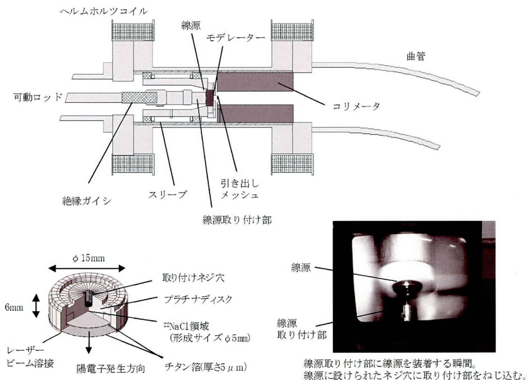
図 2.3-2 線源および陽電子発生部の構造。
