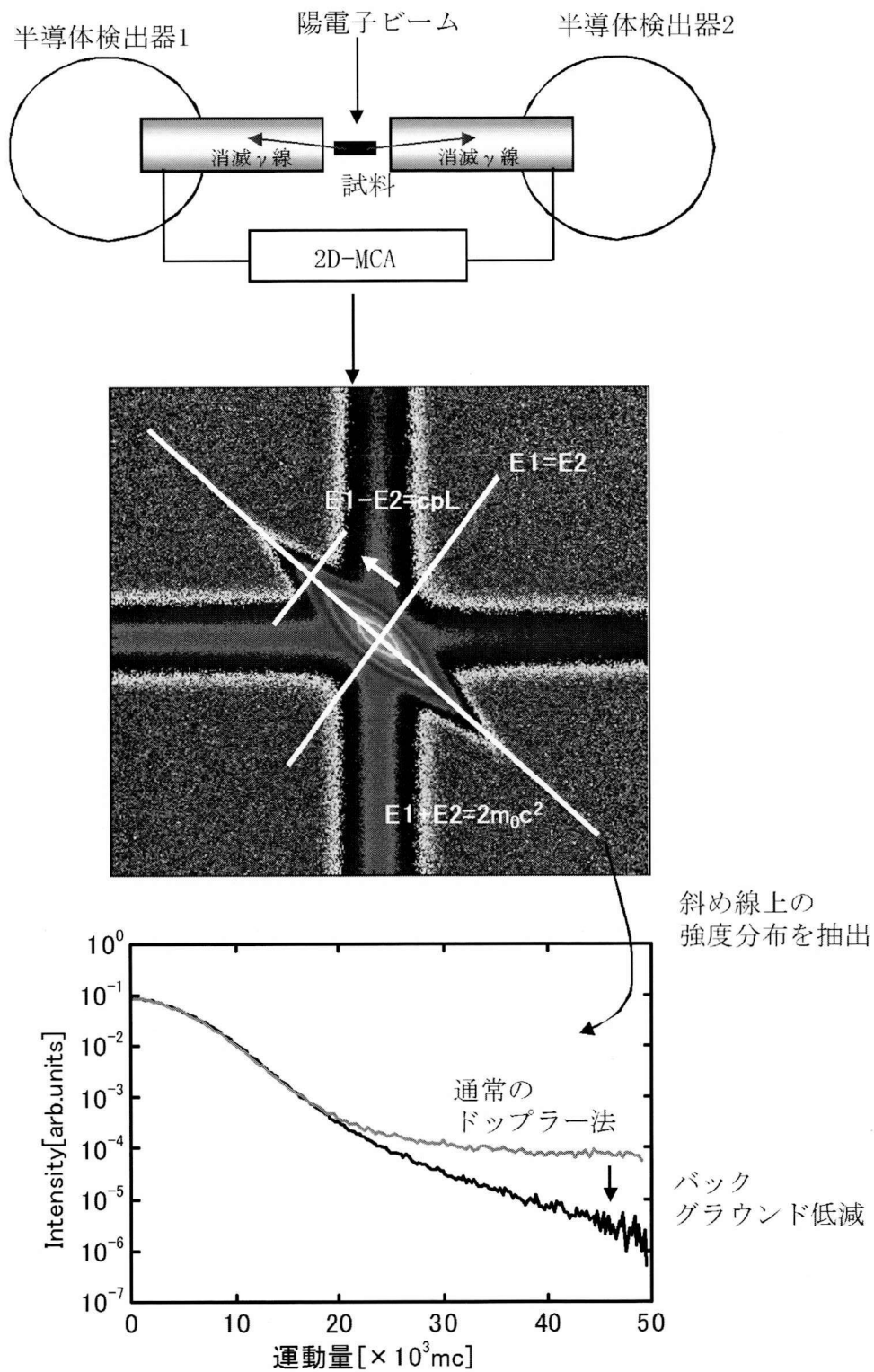
図 2.1-4 CDB 計測システムおよびデータ例
