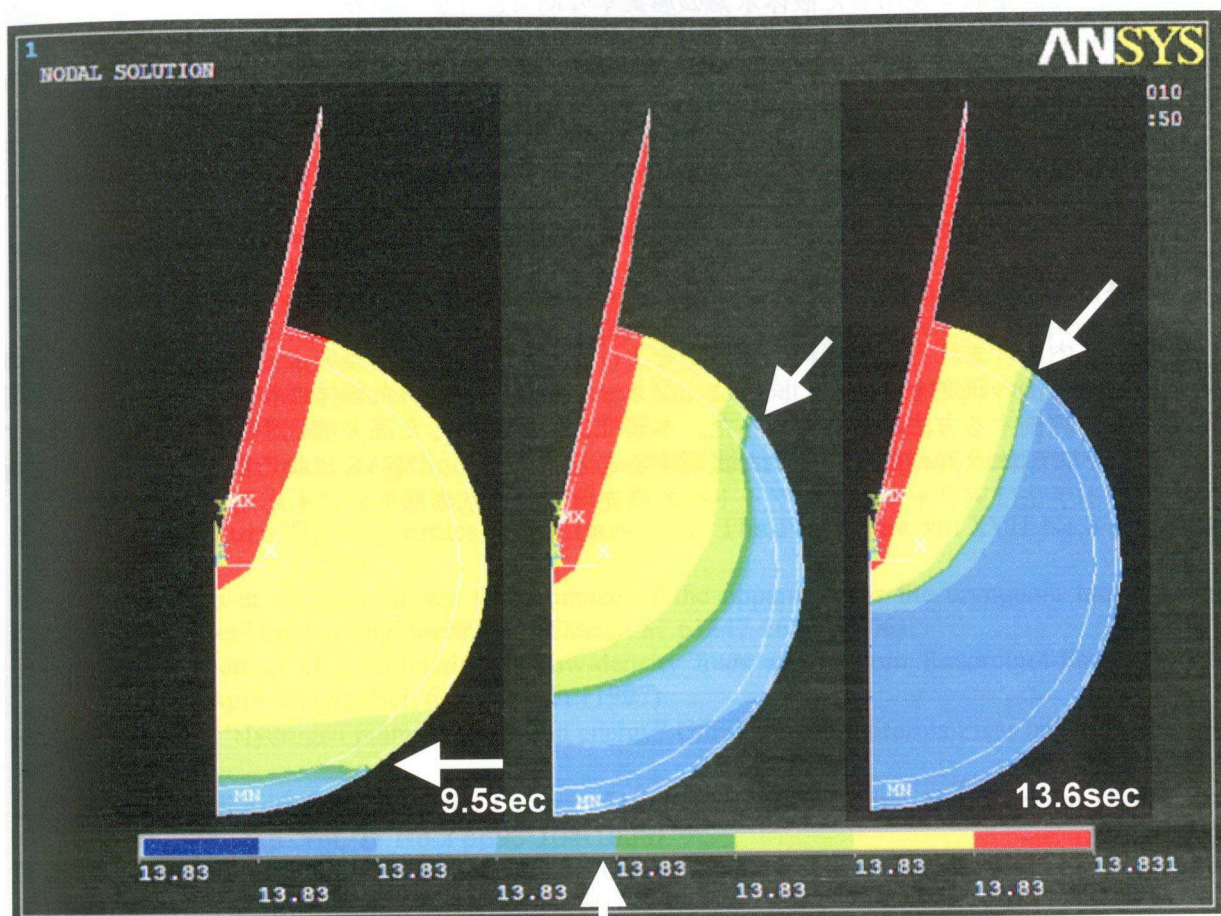
図4-25 ANSYSによる温度差は全体で1mK以下しかついていないが、矢印の部分で層変化が起こっている。
