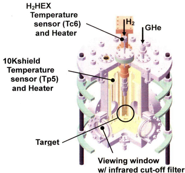
図5-2 ターゲット容器の詳細。ガスヘリウムはターゲット容器内部に、水素ガスはターゲットに充填できるようになっている。
