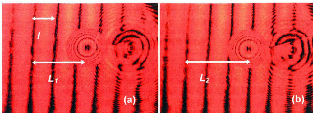
図3-11 フォームセル内部が真空状態の干渉縞(a)と、六フッ化硫黄ガスを 0.1MPa 充填した直後の干渉縞の写真(b)。このとき模擬サンプルとしてポリスチレンセルを使用した。
