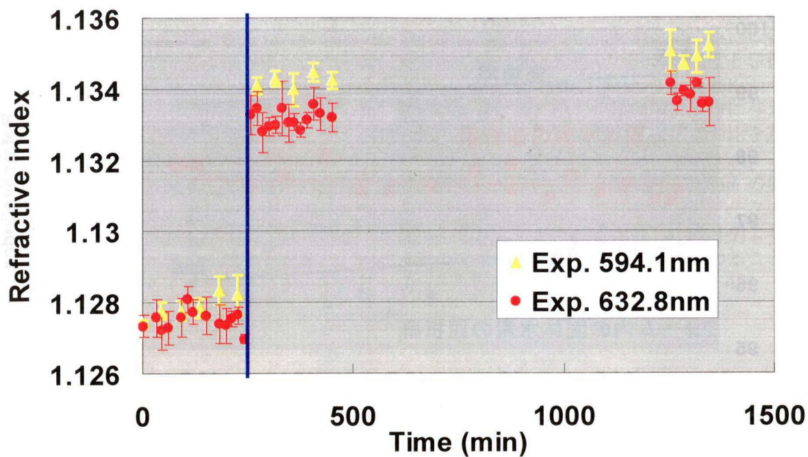
図4-2-1 フォーム内に含まれる固体水素の屈折率の時間変化。
