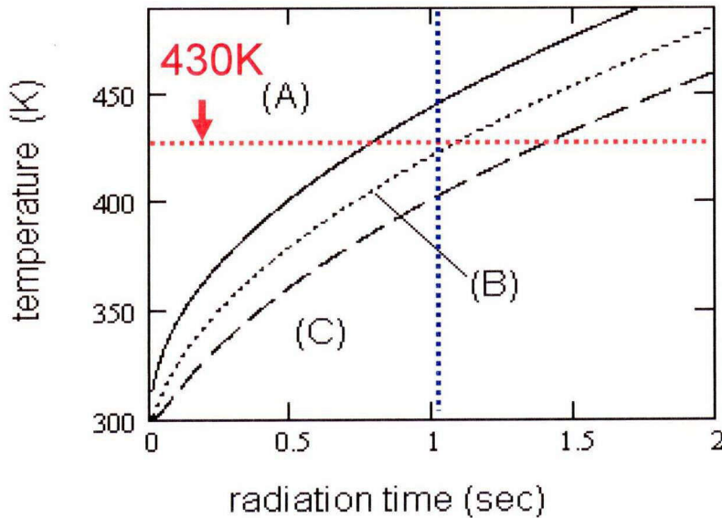
図2-3 レーザー強度を 6.4 \times 10^3 \text{ W/cm}^2 に固定し、照射時間と温度上昇の関係を計算した。(A) は表面上の温度、(B)は 50\mu\text{m} の深さの温度、(C)は 100\mu\text{m} の深さの温度を示している。
