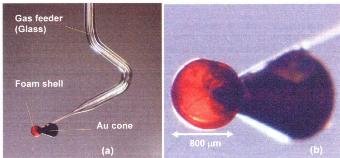
図 5-3 金コーン付き直径 800 \mu\text{m} のフォームシェルターゲットの全体図(a) とフォームターゲット部分の拡大写真(b)。
