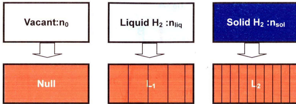
図4－3 充填した内容物と干渉縞の間隔の対応関係を模式的に示す。中に何も入っていない状態において参照光と物質光の光路をそろえることで干渉縞は null になる。シェアリング干渉計のため、参照光は光線のうちサンプルを透過していない部分を使用する。
