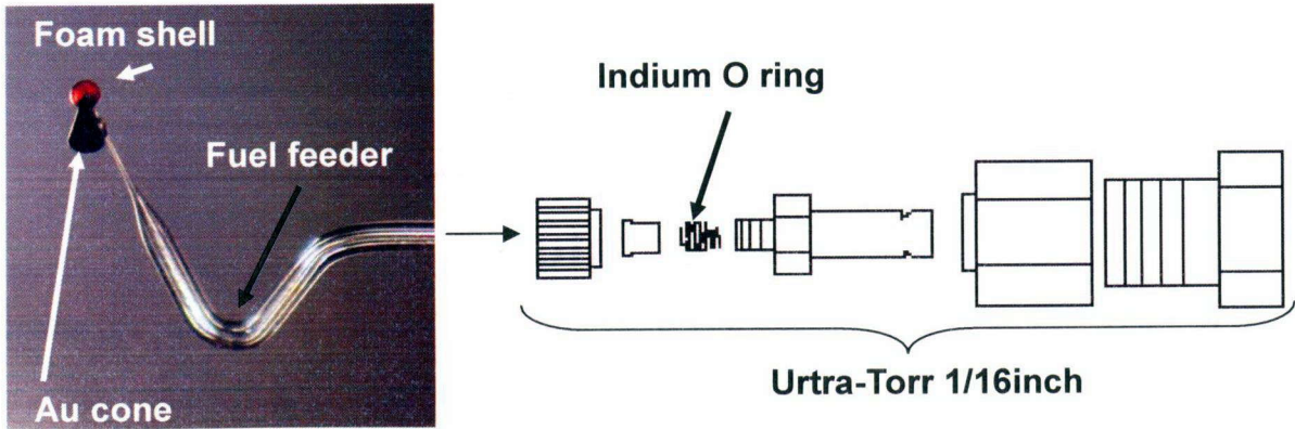
図 5-5 ターゲットの燃料導入管と水素配管の接続の概略図。インジウムを O リングとして使用した。
