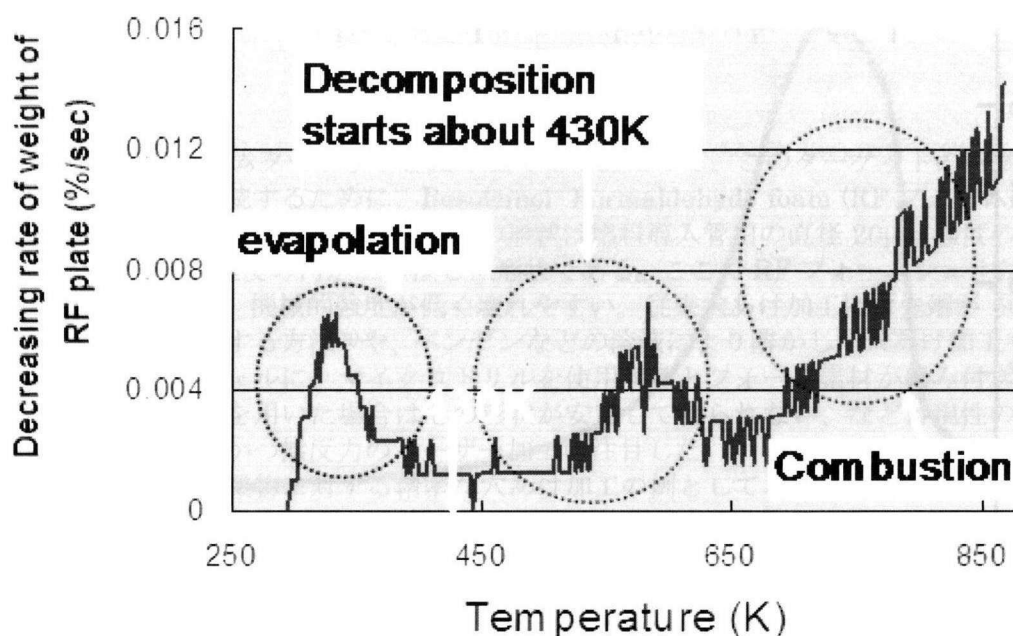
図 2-2 RF フォームの熱重量分析の結果。横軸は温度、縦軸は質量減少率である。熱分解は 430K ほどから始まっているものと考えられる。
