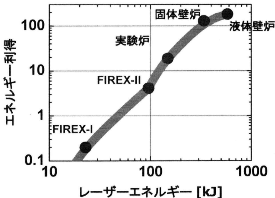
図1-4 高速点火発電に向けたロードマップ。現在は FIREX-I であり、FIREX-II にて自己燃焼のメカニズムを明らかにし、FIREX 計画の段階で炉心プラズマの基本的な物理を確立する。
