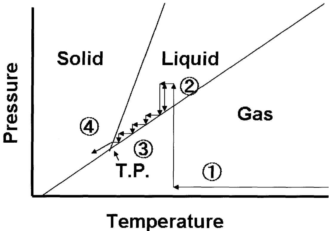
図 5-7 パリレンコーン付き直径 500 \mu m のフォームシェルターゲットを用いた燃料充填、固化実験におけるターゲット内部の温度と圧力の制御の模式図。①10K シールドの温度を 13.5K で制御し、水素ガスをシェル内に供給、飽和蒸気圧以上まで加圧し液化させる。②液体がフォーム層に充填された状態でシェル内の蒸気圧を調節することで充填量を調節・維持する。③10K シールドの制御温度を下げていく、ここで 1step あたりの温度低下は 10mK である。温度の低下とともにシェル内の蒸気圧を飽和蒸気圧に保ち、内部の充填量を一定に保つ。④10K シールドの温度を下げて固化させる。パリレンコーンにレーザーを照射し、充填率向上を目指した実験と、比較としてレーザーを照射しない場合の実験を行った。この図の T.P. はパラ水素の三重点(13.8K, 8kPa)を示す。
