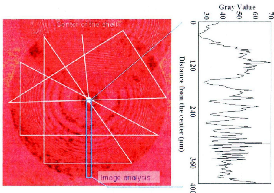
図6-2 幾何学的方法によって、直角三角形を3つ用いたその交点を干渉像におけるシェルの中心とする。シェルの干渉像に四角で囲ったエリアの濃淡を画像解析すると右図のようになる。
