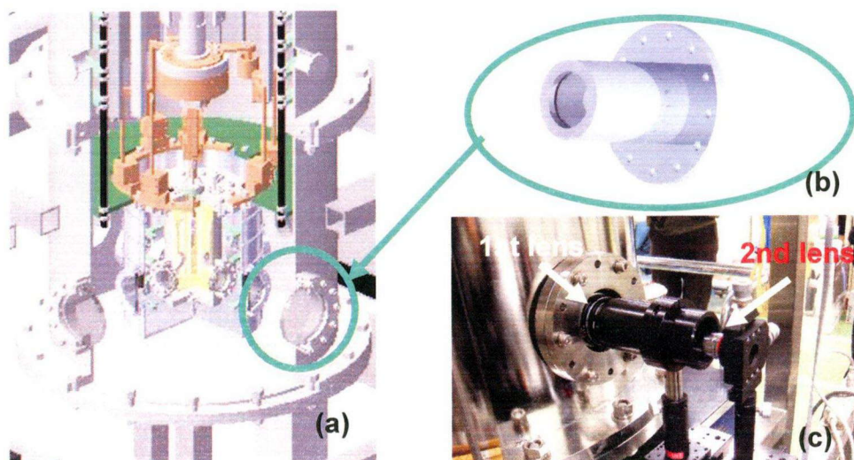
図5-1 干渉計測のための真空容器側改良を示す図。真空断熱層と大気の間にある外側チャンバーの計測用窓(a)に計測窓つき筒(b)を差込み(c)にしめすように1st レンズをターゲット容器により近づける。
