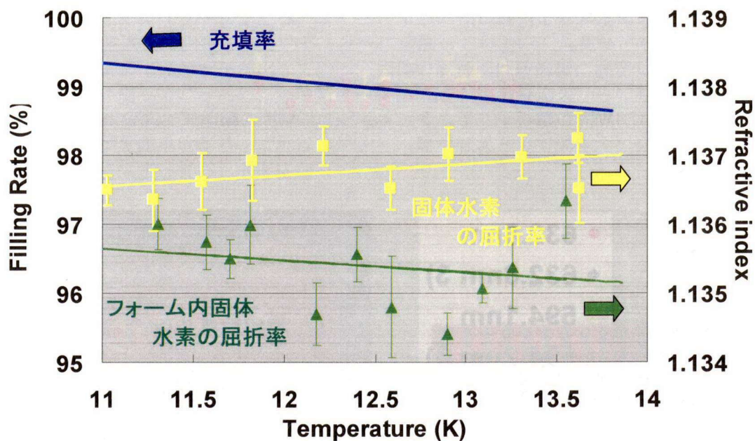
図4-24 黄色レーザーの結果を用いて RF フォーム内の固体水素の充填率を評価した。青色直線が充填率のグラフであり、左側の軸の値を取る。黄色四角は固体水素の屈折率であり、その最小二乗法による直線が黄色の線である。フォーム内の固体水素の屈折率は緑三角で表現しており、この最小二乗法による直線が緑色線である。固体水素の屈折率およびフォーム内の固体水素の屈折率は右側の軸の値をとる。
