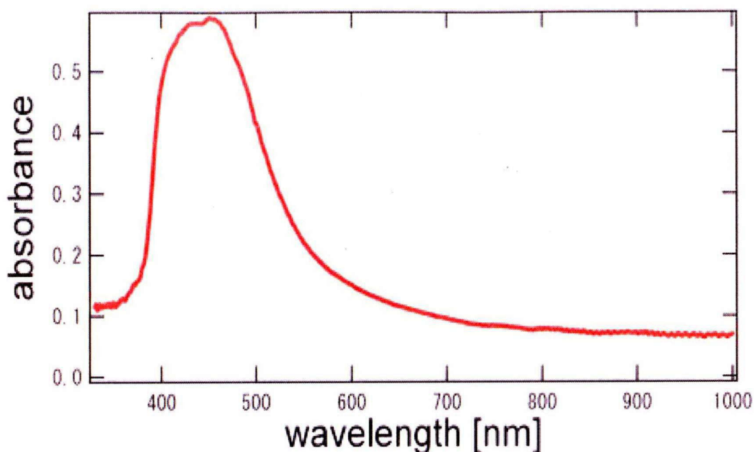
図 2－1 RF 平板の吸光度。RF 平板は厚みが 200 \mu\text{m} である。横軸は光の波長、縦軸は吸光度である。
