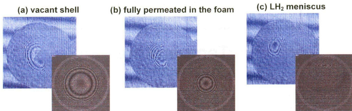
図 5-9 RF フォームシェルターゲットに模擬燃料を充填していく様子。(a)空の状態から、(b)液化が進み、(c)コーン付近にメニスカスができいくそれぞれの干渉縞の写真 (左上)。及び Shell's Optic Model により計算した干渉縞の計算結果 (右下)。
