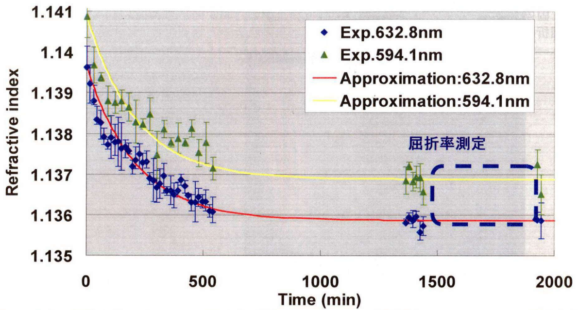
図4－18 固体水素のオルソーパラ水素変換に伴う屈折率の時間変化。式4－12による近似式を図中に示す。
