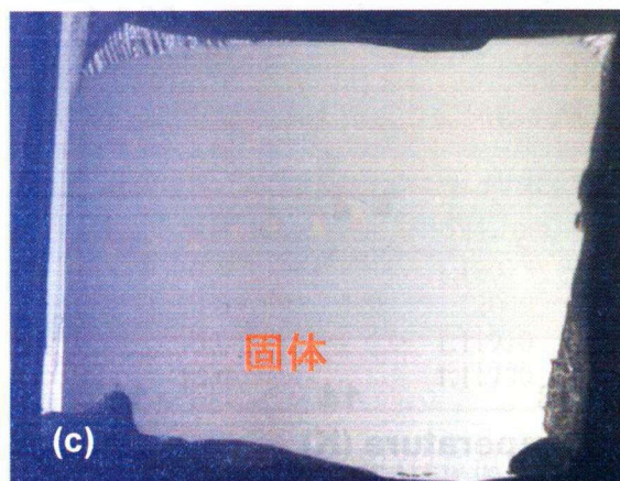
図4-17 実体顕微鏡による各状態における写真。(a)水素を加圧していき気液界面がウェッジの鋭角な側から生じた。界面を境に気体側が null、液体側に干渉縞が生じた。(b)温度を下げるにつれ下部から固液界面が発生し上に向かっていった。界面にあわせて干渉縞がシフトし、固化後は縞間隔が狭くなっている。(c)全体が固化した写真。
