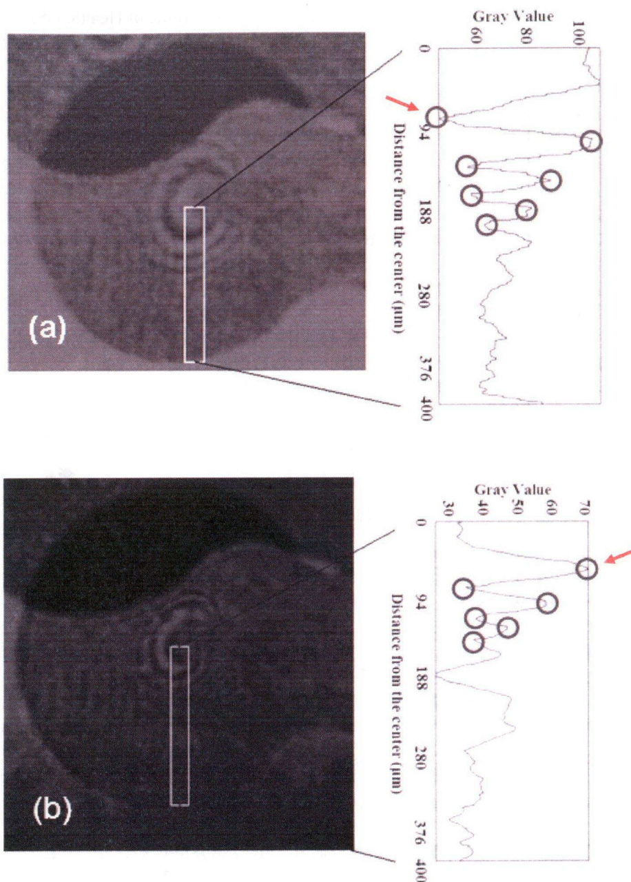
図6-3 干渉縞の写真と、その画像解析した強度プロファイルを示す。(a)水素を充填していない状態と(b)液体状水素を充填後、固化させた24時間経過後の状態。赤矢印は基準となる明線もしくは暗線。
