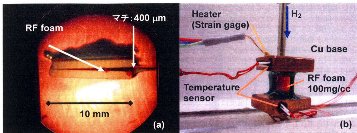
図4－9 燃料充填率測定実験に用いるサンプルの写真。フォームの入ったウェッジの上部から観察したもの(a)、と完成図(b)。
