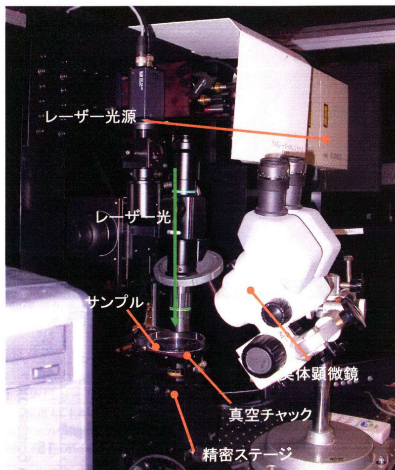
図 2-4 レーザー加工用実験装置の写真。実体顕微鏡は斜めからターゲットとレーザー光を観察する。
