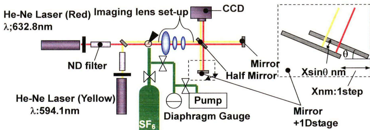
図 3-10 気密性を試験するための装置の概略図。1 軸ステージの移動分解能を高める技術の概略を右上に示す。
