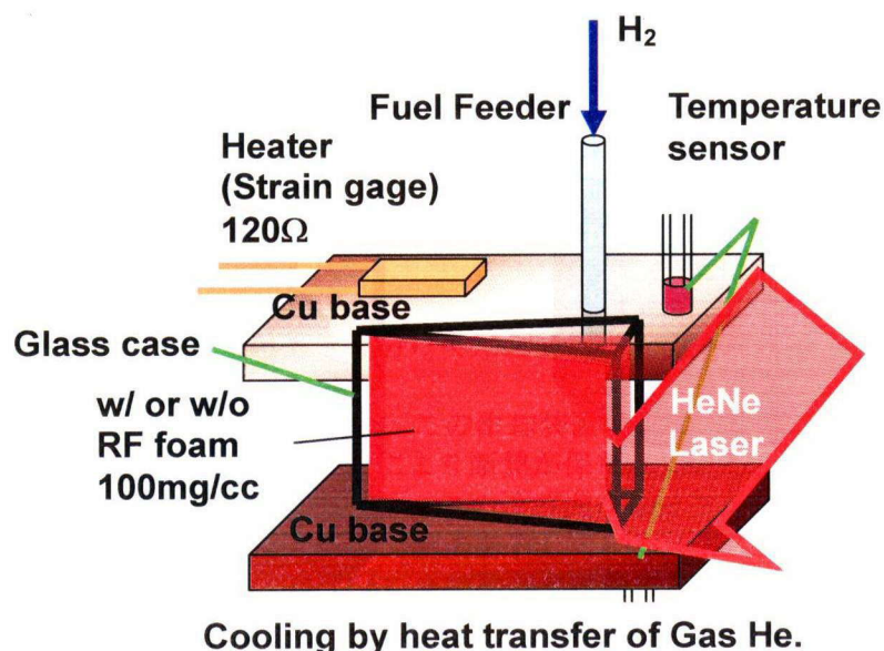
図 4－7 燃料充填率測定実験に用いるサンプルの模式図。
