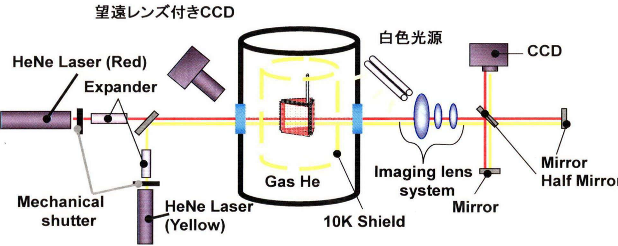
図4-13 計測装置の概略図。二種類のレーザーによる干渉計と、実体顕微鏡による計測から成り立っている。
