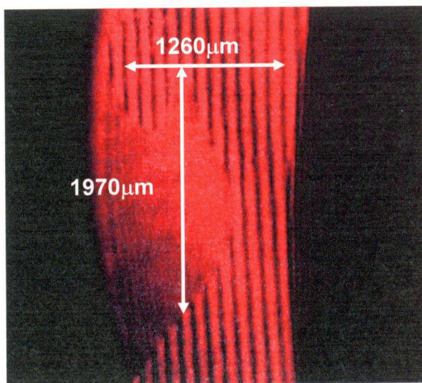
図4-26 液体水素を充填したフォームなしウェッジサンプルの赤色( \lambda=632.8\text{nm} )レーザーによる干渉像。
