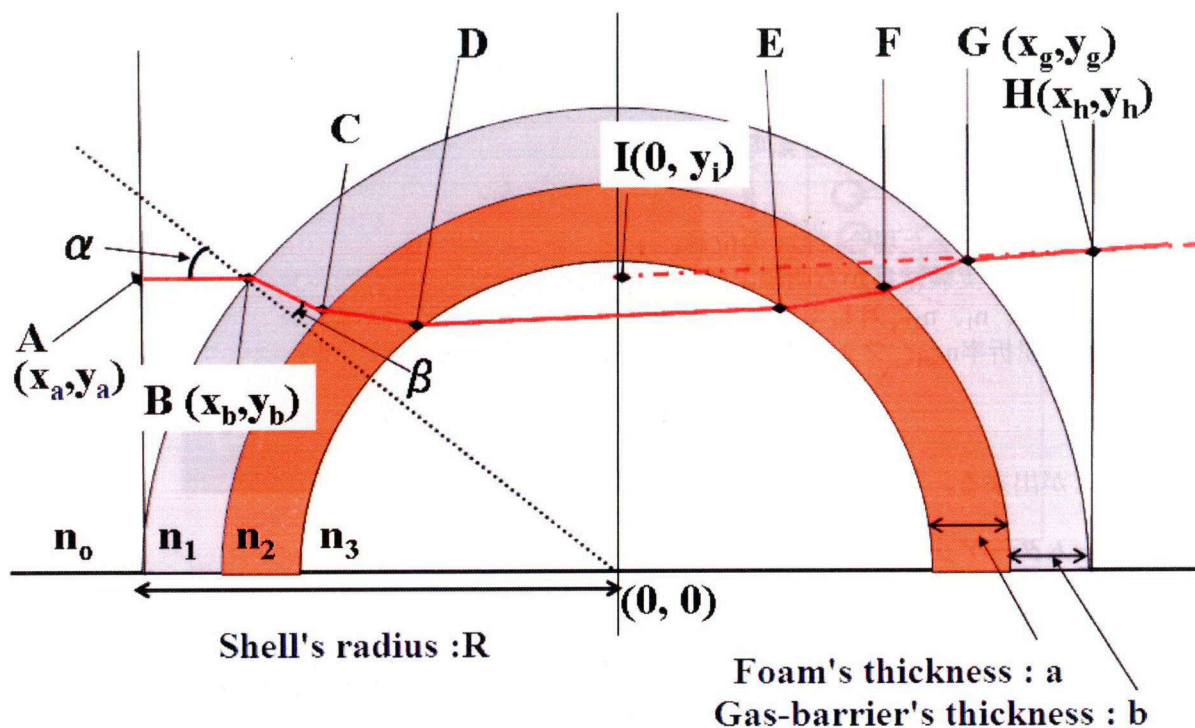
図6-1 二重シェル内部を透過する光線の光路を示すモデル図。
