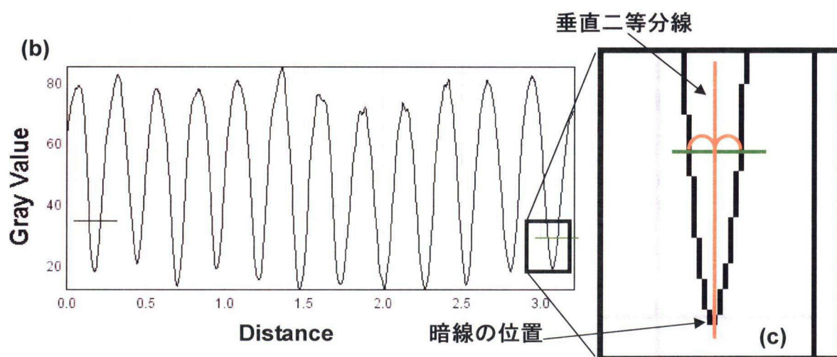
図4-16 フォームの入っていないウェッジに液体水素を充填したものも黄色( \lambda=594.1\text{nm} )のレーザーを用いた場合の干渉像(a)。図(a)中の四角に囲んだ部分の濃淡を数値化したもの(b)。谷(山)の中腹で値が同じ二点の中心を暗線(明線)の位置とした(c)。
