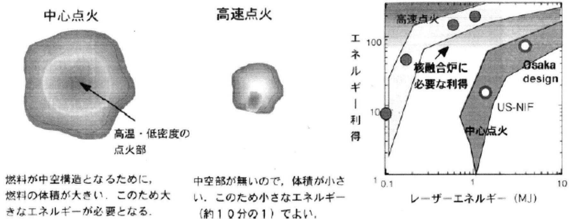
図1-3 中心点火と高速点火の燃料構造の違い。高速点火方式では同程度のエネルギー利得を得るために必要なレーザーのエネルギーが中心点火に比べて一桁小さい。ここで実際の商業炉を考えた場合にはエネルギー利得は100以上が必要とされる。
