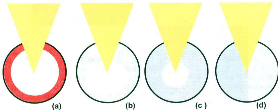
図 5-15 ターゲットに液体水素が入っていくときの水素の状況の干渉計測を行った方向の模式図。(a)は何も入っていない状態、(b)はフォーム層内全てに液体水素が充填され、さらに過量の液体水素によりコーン周辺にメニスカスが出来た状態、(c)はさらに液体の流入が進行しフォームシェルに半分程度入った状態、(d)はフォームシェル全てに液体水素が満たされた状態。
