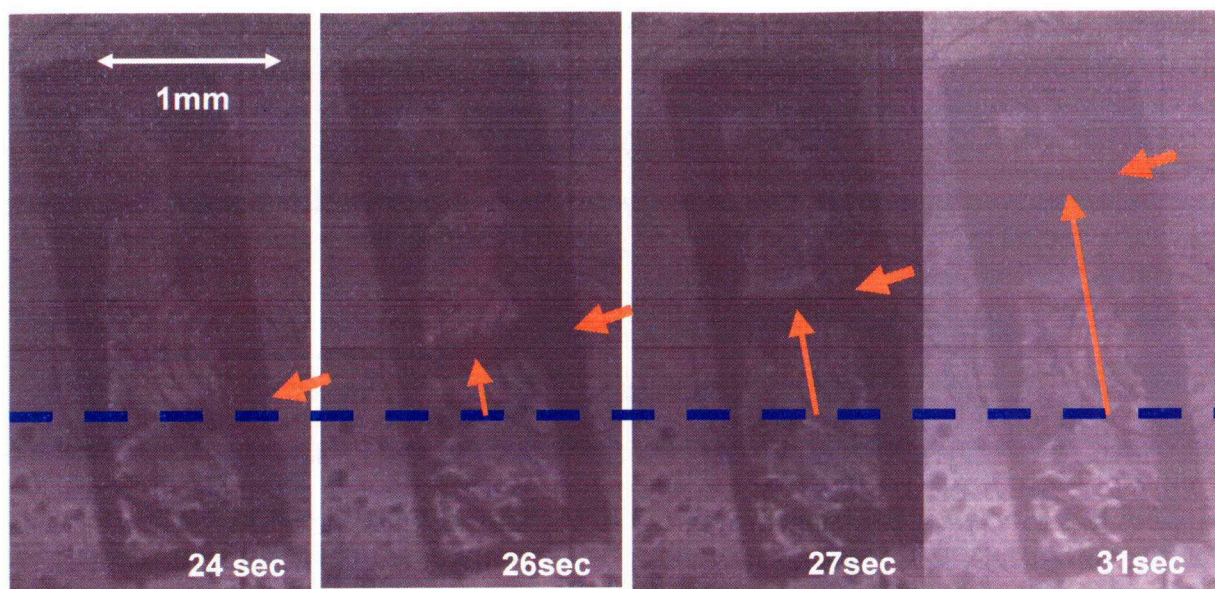
図 4－6 フォーム平板に液体重水素が浸透していく様子を観察した写真。時間の経過と共に気液界面と思われる黒い領域が画面上方に動いていく。
