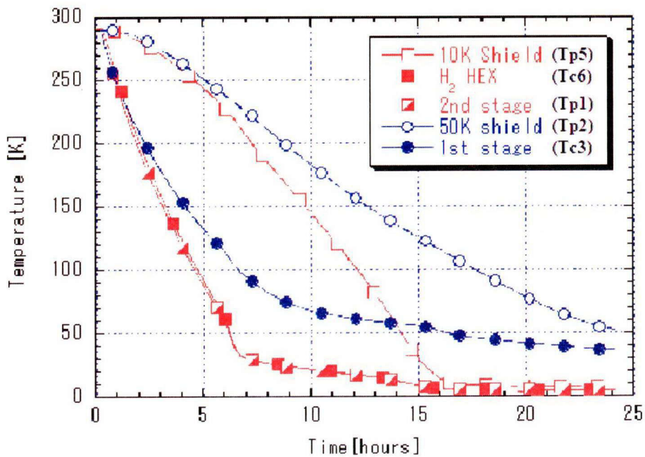
図 4-1-2 冷却装置におけるそれぞれの位置の冷却曲線。10K シールドと H 2 HEX が 10K 前後になると実験を開始できる。
