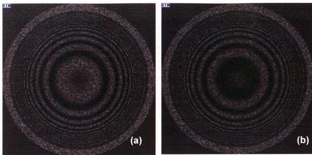
図 3－8 直径 500mm、RF フォーム 100mg/cc が 20mm、蒸発防止膜 5mm のターゲットの干渉図。 (a)は内部が真空、(b)は内部に六フッ化硫黄ガスが 0.1 MPa 充填されている。Shell optic model (Lebedev Physical Institute,Moscow) 3) を用いて計算した。
