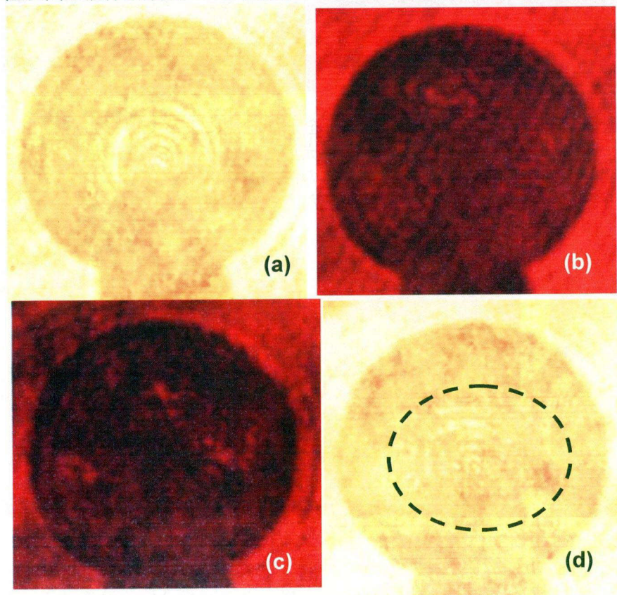
図5-16 固体水素形成実験における干渉像。水素充填前の干渉像(a)、とレーザーを照射せずに固化させた場合の干渉像(b)、(c)及び(d)はレーザーを照射したまま固化させた場合の干渉像。
