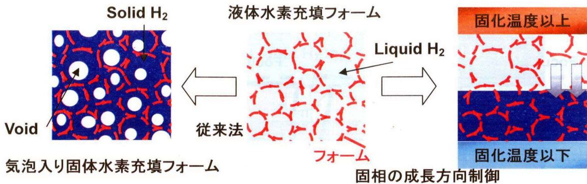
図4－5 全体を急速に固化させた場合では固化した際に各セル内で固相への転位が完結し、フォーム内に気泡が残ってしまう。温度勾配をつけ、一方向から固化を進行させることで常に固化面は液面と接しており、燃料の流入が生じる。
