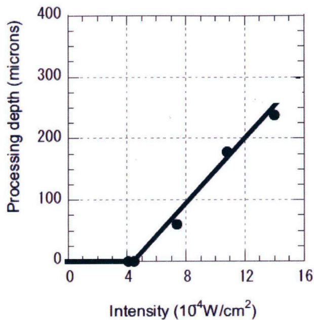
図 2-7 RF フォーム平板( 168 \text{ mg/cm}^3 )のレーザー加工において、レーザー強度と加工深さの関係。直線は線形な関係であることを見やすくするための補助線。 3.6 \times 10^4 \text{ W/cm}^2 以上の強度であれば加工痕は観察できた。
