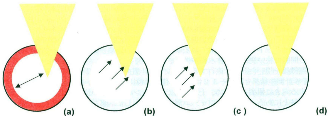
図 5-13 ターゲットに液体水素が入っていくときの水素の状況の模式図。(a)は何も入っていない状態。両矢印はコーンとシェル壁が最も遠いと考えられる位置。(b)はフォーム層内全てに液体水素が充填され、さらに過量の液体水素によりコーン周辺にメニスカスが出来た状態、(c)はさらに液体の流入が進行しフォームシェルに半分程度入った状態、(d)はフォームシェル全てに液体水素が満たされた状態。図中の片矢印は液体の界面が視認できる場所を示す。
