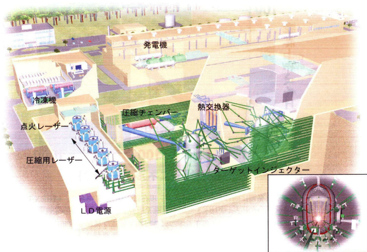
図 1 - 6 高速点火レーザー核融合発電所 (KOYO-Fast) の鳥瞰図
