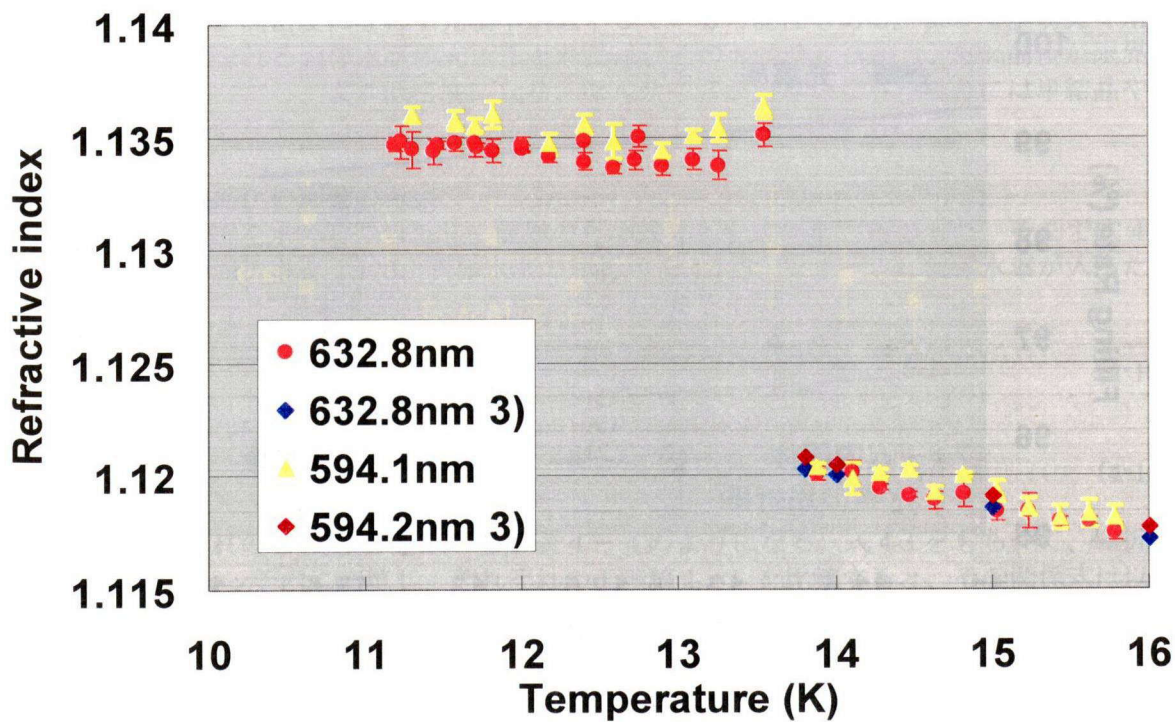
図4-2-2 フォーム内に含まれる水素の屈折率の温度依存性。(測定原理からフォームの屈折率は相殺されている。) 青色の菱形、茶色の菱形は参考文献 3) よりもとめた理論上の液体水素の屈折率。
