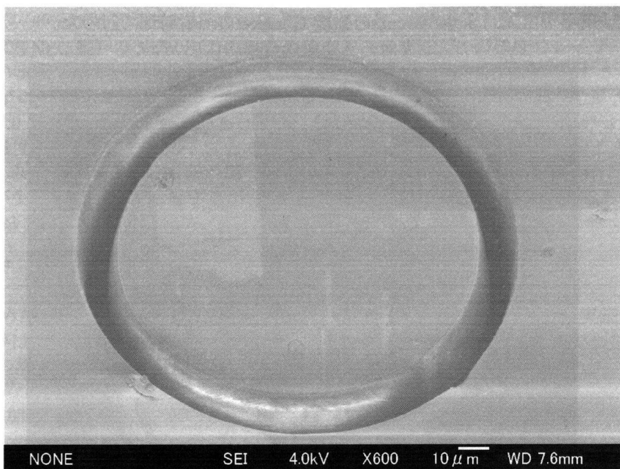
図 2-5 RF フォーム平板に対して円形にレーザー加工した加工痕の SEM 画像
