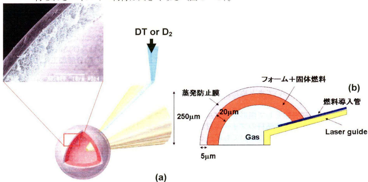
図 1-9 FIREX-I 計画用ターゲットの模式図(a)。FIREX-I 計画用フォームクライオターゲットの寸法を表記した断面の模式図(b)
