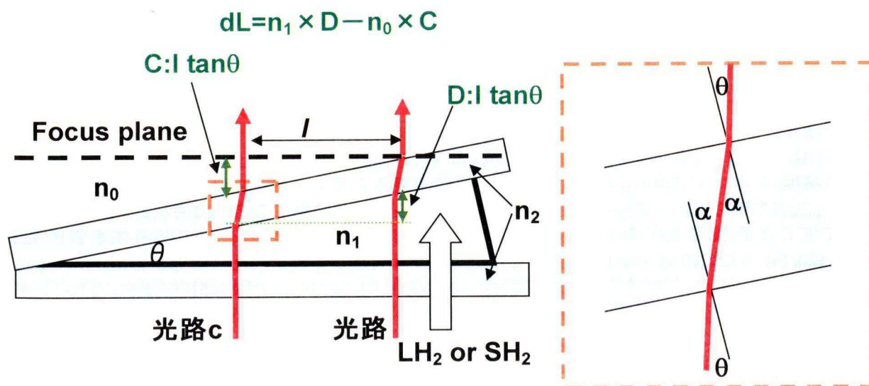
図4-2 ウェッジ型サンプルの断面の概略図。簡単のため \theta = \beta と仮定する。
