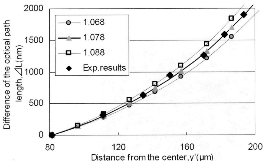
図6-4 RFフォームの屈折率の測定結果と計算により求めた屈折率の比較。
