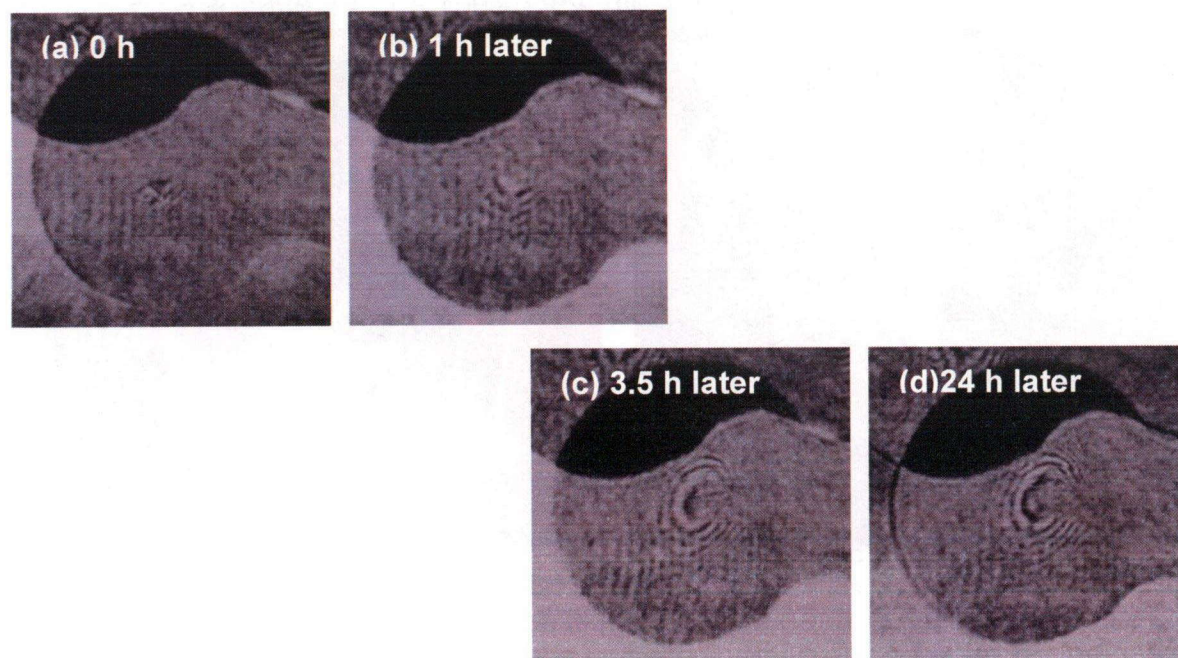
図 5-11 燃料を固化させた後の RF フォームターゲットの干渉模様の写真。(a)固化直後、(b)1 時間経過後、(c)3.5 時間経過後、(d)24 時間経過後。
