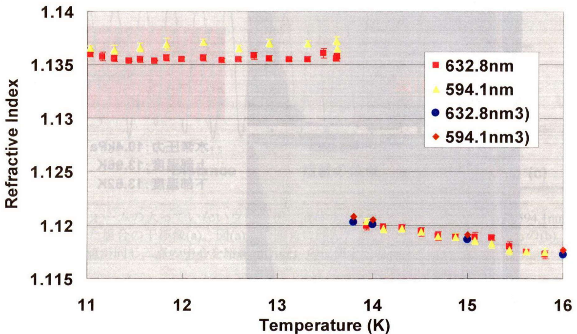
図4－19 二つの波長 632.8nm と、594.1nm の液体及び固体水素の屈折率を示す。青丸及び茶菱形は参考文献3)より求めた理論上の液体水素の屈折率である。
