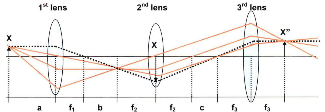
図4-14 計測装置の干渉計測に用いられるイメージレンズシステムの光路図。下のアルファベットはそれぞれの間隔を表す。また f_1 、 f_2 、 f_3 はそれぞれ1st、2nd、3rd レンズの焦点距離である。X、X'、X''はそれぞれその位置における大きさを示す。また物質像を直線で、参照光を点線にて表す。
