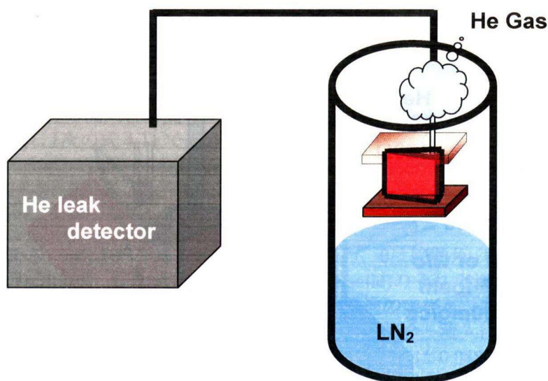
図4-8 液体窒素温度でのリーク試験方法の概略図。
