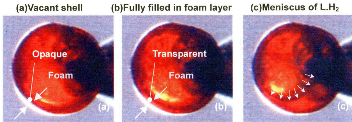
図 5-8 RF シェルターゲットに模擬燃料を充填していく様子。(a)空の状態から、(b)液化が進みフォーム層に充填され、(c)コーン付近にメニスカスができた、各写真。
