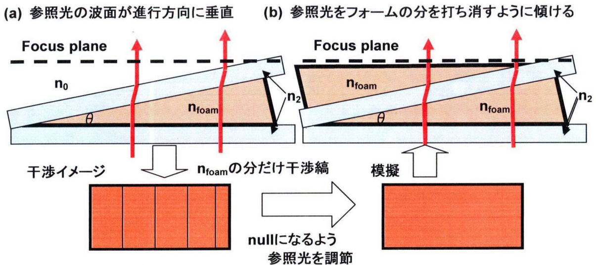
図4-4 フォーム入りウェッジのフォーム内に充填した物質の屈折率の測定方法。(a)フォームが存在する分干渉縞が発生する。(b) null にすることでフォームによる位相差は打ち消され、ウェッジの透過側に同じフォームが存在する状態と同じ効果がある。
