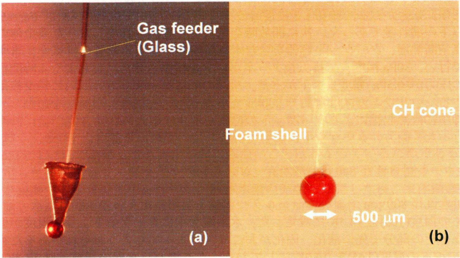
図 5-4 パリレンコーン付き直径 500 \mu\text{m} のフォームシェルターゲットの全体図(a) とフォームターゲット部分の拡大写真(b)。
