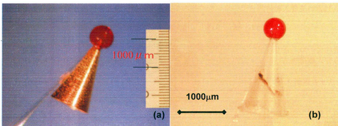
図 3-7 高速点火レーザー核融合用ターゲットの外形上の完成図。金をコーンに用いた場合(a)と、パラキシリレンをコーンに用いた場合(b)の写真。
