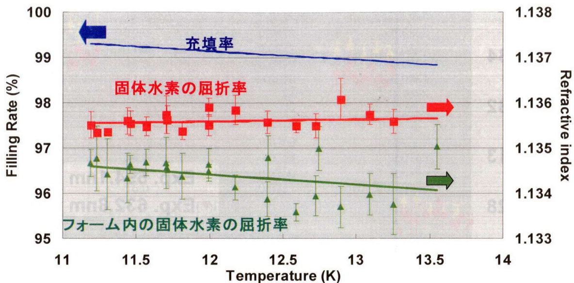
図4-23 赤色レーザーの結果を用いて RF フォーム内の固体水素の充填率を評価した。青色直線が充填率のグラフであり、左側の軸の値を取る。赤色四角は固体水素の屈折率であり、その最小二乗法による直線が赤色の線である。フォーム内の固体水素の屈折率は緑三角で表現しており、この最小二乗法による直線が緑色線である。固体水素の屈折率およびフォーム内の固体水素の屈折率は右側の軸の値をとる。
