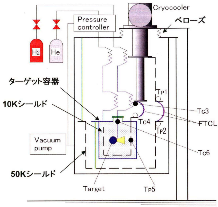
図 4-1-1 冷却装置の概略図。温度センサーの位置関係と、水素ガスとヘリウムガスの流路を示す。
