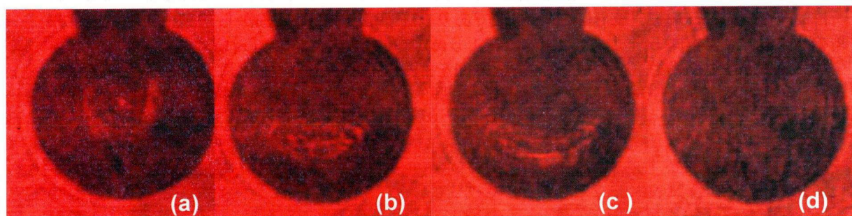
図 5-14 液体水素が入っていく様子を干渉計測によって撮影した。(a)は何も入っていない状態、(b)はフォーム層内全てに液体水素が充填され、さらに過量の液体水素によりコーン周辺にメニスカスが出来た状態、(c)はさらに液体の流入が進行しフォームシェルに半分程度入った状態、(d)はフォームシェル全てに液体水素が満たされた状態。
