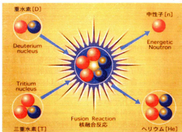
図1-1 核融合反応では、反応前の結合エネルギーと反応後の物質の結合エネルギーの差が核融合エネルギーとしてとりだされる。重水素と三重水素の DT 燃料が最も核融合反応断面積が大きい（右）、燃料として用いられる。
