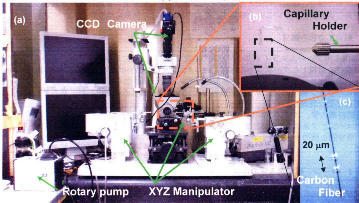
図3-2 ターゲット組み立て用装置。マニピュレータは手前に2台と奥から手前に向けて動作するものが1台。手元を照らす照明などがある(a)。キャピラリーホルダーにカーボンファイバー付きのガラス管を接続した写真。接着剤を塗りたい角度にガラス管を曲げて使用する(b)。カーボンファイバーに接着剤の水滴が付着している写真(c)。
