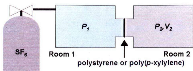
図 3-9 透過率測定用装置の概略図。Room1 には六フッ化硫黄(SF 6 )ガスのボンベが接続してあり、Room1 と Room2 には圧力計が備え付けられている。
