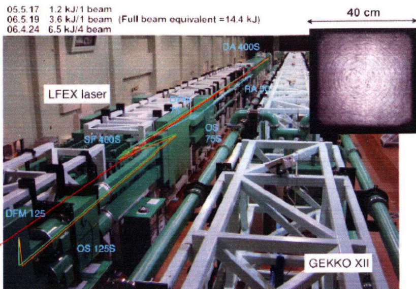
図 1 - 5 極端パルス高強度レーザーの技術推進に伴い建設された LFEX レーザーと GEKKO XII 号。FIREX-I 計画では GEKKO XII 号を用いて燃料ターゲットを爆縮し、LFEX によって加熱する。
