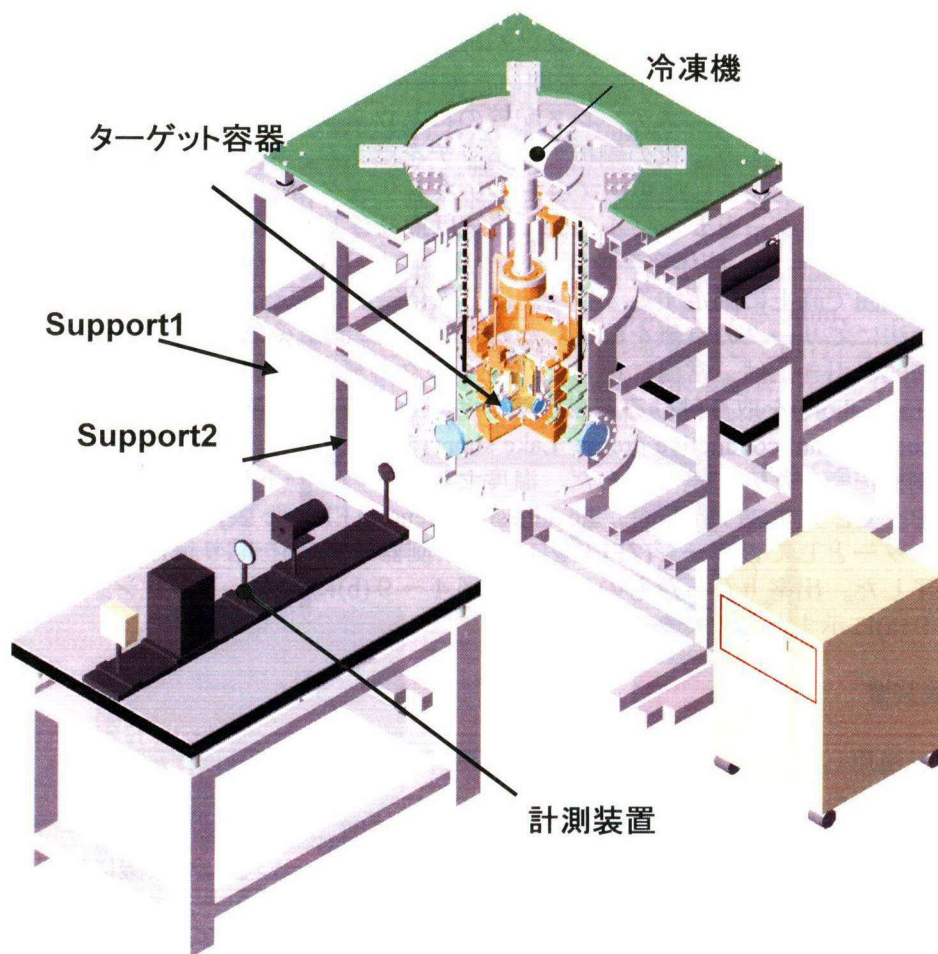
図4-10 冷却装置の全体像の模式図。
