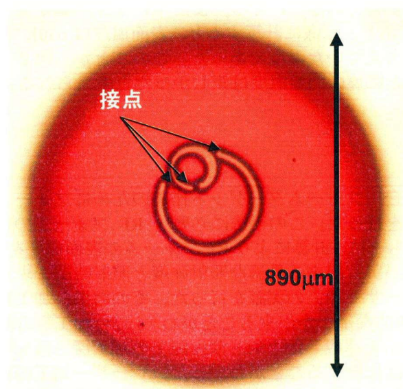
図 2-8 RF フォーム球に対してレーザー加工したものを顕微鏡で拡大した図。
