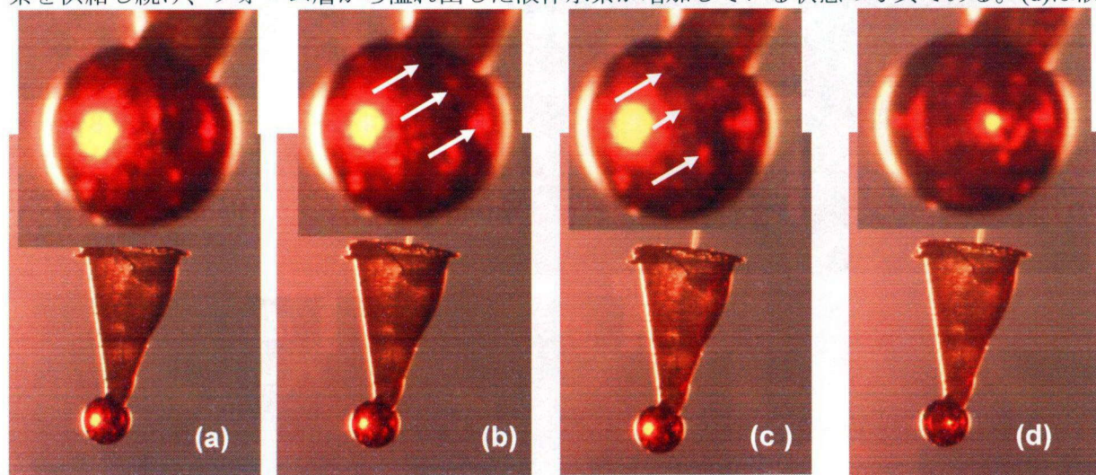
図5－12 液体水素が入っていく様子を実体顕微鏡を用いて撮影した写真。(a)は何も入っていない状態、(b)はフォーム内にはすべて液体水素が充填され、さらに過量の液体水素によりコーン周辺にメニスカスが出来た状態、(c)はさらに液体の流入が進行しフォームシェルに半分程度入った状態、(d)はフォーム層から溢れ出した液体水素がフォームシェル全てに満たされた状態。図中の矢印は液体の界面が視認できる場所を示す。
