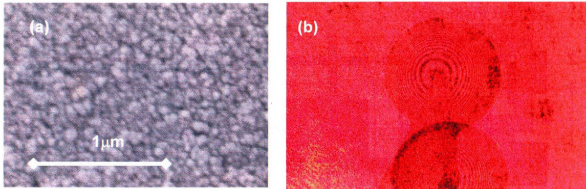
図 3-6 RF フォームの平板にパリレンをコーティングした表面の電子顕微鏡写真(a)。パリレンコーティング後の干渉写真(b)。
