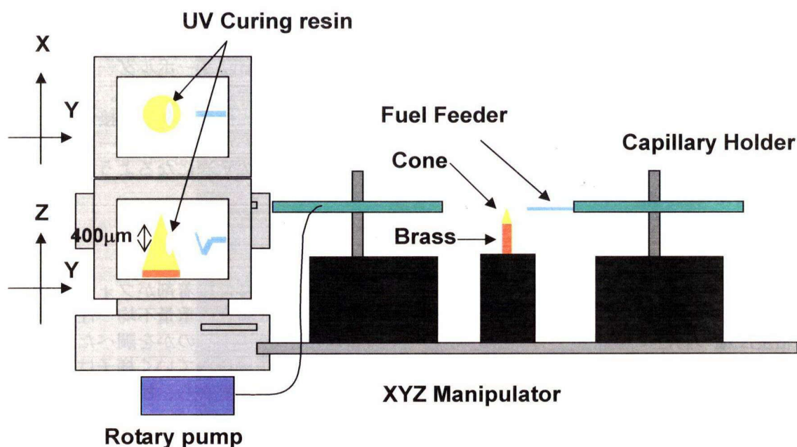
図 3-4 コーンと燃料導入管を接続する様子の概念図。コーンと燃料導入管をつなげる接着剤はコーンの先端より 400μm よりも下側に塗布した。
