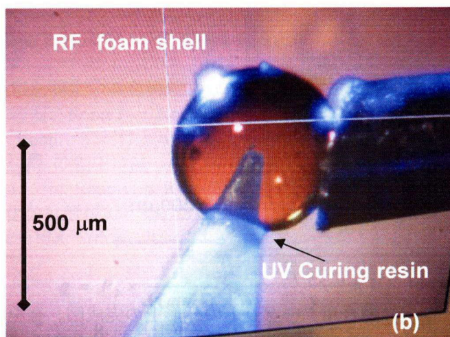
図3-5 フォームシェルと燃料導入管+コーンを接続する概念図(a)。紫外線硬化樹脂に紫外線をあて硬化させている写真(b)。
