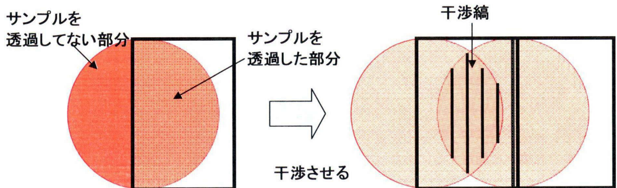
図4-15 シェアリング干渉計のイメージ図。レーザー光をサンプルの端が中央になるように調節し、ハーフミラーで分けたのち、サンプルを透過した部分と透過していない部分を干渉させる。
