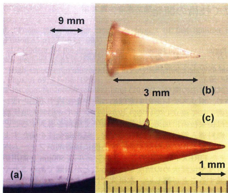
図3-1 ガラス製燃料導入管(a)とパリエン製コーン(b)の写真。(c)は金製コーンの写真。金製コーンには厚さ等の測定をするためにガラス管を接着している。
