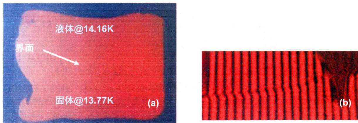
図4-20 ウェッジ型の中にフォームをいれ、液体水素を充填した後に温度差による固相の成長制御を実行し界面が下部から上部へと移動している時の実体顕微鏡写真(a)。そのときの干渉像(b)。
