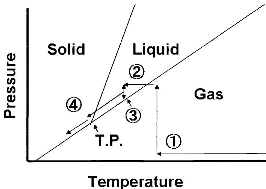
図5-6 金コーン付き直径 800 \mu m のフォームシェルターゲットを用いた燃料充填、固化実験におけるターゲット内部の温度と圧力の変化の模式図。①10K シールドの温度を 14.0K まで下げ、水素ガスを加圧する。②温度を下げ、気体から液体へ変化させる。③セル内の蒸気圧を調節することでフォームに充填された液体水素量を調節する。④温度を下げていき、固化させる。温度とともに蒸気圧は下がる。温度を維持し、光学計測を行った。この図で T.P はパラ水素の三重点 (13.8K, 8kPa) を示す。
