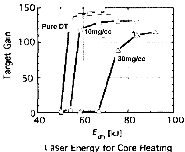
図 1-8 フォームの密度を変化させて、追加熱レーザーの強度とエネルギー利得の関係を計算により求めたもの。横軸に追加熱レーザーの強度をとり、縦軸にエネルギー利得(核融合エネルギー/レーザーエネルギー)をとった。利得 100 を達成するためには 10\text{mg/cc} の低密度フォームの開発が必要となる。Eulerian hydrodynamic code を用いて計算したもの。
