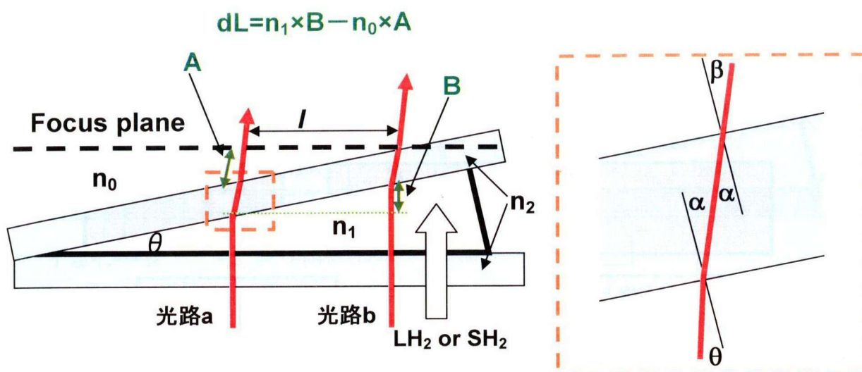
図4-1 ウェッジ型サンプルの断面の概略図。レーザーの光路と入射角と屈折角を示す。
