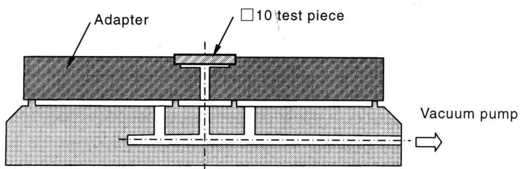
Fig. 6-4 \square 10 mm 試料固定部
