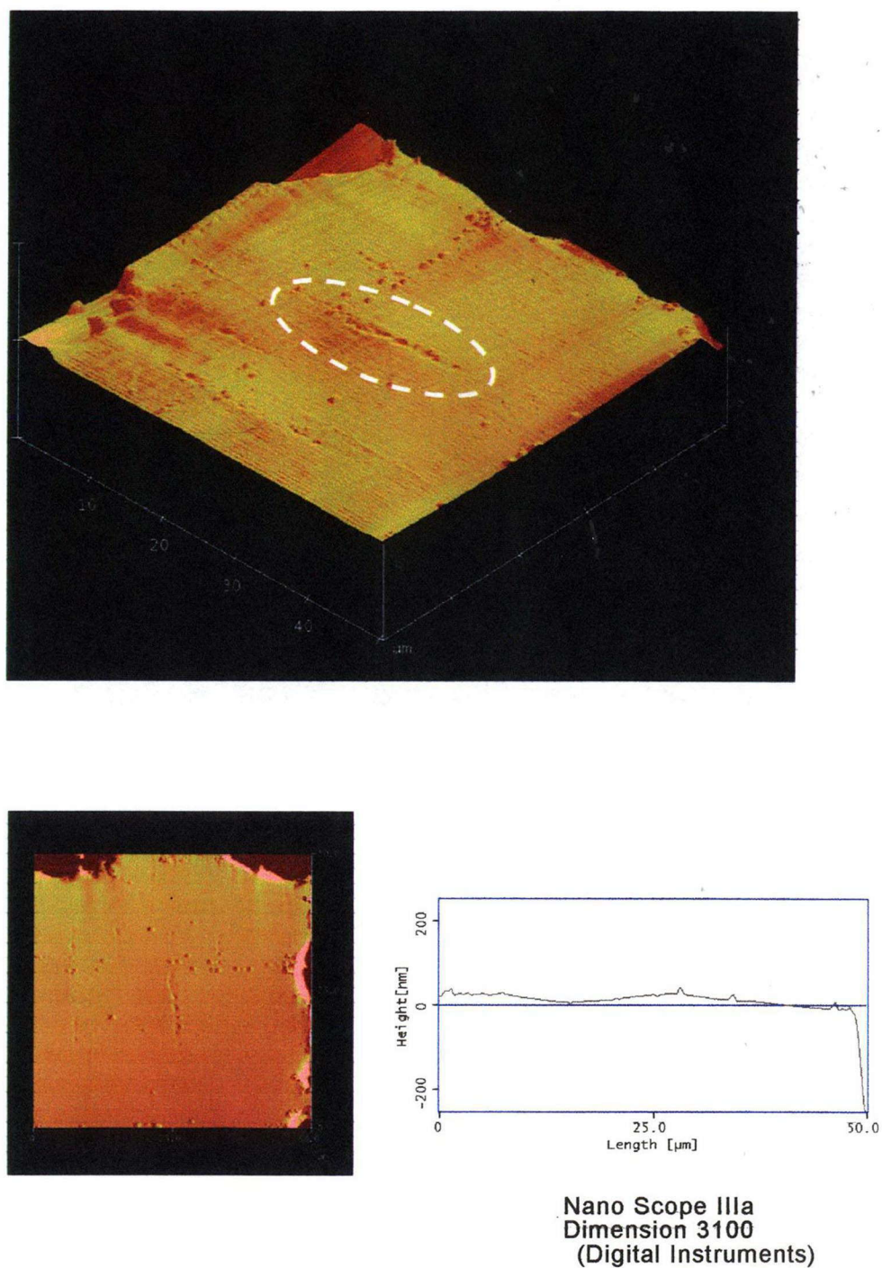
図 6-6 (f) レーザ微粒子集積痕のポリシング実験 (T= 9 min)
