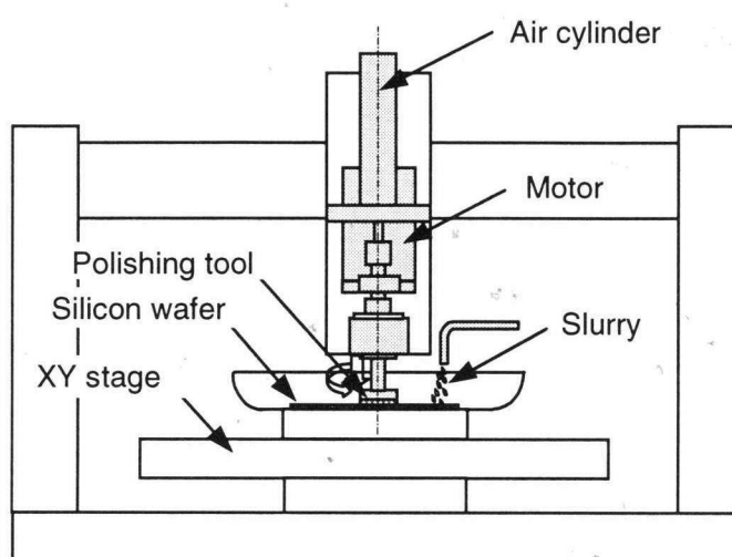
Fig. 6-1 ポリッシング実験装置概要
