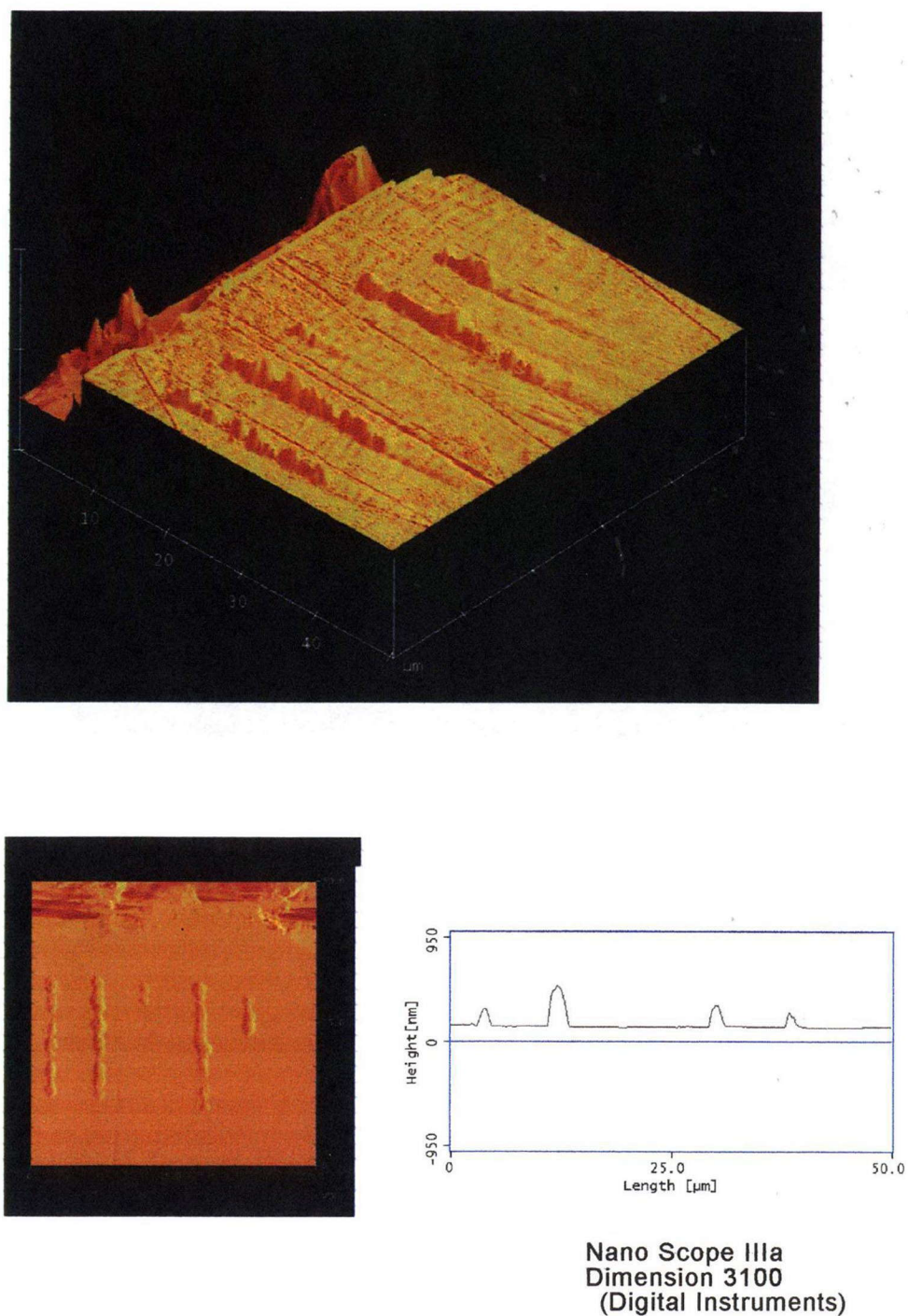
図 6-6 (d) レーザ微粒子集積痕のポリシング実験 (T= 3 min)
