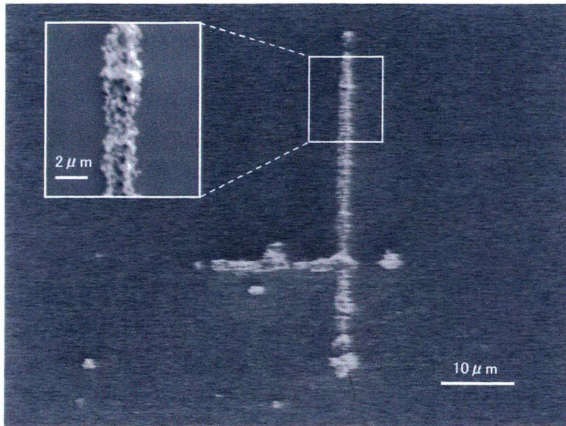
Fig. 5-5 シリコンウェハ表面に形成されたレーザ集積痕(SEM)
