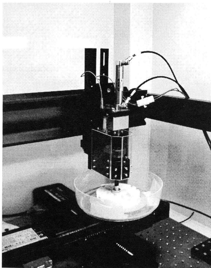
Fig. 6-2 ポリッシング実験装置写真
