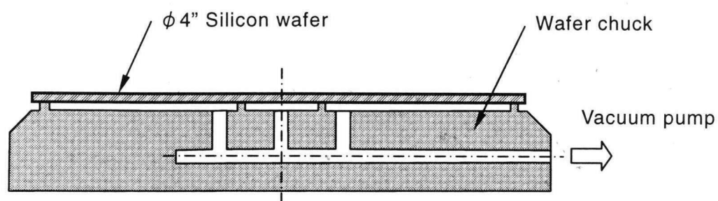
Fig. 6-3 \phi 4 インチシリコンウェハ固定部
