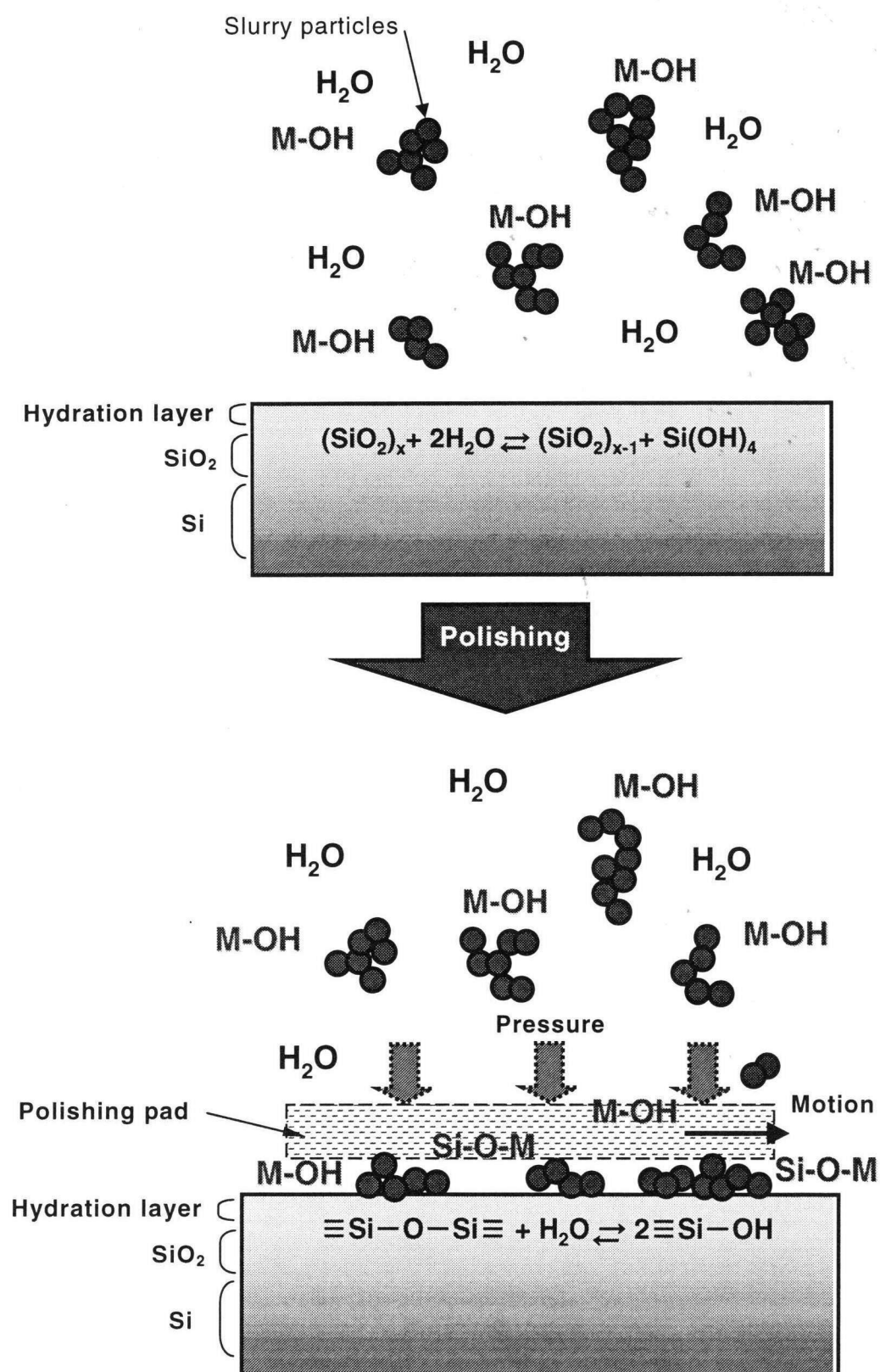
Fig. 2-4 ポリッシングにおける \text{SiO}_2 の除去機構の模式図
