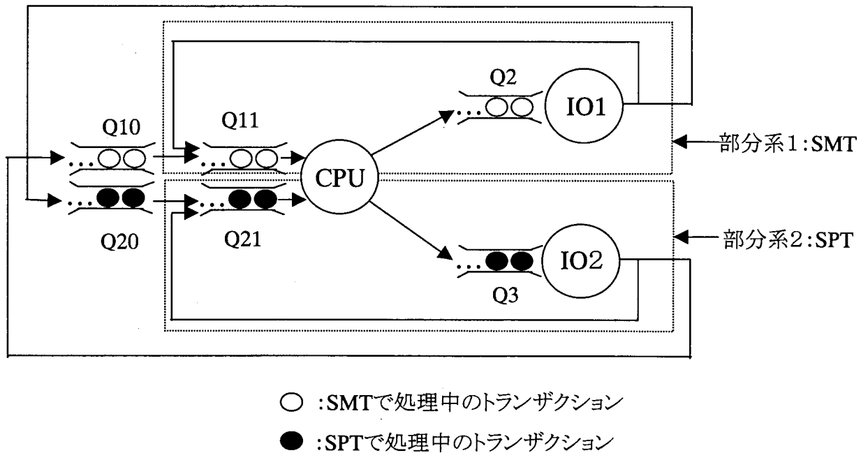
図5.4 トランザクション処理システムの待行列モデル
