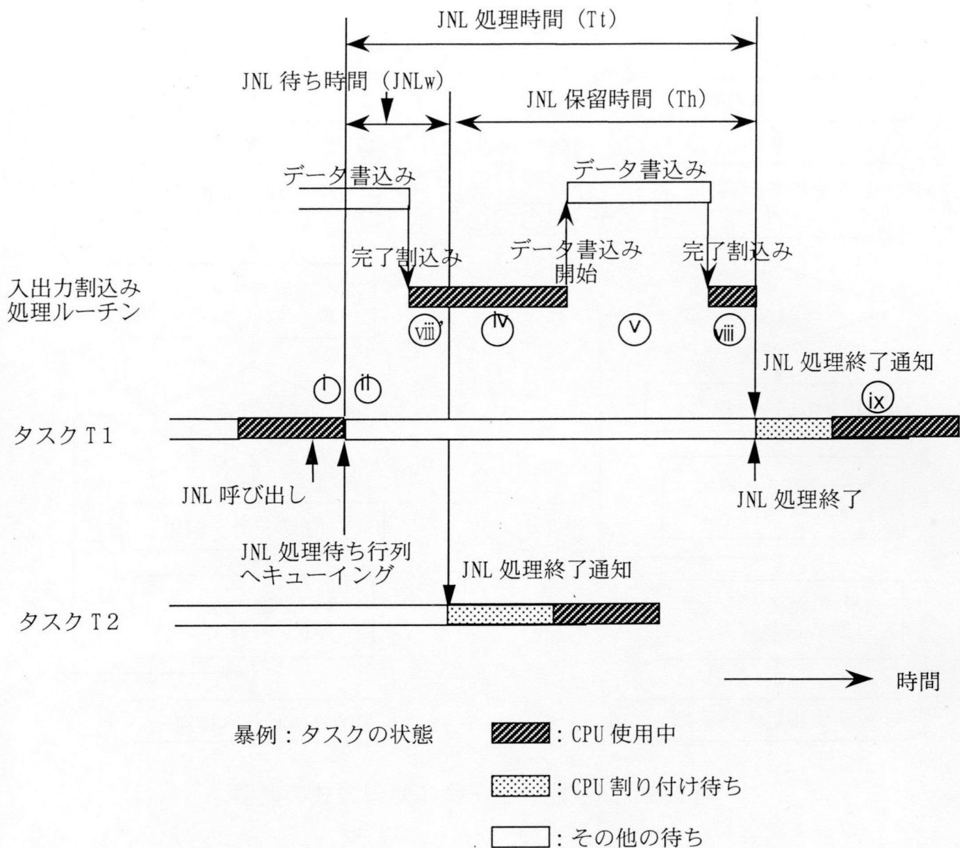
図 3.10 高性能ジャーナル処理ルーチンの動作
