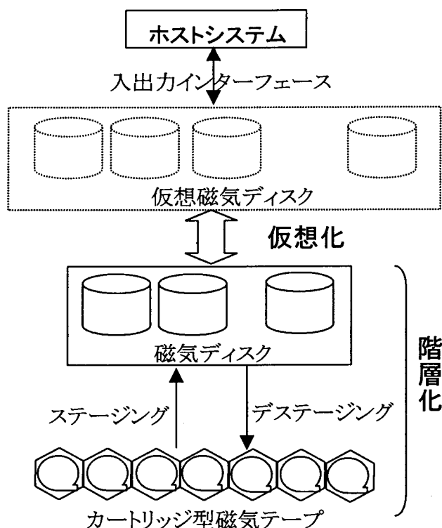
図 4.1 仮想ディスク方式の概念図
