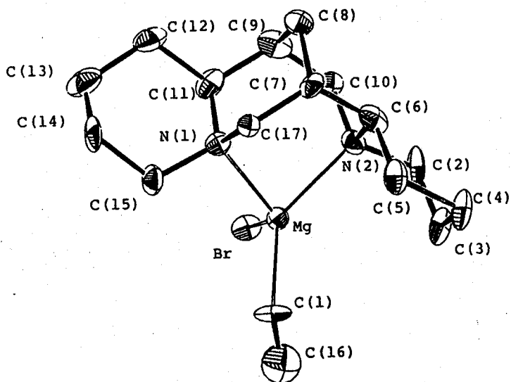
Figure 2. A perspective view(ORTEP II) of 4a
