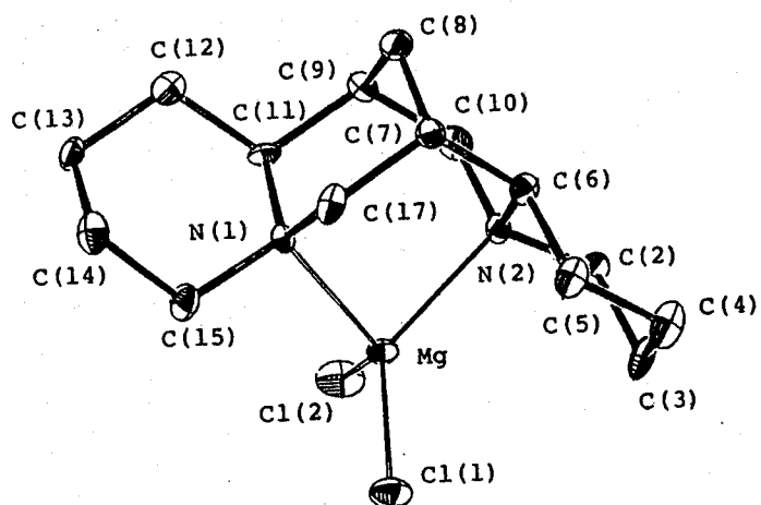
Figure 4. A perspective view(ORTEP II) of 4g'
