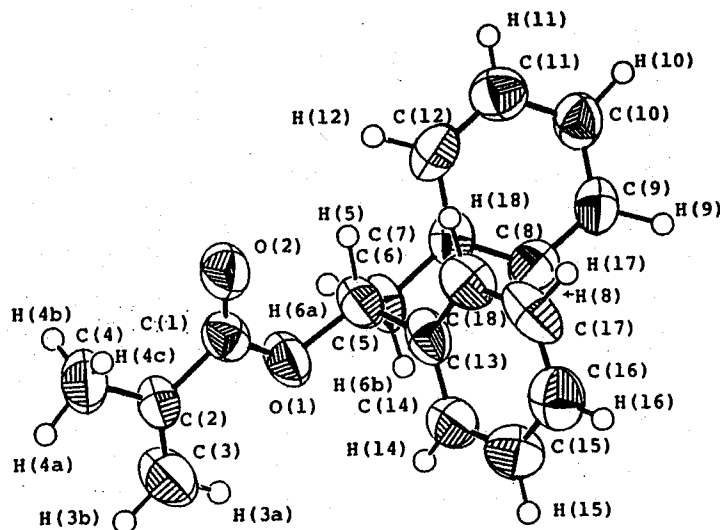
Figure 29. The molecular structure of DPMA-1,2 (ORTEP II)
