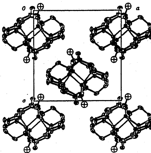
Figure 16. The crystal structure of 4a (ORTEP II)
