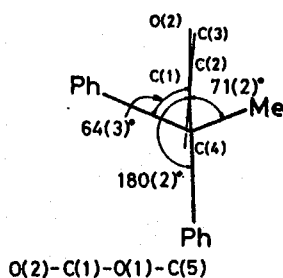
ChMA
