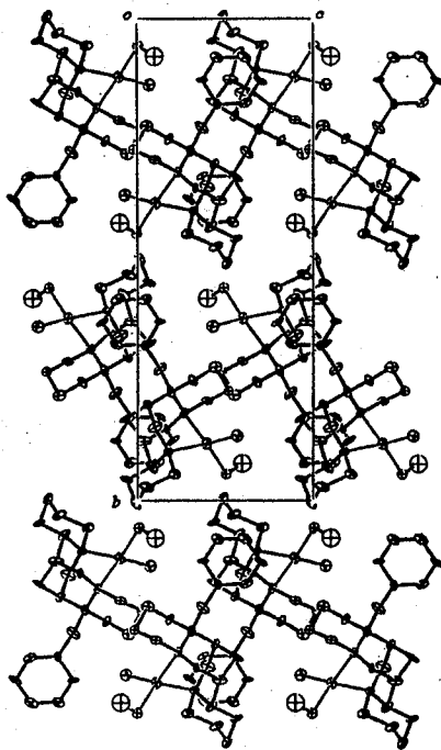
Figure 20. The crystal structure of 7 (ORTEP II)
