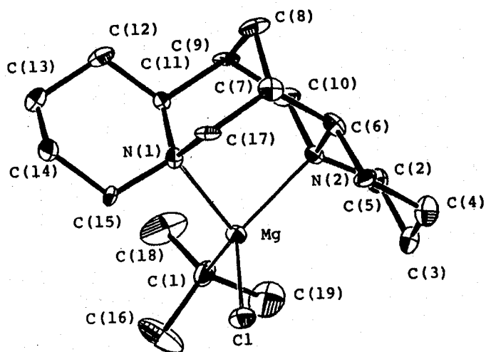
Figure 3. A perspective view(ORTEP II) of 4g
