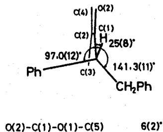
(R)-DPEMA-1,2
