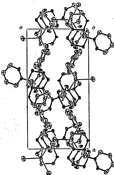
Figure 21. The crystal structure of 7' (ORTEP II)
