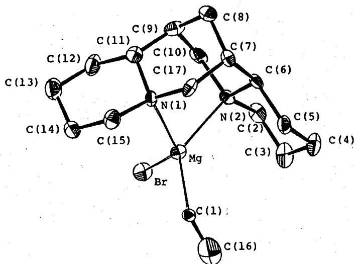
Figure 5. A perspective view(ORTEP II) of 5
