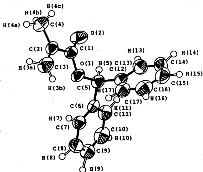
Figure 26. The molecular structure of DPMMA (ORTEP II)
