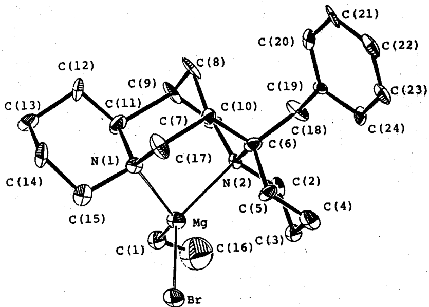
Figure 6. A perspective view(ORTEP II) of 7
