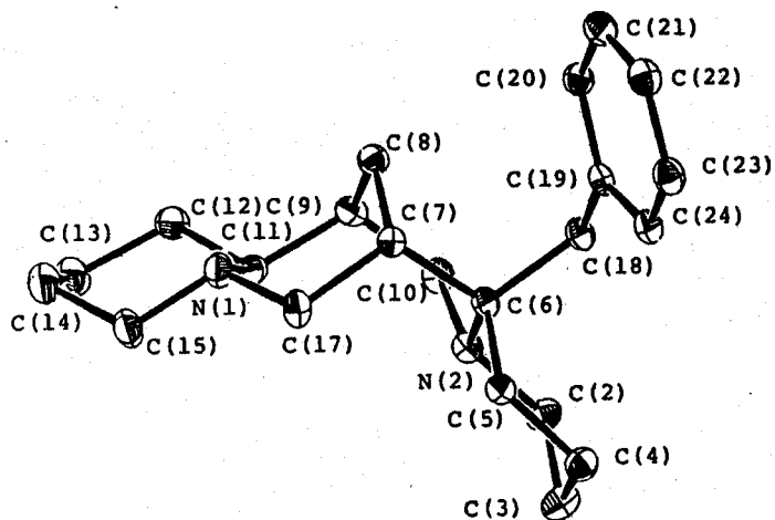
Figure 1. A perspective view(ORTEP II) of 2c
