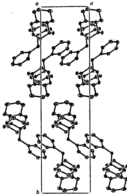
Figure 15. The crystal structure of 2c (ORTEP II)
