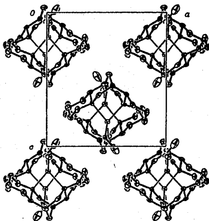
Figure 19. The crystal structure of 5 (ORTEP II)
