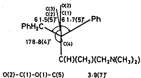
ChMA
