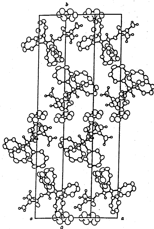
Figure 41. The crystal structure of TrBzMA (ORTEP II)
