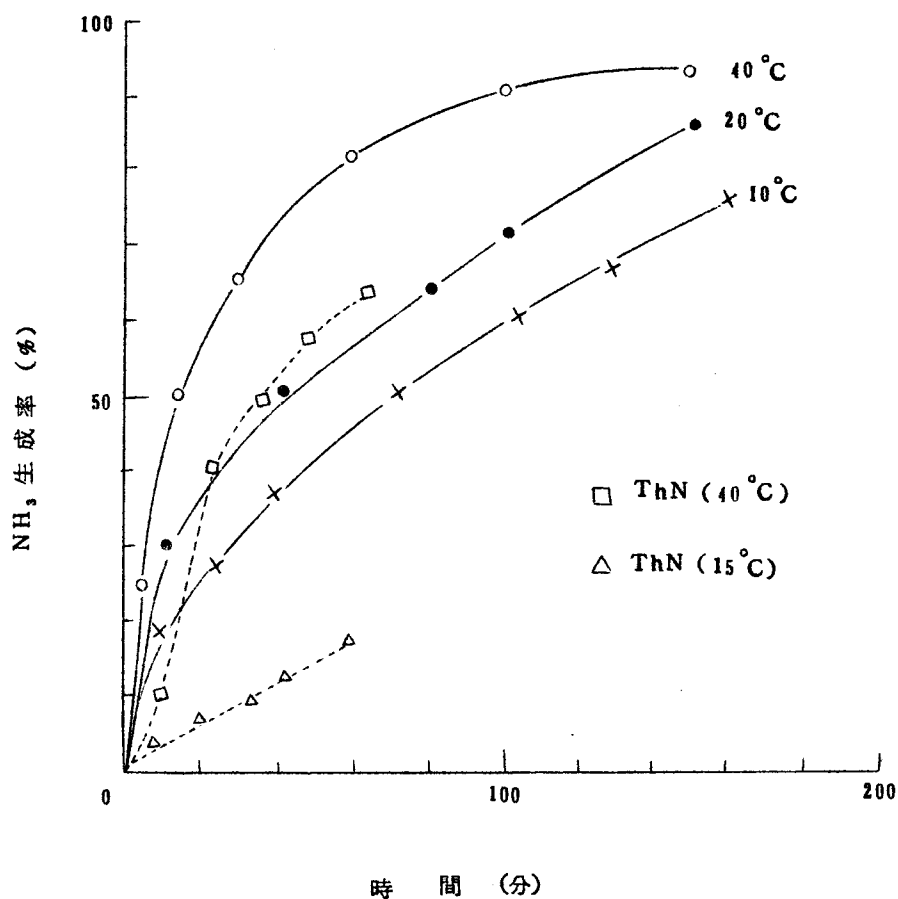
第35図 \text{ThC}_{0.42}\text{N}_{0.38} と \text{ThN} の加水分解
