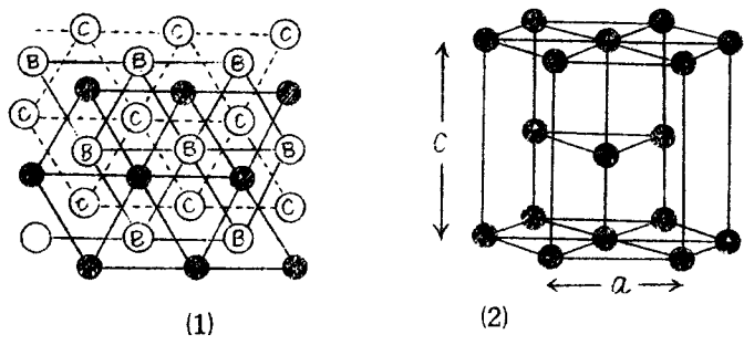
第41図 六方最密構造 (1) つみ重ね (2) 単位胞
