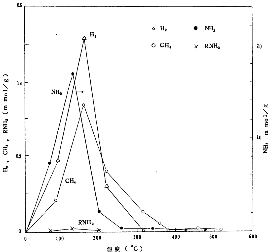
第22図 \text{ThC}_{0.11}\text{N}_{0.81} の加水分解
