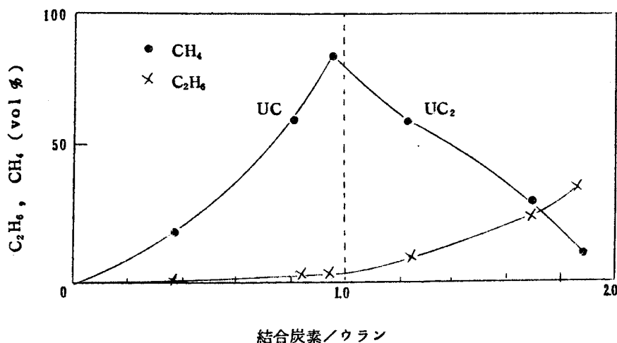
第43図 加水分解生成ガスの相による変化 (42)
