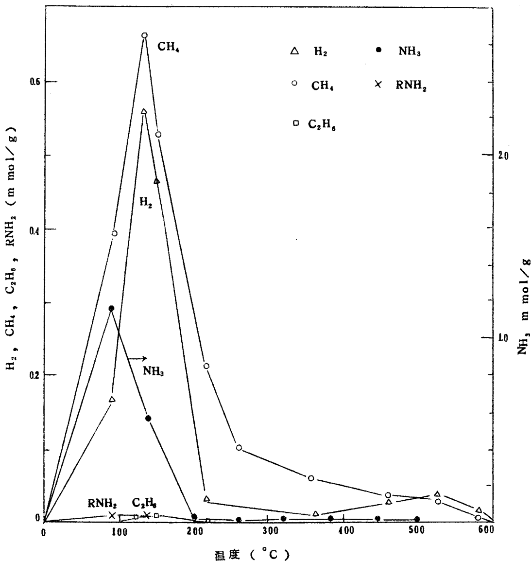
第23図 \text{ThC}_{0.53}\text{N}_{0.47} の加水分解
