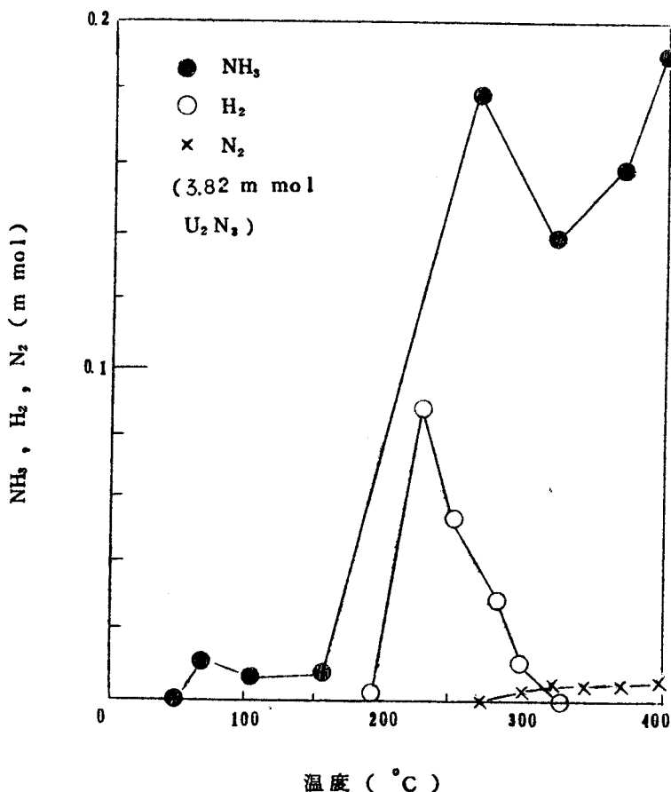
第6図 \text{U}_2\text{N}_3 の加水分解
