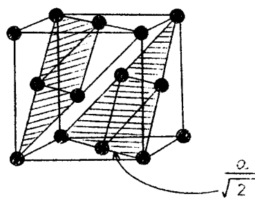
第42図 面心立方構造，最密(111)面
