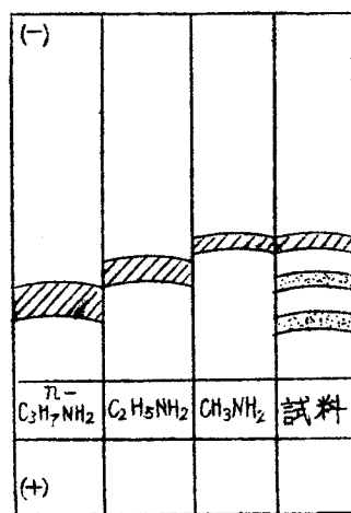
第12図 加水分解により生成したアミンと標準のアミンの通電ペーパークロマトグラフィ
