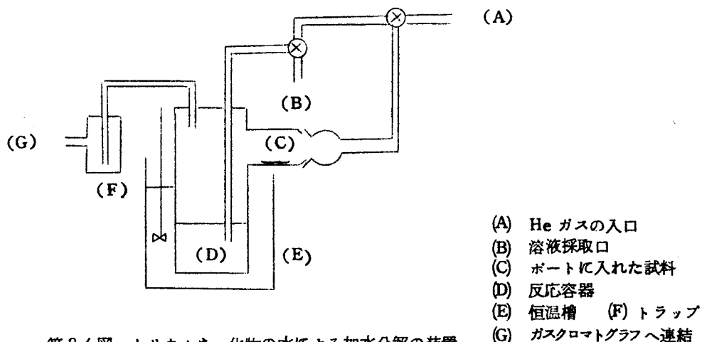
第26図 トリウムちっ化物の水による加水分解の装置
