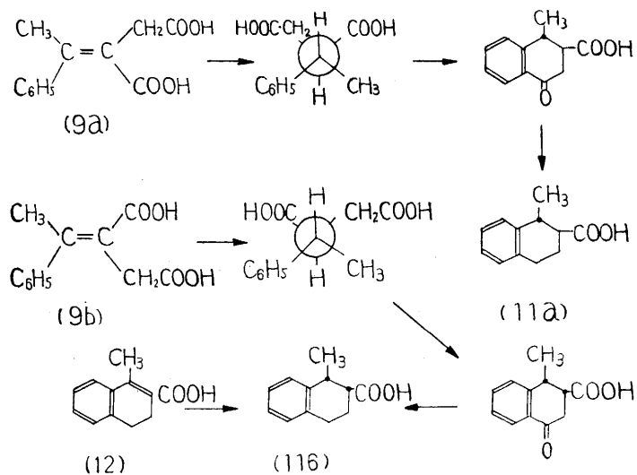
第三図 1.2.3.4-Tetrahydro-1-methyl-4-oxo-2-naphthoic Acid の立体異性体
