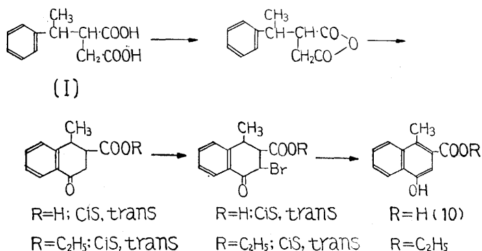
第二図 1.2.3.4-Tetrahydro-1-methyl-4-oxo-2-naphthoic Acid の合成
