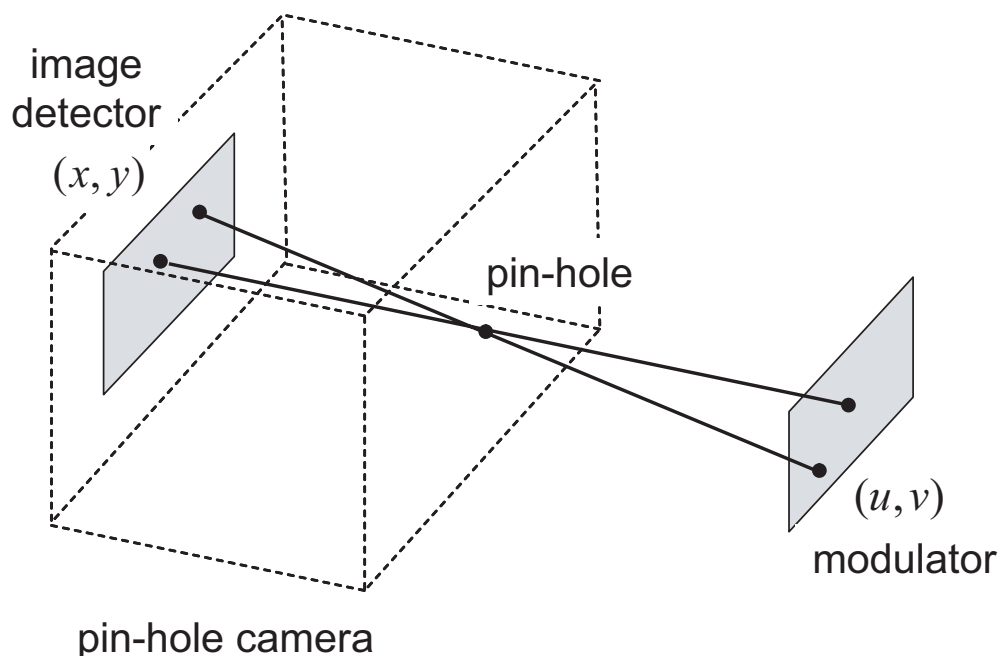
図 3.2: カメラと調光機器の位置関係
