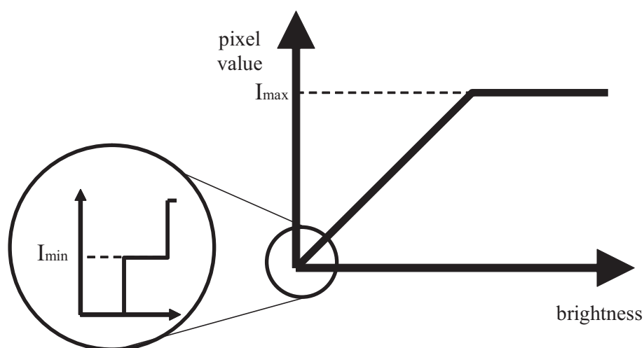
図 2.3: 受光特性の例
