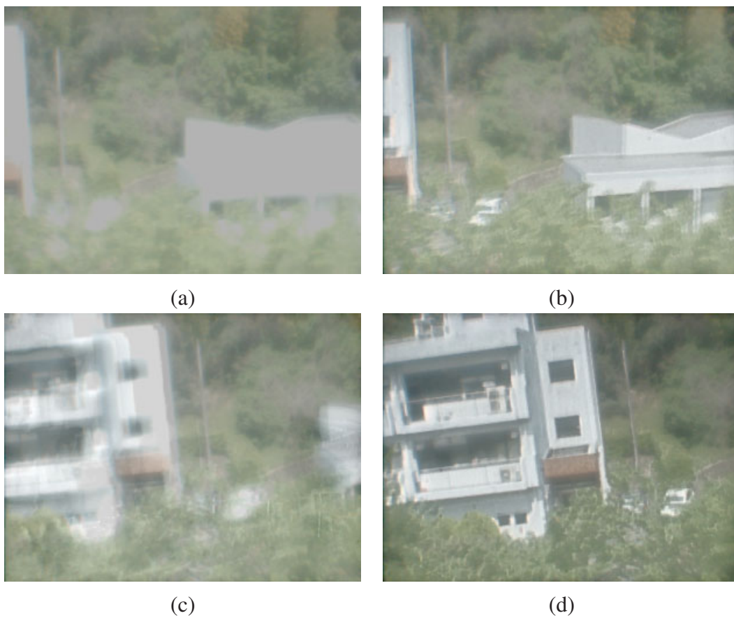
図 5.18: 動きのあるシーンの高ダイナミックレンジ画像
