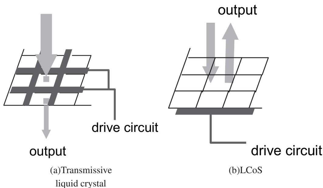
図 3.4: 液晶のモデル
