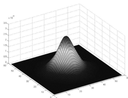
図 4.10: 広がり関数
