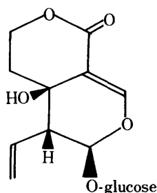
swertiamarin ( II )
