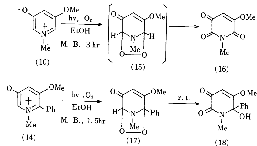
Scheme VI
