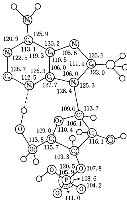
bond angles
