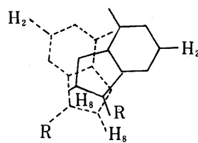
3'-syn, 5'-anti
