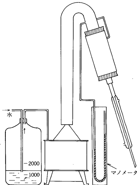
図27 通蒸気度補正装置
