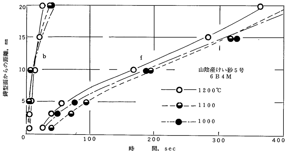
図10 水分凝縮層の移動 (ばく熱温度の影響)
