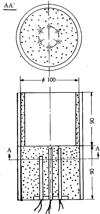
図51 試験鑄型（アルミニウム）
