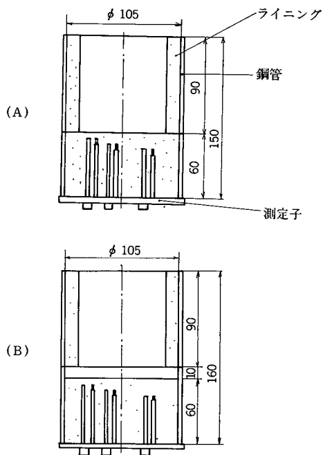
図36 試験鑄型
