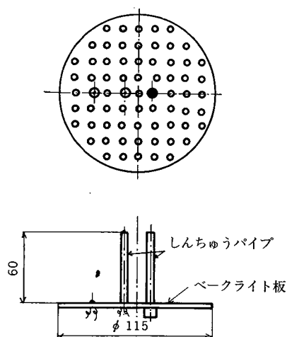
図35 測定子
