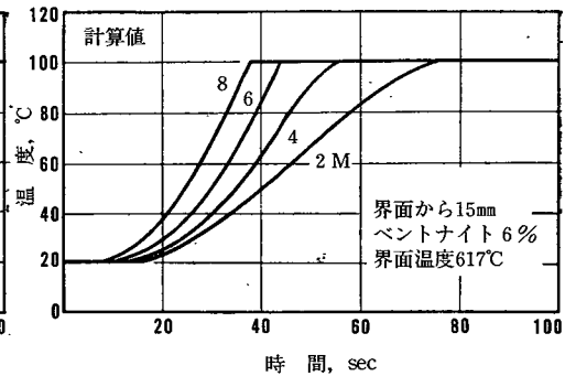
図61 凝縮域の温度分布 (水分率の変化)
