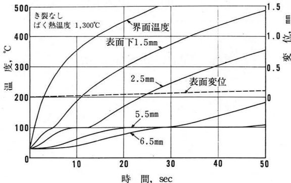
図79 試片内の温度変化（垂直方向）と変位
