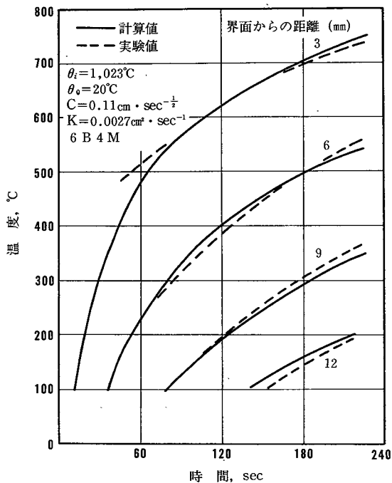
図53 乾燥域の温度分布 (鑄鉄)
