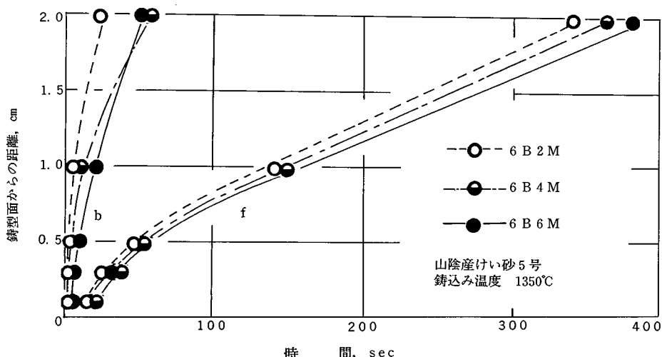
図13 水分凝縮層の移動(水分率の影響)
