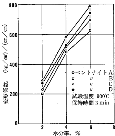
図94 高温の変形係数
