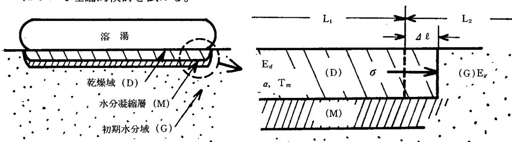
図96 すくわれ発生時の鑄型内の状態
