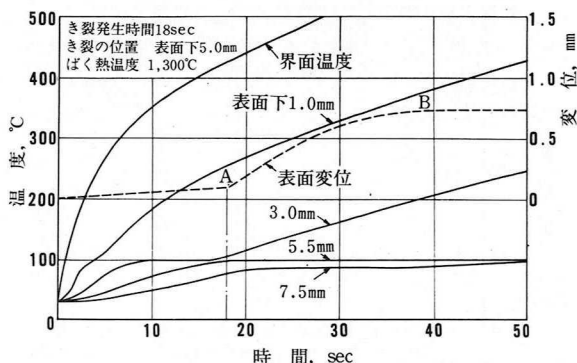
図78 試片内の温度変化（垂直方向）と変位
