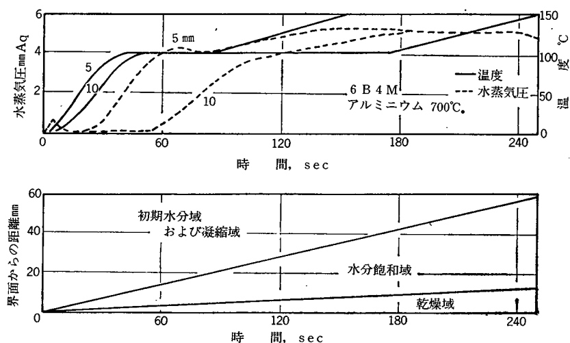
図9 水分凝縮層の移動状況
