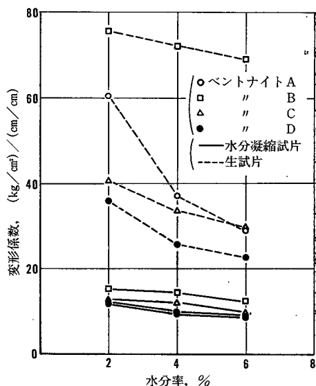
図92 湿態および水分凝縮層の変形係数
