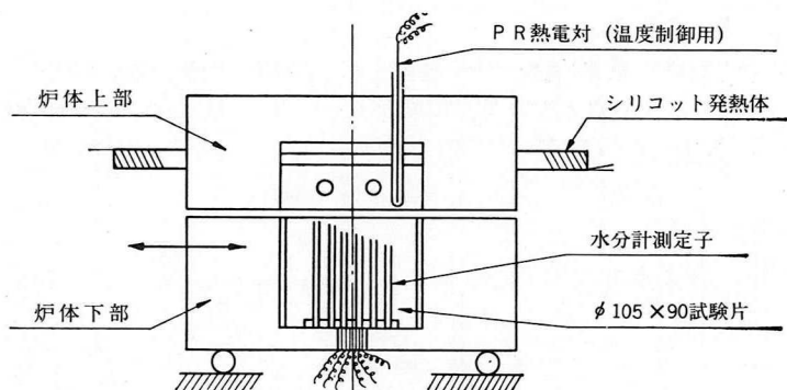
図4 シリコニット炉 (ばく熱用)
