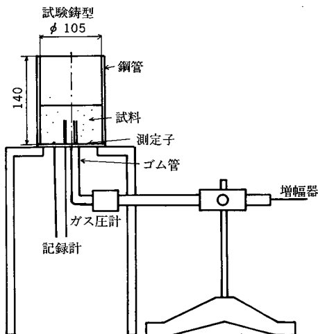
図34 実験装置
