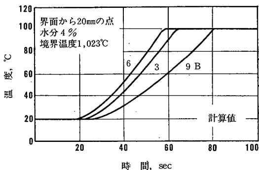
図59 凝縮域の温度分布 (ベントナイト量の変化)
