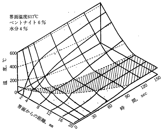
図49 生型の温度分布 (III)
