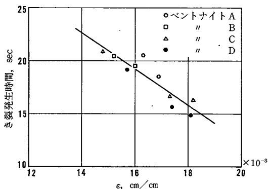
図98 き裂発生時間と膨張量との関係
