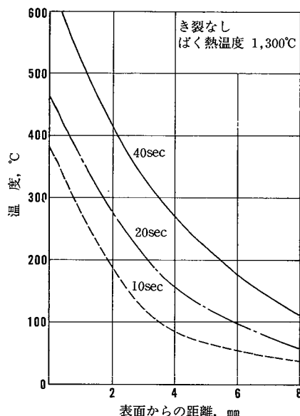
図85 試片内温度分布 (垂直方向・乾燥型)
