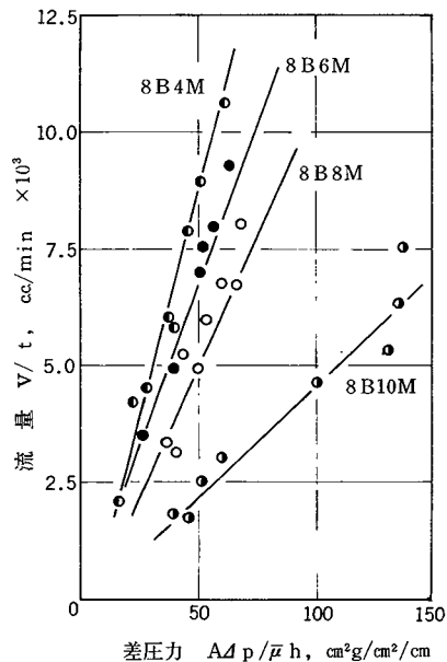
図32 流量と差圧力の関係(Ⅳ)
