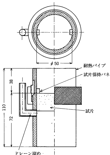
図26 試片筒
