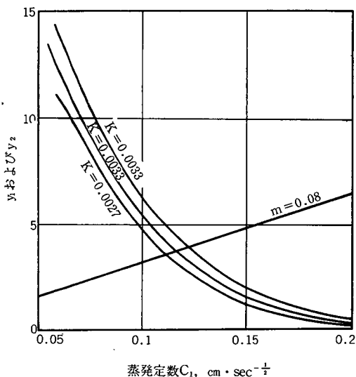
図44 温度拡散率と蒸発定数との関係
