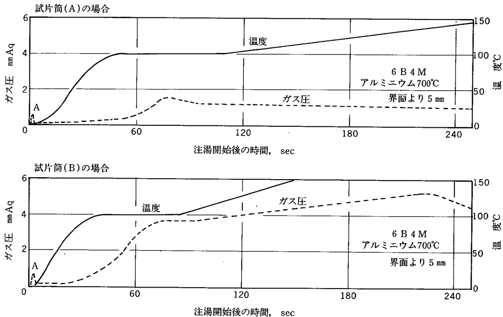
図37 鋳込み後の温度、ガス圧変化
