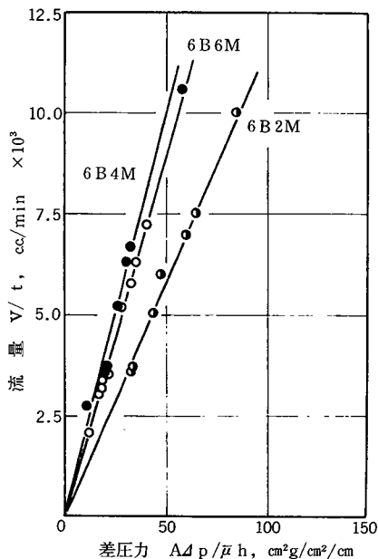
図31 流量と差圧力の関係(Ⅲ)
