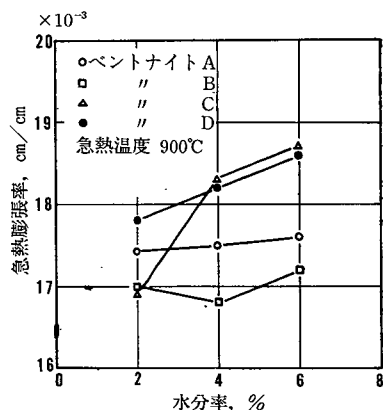
図95 急熱膨張量
