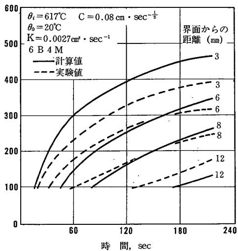
図54 乾燥域の温度分布 (アルミニウム)
