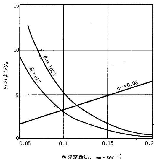
図45 界面温度と蒸発定数との関係
