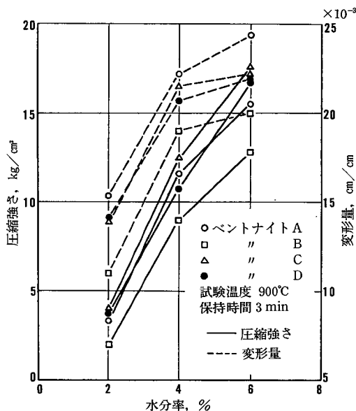
図93 高温圧縮強さと変形量
