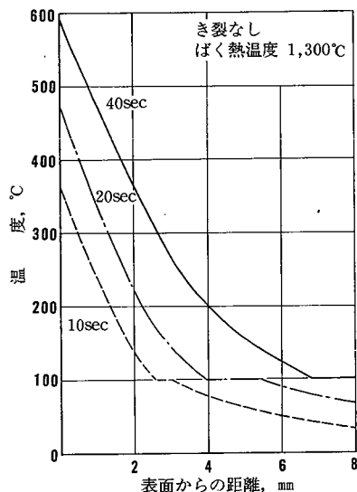
図81 試片内の温度分布
