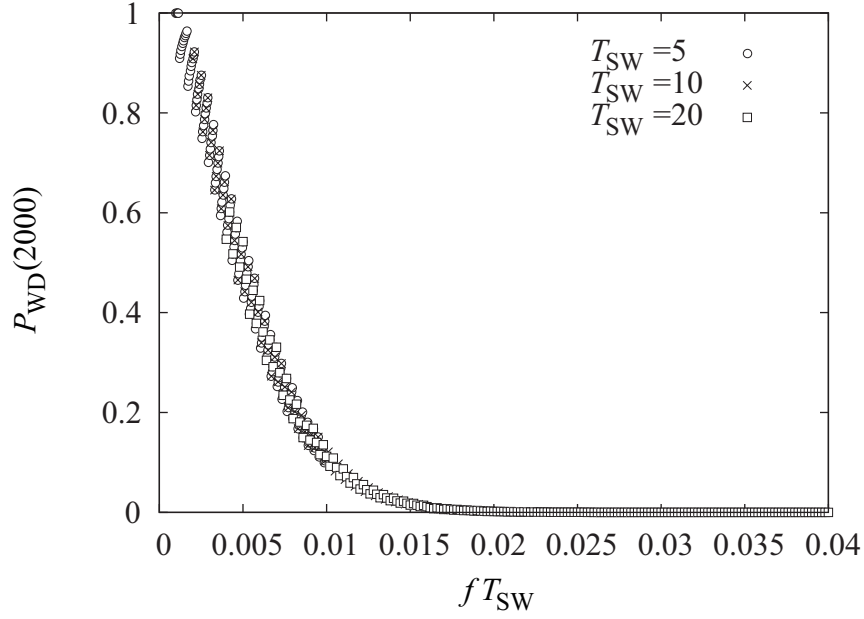
図 2.3: fT_{\text{SW}} の関数とみなした誤検出確率 ( R = 4,000 , r = 2,000 , \epsilon = 0.01 )
