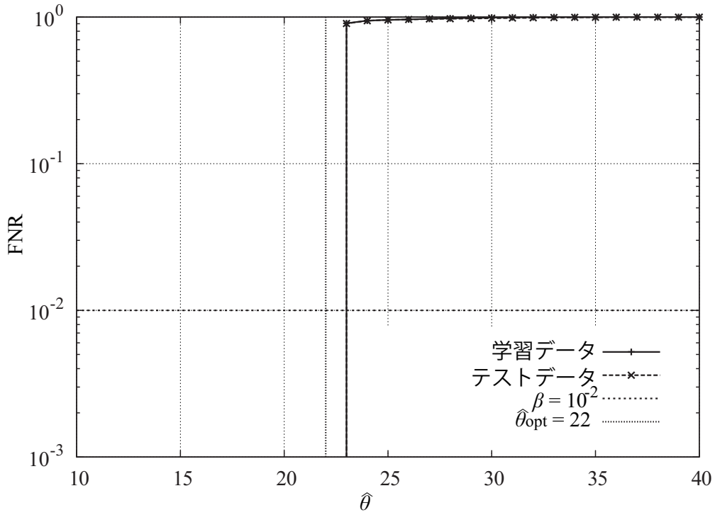
図 4.8: f = 1 としたときの FNR と閾値の関係
