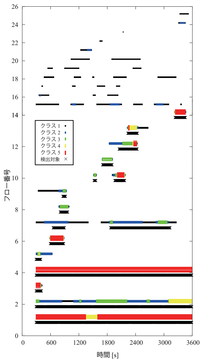
図 3.7: 検出対象と検出結果 (バックボーン).
