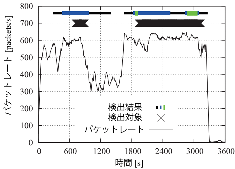
図 3.9: バックボーントレースのフロー 7 のパケットレート
