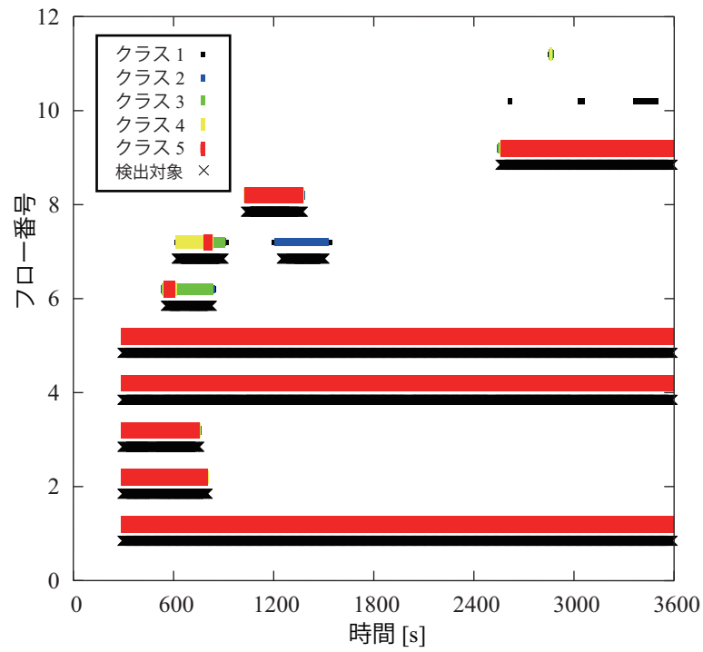
図 3.8: 検出対象と検出結果 (ボックスキャッタ).
