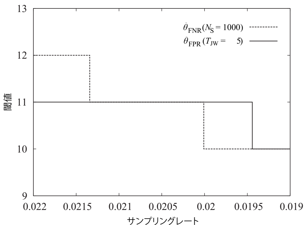
図 4.10: 交点付近における閾値 \hat{\theta}_{FPR}(T_{JW} = 5) および \hat{\theta}_{FNR}(N_S = 1000) とサンプリングレートの関係
