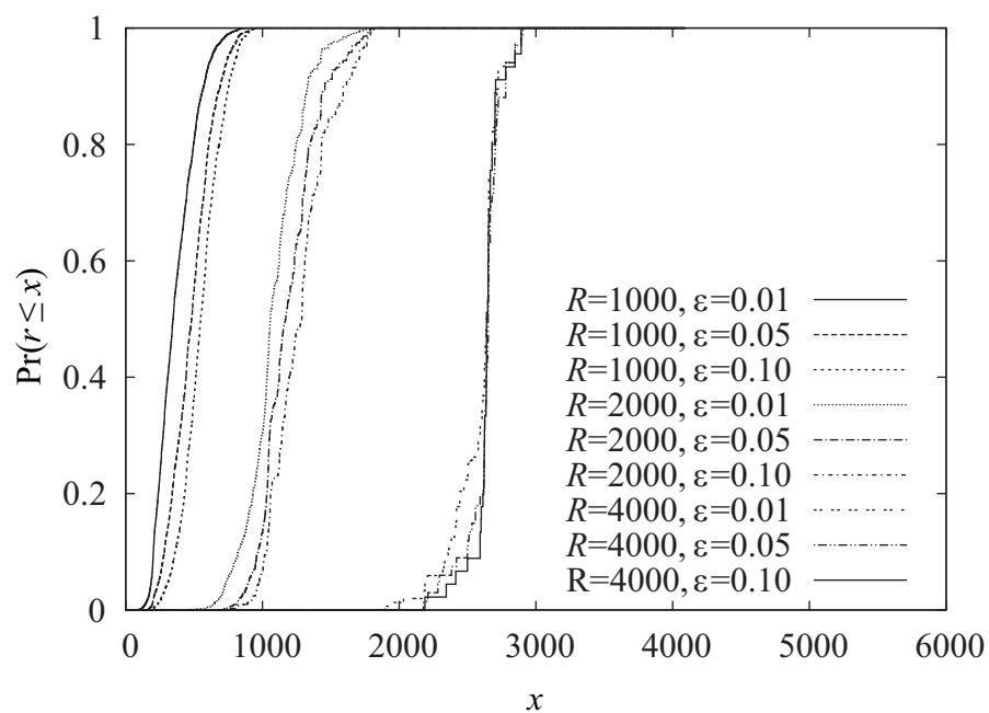
図 2.8: 誤検出されたフローのパケットレートの累積分布 ( T_{D\_max} = 20 )
