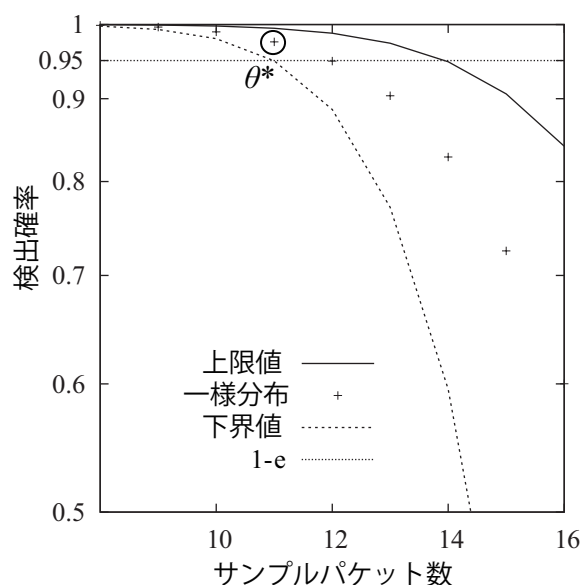
図 3.6: 一様分布フローと検出確率の関係 (バックスキャッタ)
