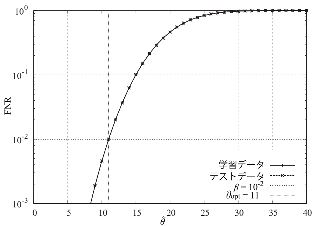
図 4.12: f = \hat{f}_{opt} としたときの FNR と閾値の関係
