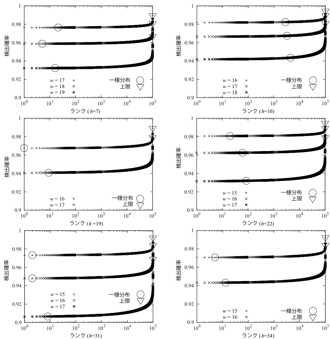
図 D.1: ランダムに生成した MTF の検出確率 ( s = 2 , m = 3 , z^* = 30,000 , f = 9.8 \times 10^{-4} , 試行回数 = 10^6 , 生成パターン数 = 10^5 , h = 4, 5, 6, 7, 8, 9 )
