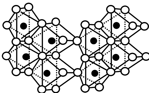
B-type monoclinic ( C2/m )
