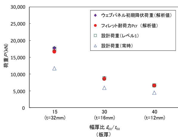
(a) SM570, 突出率 10%
