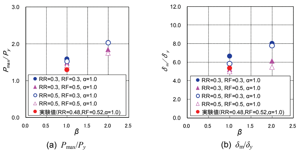
図-2.3.29 柱部フランジ幅とウェブ幅の比 \beta の影響 (最大荷重時)
