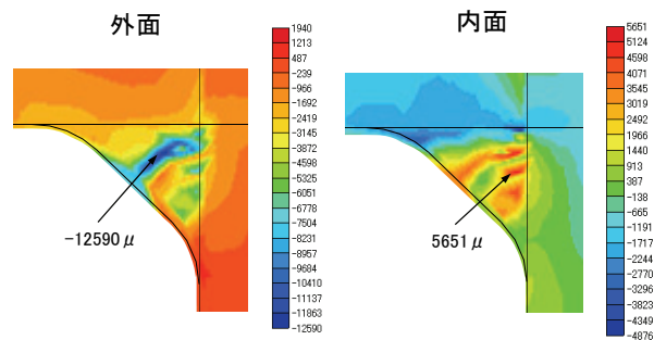
図-3.5.24 フィレットの発生ひずみ (レベル1, SM570, 突出率 15%)
