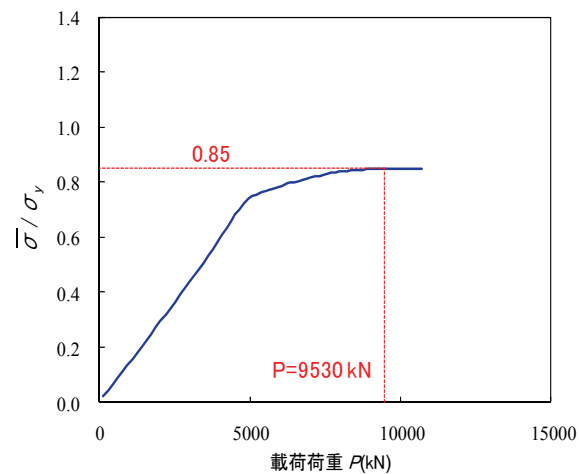
(e) CASE9 (板厚 16mm)
