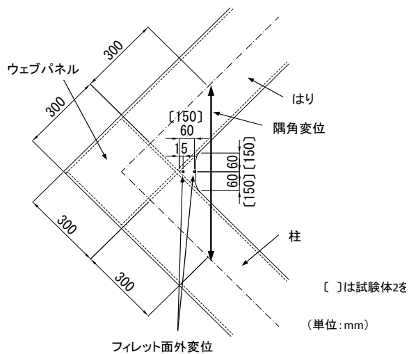
図-3.4.7 変位の計測位置
