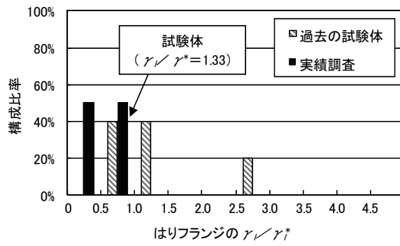
(c) はりフランジの \gamma_t/\gamma_t^*
