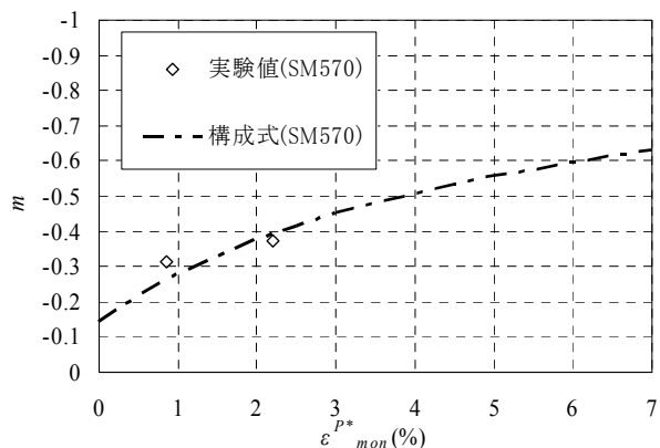
図-2.3.12 \varepsilon_{\text{mon}}^{p*} と m の関係
