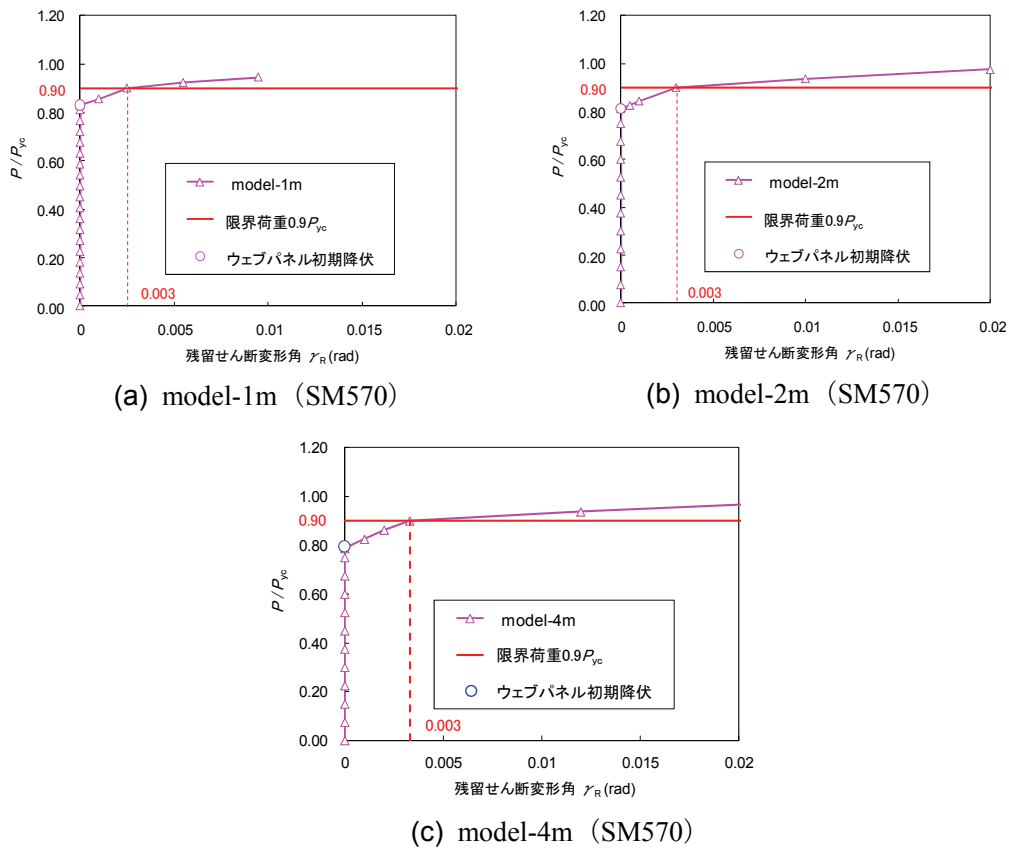
図-2.4.22 荷重とウェブパネル残留せん断変形角の関係（弾塑性有限変位解析）
