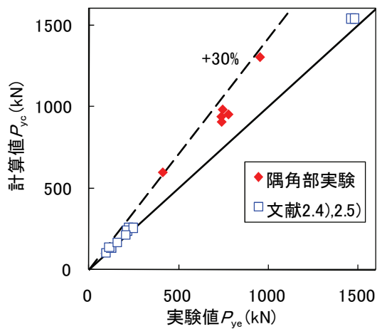
図-2.4.6 従来の方法と実験値による 降伏荷重の比較
