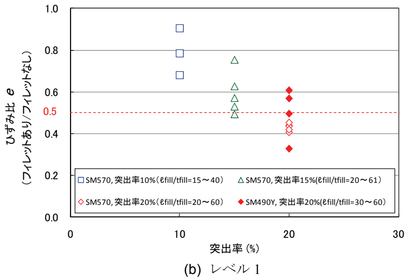
図-3.6.1 ひずみ集中低減効果とフィレット突出率の関係
