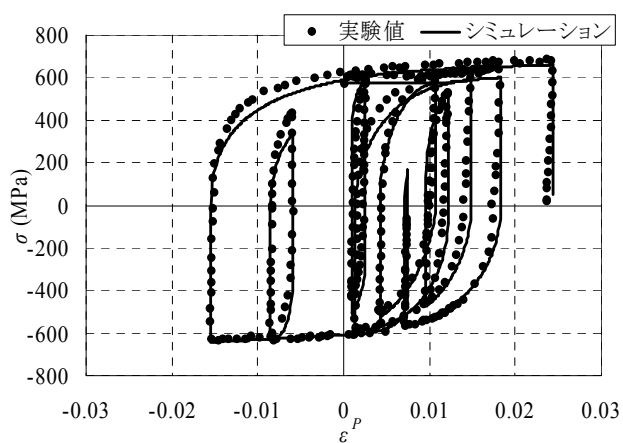
図-2.3.13 ランダム载荷試験と数値シミュレーションの比較
