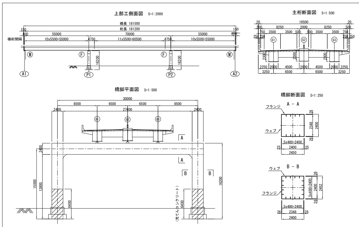
図-4.5.3 構造一般図 (model-1)
