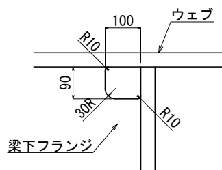
(a) 実構造物サイズ ( t=30\text{mm} )
