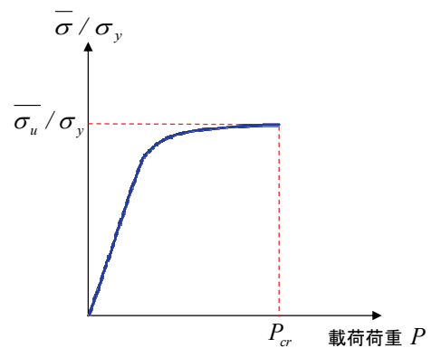
図-3.6.3 フィレット座屈荷重の算定方法
