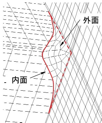
図-3.5.15 フィレット変形図 (CASE6)
