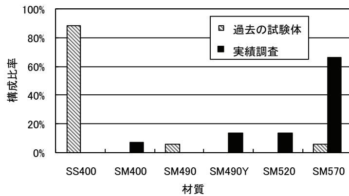
図-2.2.3 隅角部の材質の実績調査結果
