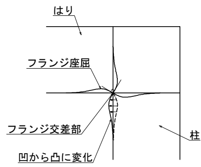
図-2.2.29 荷重低下時のフランジ変形挙動
