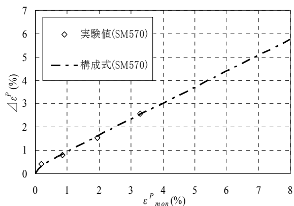
図-2.3.11 \varepsilon_{\text{mon}}^p と \Delta\varepsilon^p の関係
