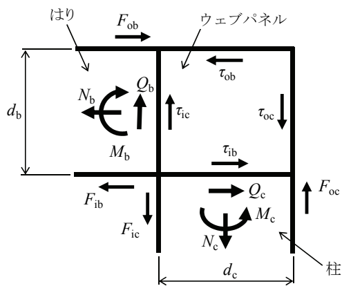
図-2.4.4 隅角部に作用する断面力 および応力度の定義
