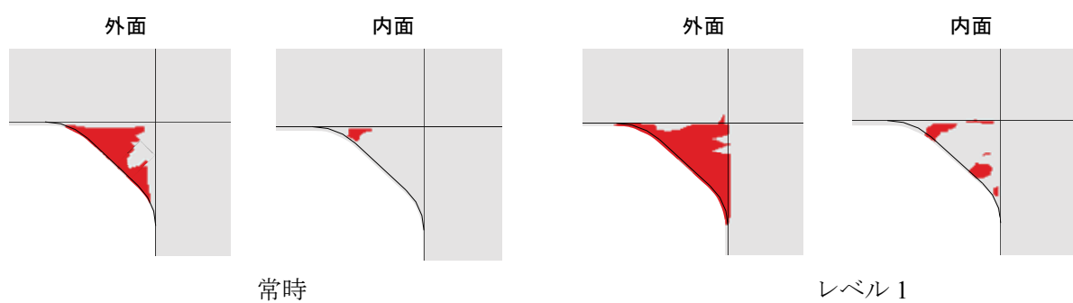
(d) CASE17 (SM490Y, 突出率 20%)
