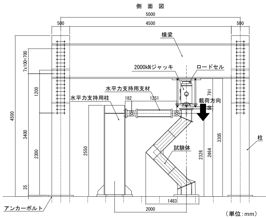
図-3.4.4 実験装置
