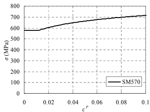
図-2.3.7 単調载荷曲線
