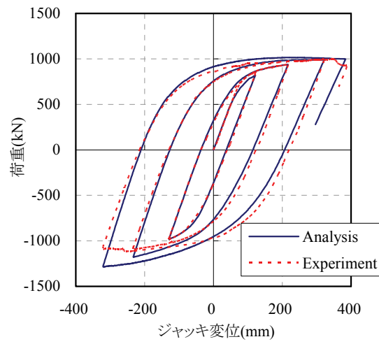
図-2.3.18 実験結果と解析結果の比較
