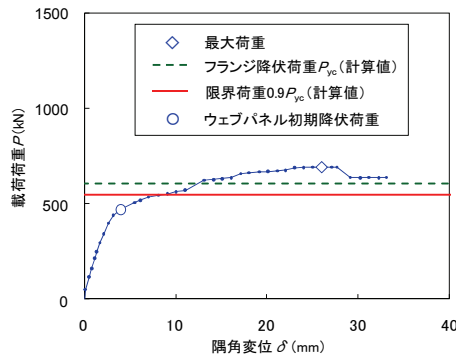
図-2.4.16 荷重と隅角変位の関係（正負交番載荷実験）
