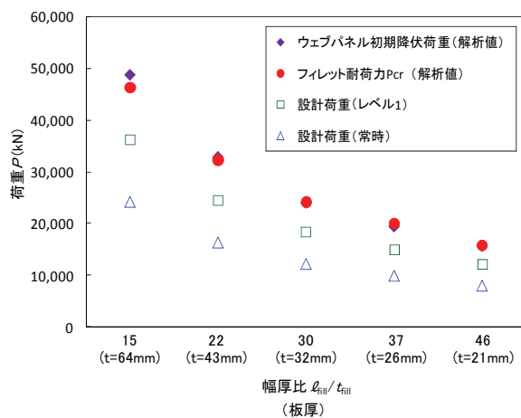
(b) SM570, 突出率 15%
