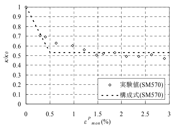
図-2.3.9 \varepsilon^P_{\text{mon}} と \kappa/\kappa_0 の関係
