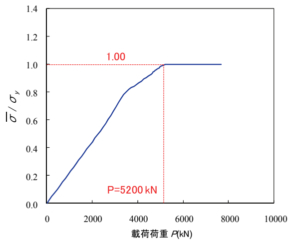
(c) CASE4 (板厚 12mm)
