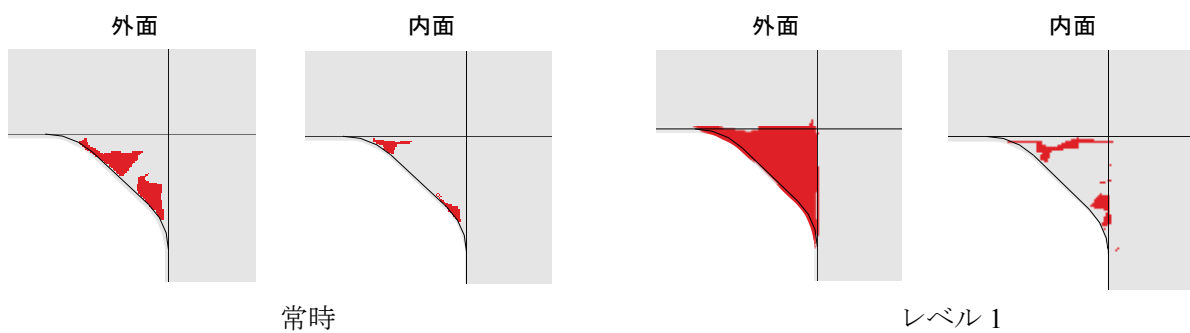
(b) CASE6 (SM570, 突出率 20%)
