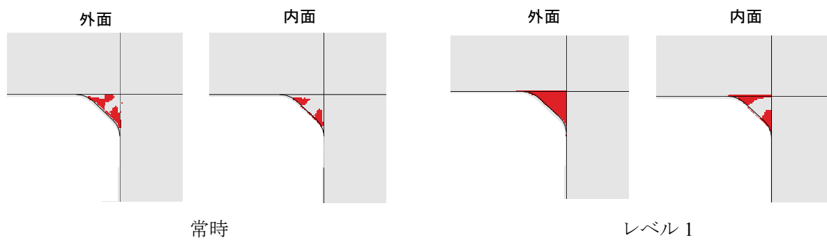
(a) CASE2 (板厚 32mm)
