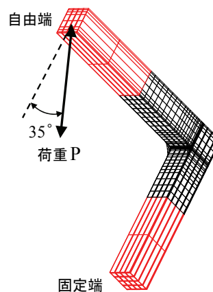
図-2.3.14 解析モデル
