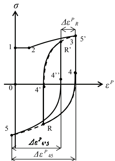
図-2.3.5 非線形遷移領域での再反転
