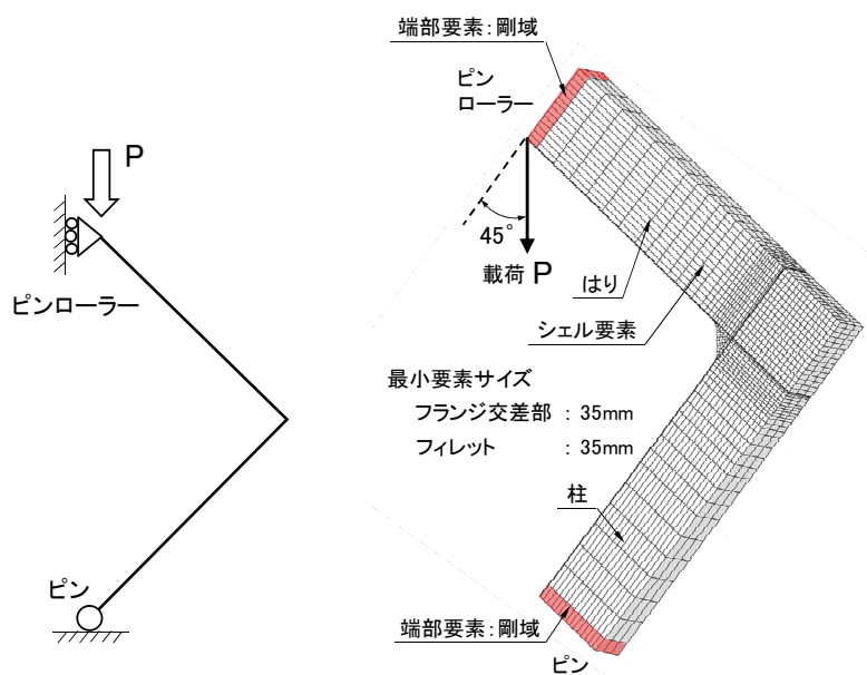
図-3.5.3 境界条件
