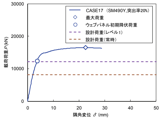
(b) CASE17 (SM490Y, 辺長比 1.0, 突出率 20%)
