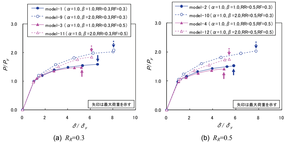
図-2.3.28 柱部フランジ幅とウェブ幅の比 \beta の影響
