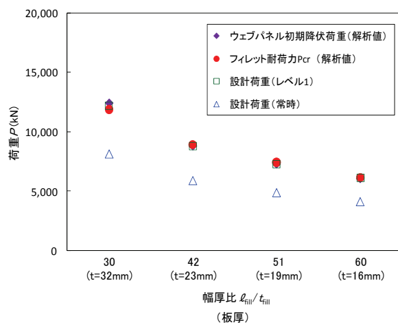
(d) SM490Y, 突出率 20%
