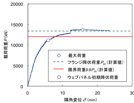
図-2.4.17 載荷荷重と隅角変位の関係（弾塑性有限変位解析）
