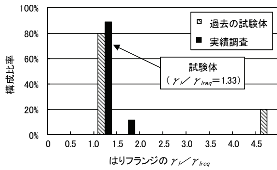
(a) はりフランジの \gamma_t/\gamma_{req}
