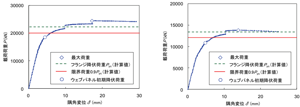
図-2.4.16 荷重と隅角変位の関係（正負交番載荷実験）
