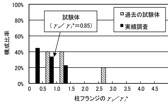
(d) 柱フランジの \gamma_t/\gamma_t^*
