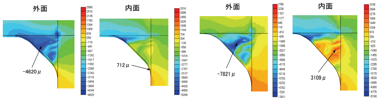
(a) CASE5 (板厚 48mm)
