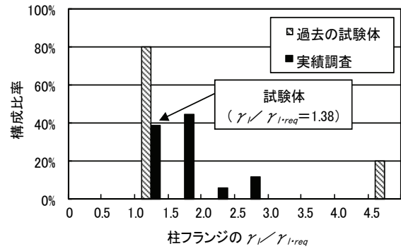
(b) 柱フランジの \gamma_t/\gamma_{req}
