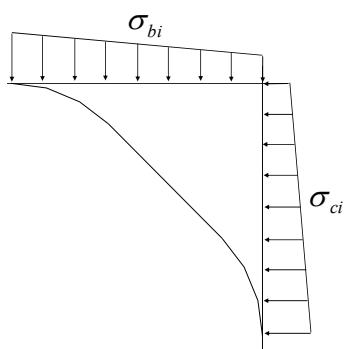
図-3.6.2 フィレット境界辺の主応力分布（模式図）
