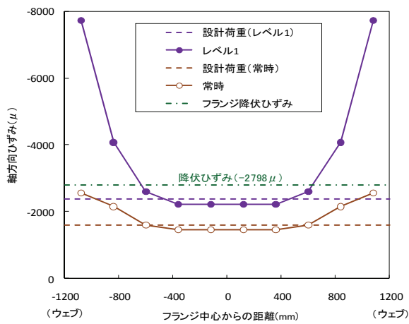
(a) CASE1 (フィレットなし, 板厚 32mm)
