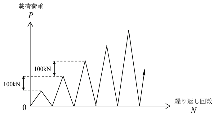
図-3.4.5 荷重載荷パターン
