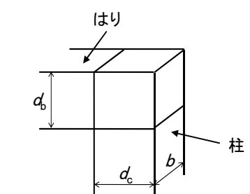
図-3.5.5 隅角部寸法の定義
