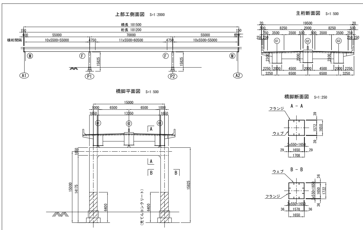
図-4.5.4 構造一般図 (model-2)
