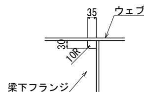
(b) 試験体サイズ ( t=10\text{mm} )
