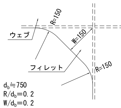
図-2.2.6 フィレット形状
