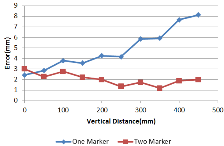
Fig.4-12. Errors per y distance
