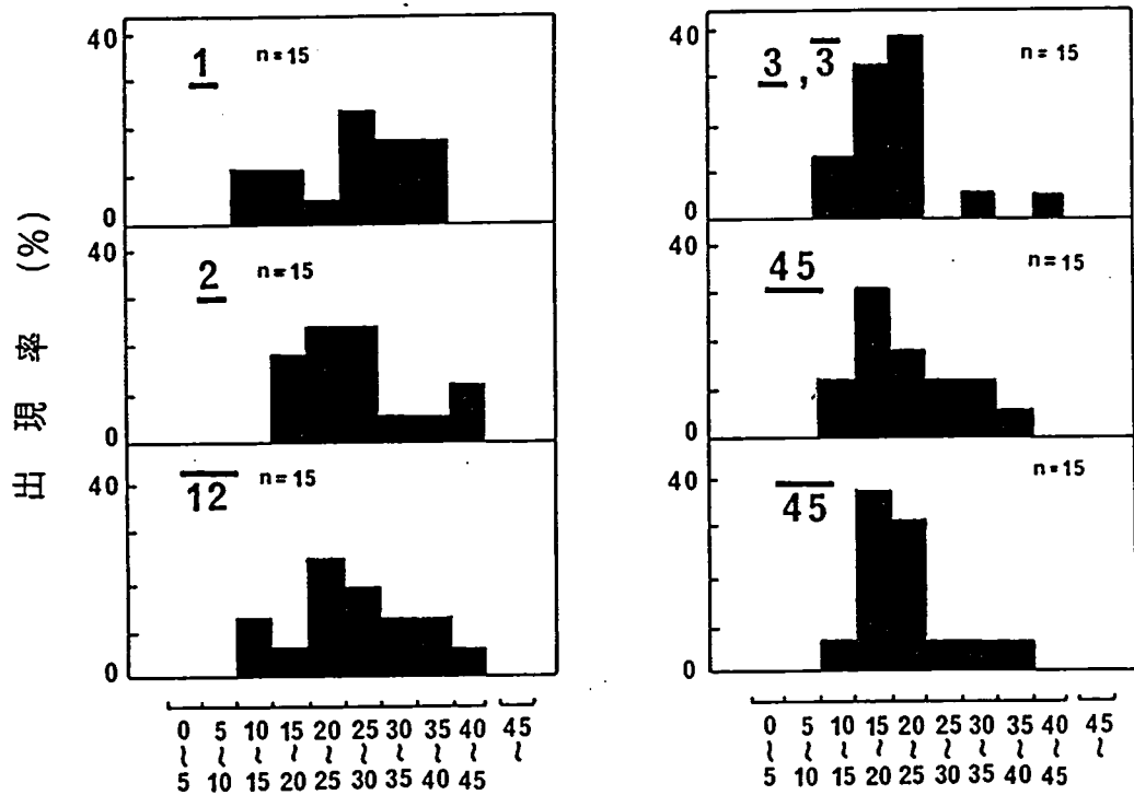
ディボンディングに要する力 (kgf)
