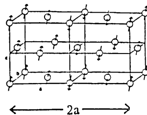
図3 磁気構造
