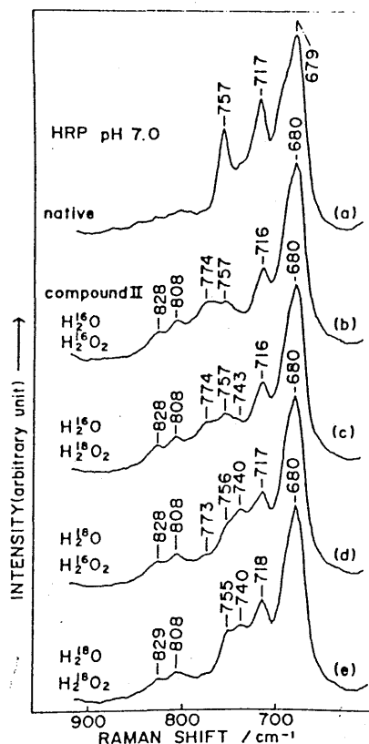
図1 Compound IIの共鳴ラマンスペクトル
