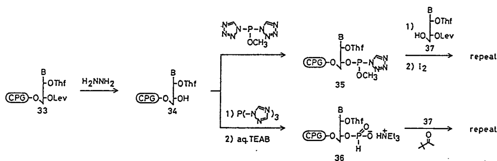
図26 5'→3'方向のホスファイト法およびH-ホスホネート法によるオリゴリボヌクレオチドの固相合成の検討
