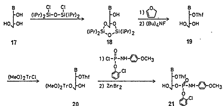
図16 モノマー ユニットの合成
