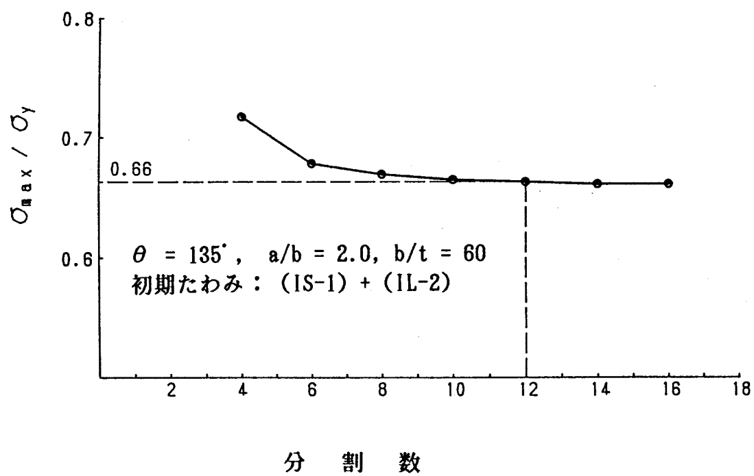
図 2. 5 軸方向分割数
