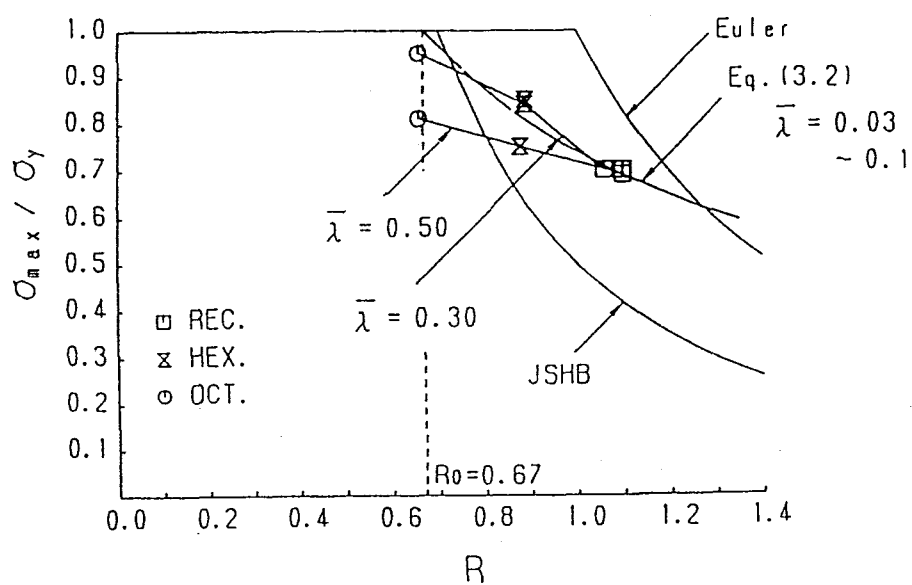
图 5. 9 最大平均应力 \sim R 曲线
