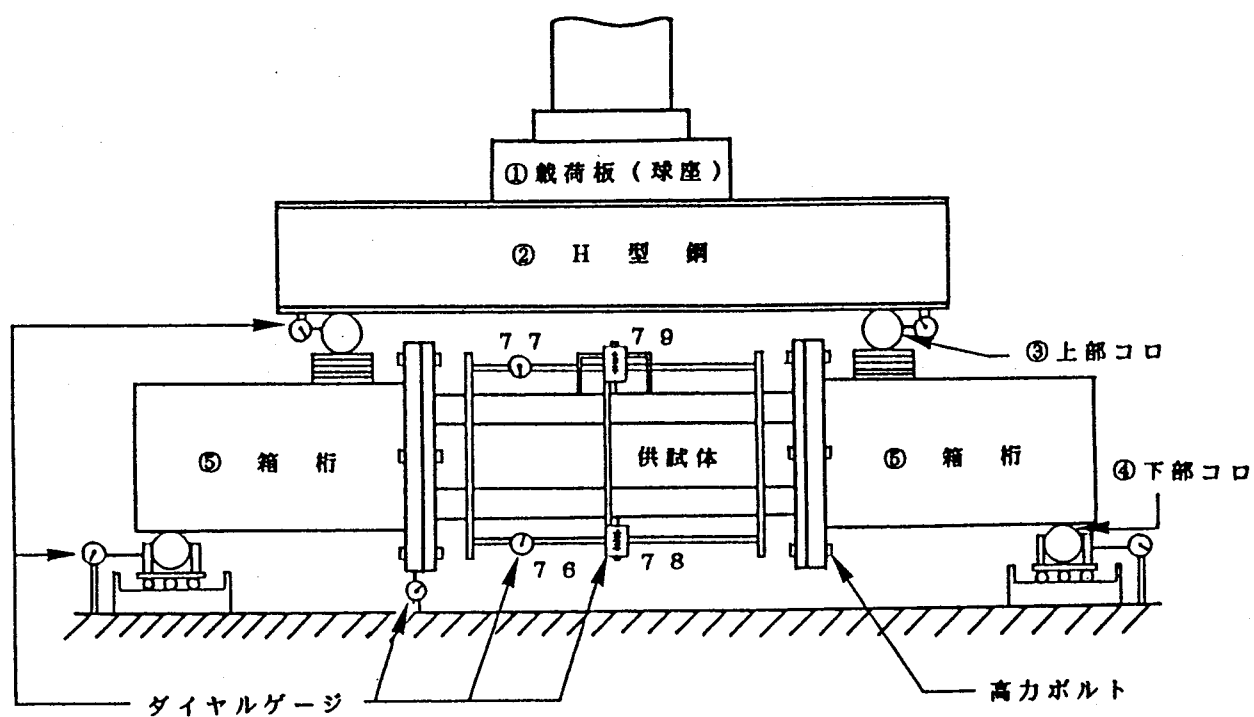
図 4. 2 載 荷 装 置
