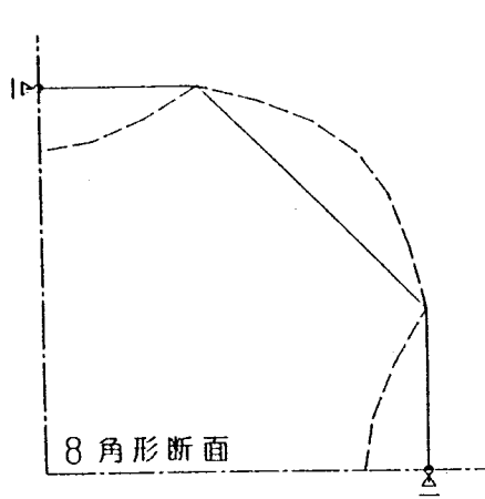
図 2. 1 1 解析モデルおよび初期たわみ
