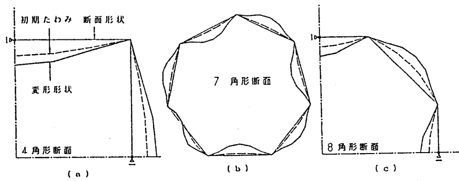
図 2. 17 変形形状
