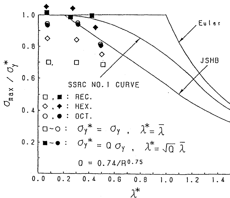
图 5. 1 0 最大平均应力 \sim \lambda 曲线
