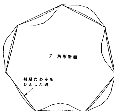
図 2. 1 2 5、7 角形断面の変形形状
