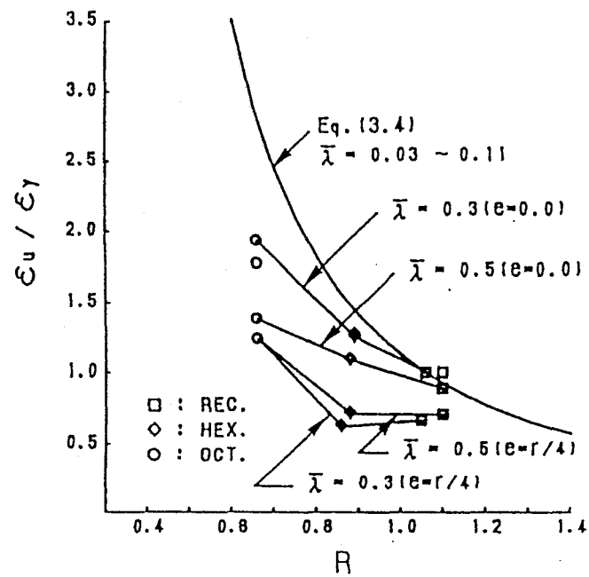
図 5. 1 2 最大平均応力時のひずみ～R 曲線
