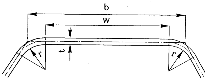
図 3. 1 9 板要素の幅
