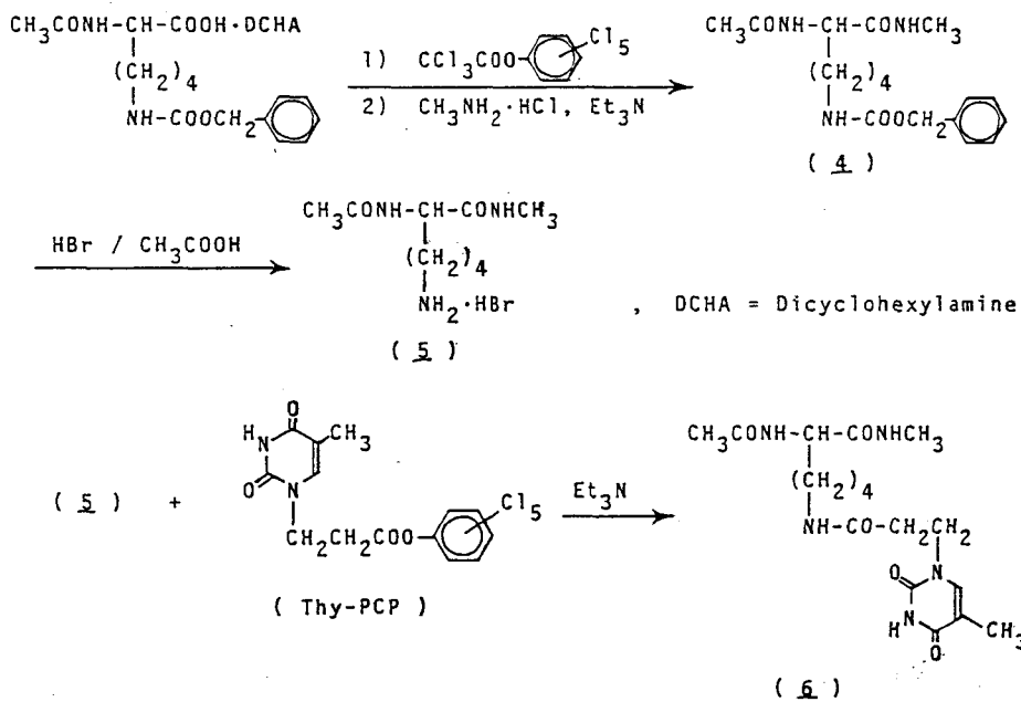
( Scheme III-2 )
