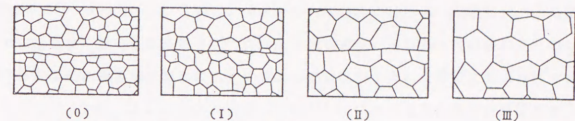
(0)接触前、(I)接合面の部分的接触と接触部の変形、(II)接触部の接合とボイドの収縮、(III)ボイドの消滅と粒界移動
