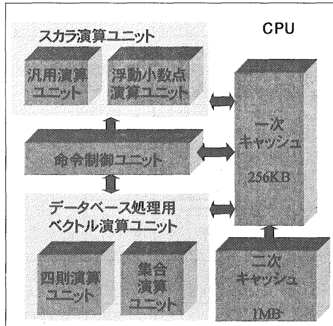
図 4.9 M-680H/IDP の CPU 構成
