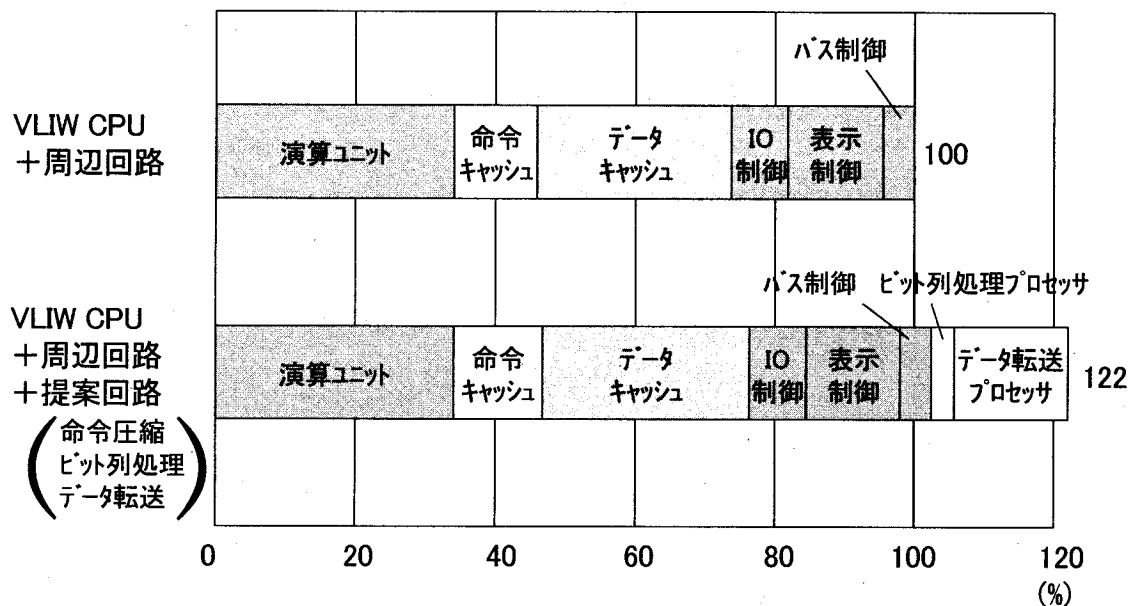
図 2.11 提案回路の実装面積オーバーヘッド
