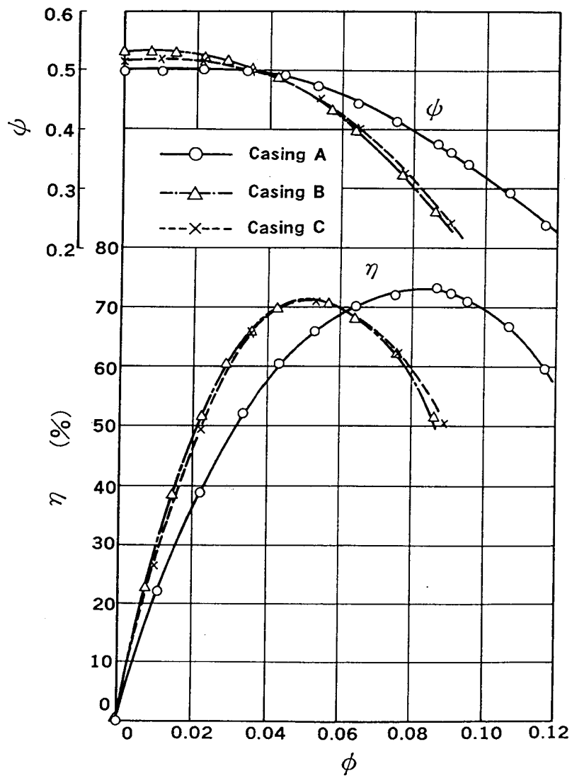
図11 ポンプ特性
