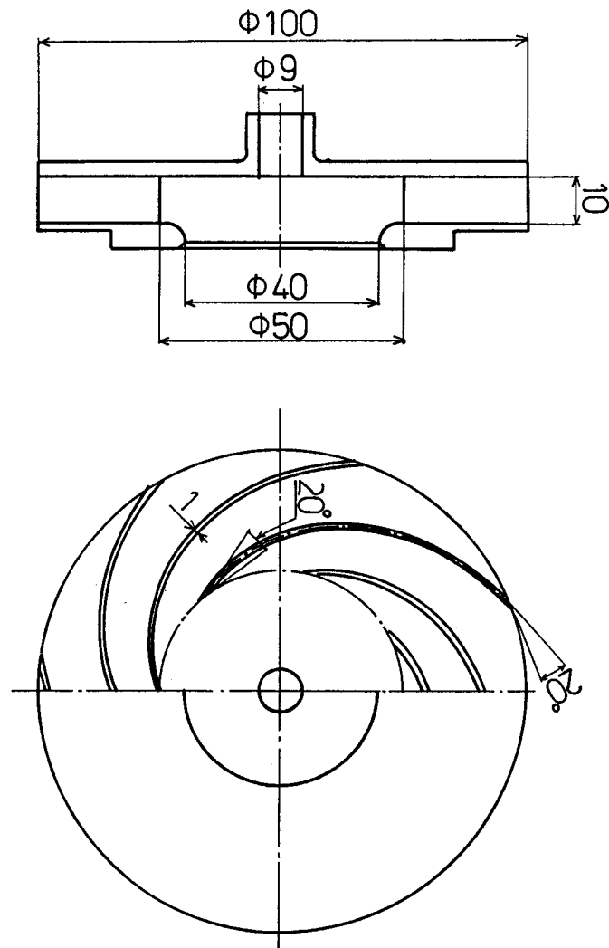
図5 供試羽根車
