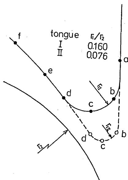
(b) 舌部形状
