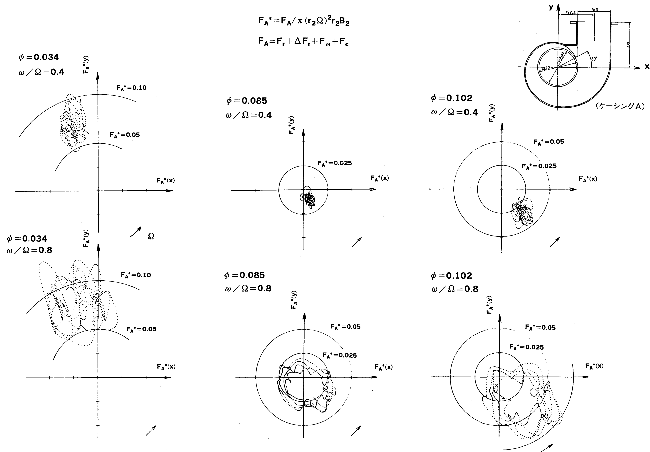
図13 羽根車に作用する力のリサージュ線図 (ケーシングA)
