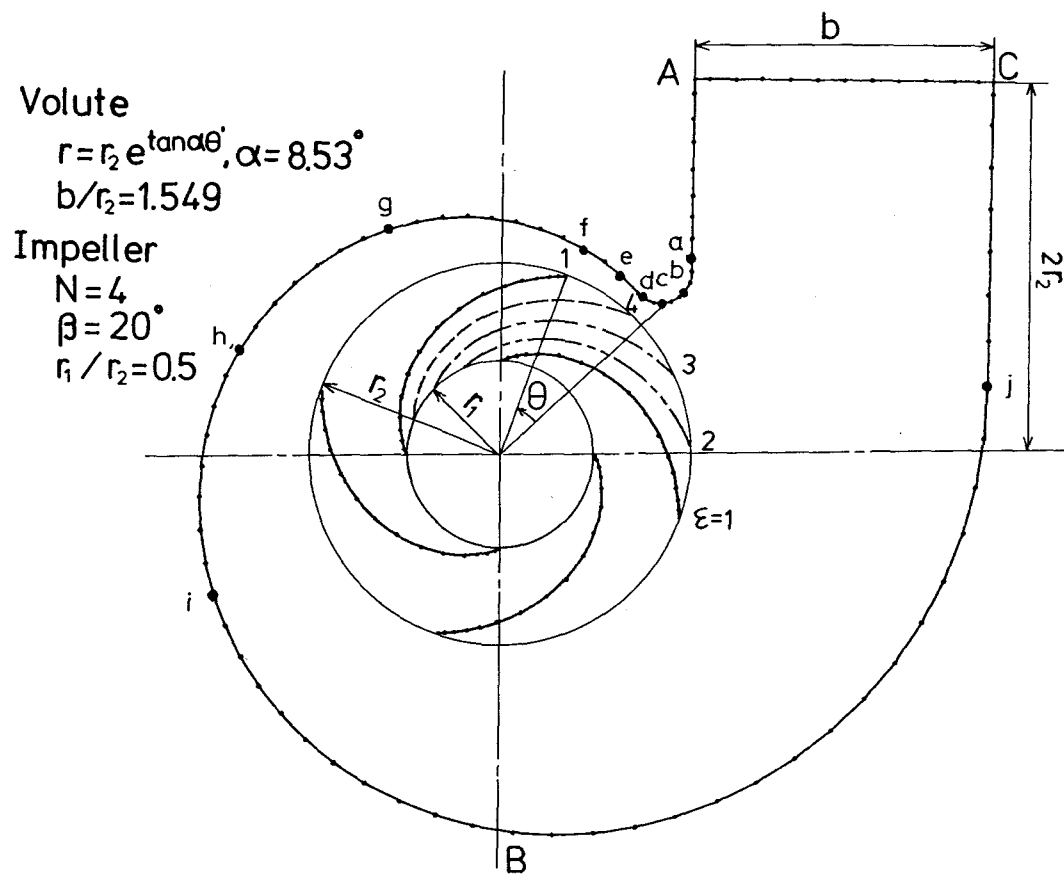
(a) 羽根車とケーシングの形状
