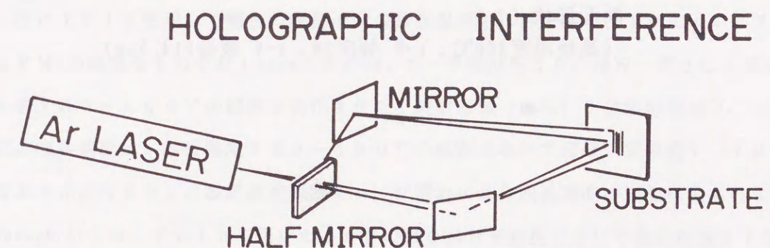
図3.12 二光束干渉法による縞状パターンの照射方法
