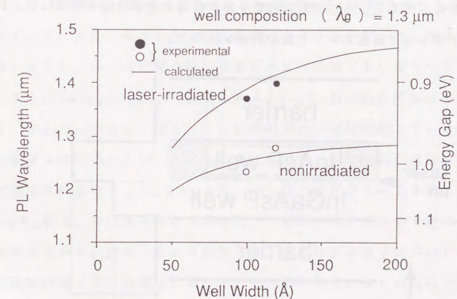
図5. 18 \text{In}_{1-x}\text{Ga}_x\text{As}_{1-y}\text{P}_y 井戸層の膜厚を変えた場合のMQWのPLピーク波長 上は井戸層にレーザ照射した場合、下は照射せずに成長した場合。 障壁層： \text{In}_{1-x}\text{Ga}_x\text{As}_{1-y}\text{P}_y ( \lambda_g=1.0\mu\text{m} ) (基板温度 520^\circ\text{C} 、レーザ強度5W、レーザ波長オールライン)
