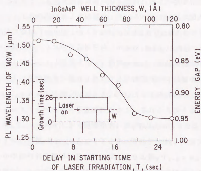
図5.20 レーザ照射を用いて成長した非対称量子井戸におけるバンドギャップ波長と照射開始の遅延時間(T)との関係(基板温度520℃、レーザー強度5W、レーザー波長オールライン)
