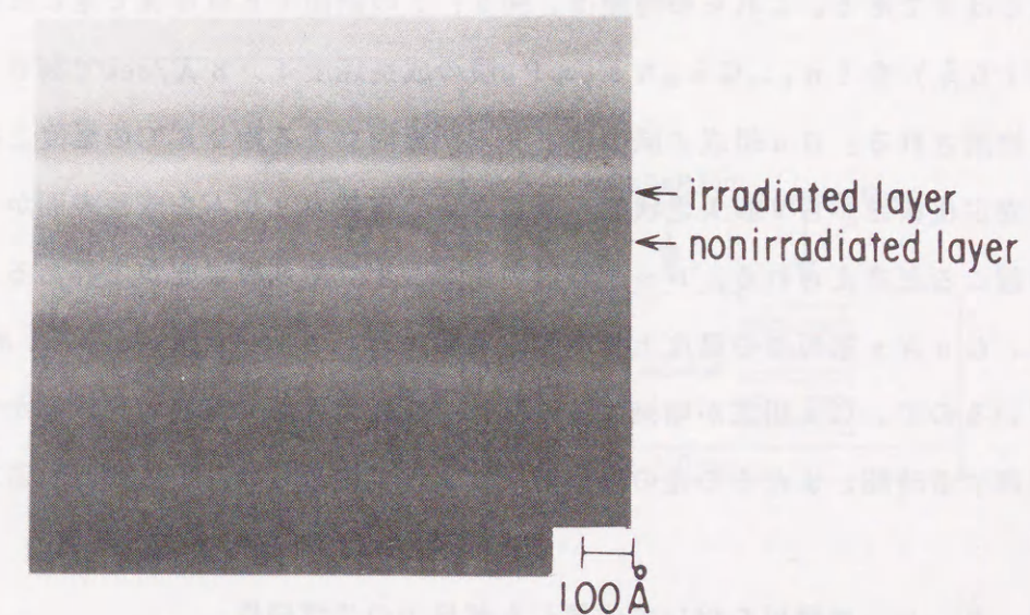
図5.7 \text{In}_{1-x}\text{Ga}_x\text{As}_{1-y}\text{P}_y 膜成長中にレーザ照射をオン、オフした領域の断面TEM写真 (基板温度510℃、レーザ強度5W、レーザ波長0.488μm)
