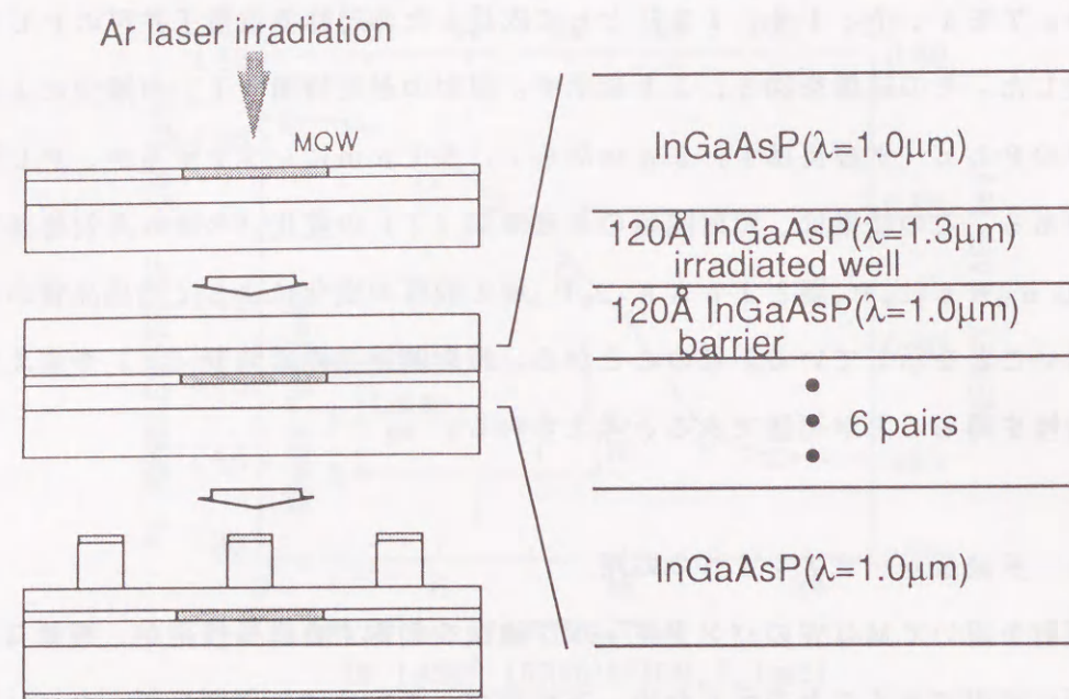
図5.22 リッジ型2波長レーザアレイの作製方法
