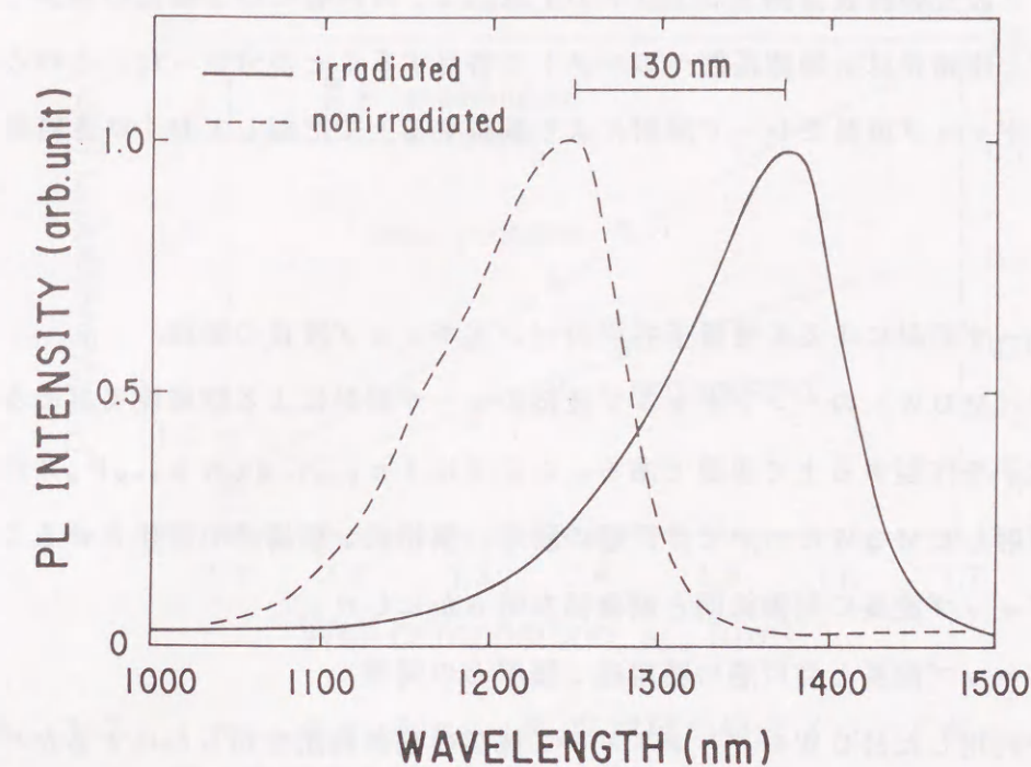
図5.15 \text{In}_{1-x}\text{Ga}_x\text{As}_{1-y}\text{P}_y 井戸層成長中にレーザ照射して成長したMQWと照射を行わずに成長したMQWの室温のPLスペクトルの比較（障壁層：InP膜、基板温度510℃、レーザ強度5W、レーザ波長0.7μm）
