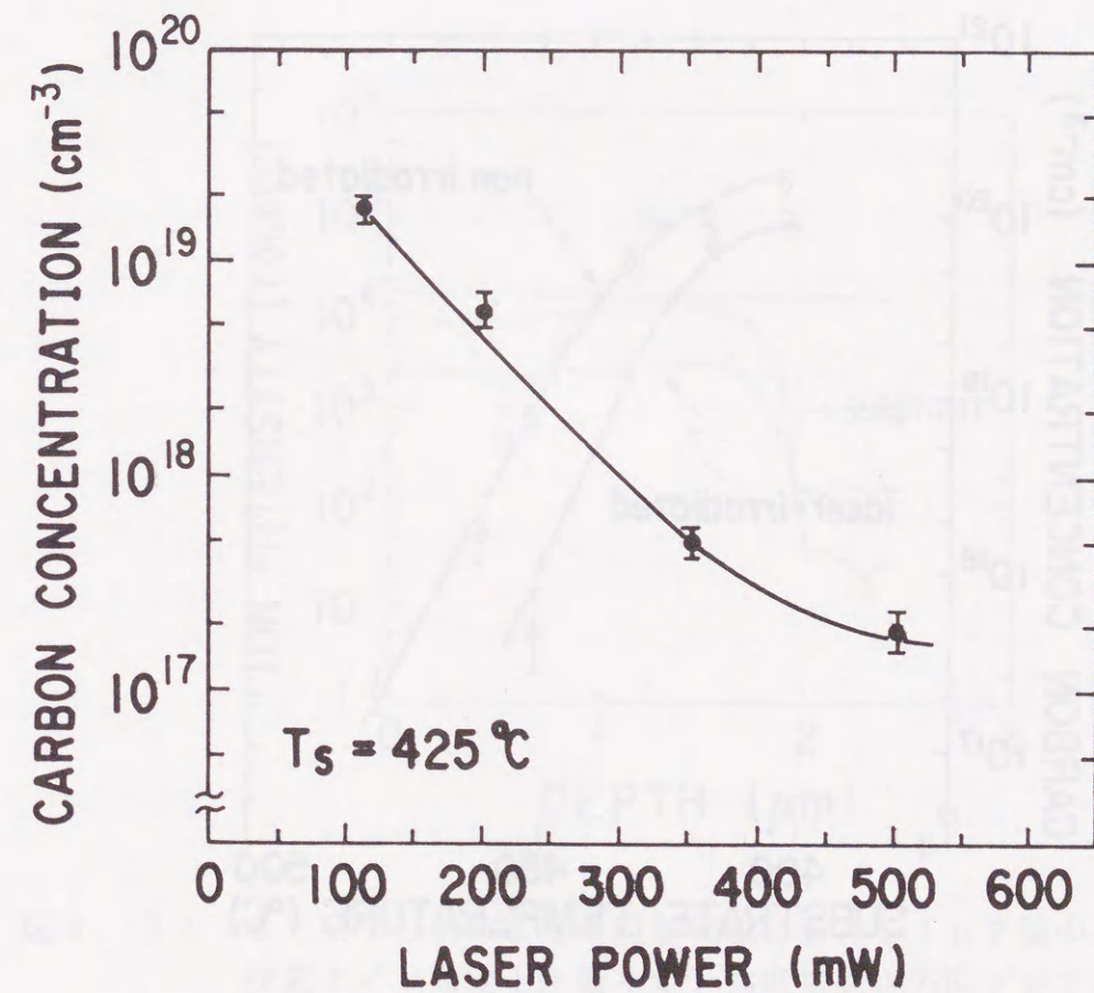
図3. 22 レーザー照射領域におけるGaAs膜中の炭素濃度のレーザー強度依存性 (基板温度425℃、レーザー波長514.5nm)
