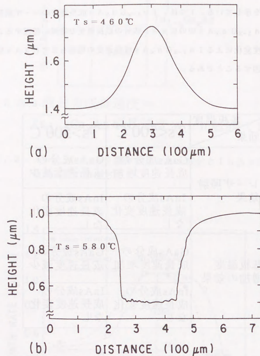
図4.4 レーザ照射領域の断面形状
