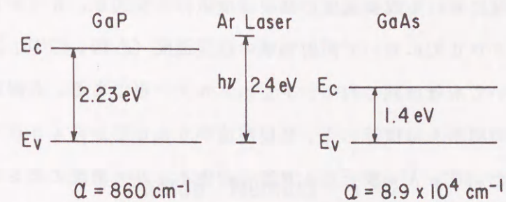
図 3.5 (a) GaAs 膜と GaP 膜におけるアルゴンレーザー光 (波長 514.5 nm) に対する吸収係数の比較
