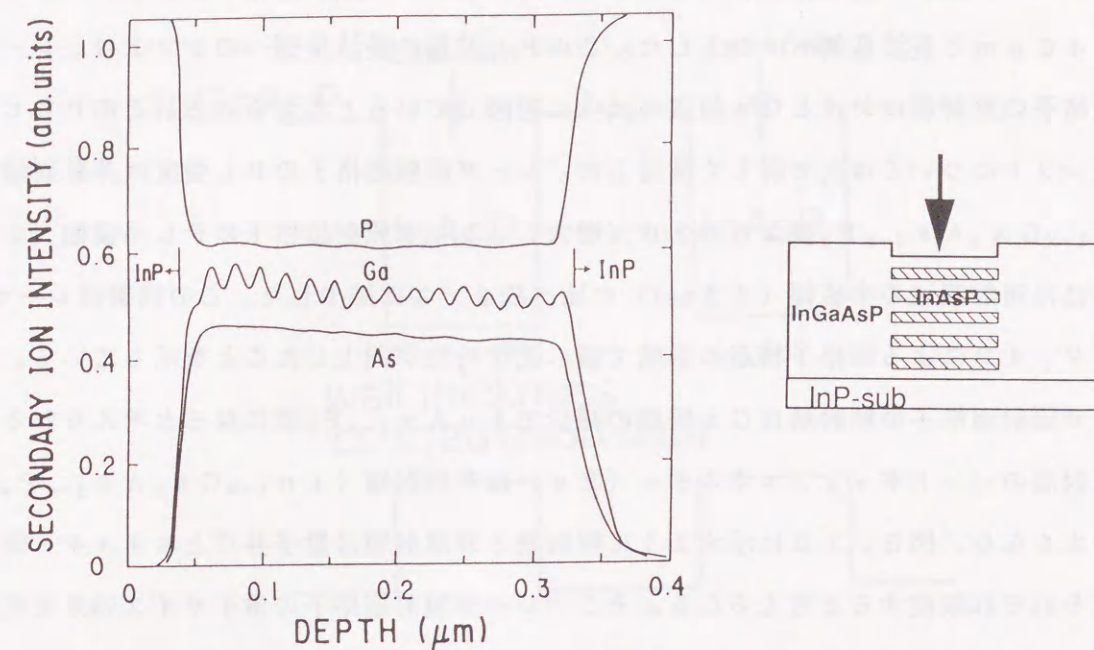
図5. 8 レーザ照射のオン、オフによって成長した超格子中のGa、As、Pイオン強度の深さ方向プロファイルをSIMS分析で調べた結果 (基板温度510℃、レーザ強度5W、レーザ波長0.7μm)
