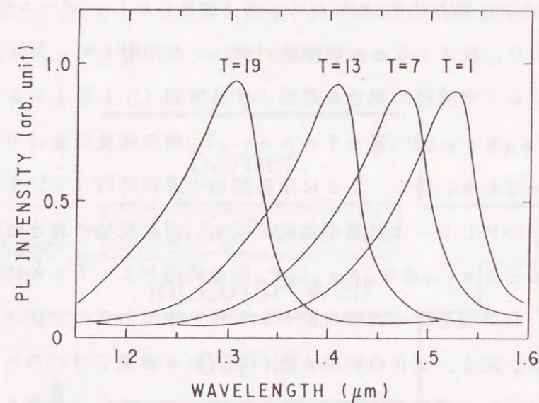
図5.21 レーザ照射を用いて成長した非対称量子井戸のPLスペクトルと照射開始の遅延時間(T)との関係(基板温度520℃、レーザー強度5W、レーザー波長オールライン)
