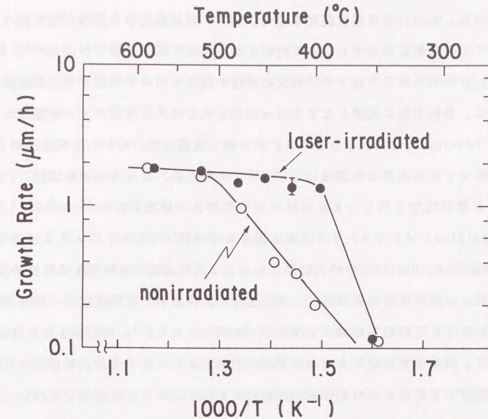
図3.1 レーザ照射領域と非照射領域におけるGaAs成長速度の基板温度依存性 (レーザ強度500mW、レーザ波長514.5nm)
