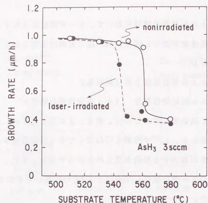
図4.7 基板温度500℃以上におけるレーザ照射領域と非照射領域の \text{In}_{1-x}\text{Ga}_x\text{As} 成長速度の基板温度依存性（レーザ強度500mW、レーザ波長514.5nm）
