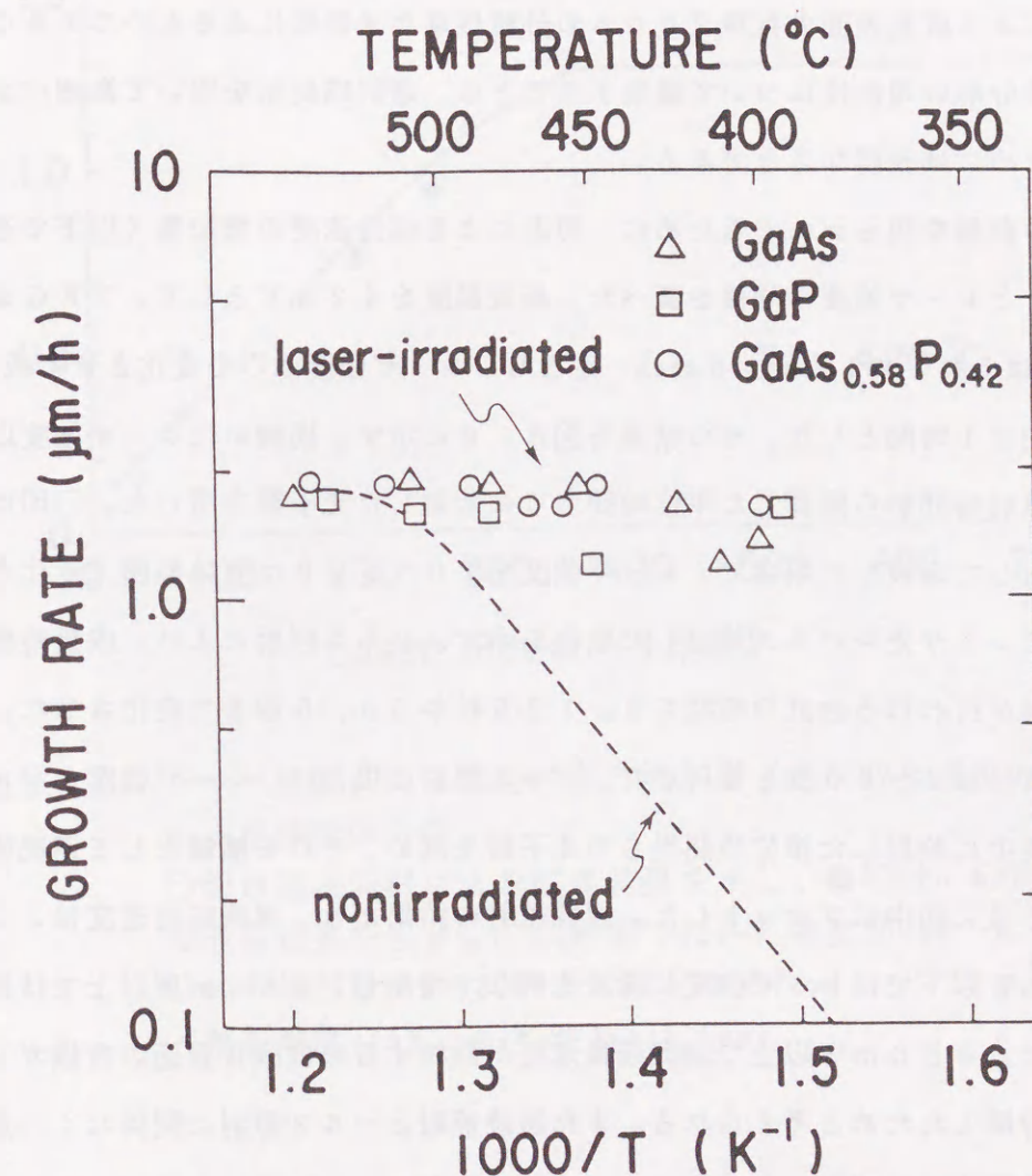
図 3.5 (b) GaAs、GaP、GaAs 0.58 P 0.42 膜のレーザー照射領域と非照射領域における成長速度の基板温度依存性 (レーザー強度 500 mW、レーザー波長 514.5 nm)
