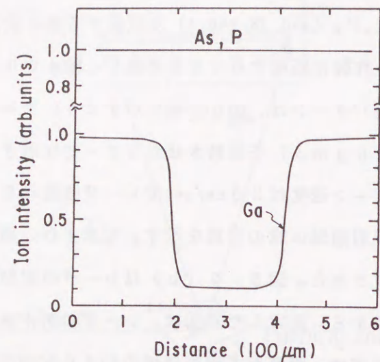
図5.3 \text{In}_{1-x}\text{Ga}_x\text{As}_{1-y}\text{P}_y 成長中にレーザ照射した膜表面の組成のSIMS分析による評価 (基板温度510℃、レーザ強度5W、レーザ波長オールライン)
