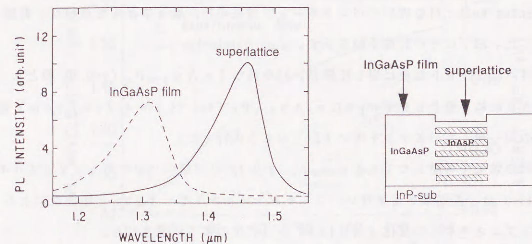
図5. 9 レーザ照射のオン、オフを用いて成長した超格子と非照射領域に成長した \text{In}_{1-x}\text{Ga}_x\text{As}_{1-y}\text{P}_y 膜の室温のPLスペクトル (基板温度510℃、レーザ強度5W、レーザ波長0.7μm)
