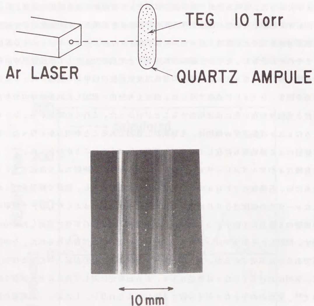
図3.10 TEGaを封入した石英管へのレーザー照射実験 (室温、レーザー強度500mW、レーザー波長514.5nm、TEGa圧力10torr)
