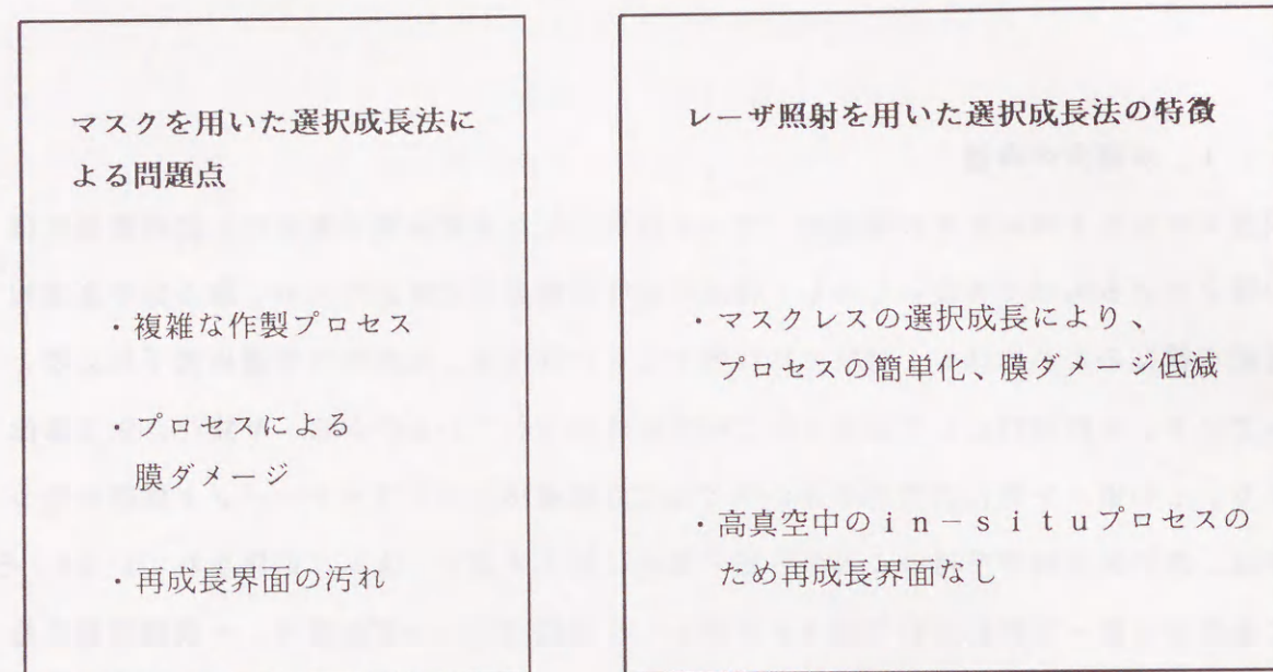
図1.1 マスクを用いた選択成長法による半導体素子の作製上における問題点とレーザー照射を用いた選択成長法の特徴との関係
