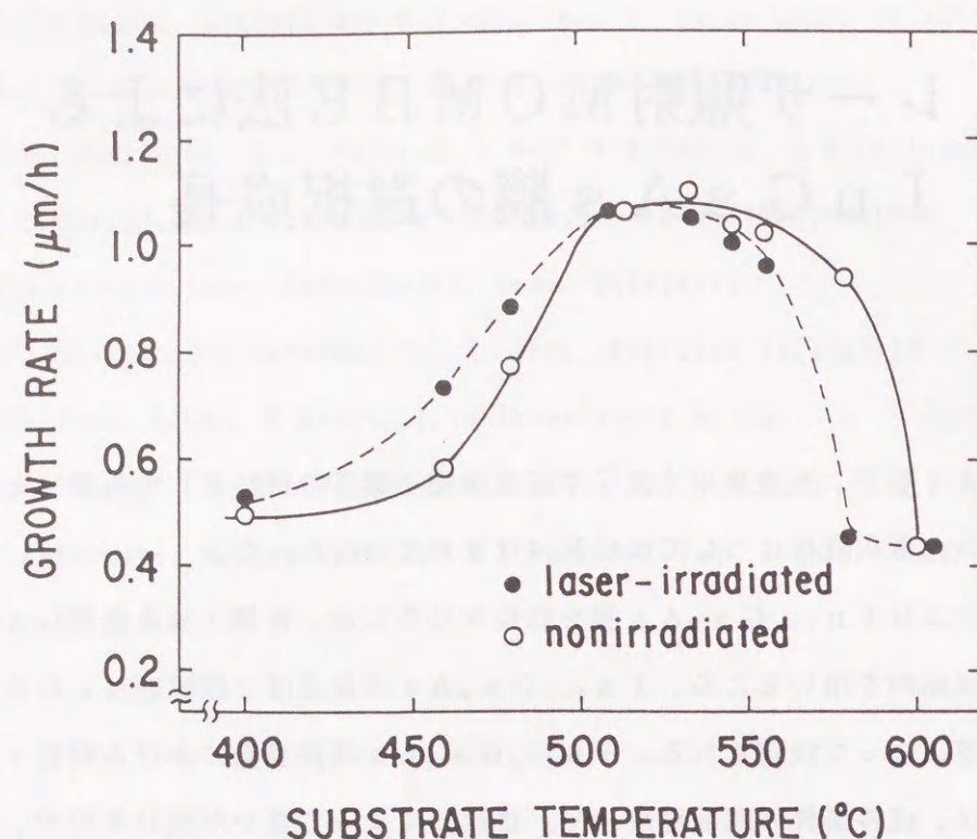
図4.1 レーザ照射領域と非照射領域における \text{In}_{1-x}\text{Ga}_x\text{As} 成長速度の基板温度依存性 (レーザー強度500mW、レーザー波長514.5nm)
