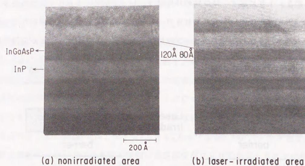
図5.14 \text{In}_{1-x}\text{Ga}_x\text{As}_{1-y}\text{P}_y 井戸層成長中にレーザ照射して成長したMQWと照射を行わずに成長したMQWの断面TEM写真の比較（障壁層：InP膜、基板温度510℃、レーザ強度5W、レーザ波長0.7μm）
