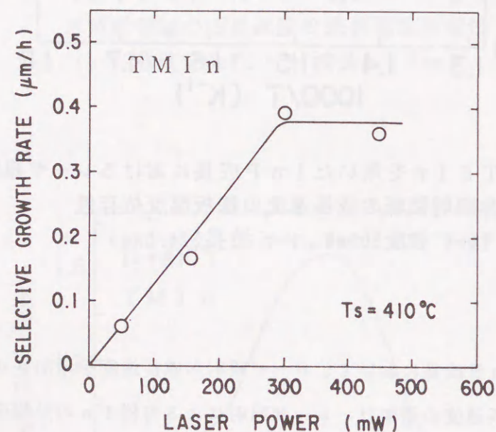
図3.17 レーザ照射によるInP成長速度の増加量（選択成長速度）のレーザ強度依存性 （原料TMIn、基板温度 410^\circ\text{C} 、連続照射、レーザ波長 514.5 \text{ nm} ）
