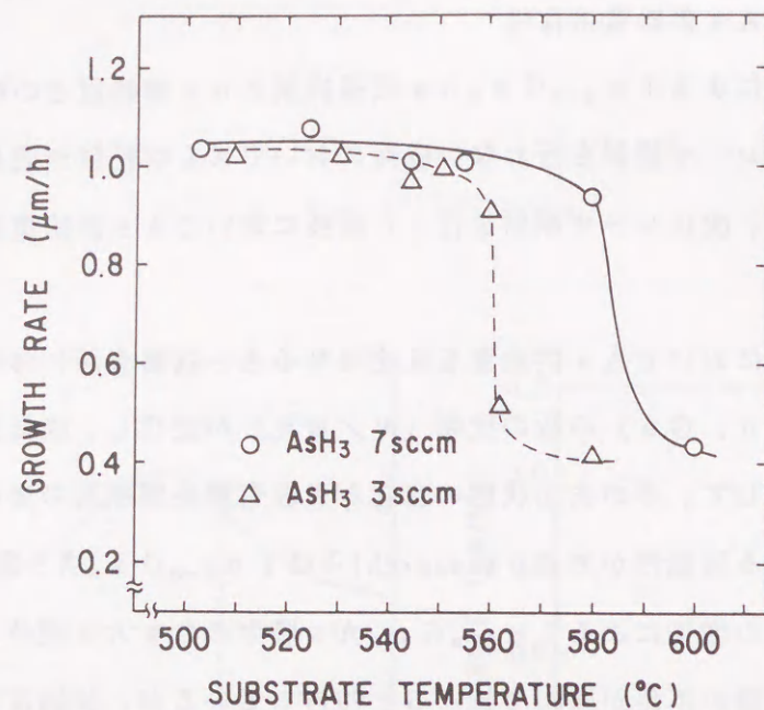
図4.10 非照射領域における \text{In}_{1-x}\text{Ga}_x\text{As} 成長速度の基板温度依存性と \text{AsH}_3 供給量との関係
