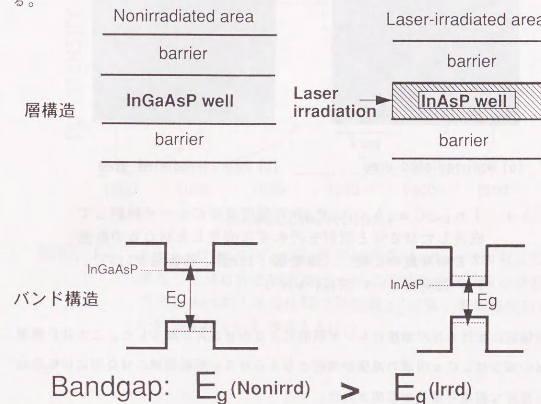
図5.13 \text{In}_{1-x}\text{Ga}_x\text{As}_{1-y}\text{P}_y 井戸層成長中にレーザ照射して成長したMQWと照射を行わずに成長したMQWの層構造の模式図とエネルギーバンド構造
