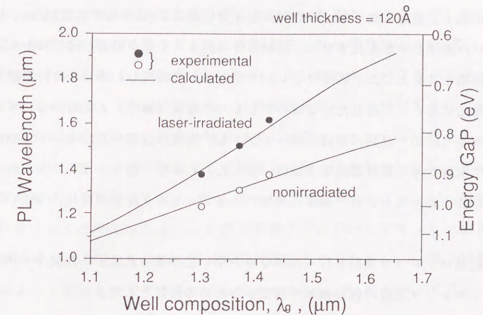
図5. 17 \text{In}_{1-x}\text{Ga}_x\text{As}_{1-y}\text{P}_y 井戸層の組成(バンドギャップ波長)を変えた場合のMQWのPLピーク波長 上は井戸層にレーザ照射した場合、下は照射せずに成長した場合。 障壁層： \text{In}_{1-x}\text{Ga}_x\text{As}_{1-y}\text{P}_y ( \lambda_g=1.05\mu\text{m} ) (基板温度 520^\circ\text{C} 、レーザ強度5W、レーザ波長オールライン)
