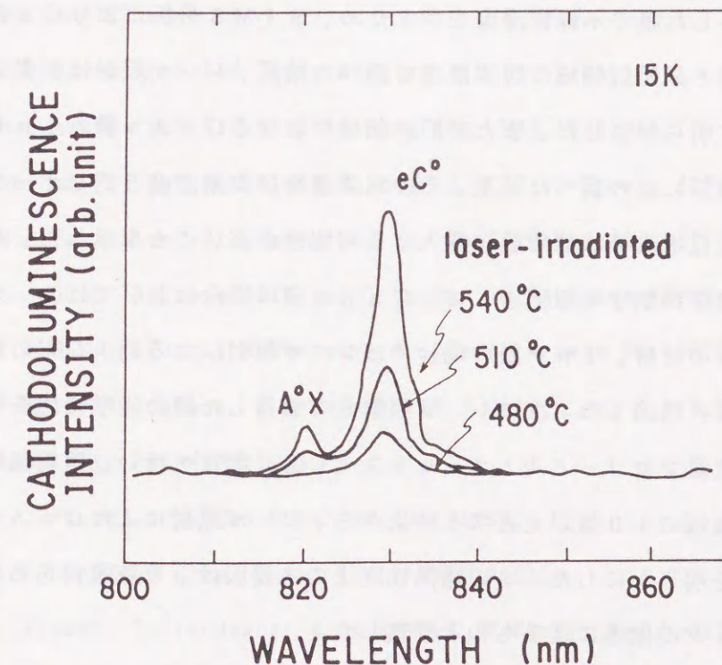
図3.28 レーザ照射領域におけるGaAs膜のCLスペクトルの基板温度依存性(レーザー強度500mW、レーザー波長514.5nm)
