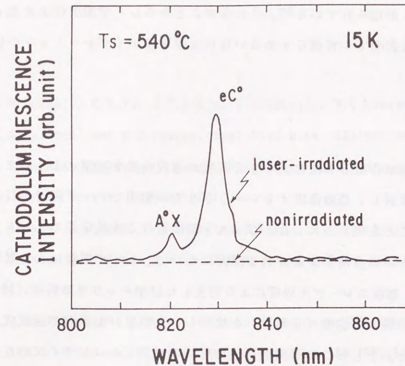
図3.27 レーザ照射領域と非照射領域におけるGaAs膜のCLスペクトル (基板温度540℃、レーザー強度500mW、レーザー波長514.5nm)
