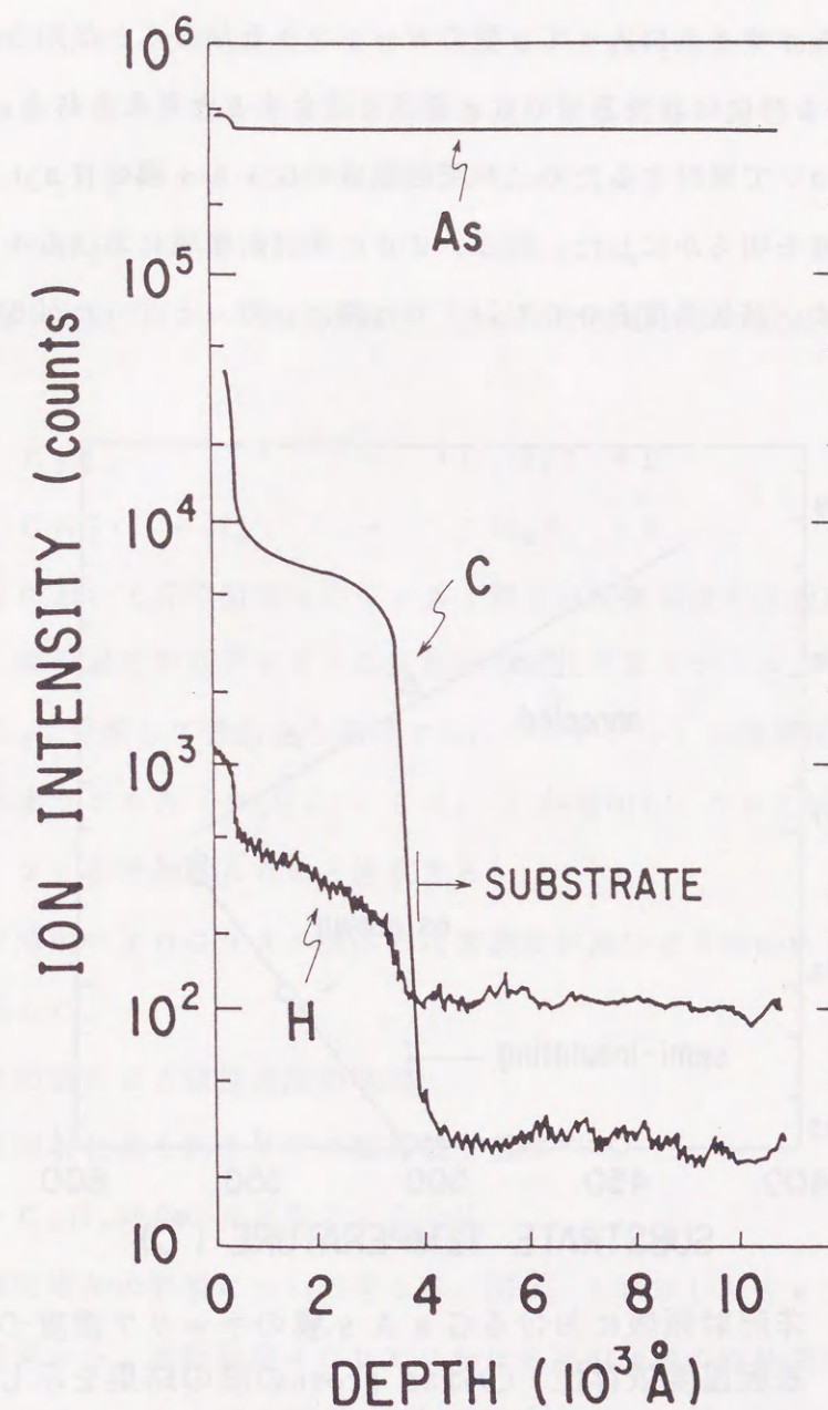
図3.19 SIMS分析による非照射領域におけるGaAs膜中の炭素イオン強度と水素イオン強度の深さ方向プロファイルの比較 (基板温度400℃) 炭素のイオン収率は、水素の約10倍。
