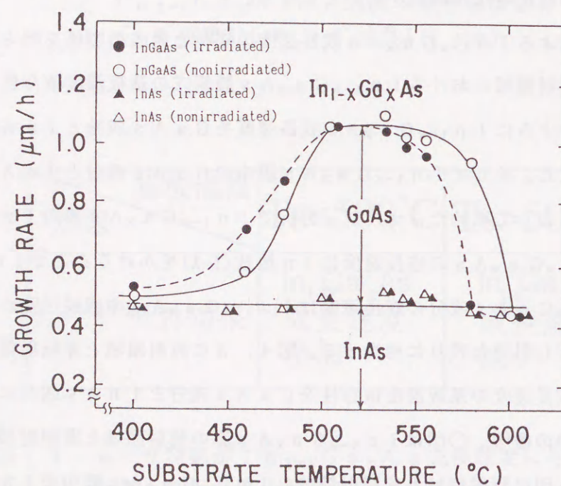
図4.3 レーザ照射領域と非照射領域における \text{In}_{1-x}\text{Ga}_x\text{As} 膜中のGaAs成分とInAs成分の成長速度の基板温度依存性 (レーザー強度500mW、レーザー波長514.5nm)
