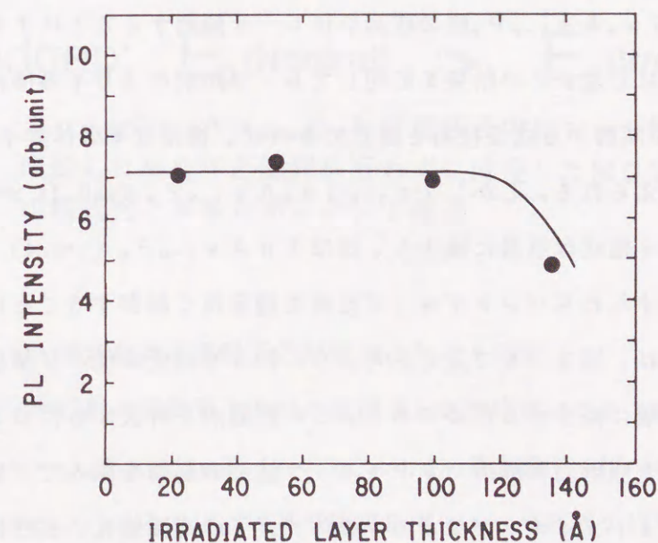
図5.12 レーザ照射のオン、オフを用いて成長した超格子のPL強度の照射層厚依存性 (基板温度 510^\circ\text{C} 、レーザ強度 5\text{W} 、レーザ波長 670\text{nm} )
