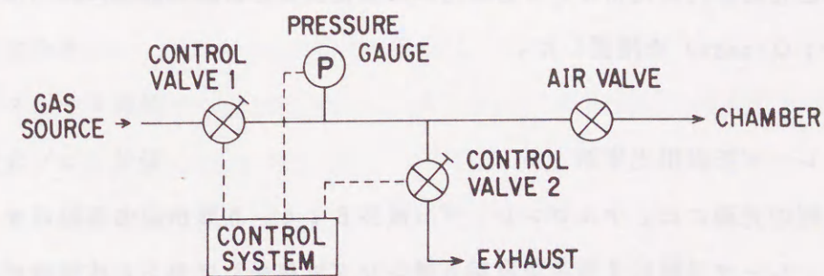
図2.2 原料ガス圧力制御系の配管図
