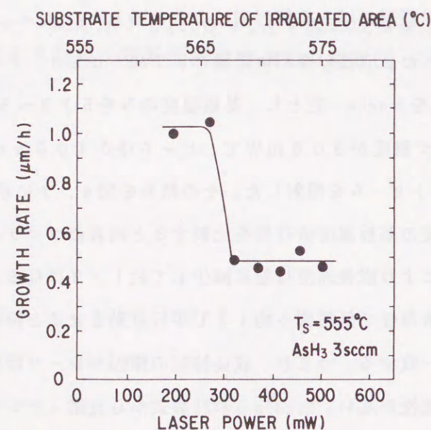
図4.8 \text{In}_{1-x}\text{Ga}_x\text{As} 成長速度のレーザ強度依存性（基板温度555℃、レーザ波長514.5nm、連続照射） 図上の横軸は、照射領域におけるレーザ強度に起因した温度上昇を含む基板温度（計算値）を示す。
