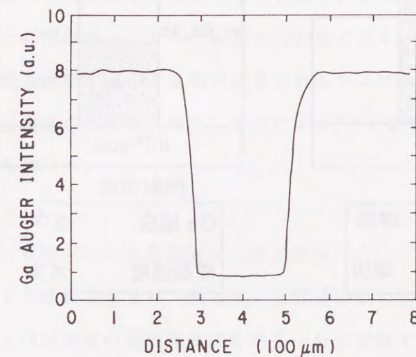
図4.5 成長抑制領域におけるGaオージェ強度の面内分布 (基板温度 580^\circ\text{C} 、レーザー強度 500\text{mW} 、レーザー波長 514.5\text{nm} )
