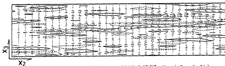
(a) 乱れ速度分布 等速度線図 \bar{u}_1 ( \delta=0.26 ) ベクトル ( \bar{u}_2', \bar{u}_3' )
