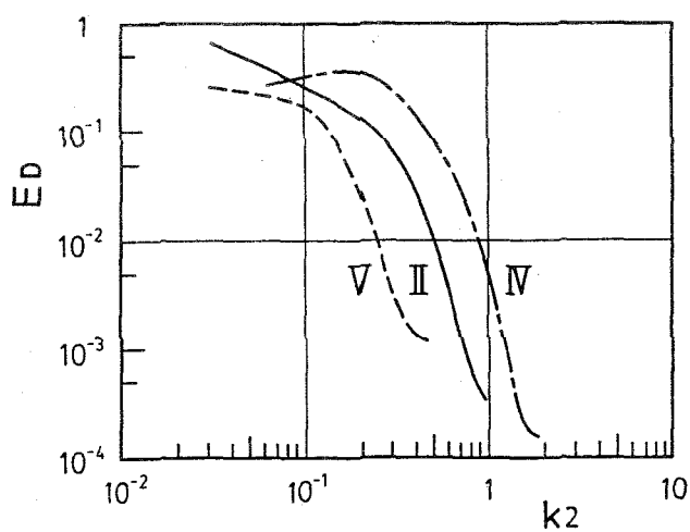
(b) 消散スペクトル
