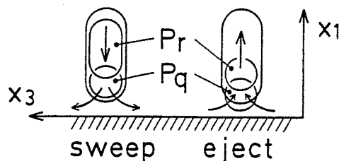
図2・20 スweepとイジェクションの構造 ( x_1 - x_3 断面内)
