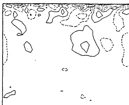
(b) 渦度 (縦渦) \bar{\omega}_2 ( \delta = 45. )
