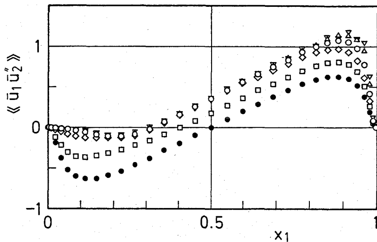
(a) 大スケール乱れの乱流せん断応力 \langle \bar{u}_1 \bar{u}_2'' \rangle
