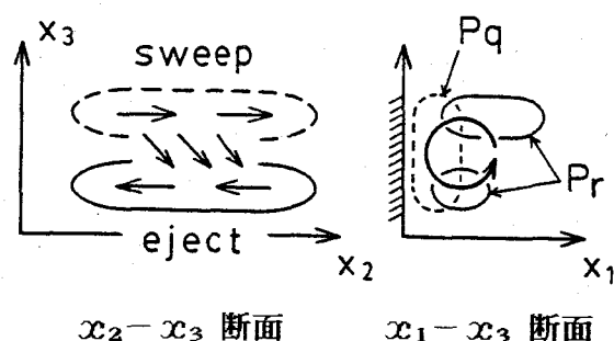
図2・21 縦渦（渦対）の構造
