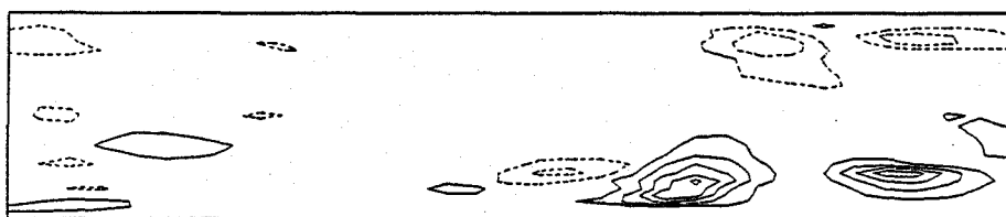
(d) レイノルズ応力 \bar{u}_1 \bar{u}_2 ( \delta = 1.5 )
