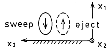
(b) スweepとイジェクション
