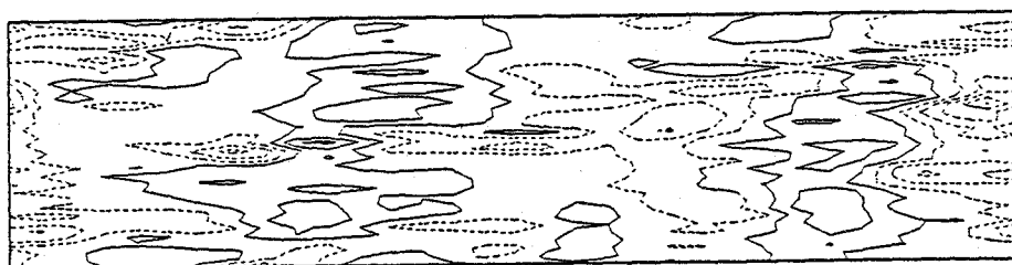
(d) 圧力 \bar{p}' ( \delta=1.41 )
