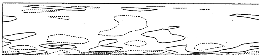
(d) 渦度 (縦渦) \bar{\omega}_2 ( \delta=45. )
