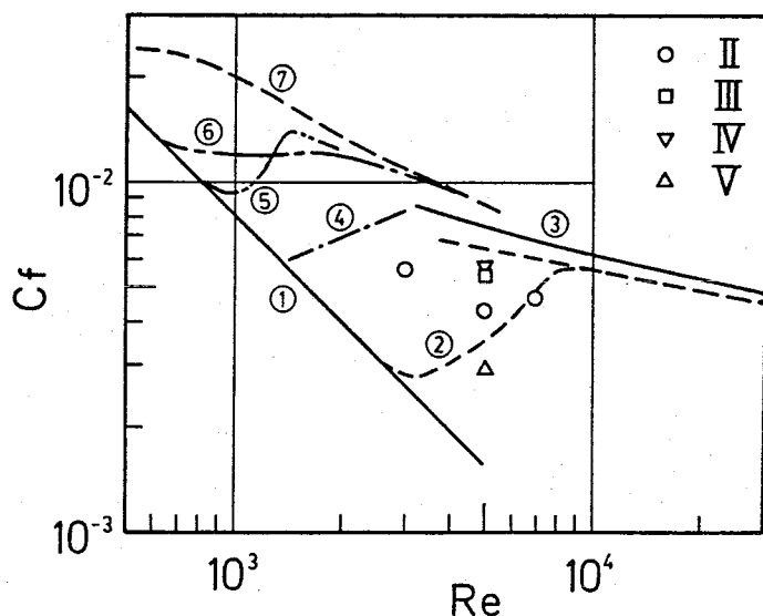
図4・6 レイノルズ数と壁面摩擦係数の関係
