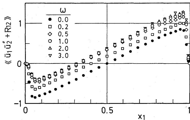
(b) 全てのスケールの乱れによる乱流せん断応力 \langle \bar{u}_1 \bar{u}_2'' + R_{12} \rangle
