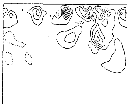
(d) レイノルズ応力 \bar{u}_1 \bar{u}_2'' ( \delta = 2.0 )
