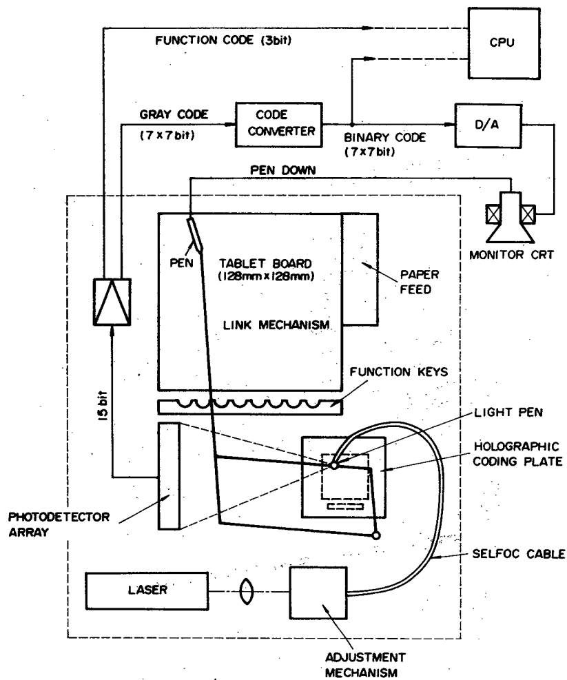
第 3.4 図 試作図形入力装置の構成。
