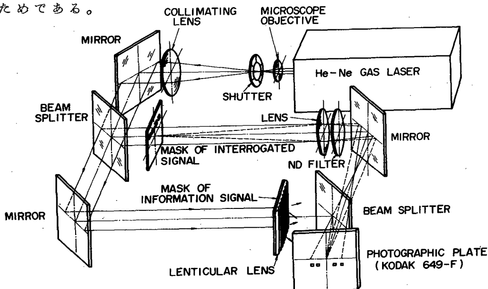
第4.7図 ホログラム連想メモリ板製作の光学配置。
