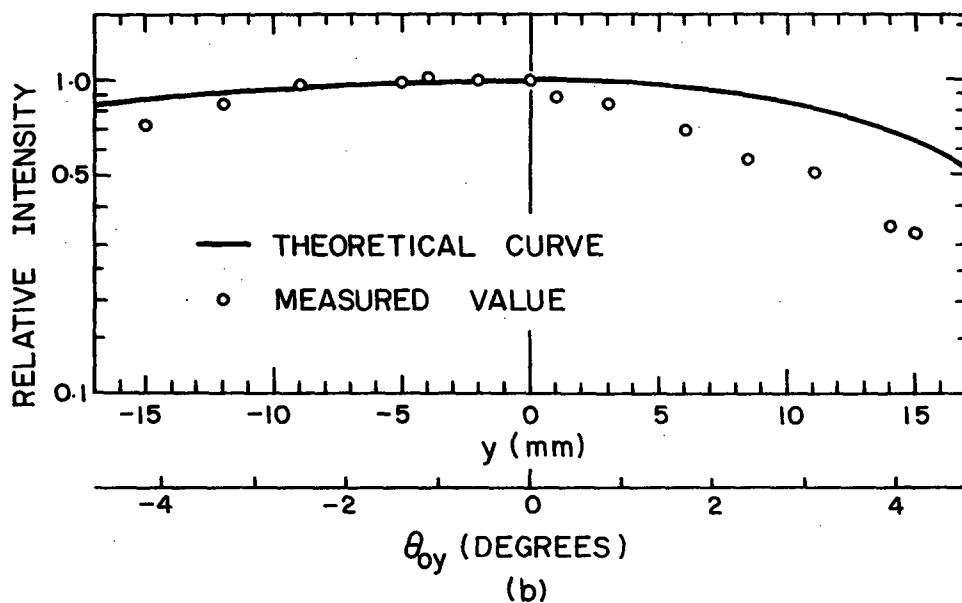
第 2・15 図 ホログラムの x = 0 の位置を直径約 1 mm のレーザー光ビームで y 方向に走査した時の \theta_{rx} = 0 なる参照光に対応する再生点像の強度変化。(a)ホログラムを逆方向照明した場合, (b)ホログラムを前側垂直照明した場合。各パラメータは次の通りである。 \lambda_o = \lambda_c = 6328 \text{ \AA} , n_e = 1.52 , L = 13.5 \mu\text{m} , \theta_{ox} = 0 , \theta_{ry} = 16.3^\circ 。
