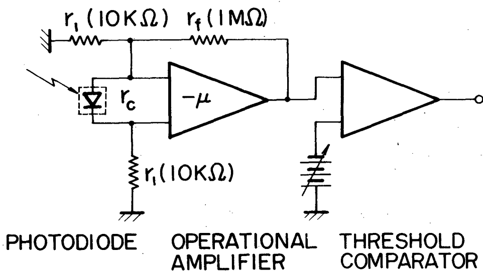
第 3.3 図 センス増幅器の回路図。
