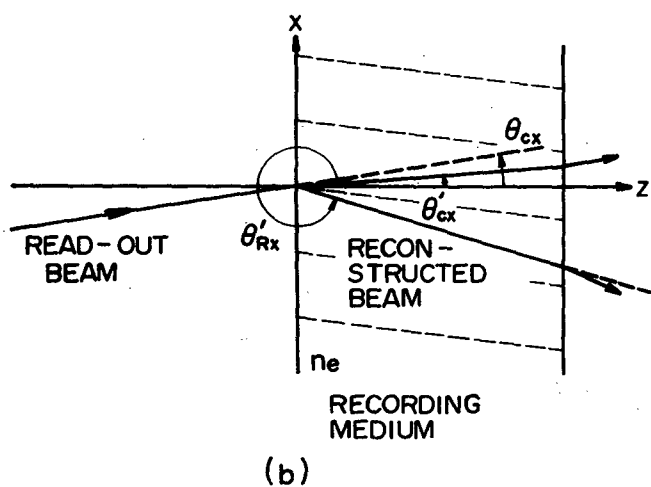
第 2・5 図 体積ホログラムの記録と読み出し。 プライムのついてゐる角度は感光材料内の値を示し、プライムのついていない角度は空気中の値を示している。(a) 記録過程、(b) 読み出し過程。
