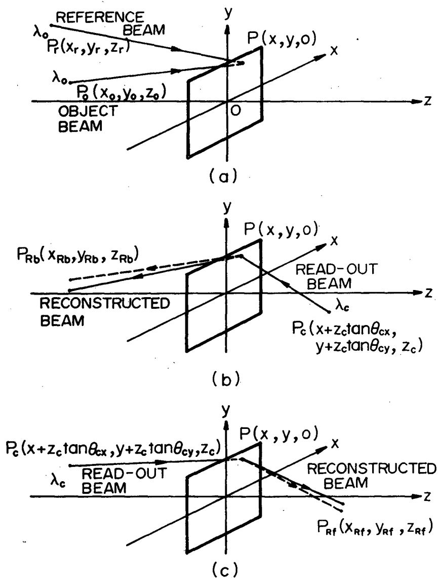
第 2・4 図 多重記録ホログラム・メモリ板の記録および読み出しにおける座標関係。(a) 多重記録ホログラム・メモリ板の記録。(b) メモリ板を後側(右側)から照明した場合の読み出し。(c) メモリ板を前側(左側)から照明した場合の読み出し。
