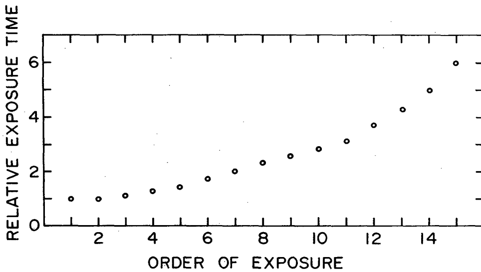
第 2・9 図 露光の順番による再生像強度変化を補償するために用いた露光の順番と露光時間の関係。
